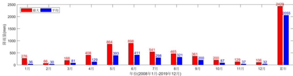
图 6.1-2 台山海洋站各月平均及最大、最小降水量统计分布图
