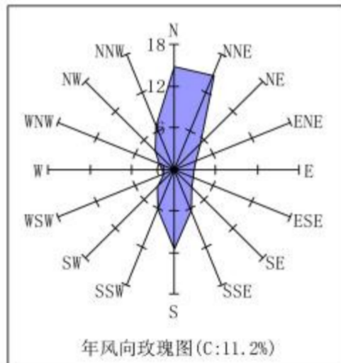
图 6.1-4 台山气象站风玫瑰图 (1995~2014)
