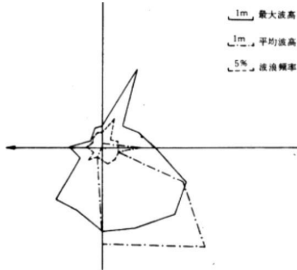
图 6.1-10 工程海区附近铜鼓站波浪玫瑰图
