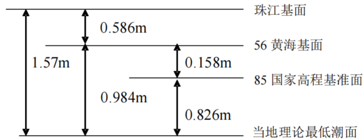
图 6.1-5 工程各基面换算关系示意图
