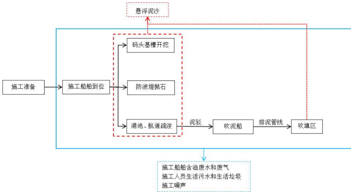
图 5.1-1 主要施工工艺流程及产污环节示意图
