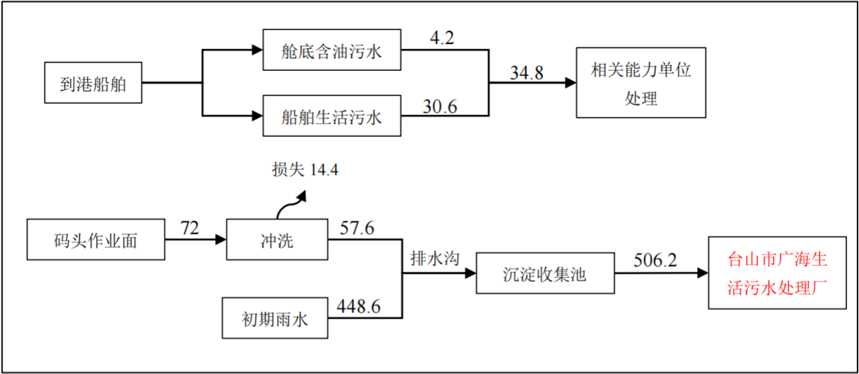
图 5.2-1 营运期水平衡图 (单位: t/d, 初期雨水为 t/次)
