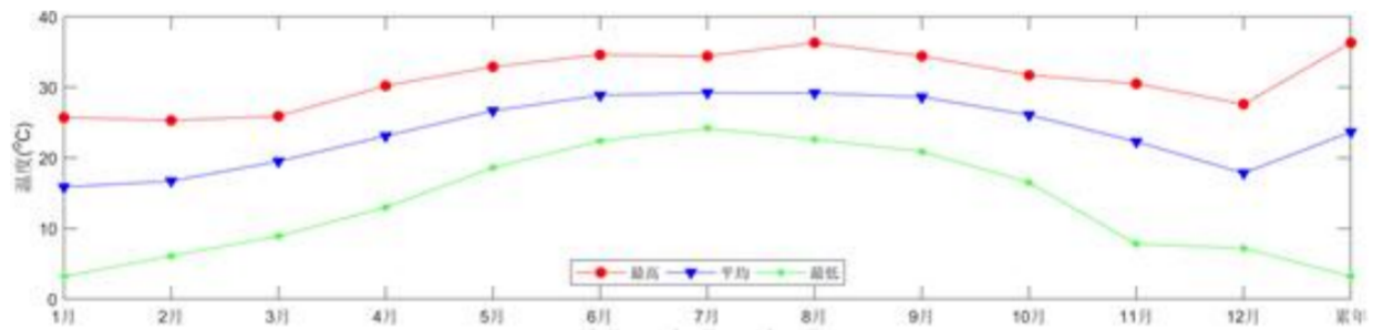
图 6.1-1 台山海洋站平均最高、最低气温月份统计曲线图
