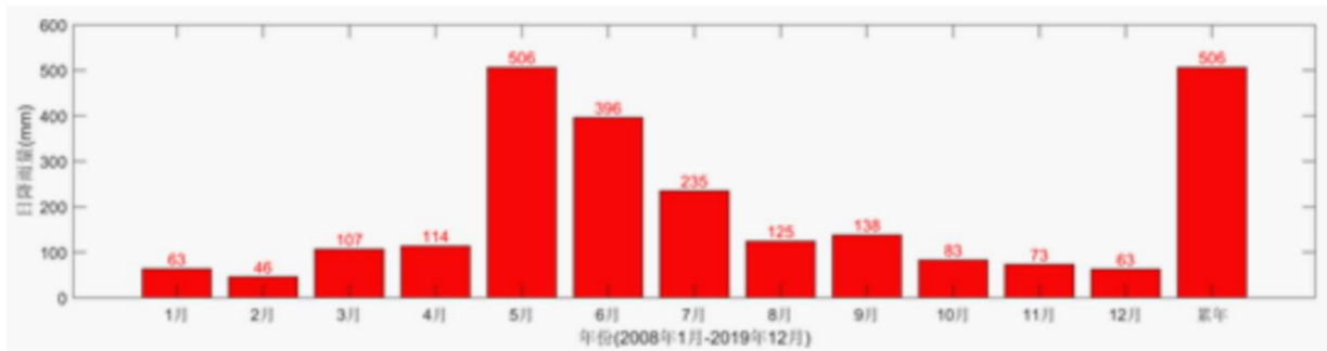
图 6.1-3 台山海洋站日最大降水量月份及累年统计直方图
