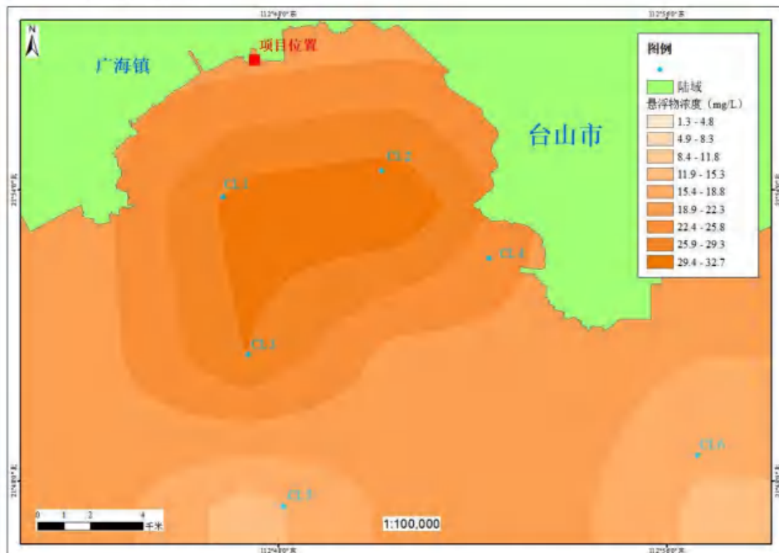
图 6.4-15 本次观测站点附近悬沙平均浓度范围渲染图
