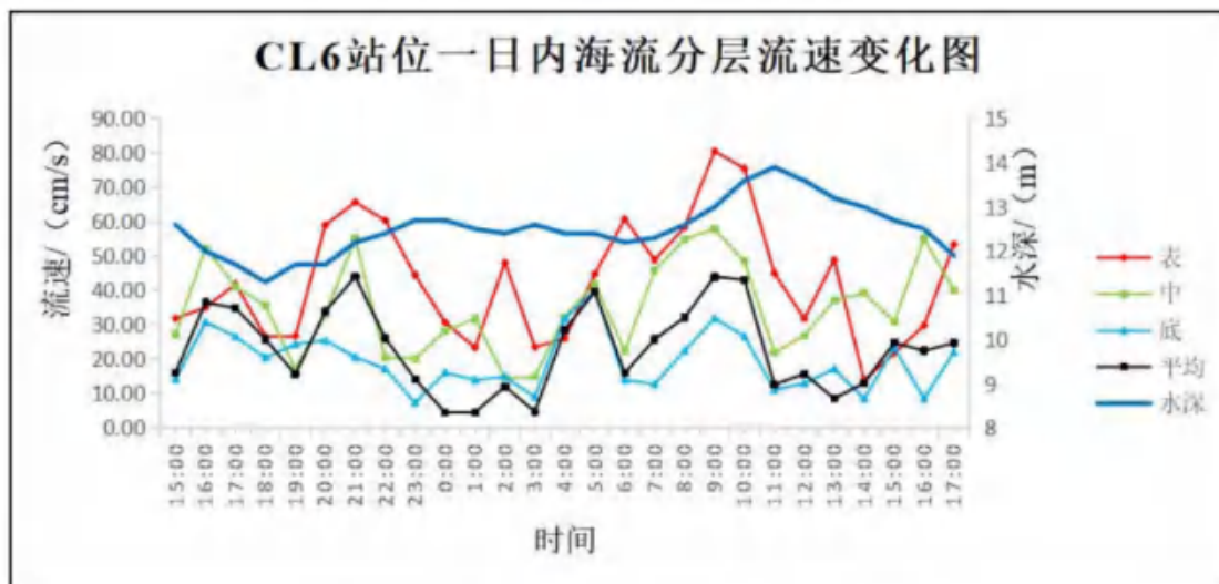
图 6.4-12 CL6 站位海流分层流速变化图
