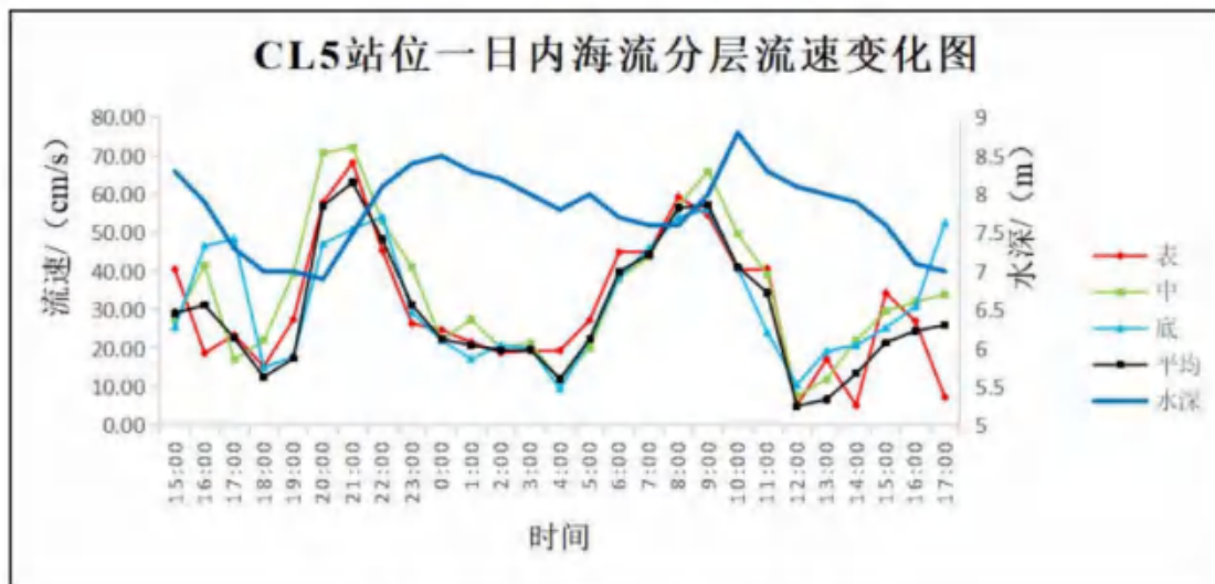
图 6.4-11 CL5 站位海流分层流速变化图
