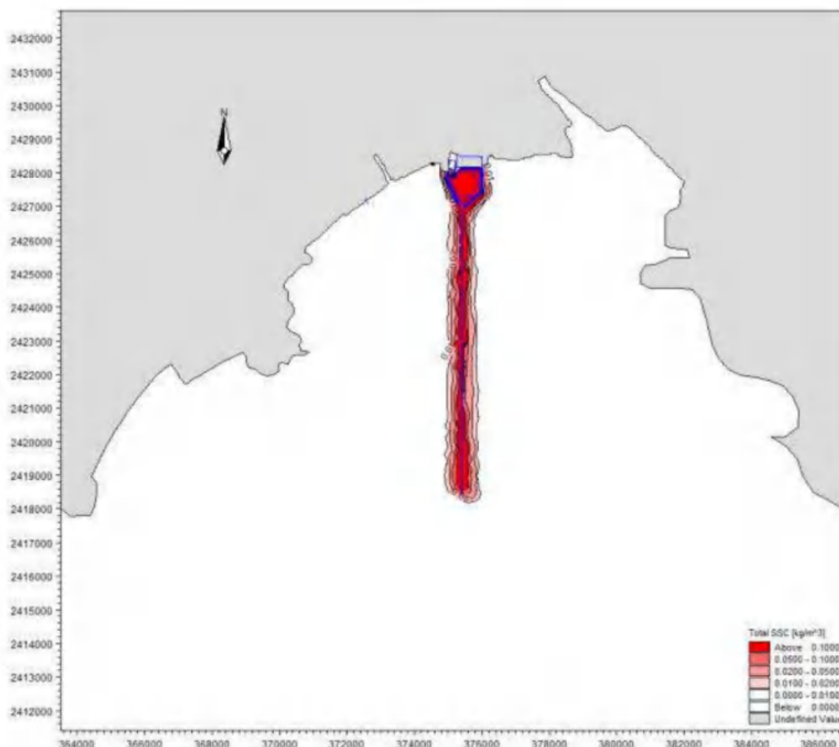
图 7.8-2 叠加各模拟工况施工悬沙增量包络线浓度图
