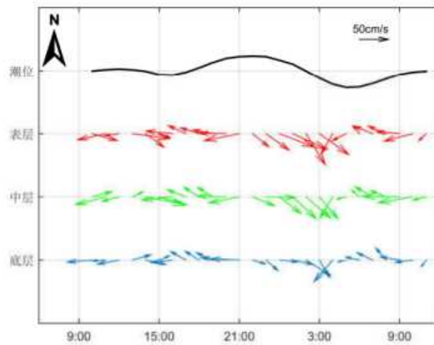
图 6.4-19 调查海域大潮 CL2 站实测海流矢量图
