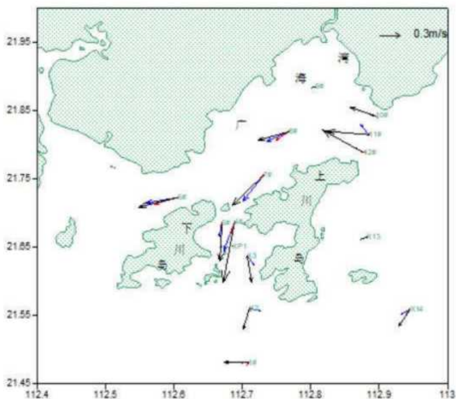
图 6.1-8 夏季小潮期表、中、底三层余流矢量（黑色：表层，蓝色：中层，红色：底层）
