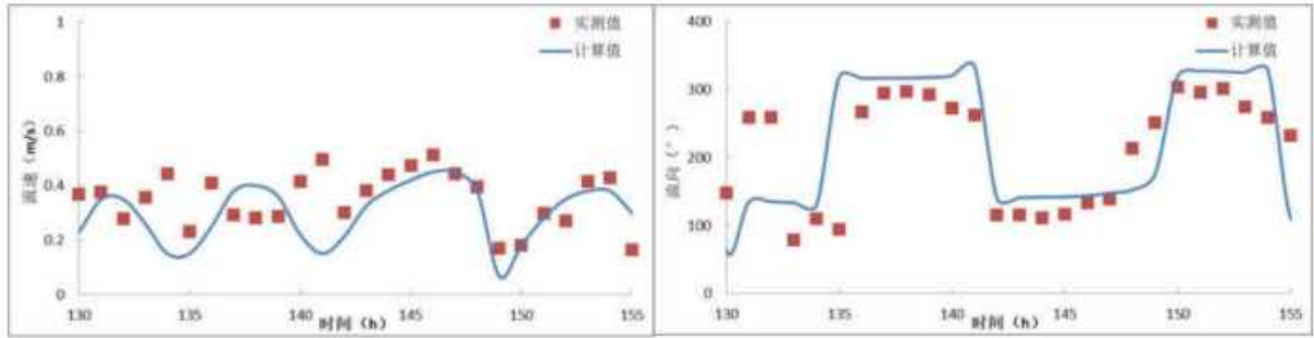
图 7.1-7 CL2 站流速、流向验证
