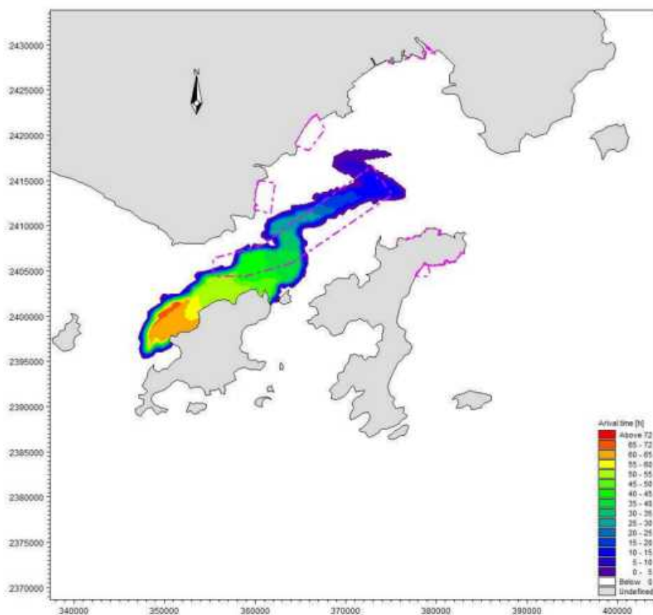
图 8.4-8 工况 7 溢油扫海范围 (72 时)
