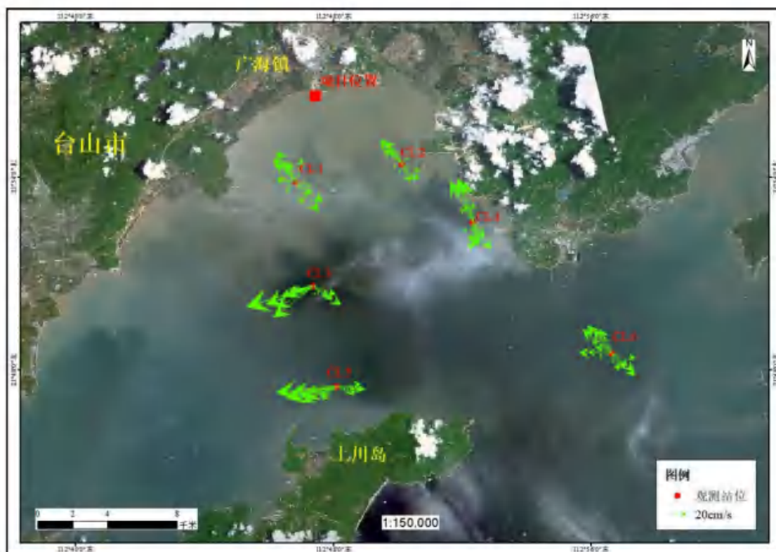
图 6.4-6 观测期间各站表、中、底 3 层平均海流矢量图
