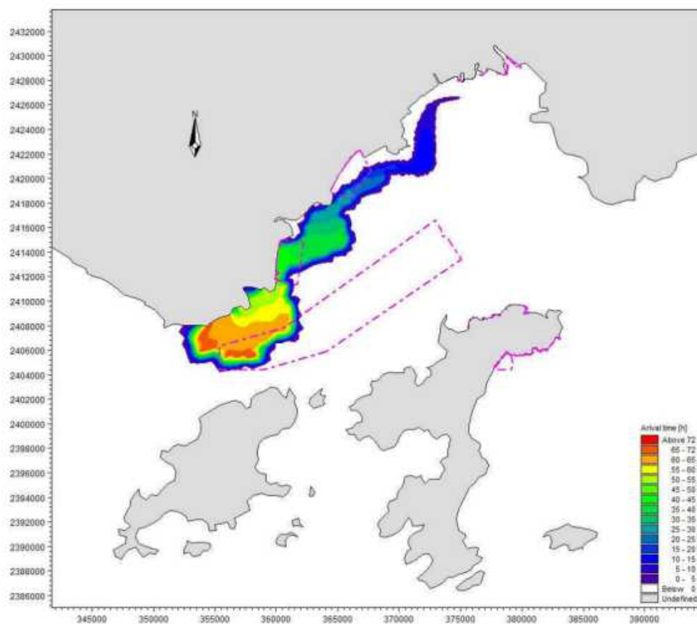
图 8.4-2 工况 1 溢油扫海范围 (72 时)
