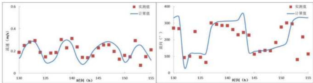
图 7.1-6 CL1 站流速、流向验证
