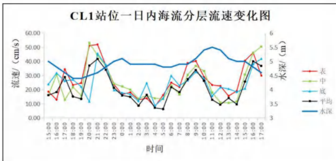
图 6.4-7 CL1 站位海流分层流速变化图
