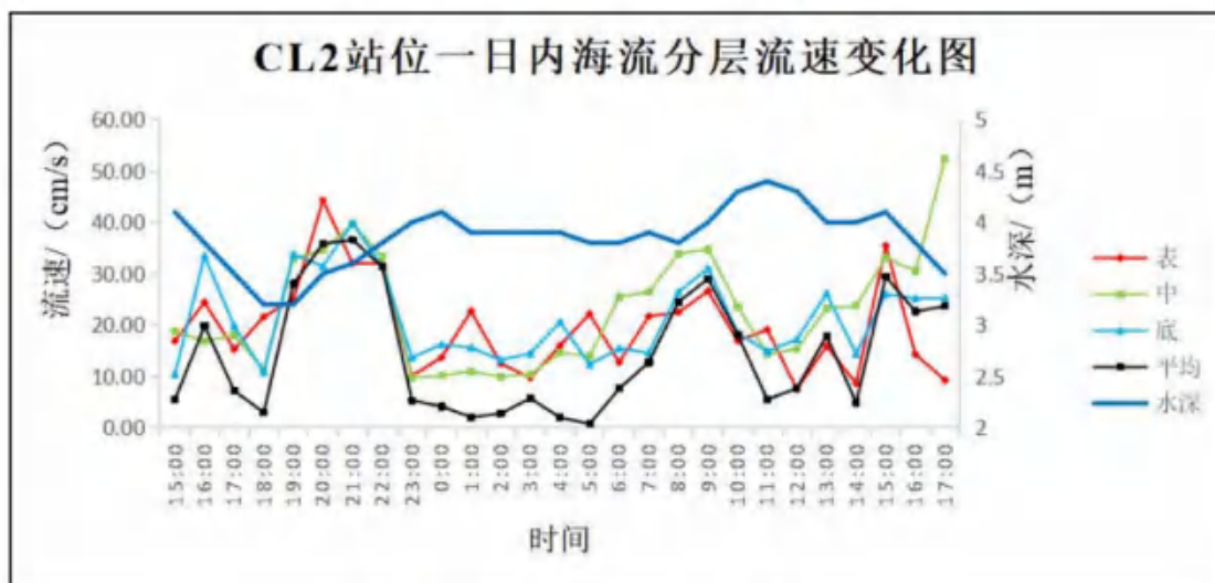
图 6.4-8 CL2 站位海流分层流速变化图
