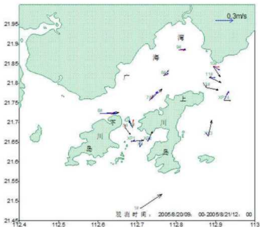
图 6.1-7 夏季大潮期表、中、底三层余流矢量（黑色：表层，蓝色：中层，红色：底层）
