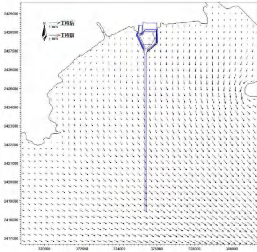
图 7.1-17 工程前后落急流场叠加图
