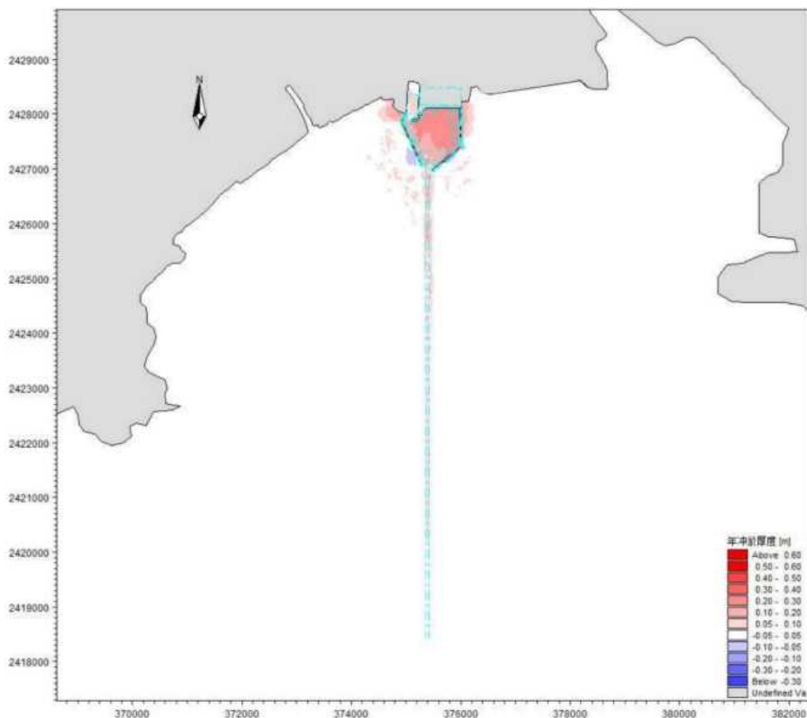
图 7.7-2 48 小时港池及航道淤淤量
