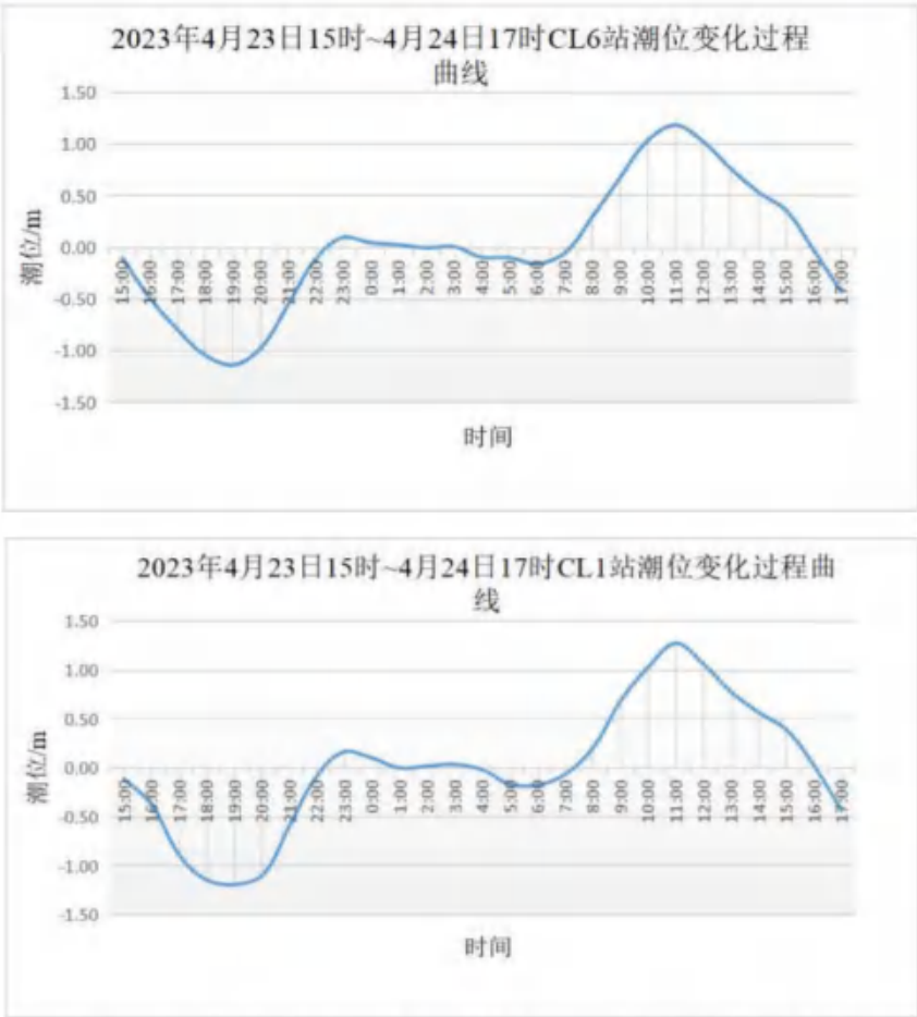
图 6.4-2 广海湾附近海域 CL1 站和 CL6 站的潮位过程曲线
