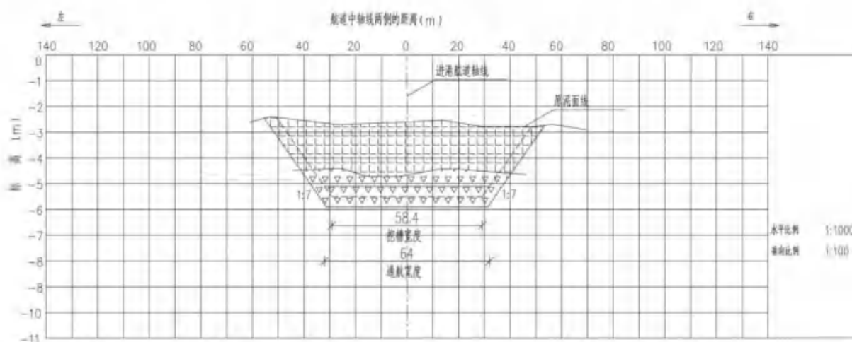
图 4.4-15 航道疏浚断面示意图
