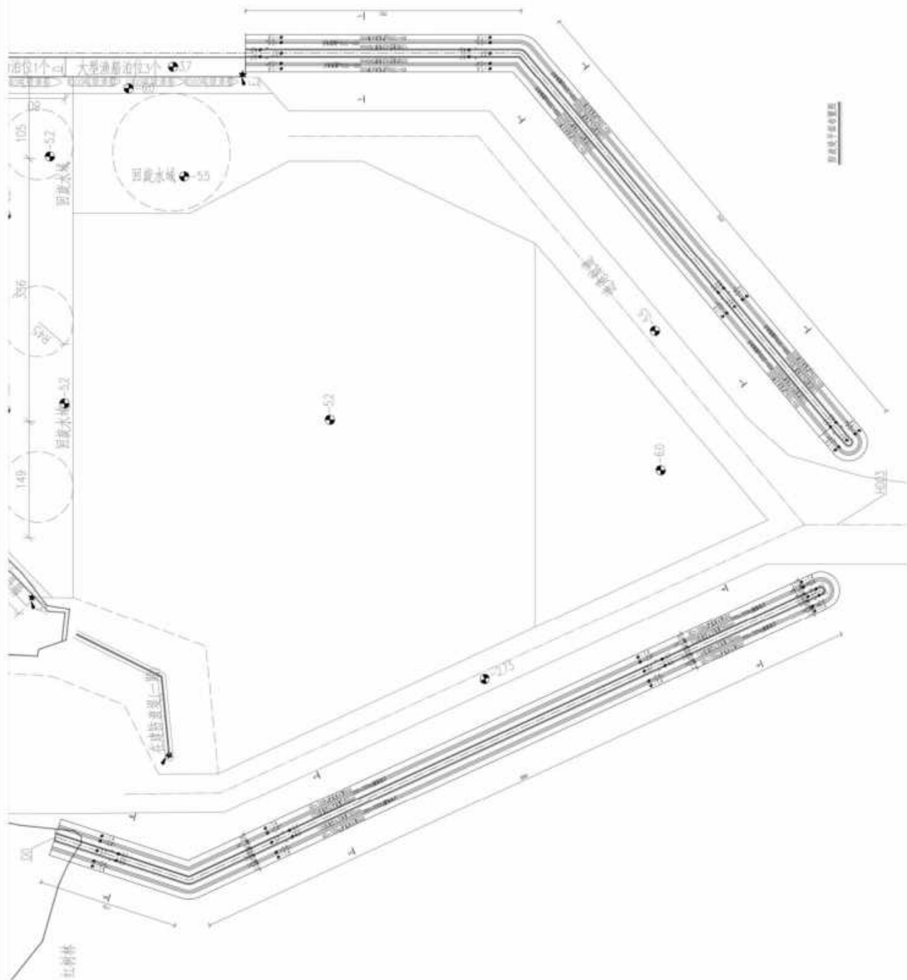
图 4.4-11 西防波堤及东防波堤结构平面图
