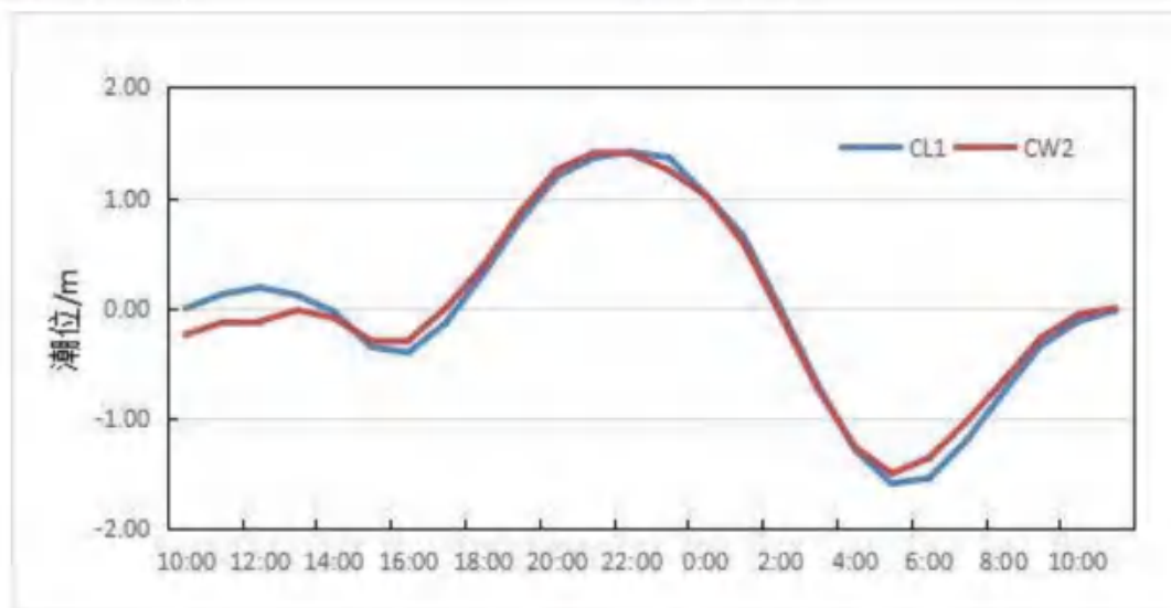
图 6.4-17 广海湾附近海域 CL1 站和 CW2 站的潮位过程曲线
