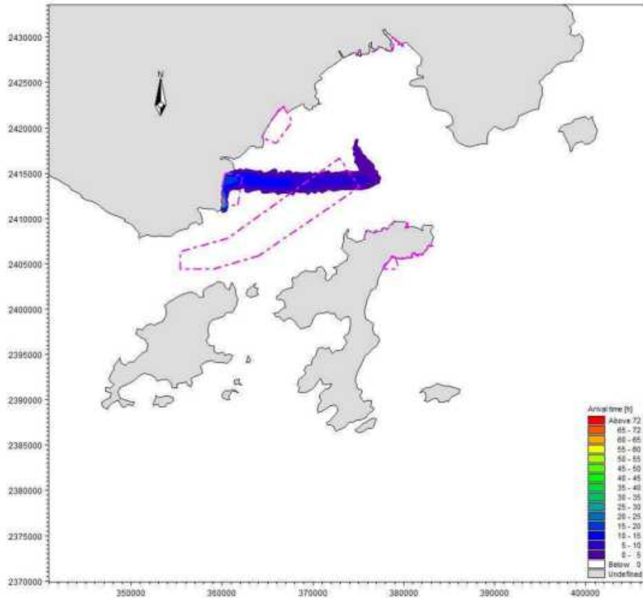
图 8.4-13 工况 12 溢油扫海范围（72 时）
