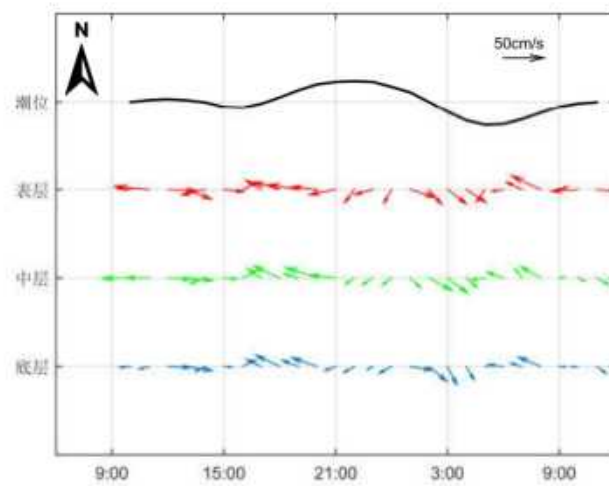
图 6.4-18 调查海域大潮 CL1 站实测海流矢量图
