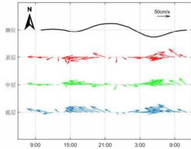
图 6.4-22 调查海域大潮 CL5 站实测海流矢量图
