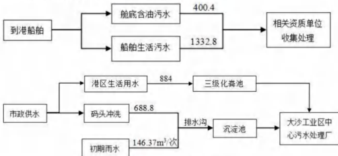
图 3.4-2 现有工程水平衡图
