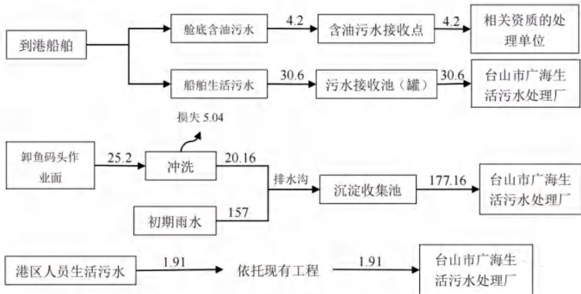
图 5.2-1 项目水平衡图（单位：t/d，初期雨水为 t/次）
