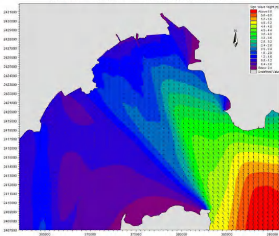
图 7.6-3 工程前 50 年一遇 SSE 向有效波高分布图
