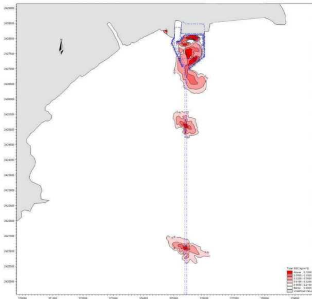
图 7.8-4 典型工况 2 的典型代表点施工悬沙扩散范围
