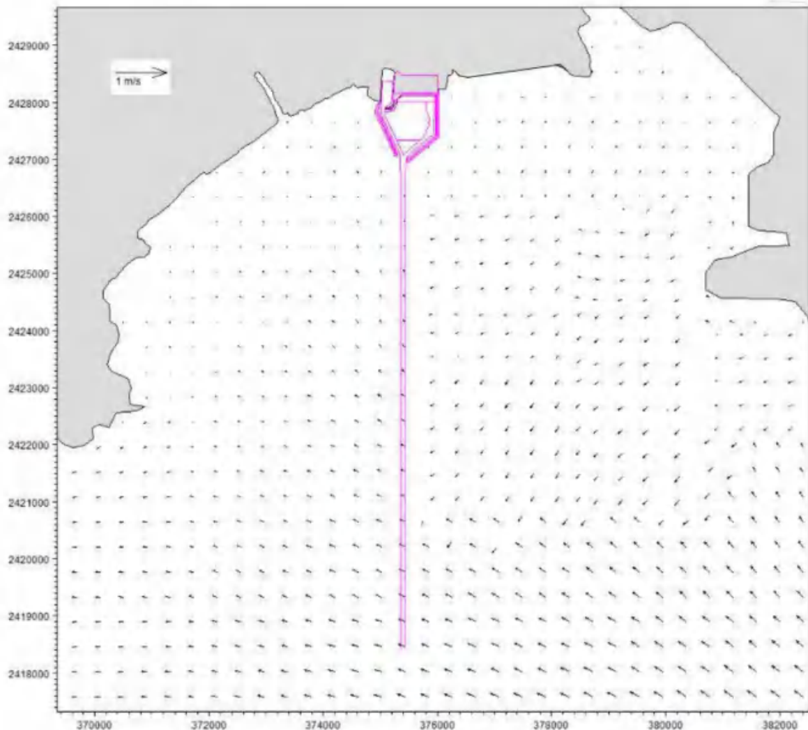
图 7.5-1 项目周边余流图
