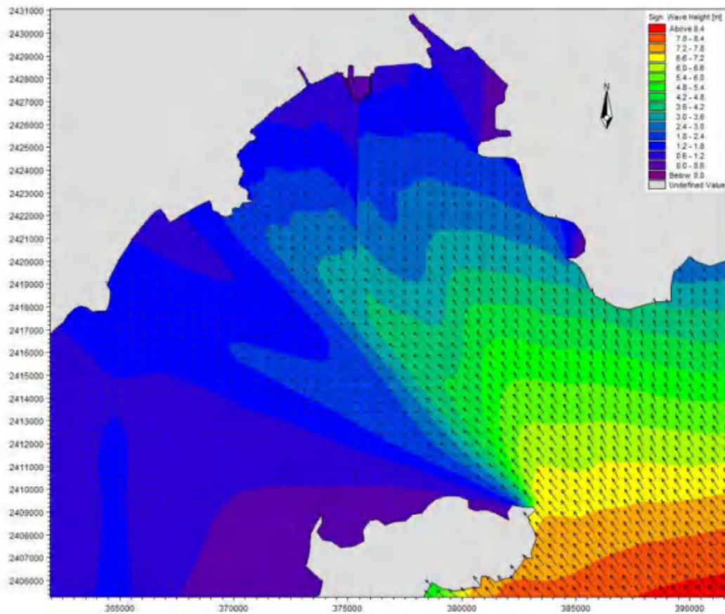
图 7.6-6 工程后 50 年一遇 SE 向波高分布图
