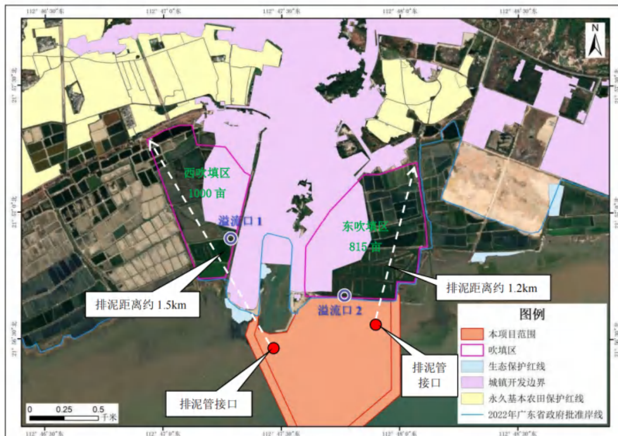
图 4.4-16 吹填区位置示意图
