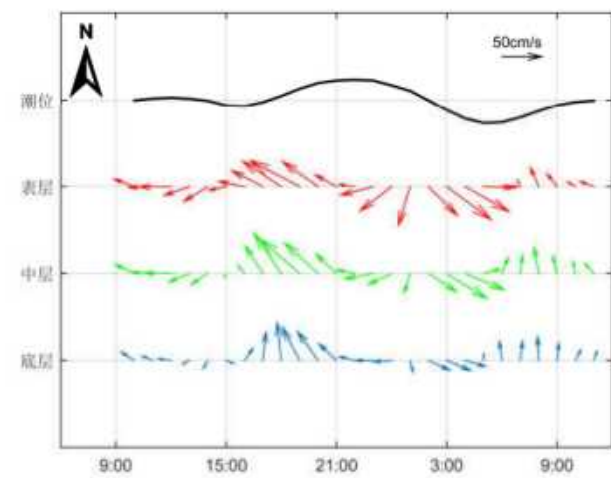
图 6.4-23 调查海域大潮 CL6 站实测海流矢量图
