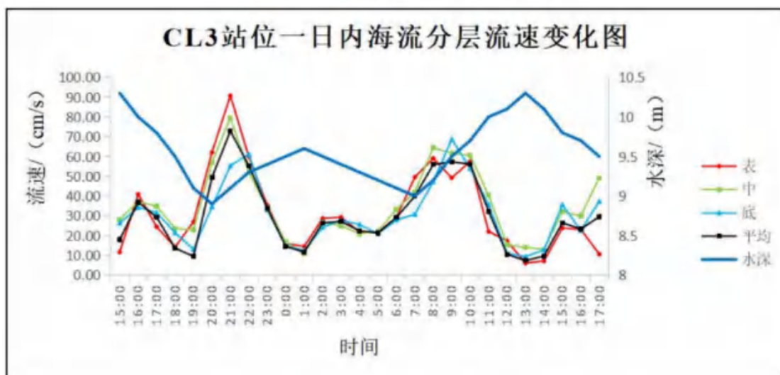
图 6.4-9 CL3 站位海流分层流速变化图
