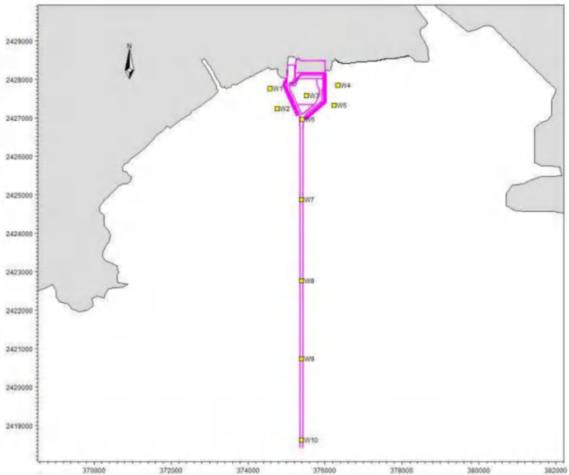
图 7.6-5 波浪代表点分布图
