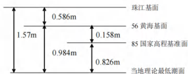
图 6.1-5 工程各基面换算关系示意图
