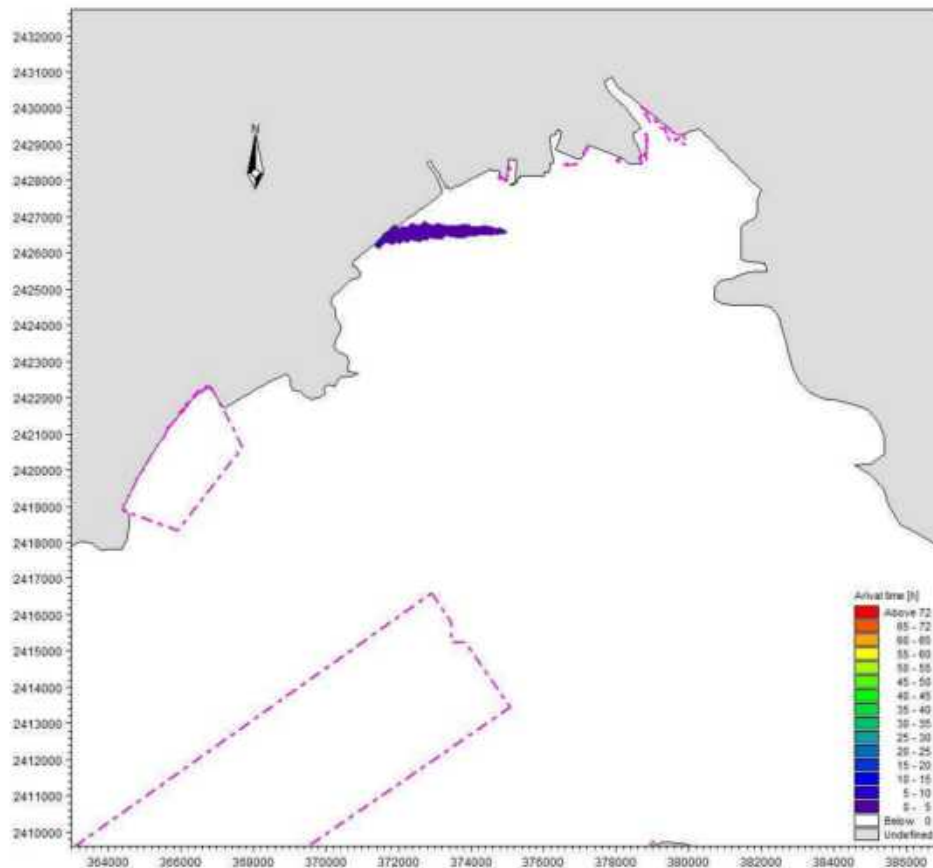
图 8.4-6 工况 5 溢油扫海范围 (72 时)
