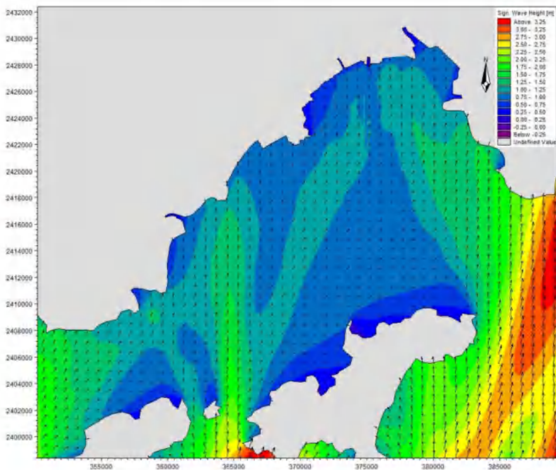
图 7.6-4 工程前 50 年一遇 SW 向有效波高分布图
