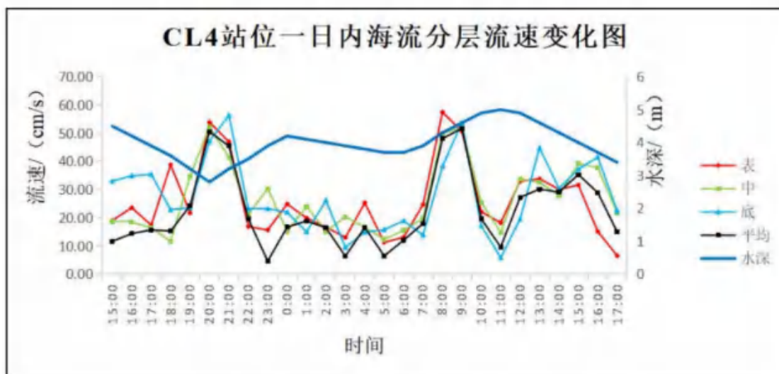
图 6.4-10 CL4 站位海流分层流速变化图
