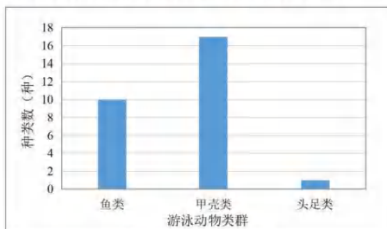
图 6.6-10 游泳动物类群组成
