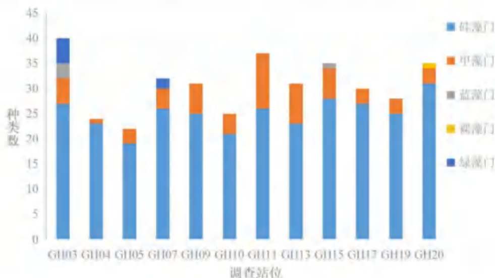
图 6.6-13 调查海域浮游植物种类数空间分布
