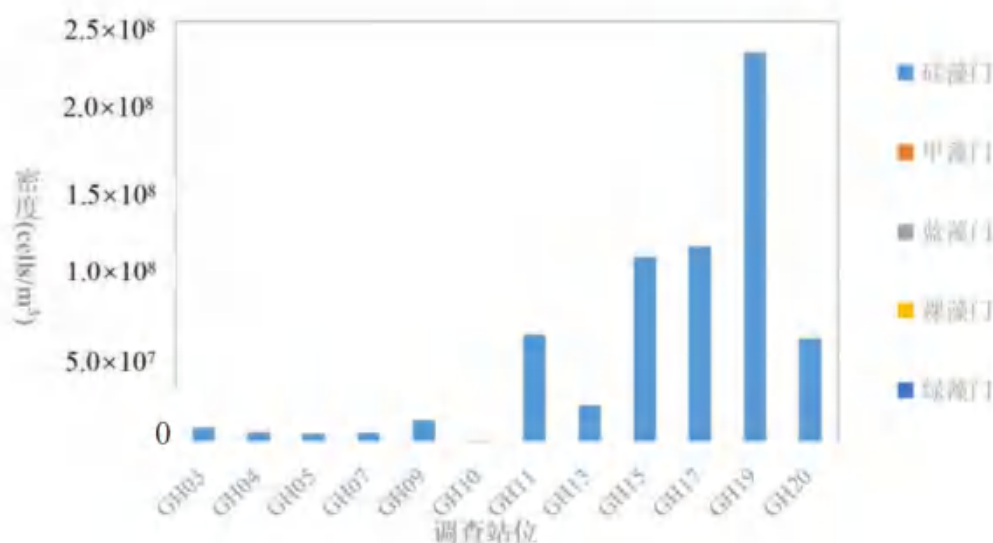
图 6.6-14 调查海域浮游植物密度分布图
