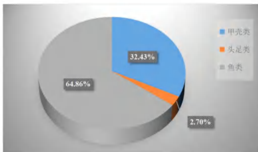
图 6.6-22 游泳动物种类组成图
