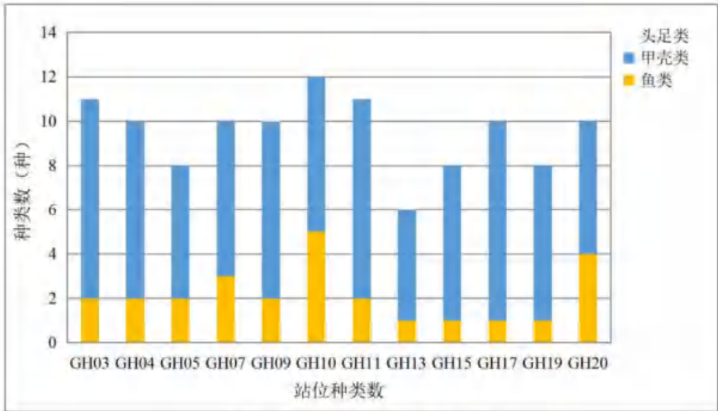
图 6.6-11 游泳动物种类空间分布
