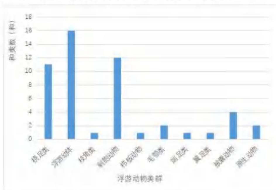
图 6.6-3 调查海域浮游动物类群组成情况
