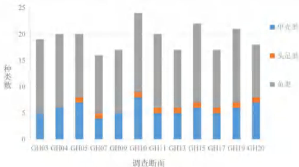
图 6.6-23 游泳动物种类分布图
