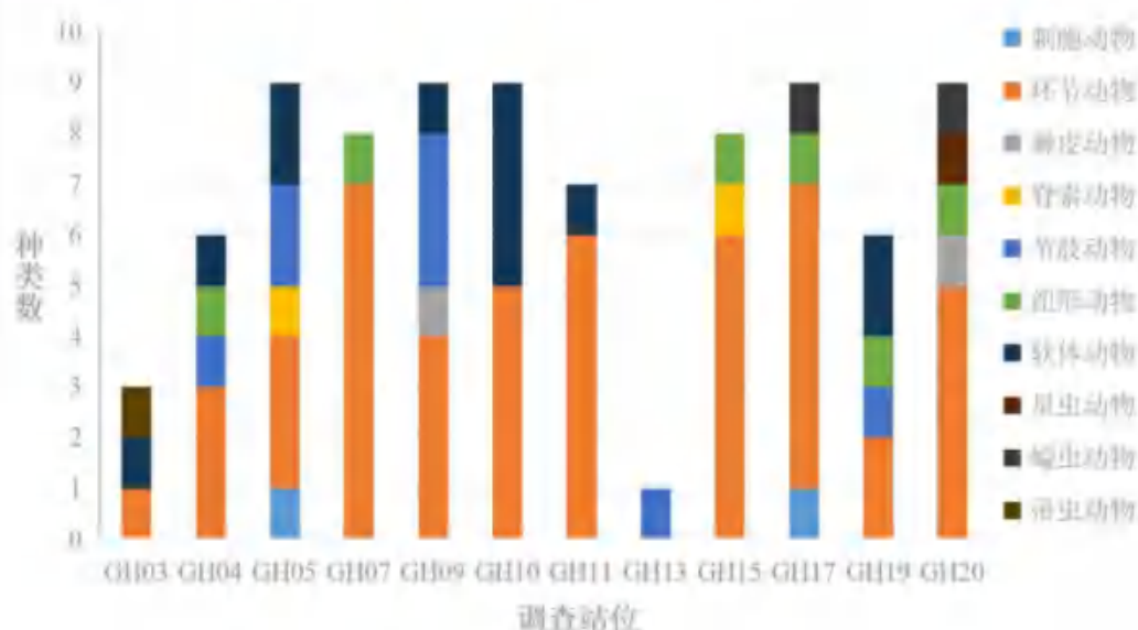
图 6.6-19 调查海域大型底栖生物种类组成的空间分布
