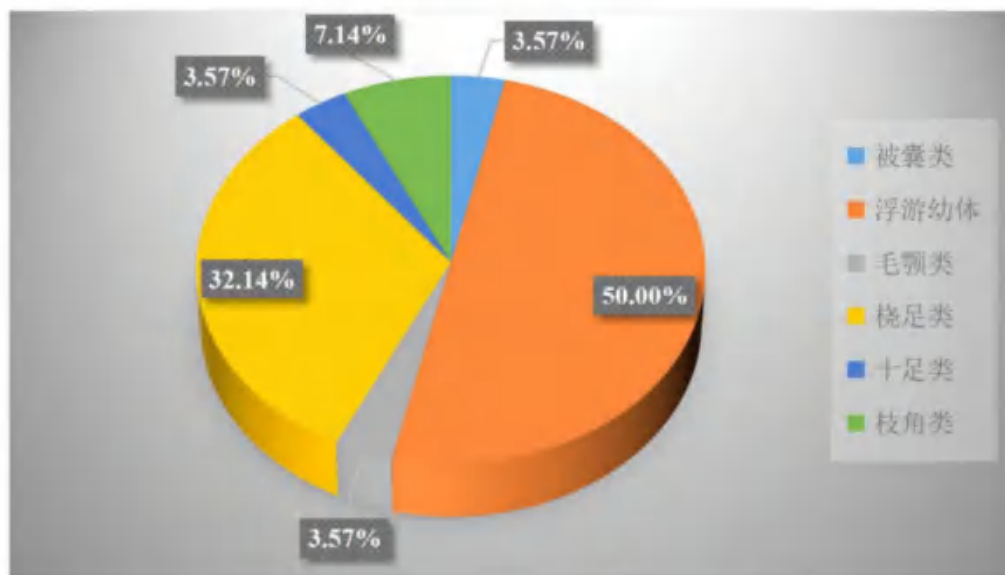
图 6.6-15 调查海域浮游动物类群组成
