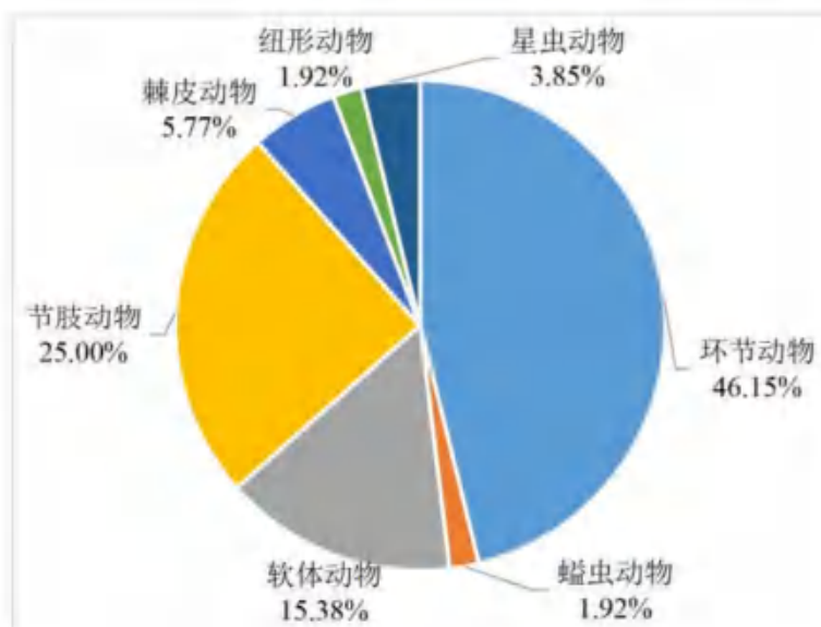
图 6.6-4 大型底栖生物种类组成
