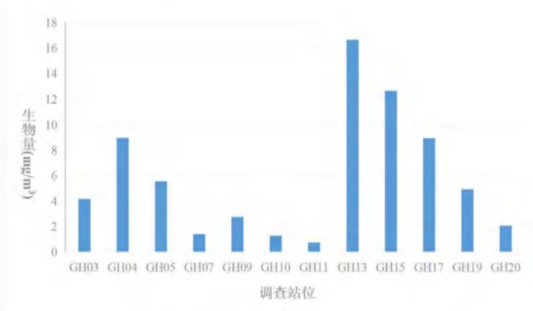
图 6.6-17 调查海域浮游动物生物量空间分布
