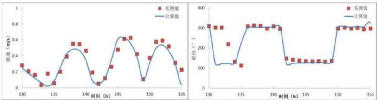
图 7.1-9 CL4 站流速、流向验证
