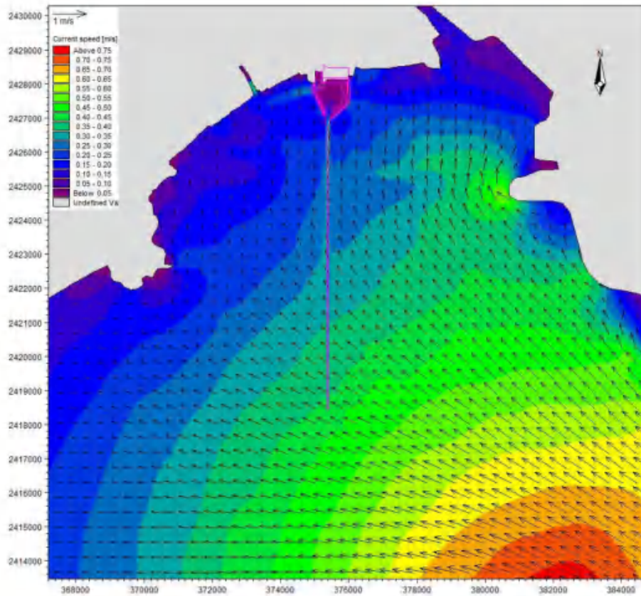
图 7.1-15 工程后涨急流场图
