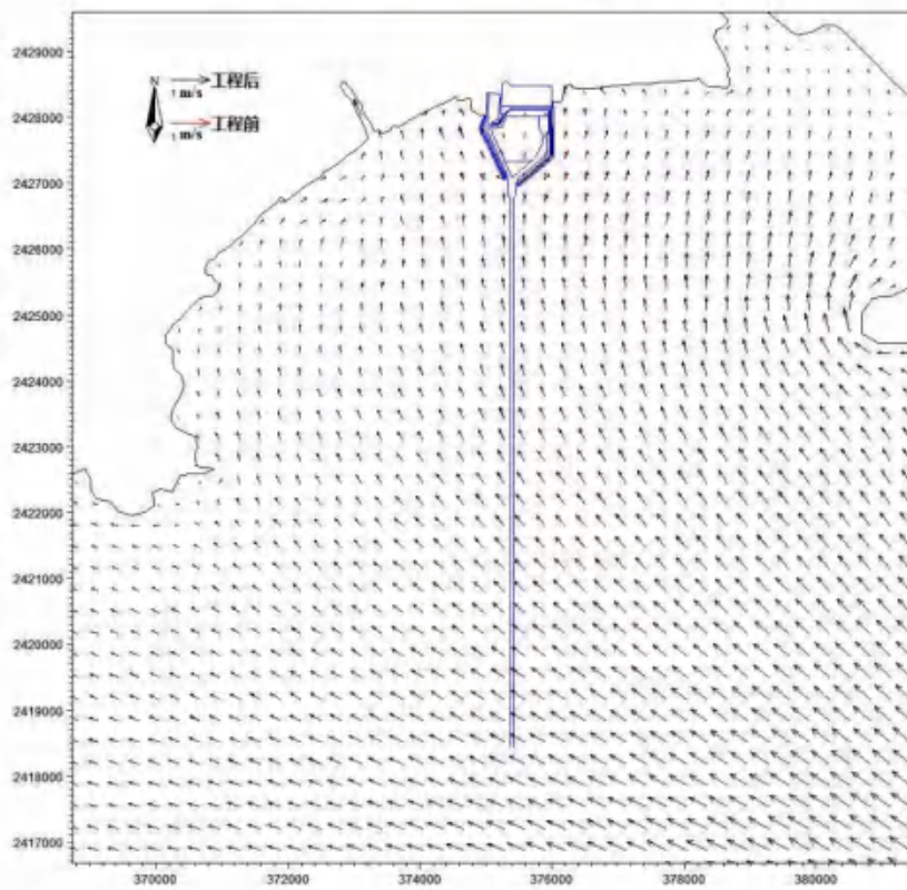
图 7.1-18 工程前后涨急流场叠加图
