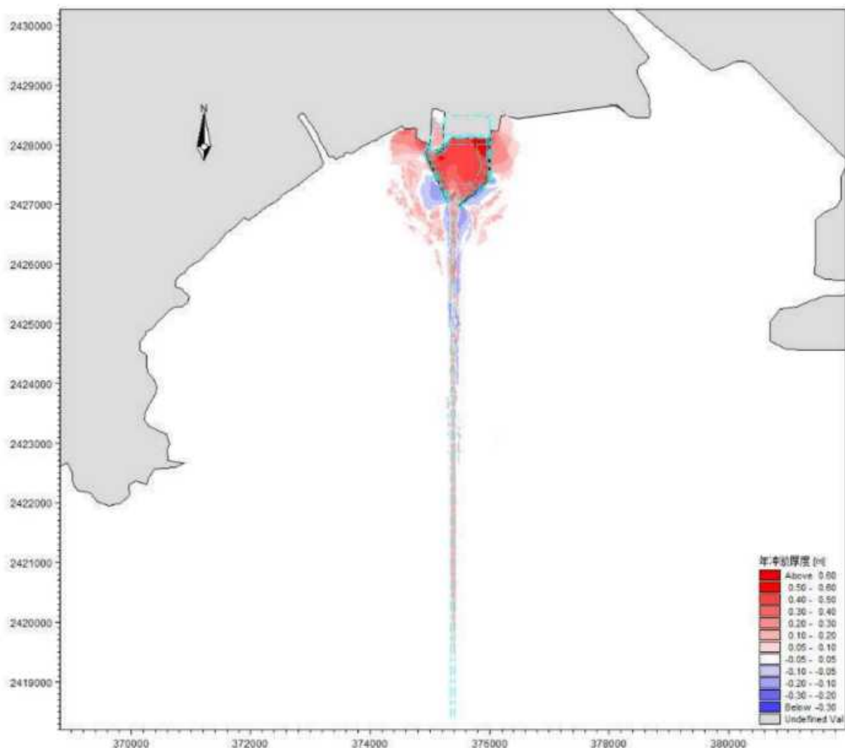
图 7.7-1 工程实施后年冲淤变化图
