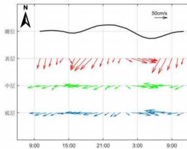
图 6.4-20 调查海域大潮 CL3 站实测海流矢量图
