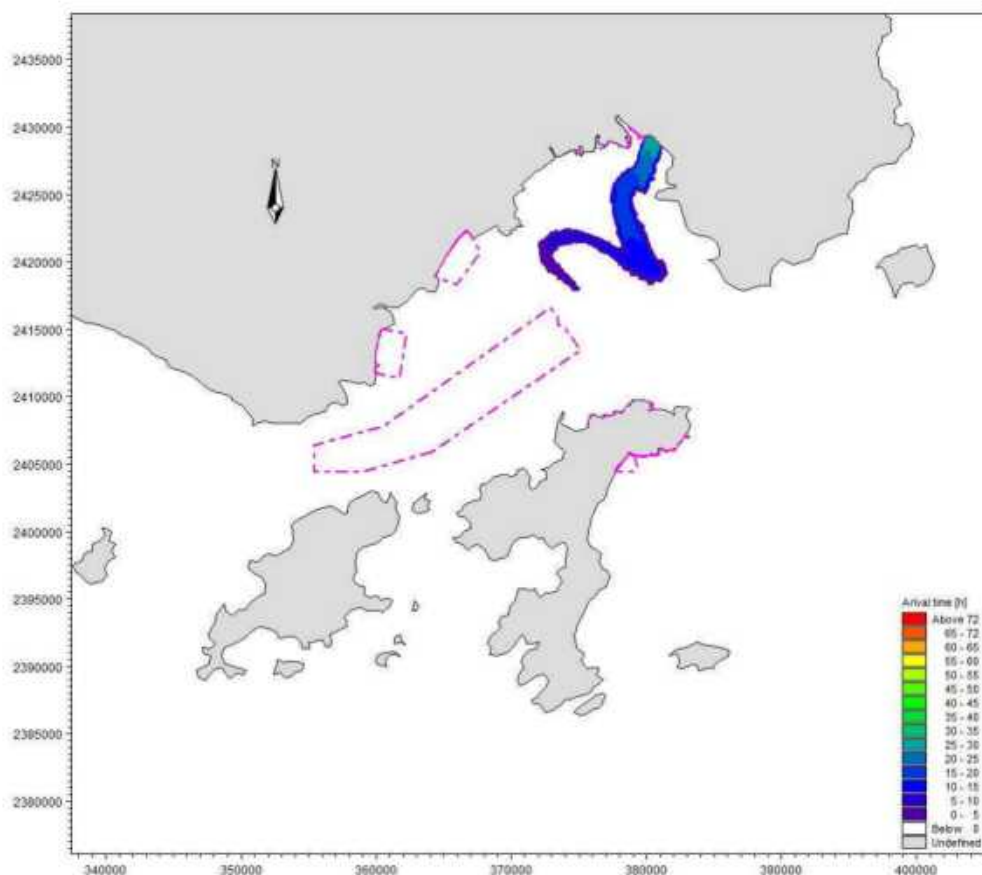
图 8.4-10 工况 9 溢油扫海范围 (72 时)
