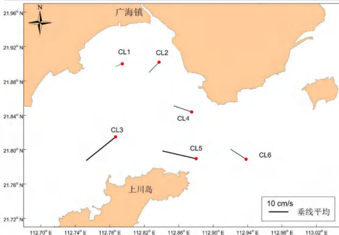
图 6.4-25 大潮期各站垂线平均余流图
