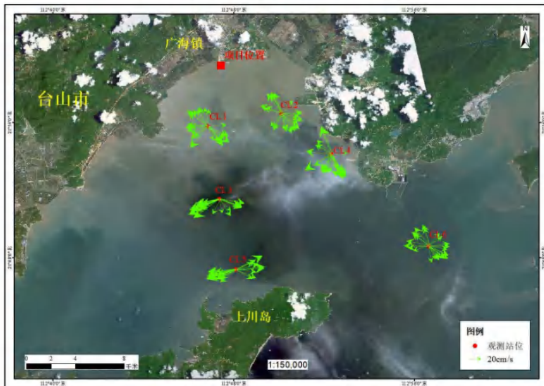
图 6.4-5 观测期间各站底层 (0.8h) 海流矢量图
