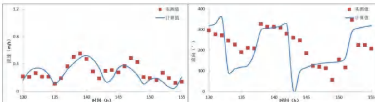
图 7.1-11 CL6 站流速、流向验证
