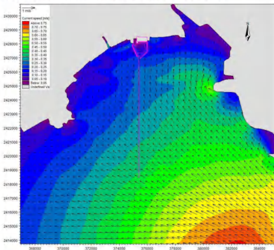
图 7.1-12 工程前工程海域涨急流场
