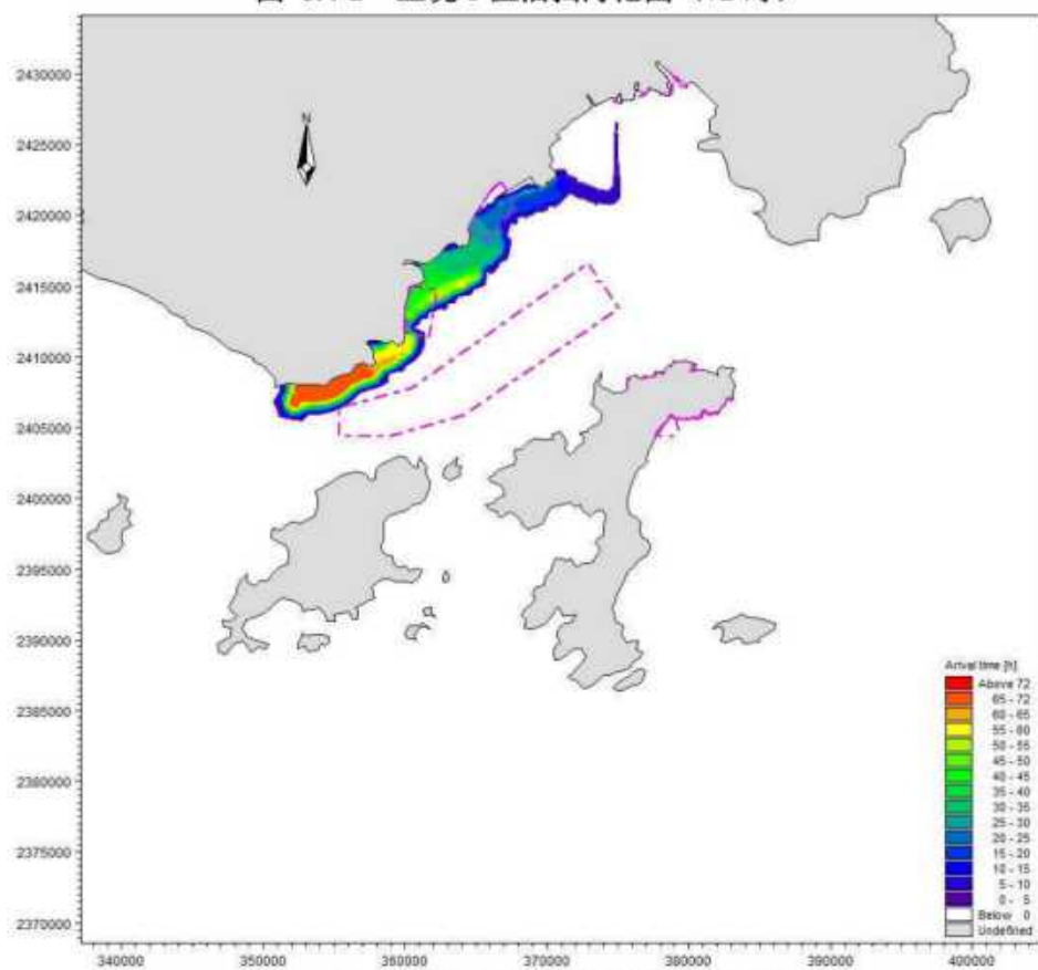
图 8.4-3 工况 2 溢油扫海范围 (72 时)
