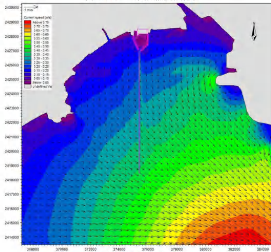
图 7.1-16 工程后落急流场图
