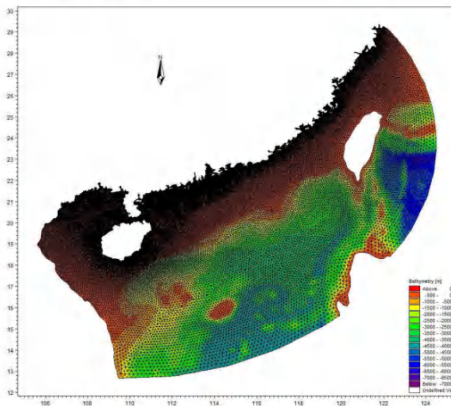
图 7.1-1 大范围模型计算范围
