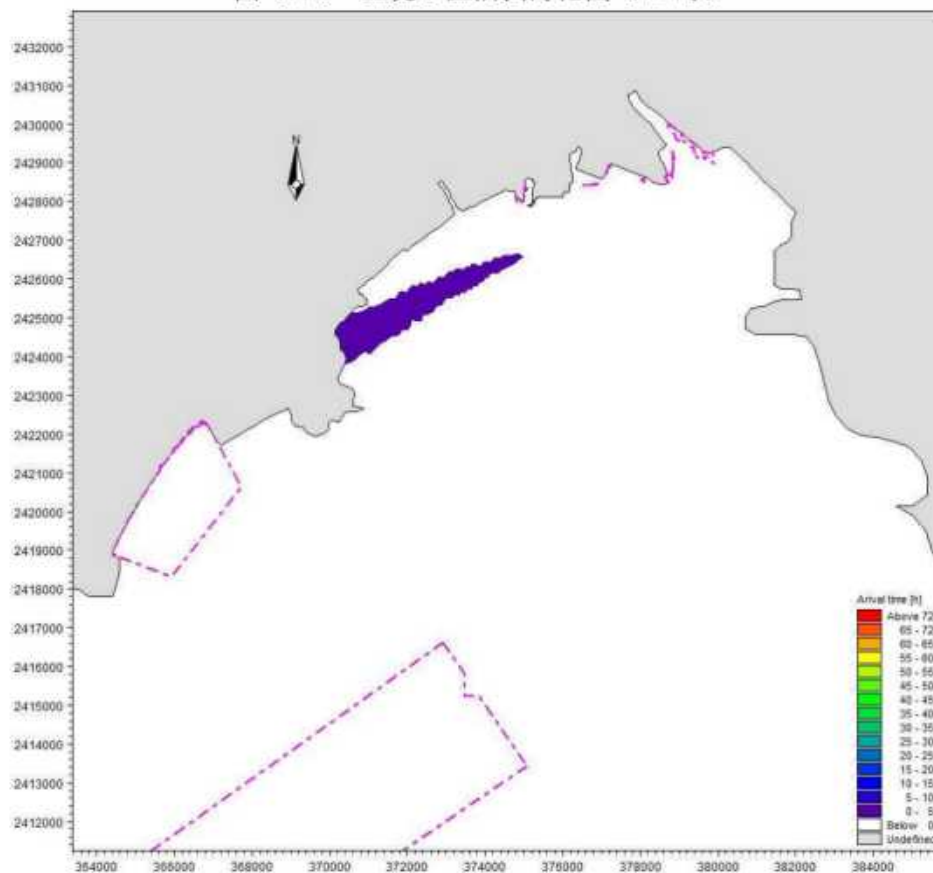
图 8.4-7 工况 6 溢油扫海范围 (72 时)
