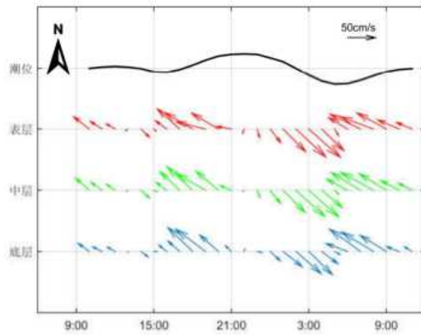
图 6.4-21 调查海域大潮 CL4 站实测海流矢量图
