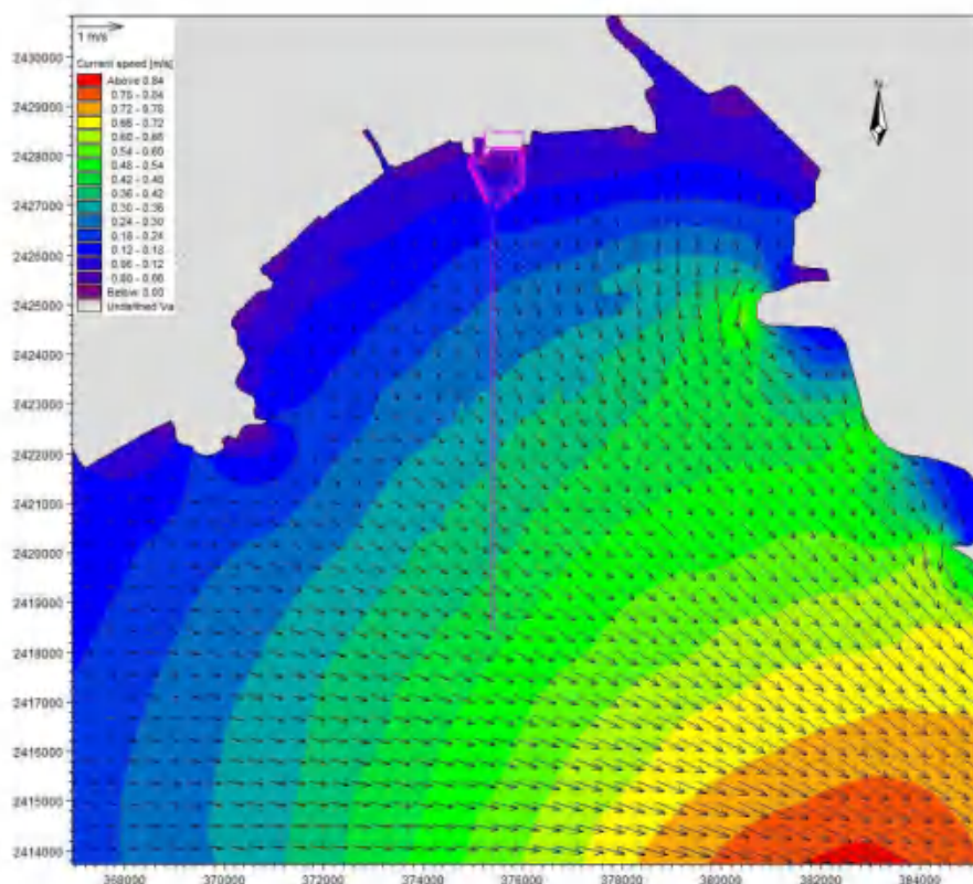
图 7.1-13 工程前工程海域落急流场
