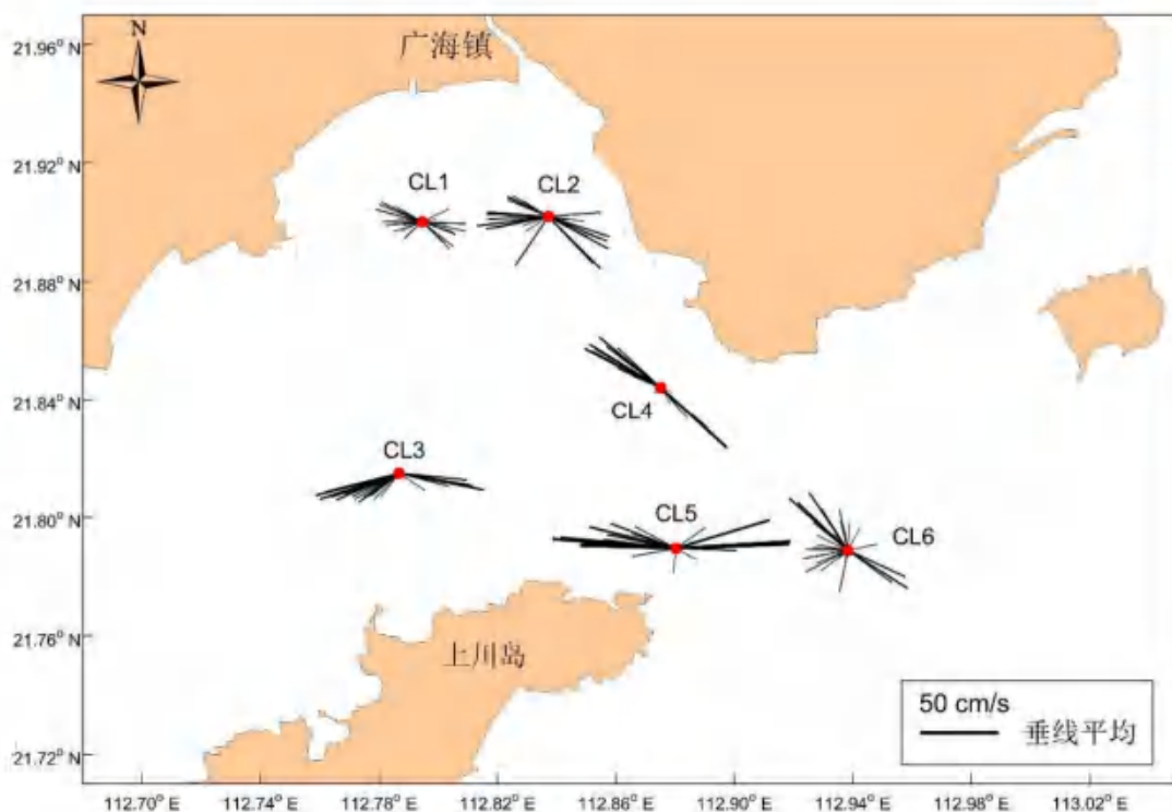
图 6.4-24 大潮期各站垂线平均海流矢量图
