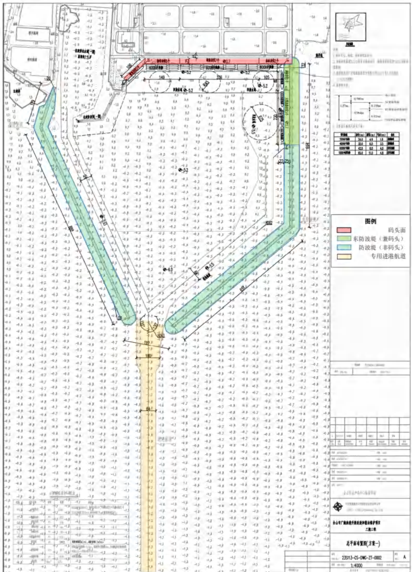
图 4.3-2 本项目水域平面布置图
