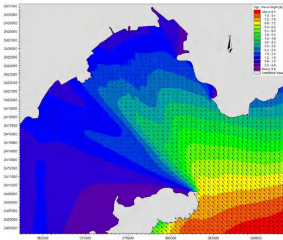
图 7.6-2 工程前 50 年一遇 SE 向有效波高分布图
