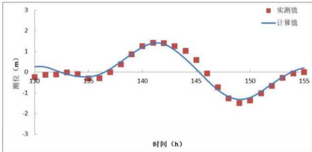
图 7.1-5 CW2 站潮位验证
