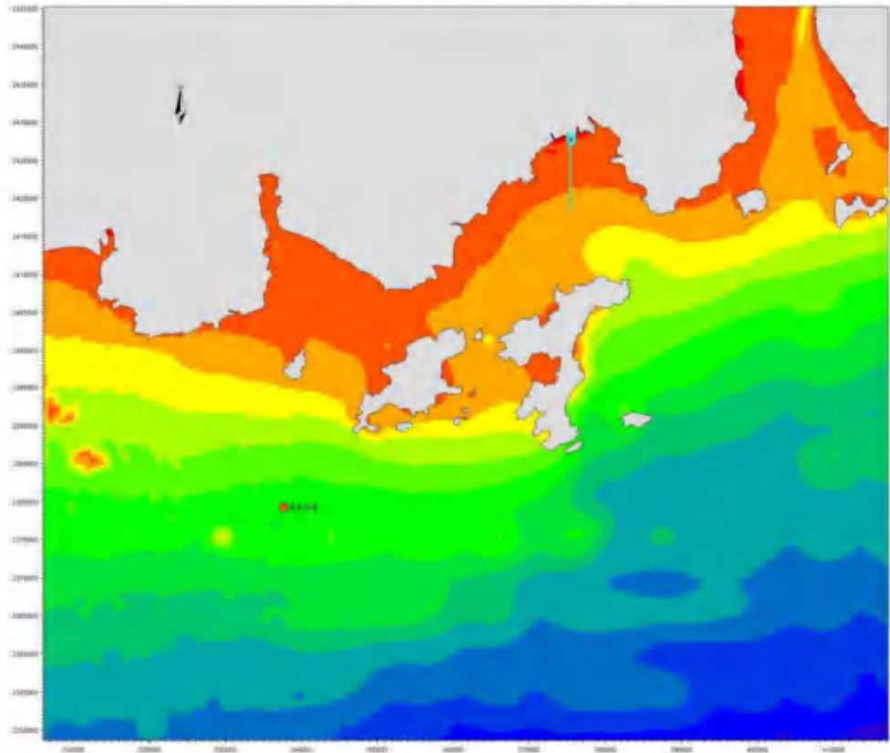
图 7.6-1 波浪验证点位置图
