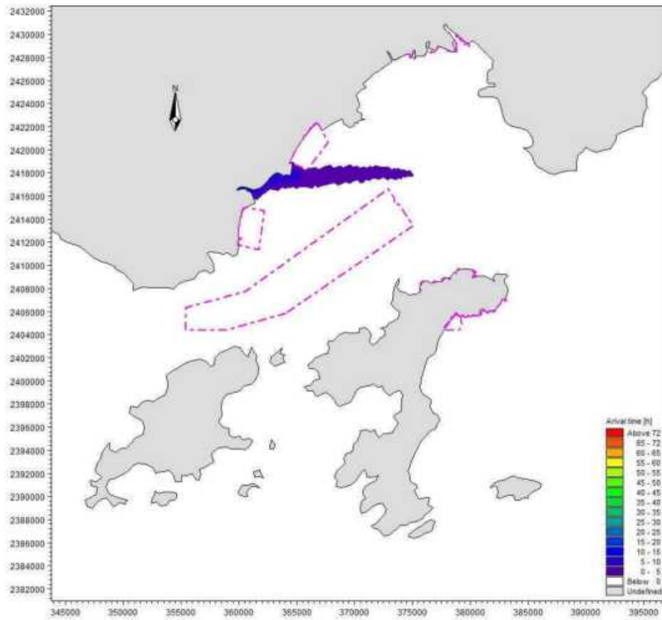
图 8.4-12 工况 11 溢油扫海范围（72 时）
