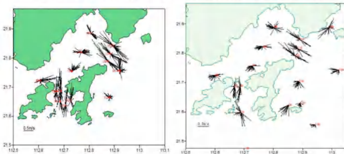
图 6.1-6 项目周边海域夏季（左）和冬季（右）大潮海流矢量分布（中层）
