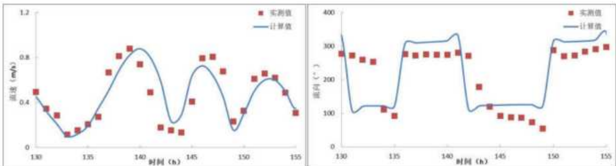
图 7.1-10 CL5 站流速、流向验证
