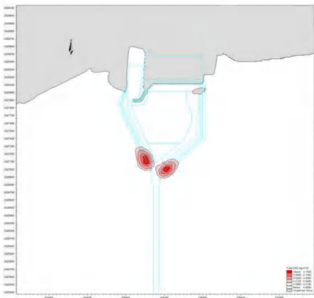
图 7.8-3 典型工况 1 的典型代表点施工悬沙扩散范围
