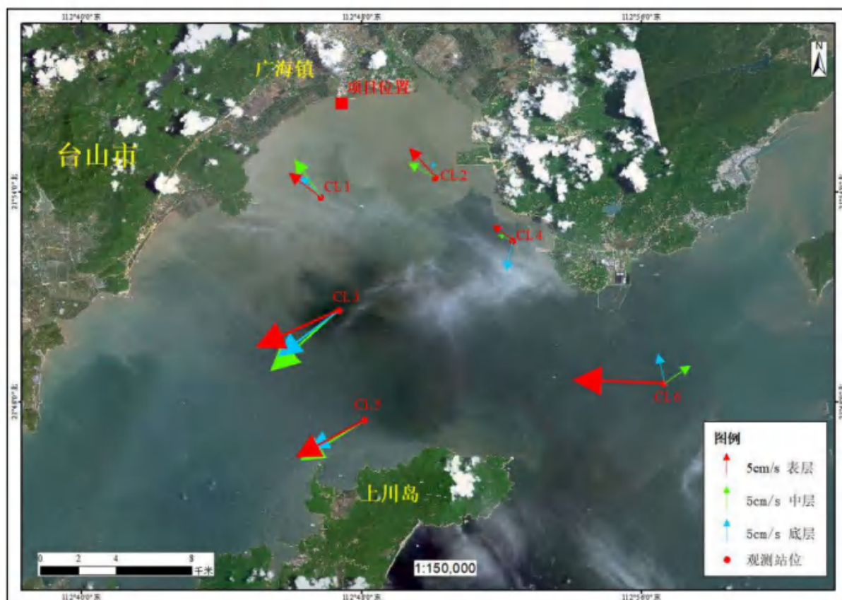
图 6.4-13 观测期间各站各层次余流图
