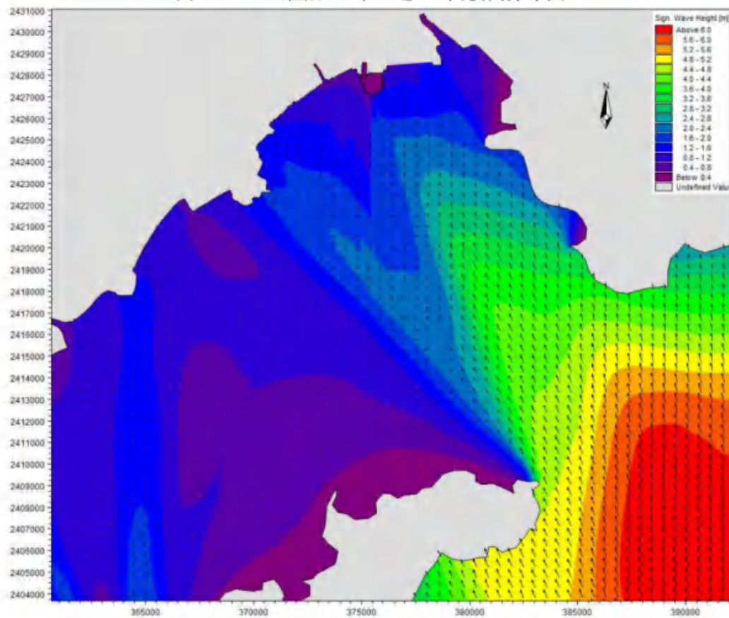
图 7.6-7 工程后 50 年一遇 SSE 向波高分布图
