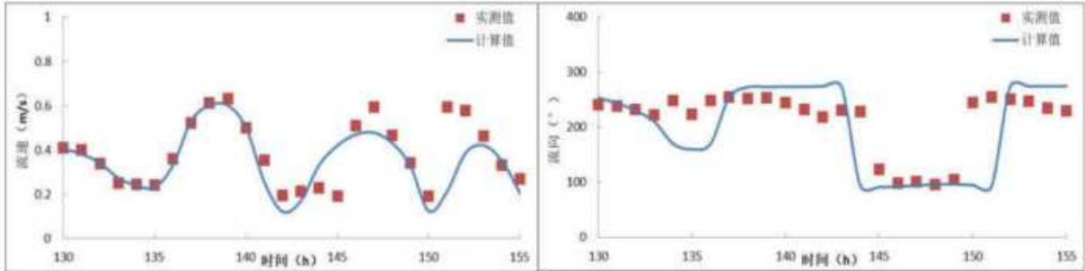
图 7.1-8 CL3 站流速、流向验证
