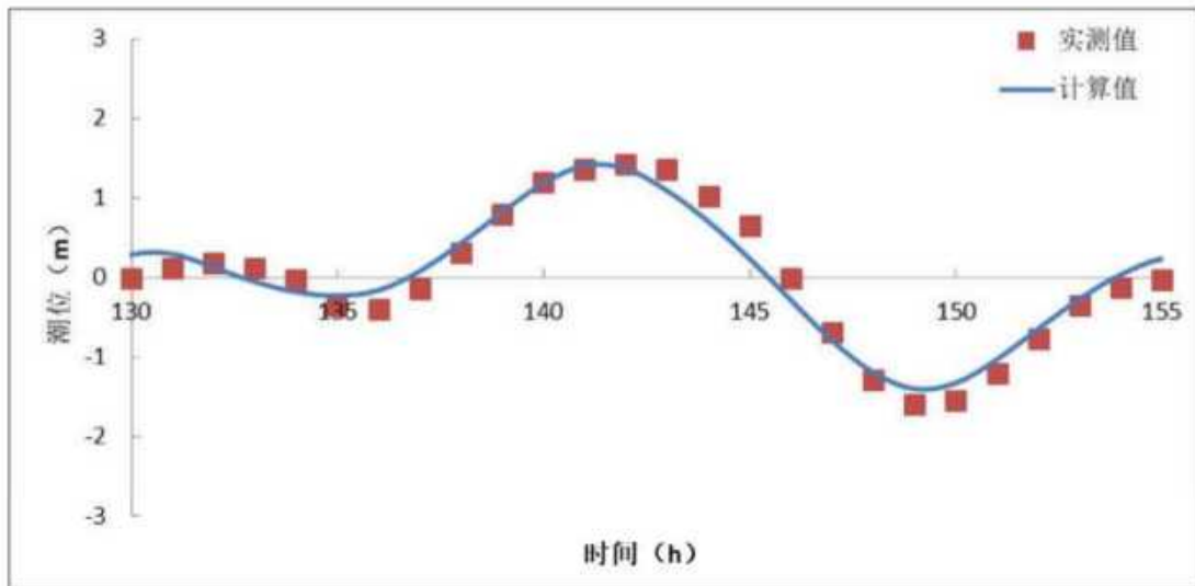
图 7.1-4 CL1 站潮位验证
