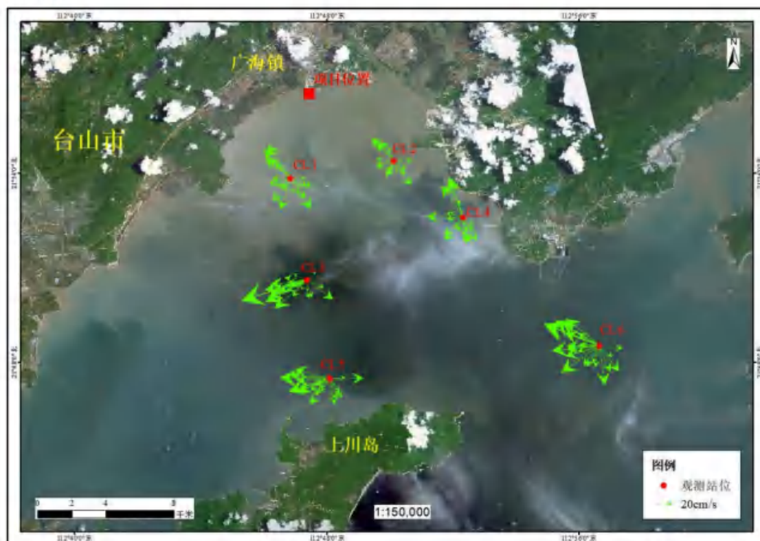
图 6.4-3 观测期间各站表层（0.2h）海流矢量图
