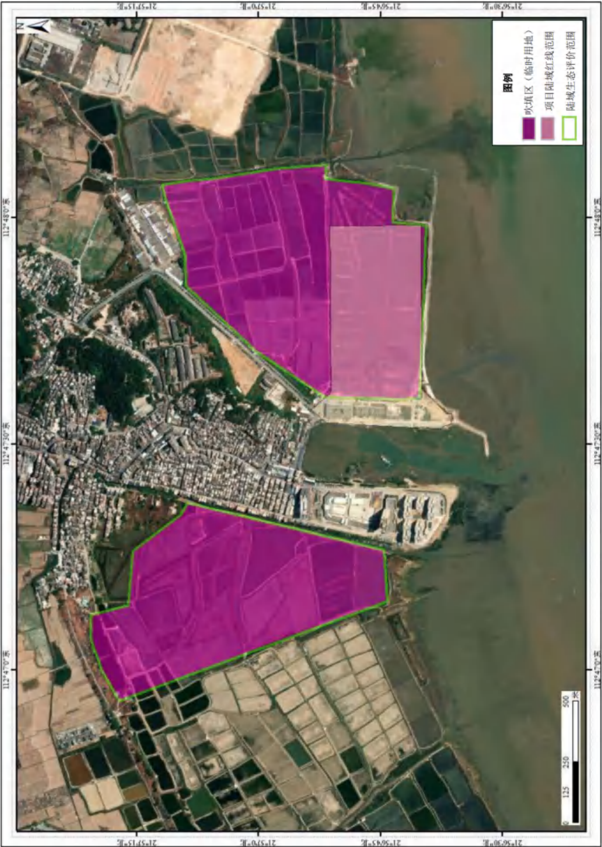
图 2.6-3 陆域生态环境评价范围
