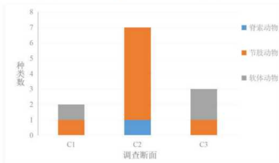
图 6.6-21 潮间带生物种类分布图
