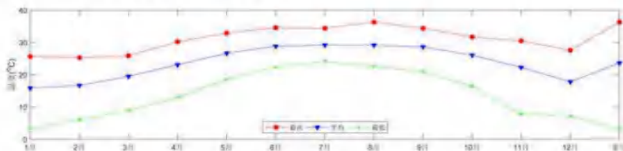
图 6.1-1 台山海洋站平均最高、最低气温月份统计曲线图
