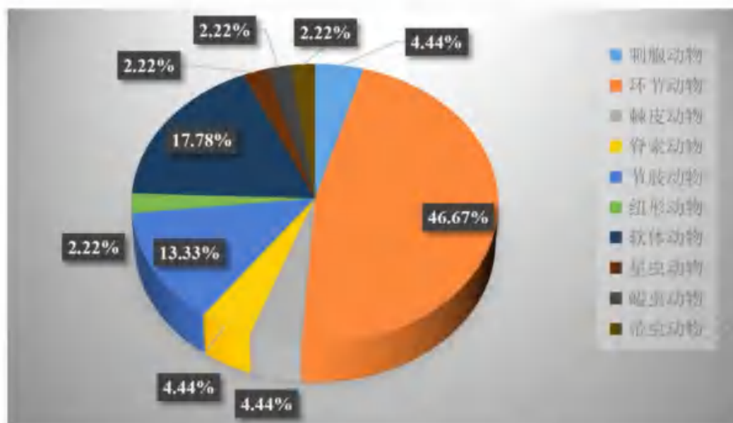
图 6.6-18 调查海域大型底栖生物种类组成
