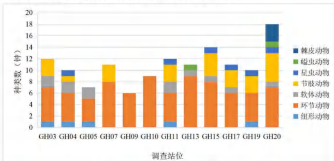
图 6.6-5 大型底栖生物种类组成的空间分布
