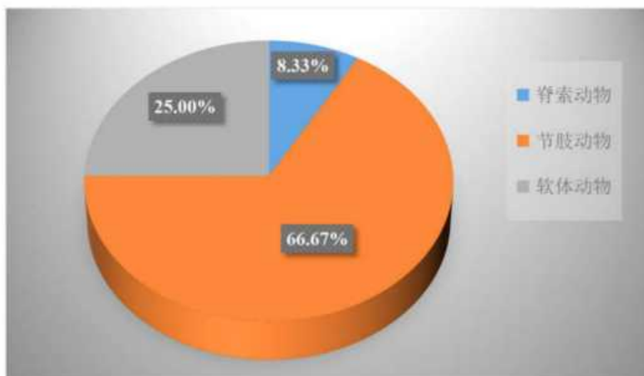
图 6.6-20 潮间带生物定性种类组成
