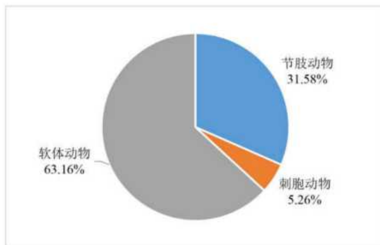
图 6.6-8 潮间带生物定量种类组成
