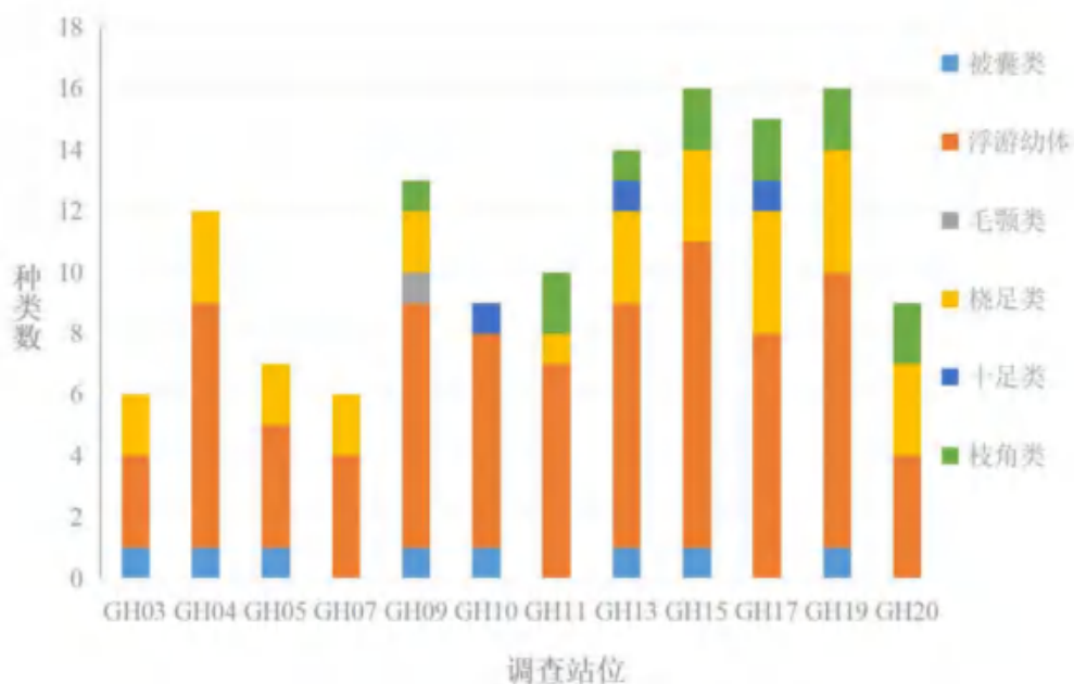
图 6.6-16 调查海域浮游动物类群空间分布
