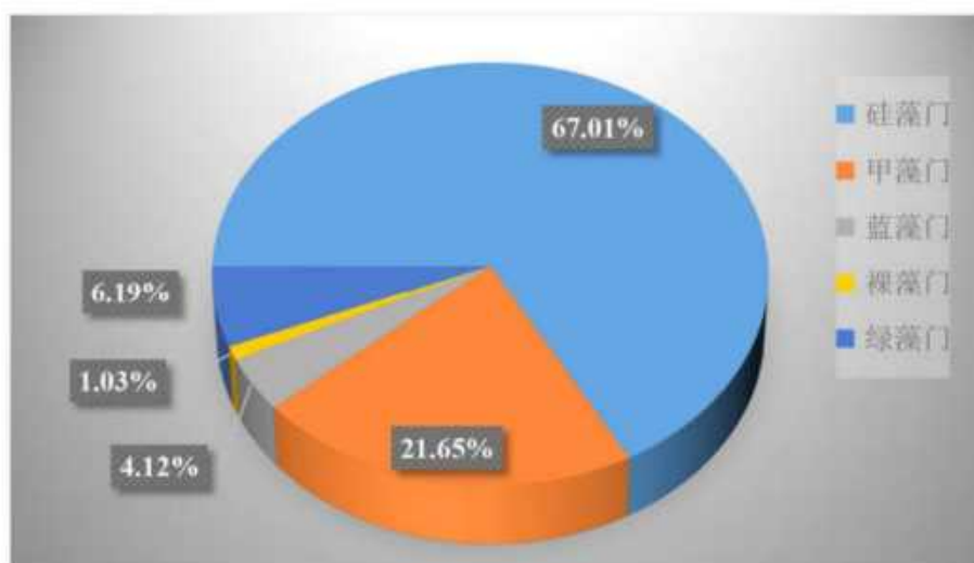
图 6.6-12 调查海域浮游植物种类组成
