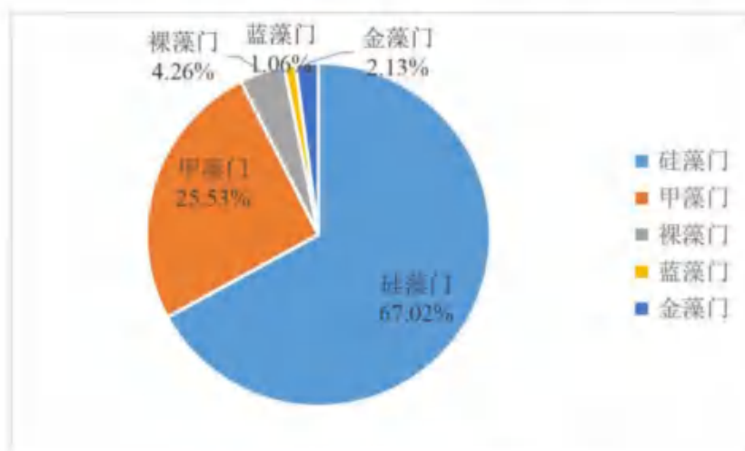
图 6.6-1 浮游植物门类组成情况
