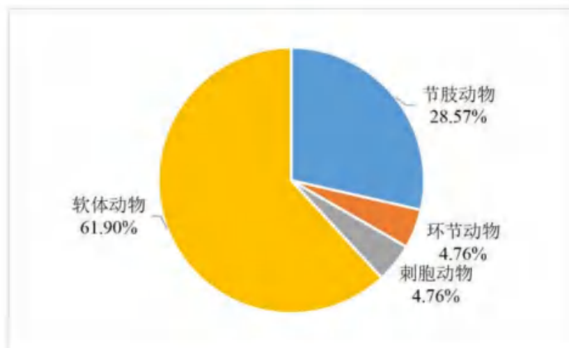
图 6.6-6 潮间带生物定性种类组成
