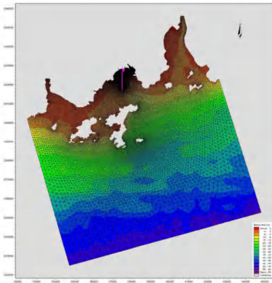
图 7.1-2 小范围模型计算范围
