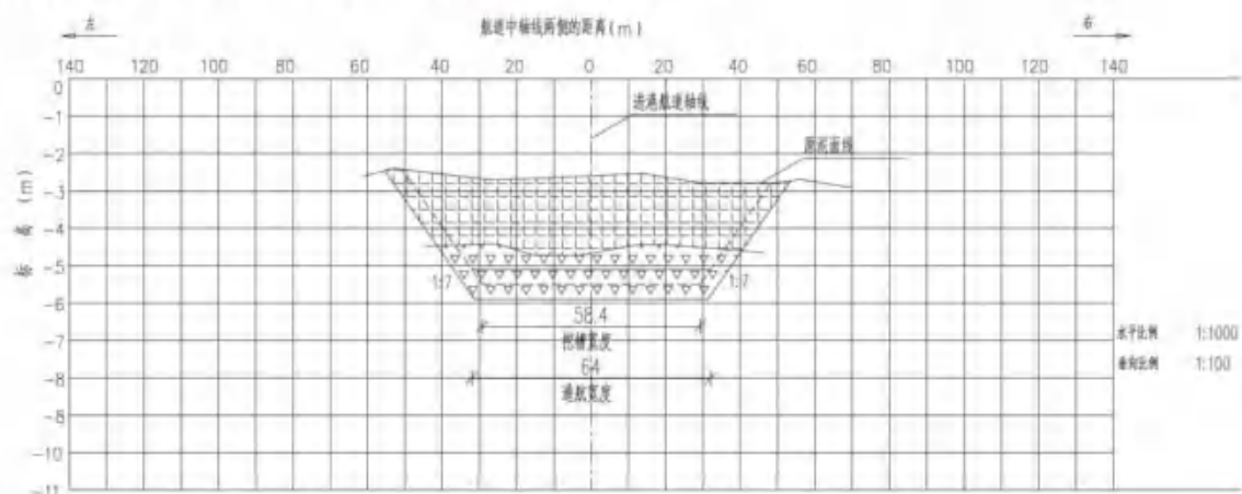
图 4.7-1 航道疏浚断面示意图
