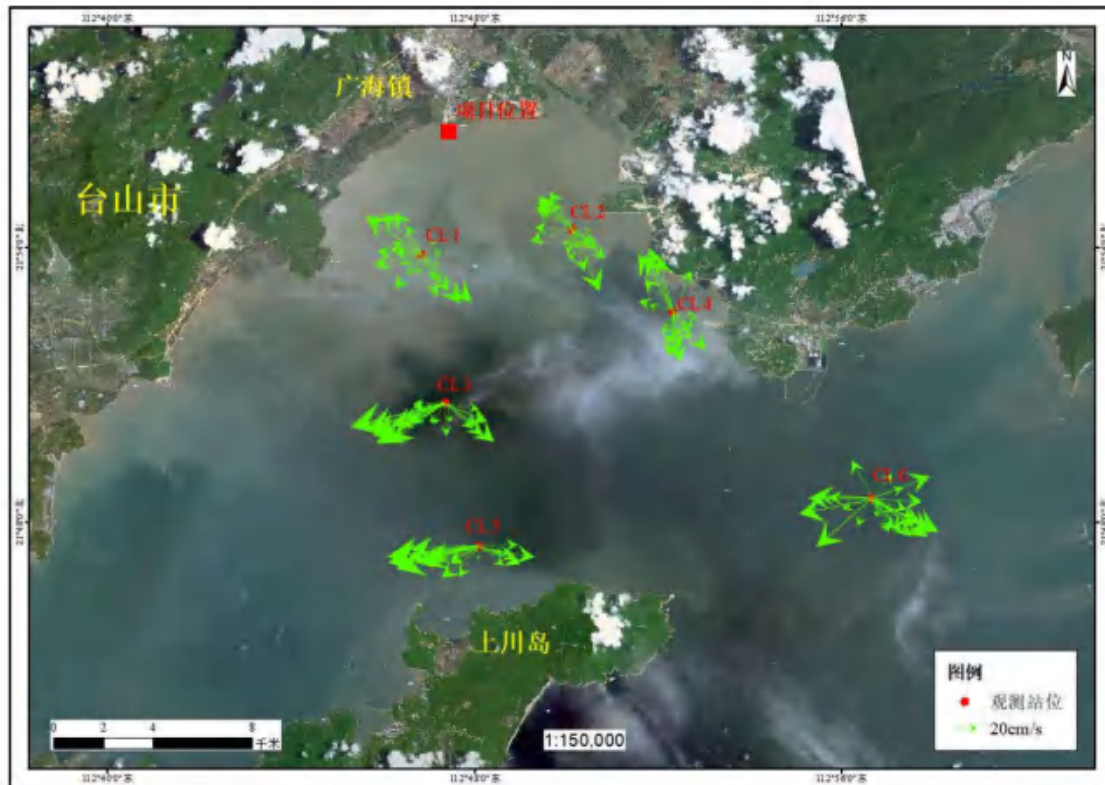
图 6.4-4 观测期间各站中层 (0.6h) 海流矢量图
