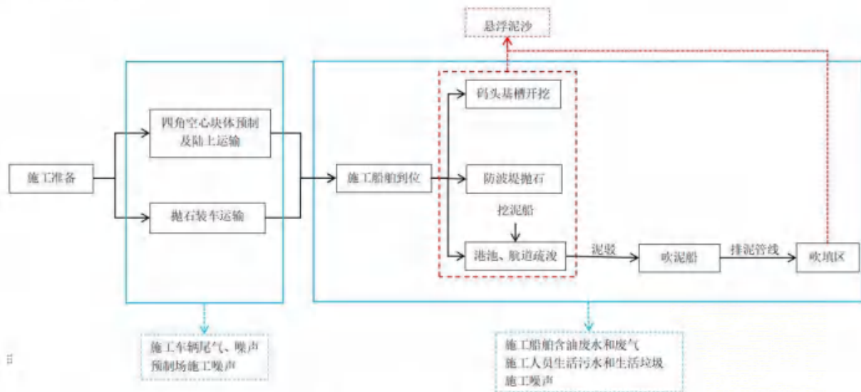
图 5.1-1 项目主要施工工艺流程及产污环节示意图
