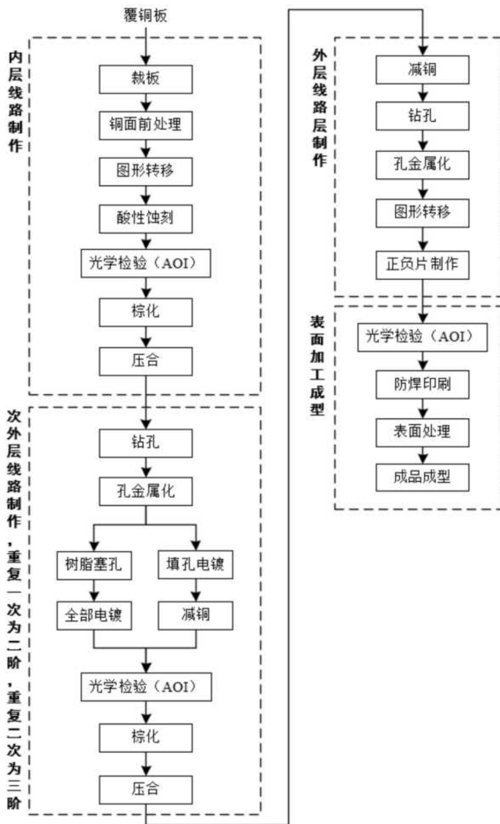
图 1.6-2 HDI 板生产工艺流程图
