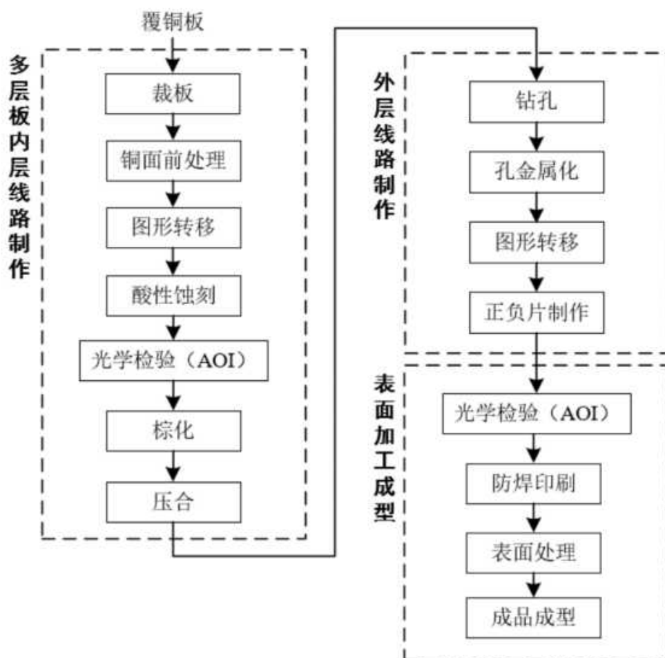
图 1.6-1 双面板、多层板生产工艺流程图
