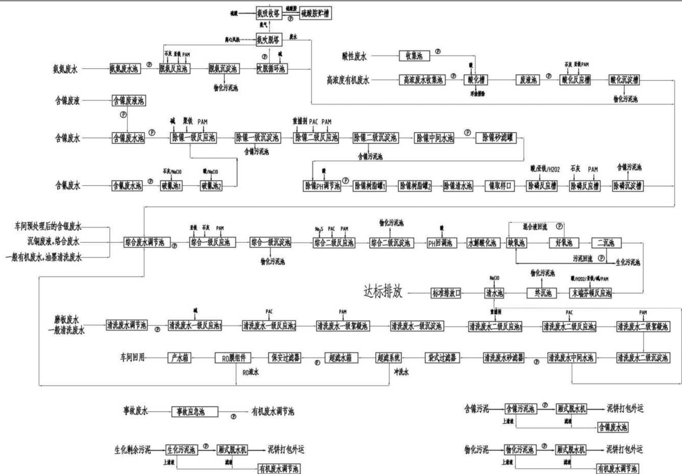
图 1.10-1 本项目生产废水处理系统工艺流程图
