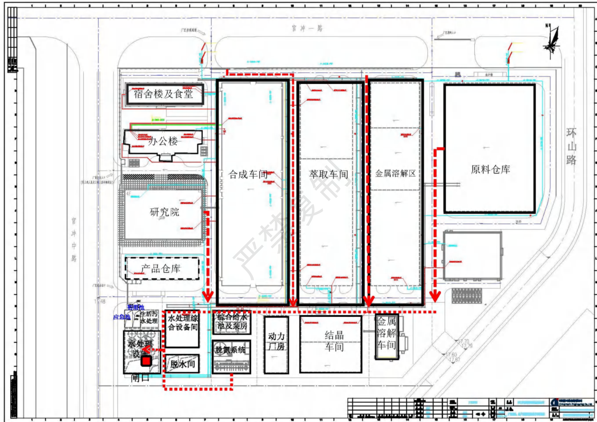
图 9.6-19 生产废水收集管网示意图
