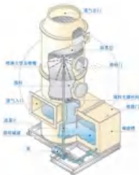
图 10.2-4 碱液喷淋装置示意图
