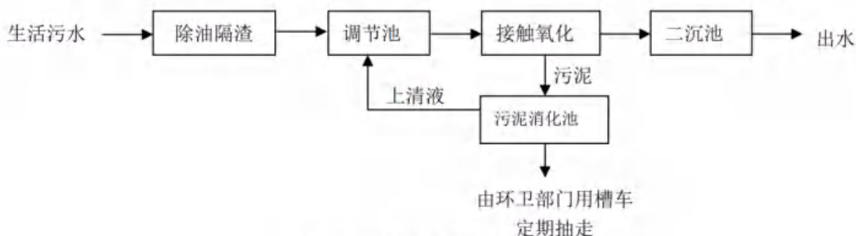
图 10.1-2 污水处理工艺流程示意图
