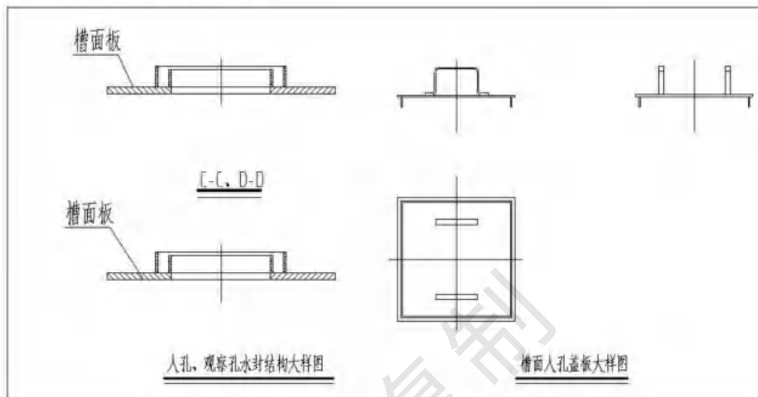
图 4.6-3 萃取槽封闭方式示意图
