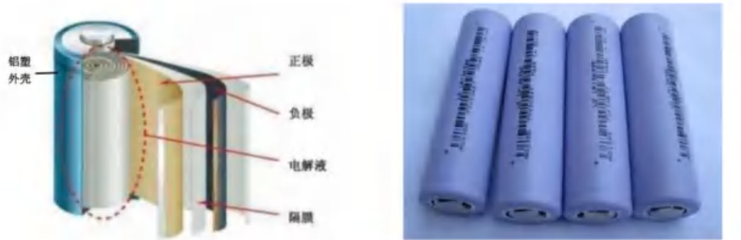
圆柱形锂电池单体结构图与实体图
