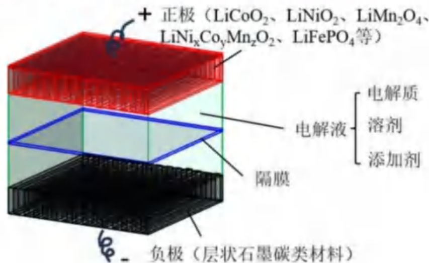
图 4.2-11 锂电池结构示意图
