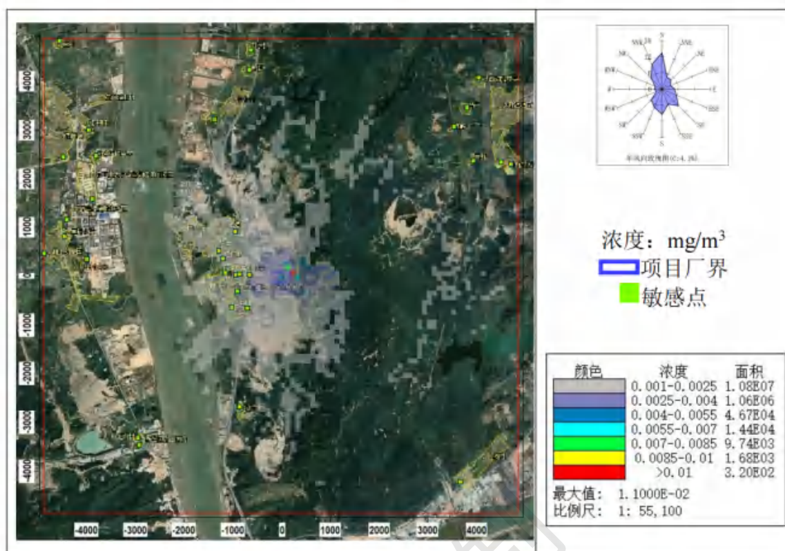
图 8.2-51 镍及其化合物小时平均浓度分布图
