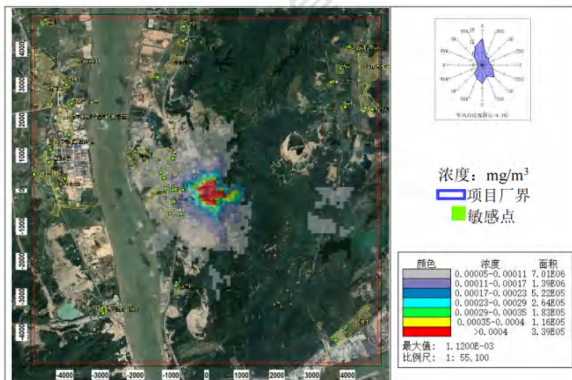
图 8.2-40 锰及其化合物日平均浓度分布图
