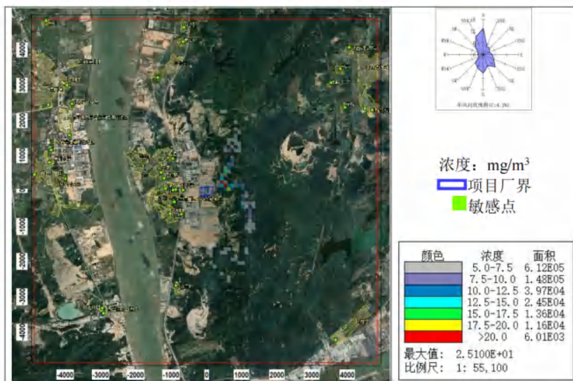
图 8.2-60 NMHC 小时平均浓度分布图（非正常排放状况）
