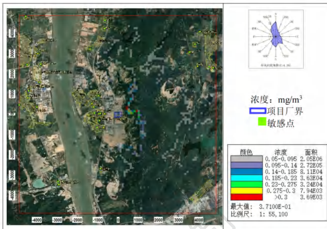
图 8.2-64 锰及其化合物小时平均浓度分布图（非正常排放状况）
