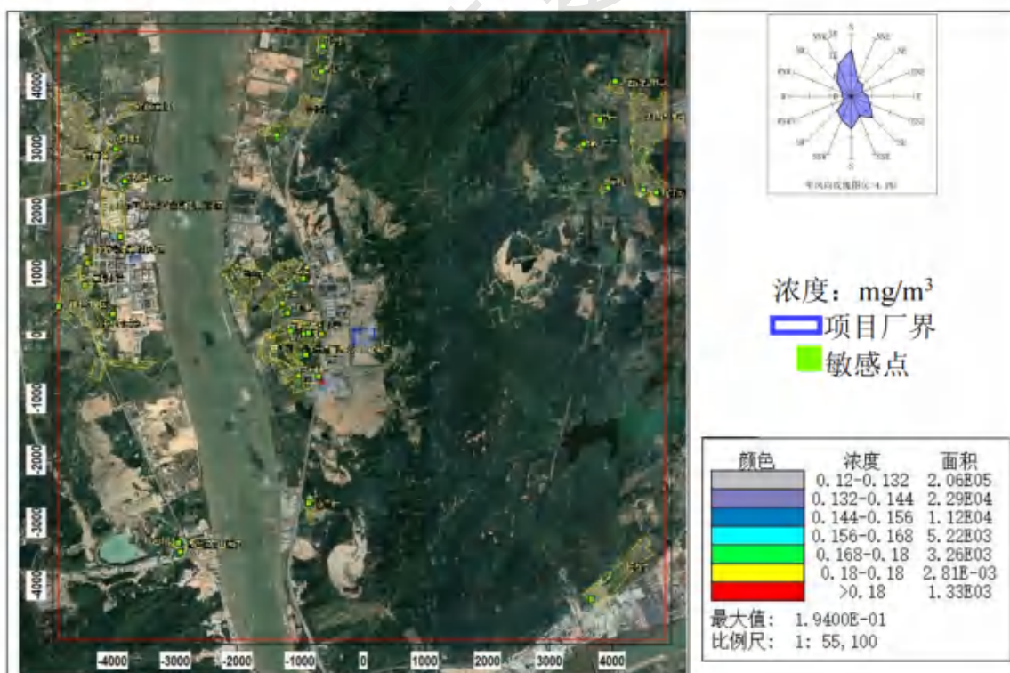
图 8.2-18 TSP 日平均浓度分布图（叠加在建、拟建源及背景后）
