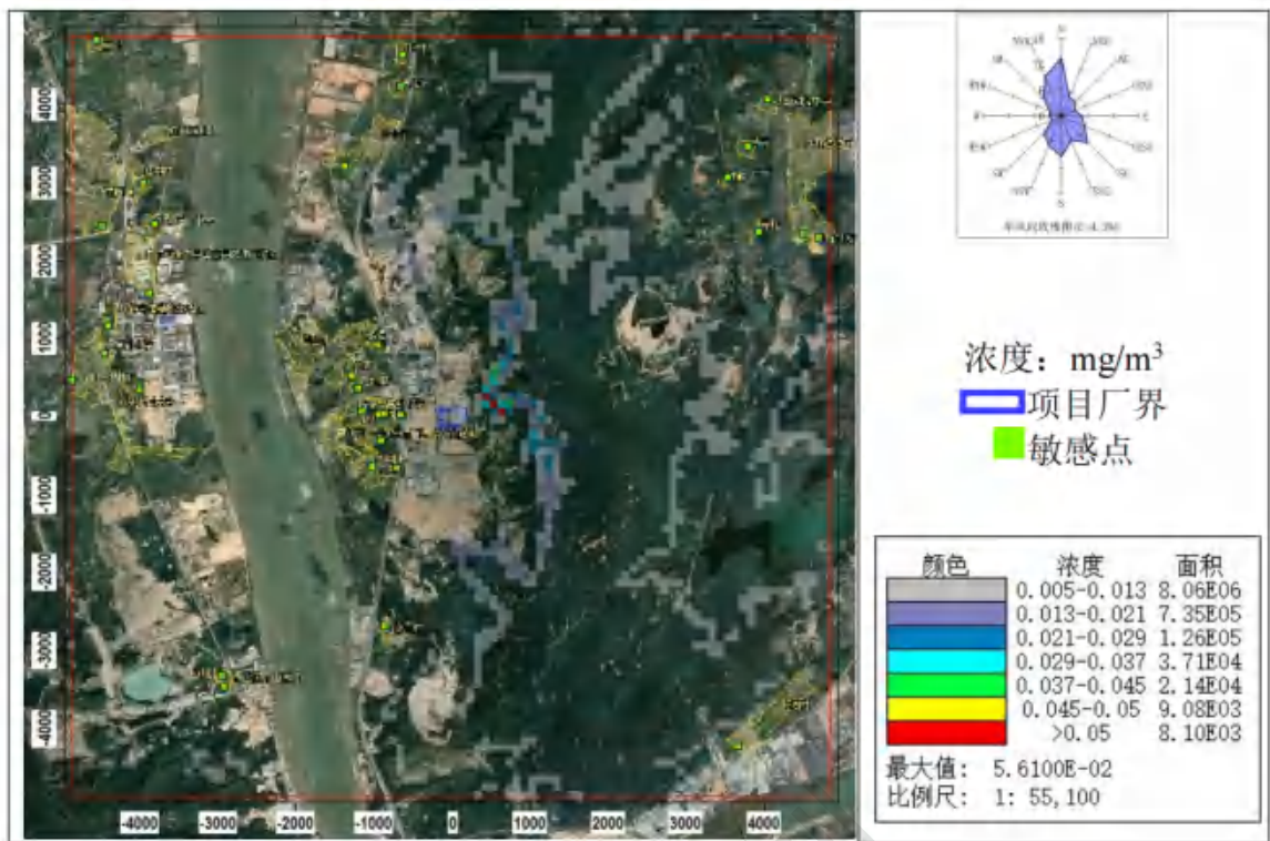
图 8.2-70 CO 小时平均浓度分布图（非正常排放状况）
