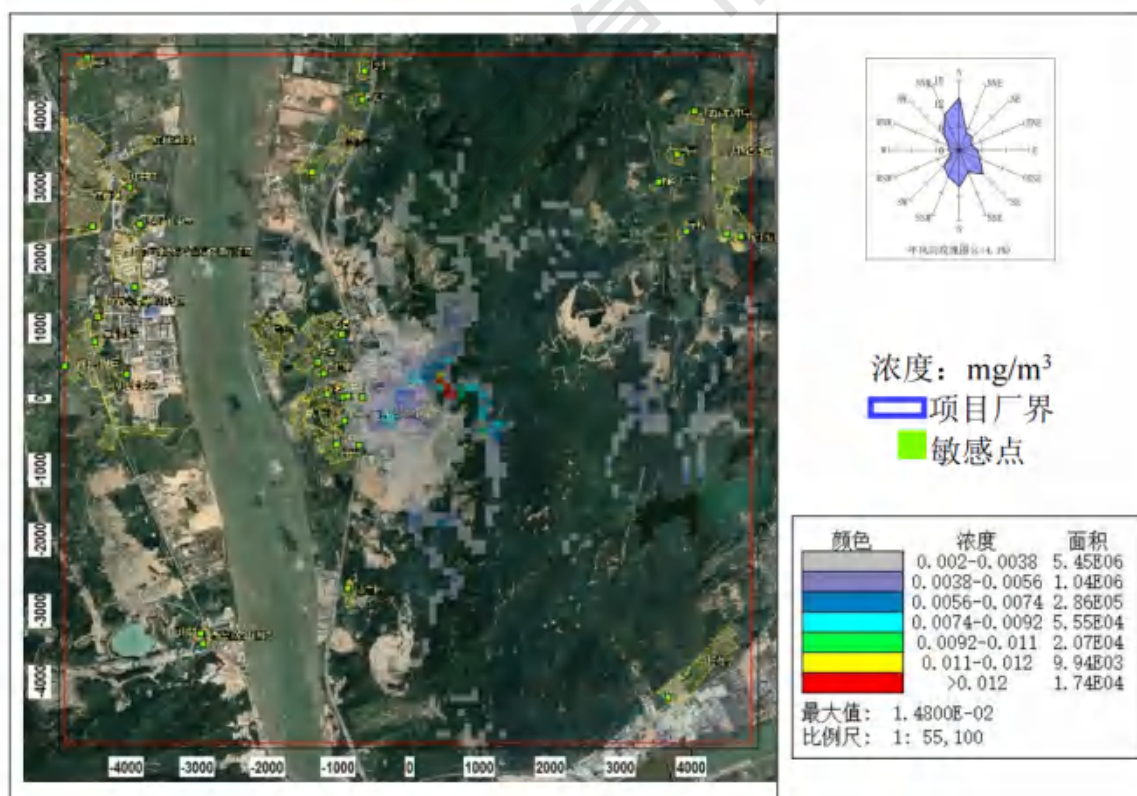
图 8.2-12 \text{NO}_2 日平均浓度分布图
