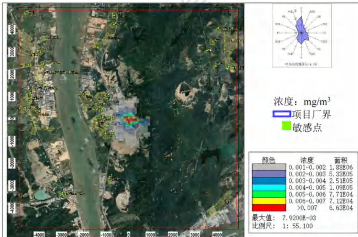
图 8.2-16 TSP 日平均浓度分布图
