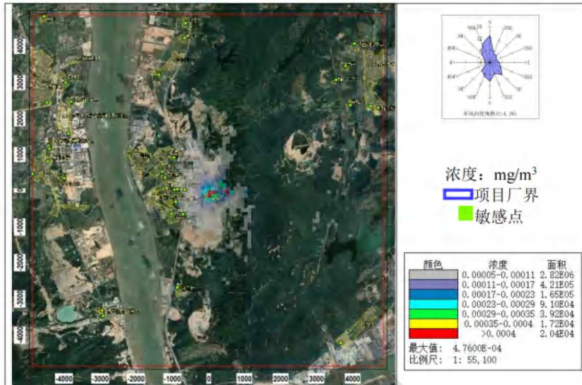
图 8.2-37 HCl 日平均浓度分布图
