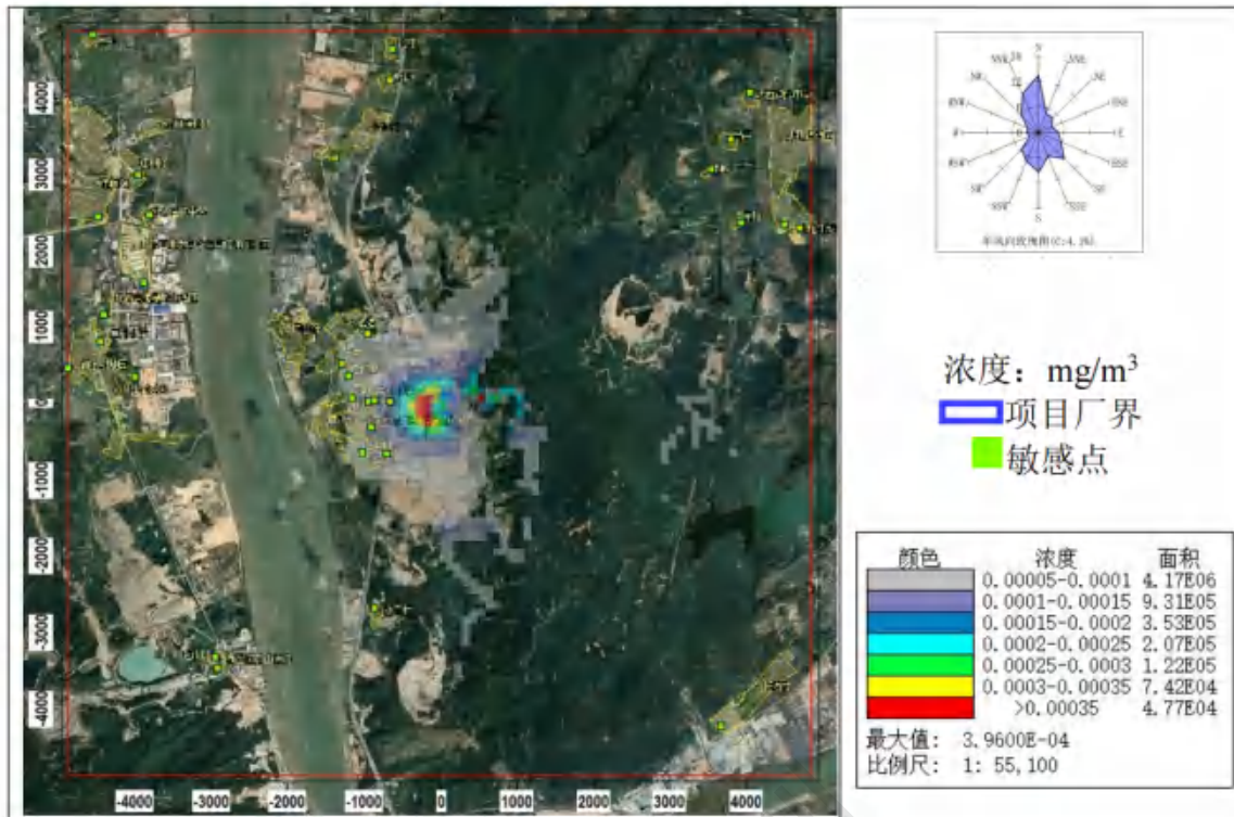
图 8.2-21 \text{PM}_{10} 年平均浓度分布图
