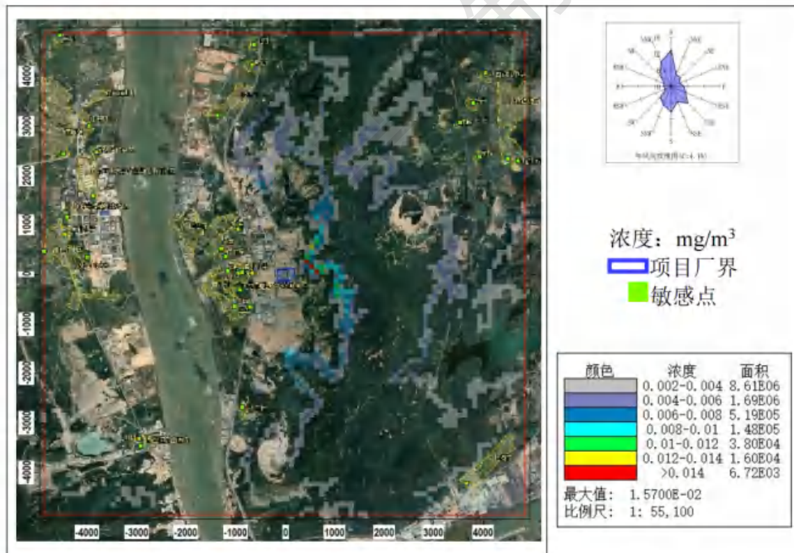
图 8.2-6 \text{SO}_2 小时平均浓度分布图（本项目贡献值）
