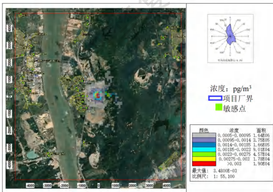
图 8.2-44 二噁英年平均浓度分布图
