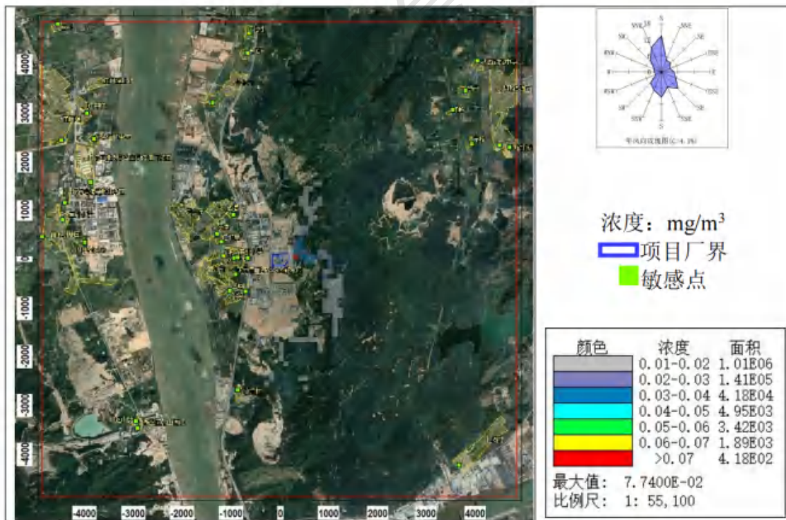
图 8.2-32 硫酸雾小时平均浓度分布图
