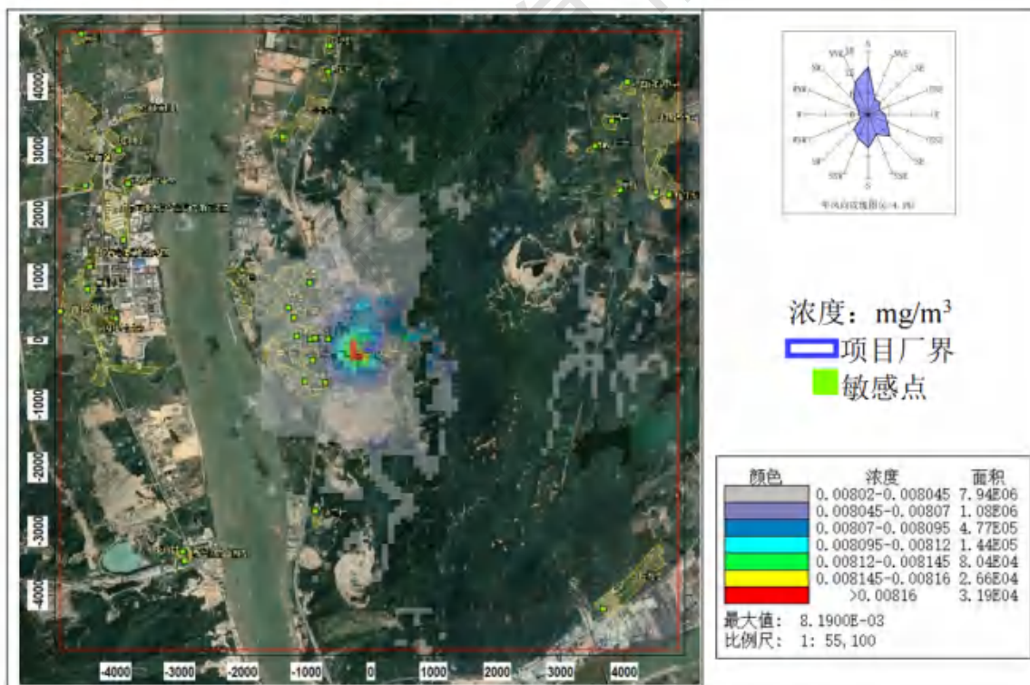
图 8.2-10 \text{SO}_2 年平均浓度分布图 (叠加在建、拟建源及背景后)
