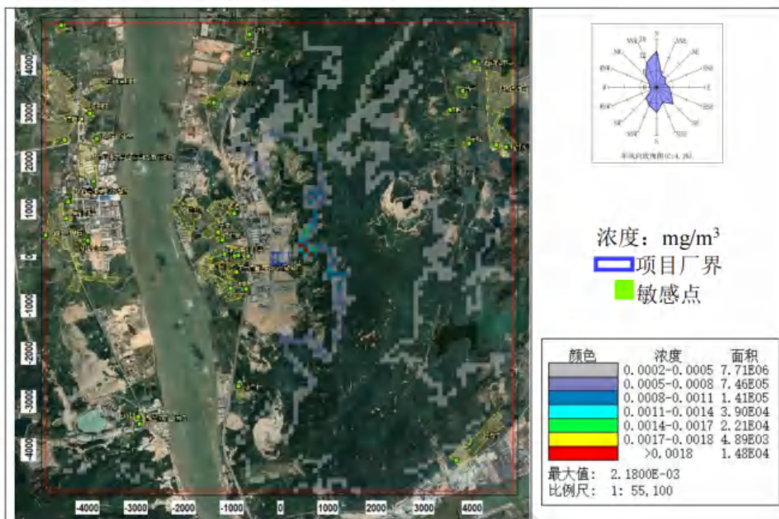
图 8.2-45 氟化物小时平均浓度分布图
