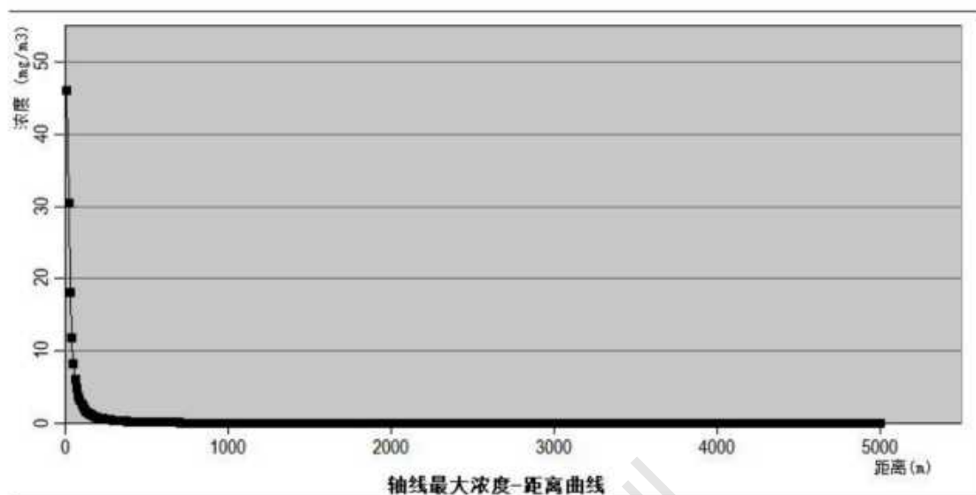
图 9.6-6 氨水泄露产生的氨气在下风向不同距离处的最大浓度（最常见气象条件，NE）
