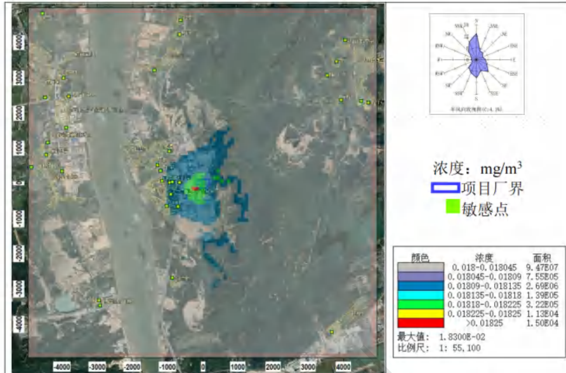
图 8.2-27 \text{PM}_{2.5} 年平均浓度分布图（叠加在建、拟建源及背景后）
