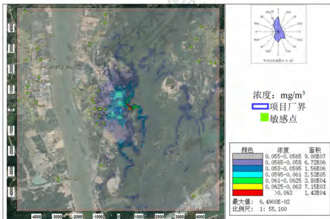
图 8.2-14 \text{NO}_2 日平均浓度分布图 (叠加在建、拟建源及背景后)
