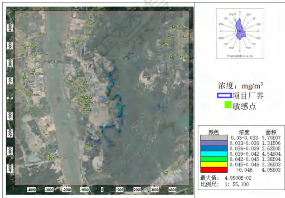
图 8.2-38 HCl 小时平均浓度分布图（叠加在建、拟建源及背景后）
