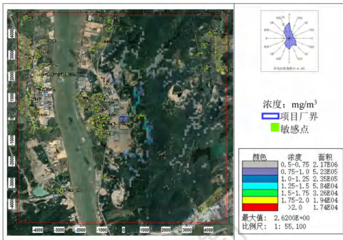
图 8.2-58 \text{PM}_{10} 小时平均浓度分布图 (非正常排放状况)
