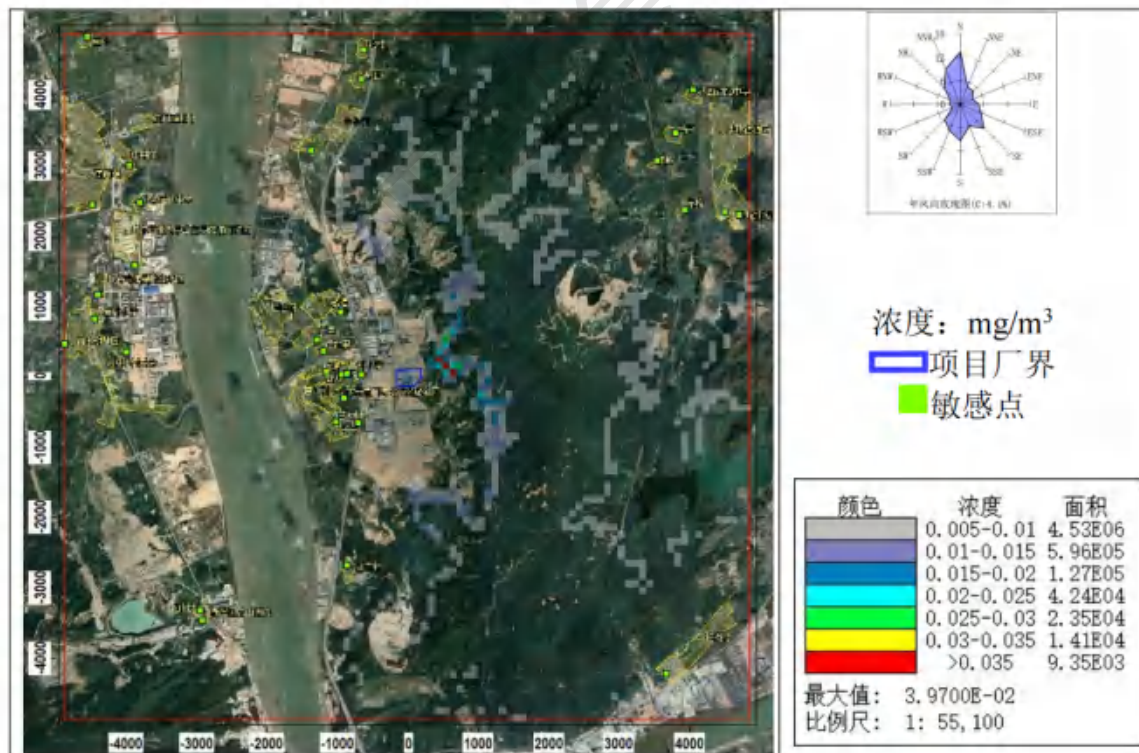
图 8.2-28 NMHC 小时平均浓度分布图
