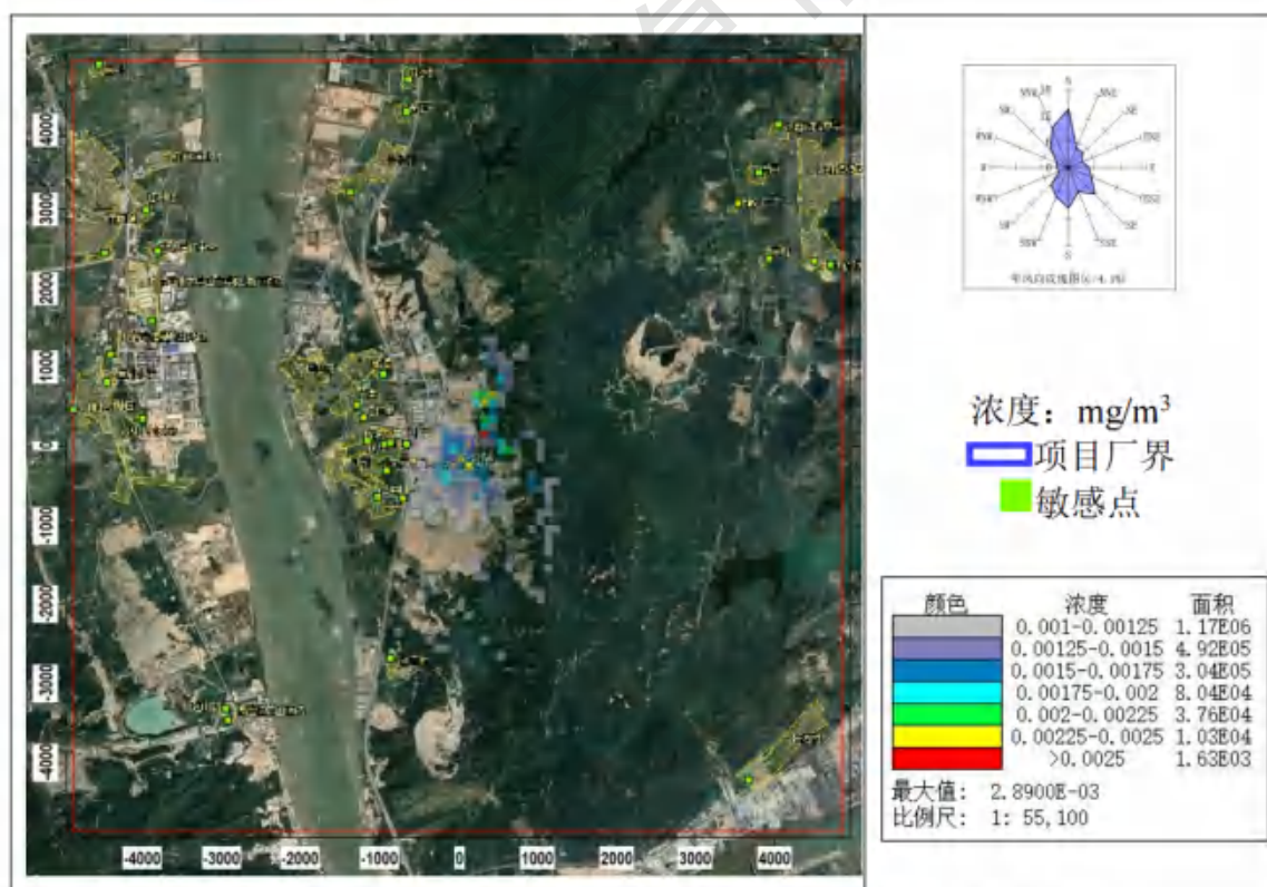
图 8.2-50 硫化氢小时平均浓度分布图（叠加在建、拟建源及背景后）
