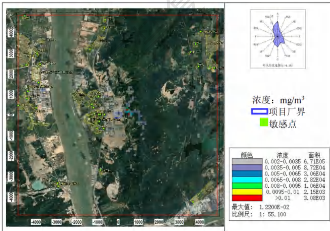
图 8.2-30 TVOC 8 小时平均浓度分布图
