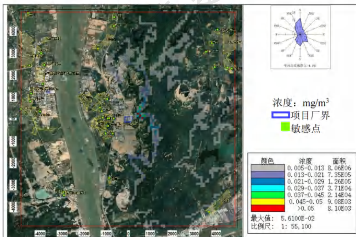
图 8.2-52 CO 小时平均浓度分布图
