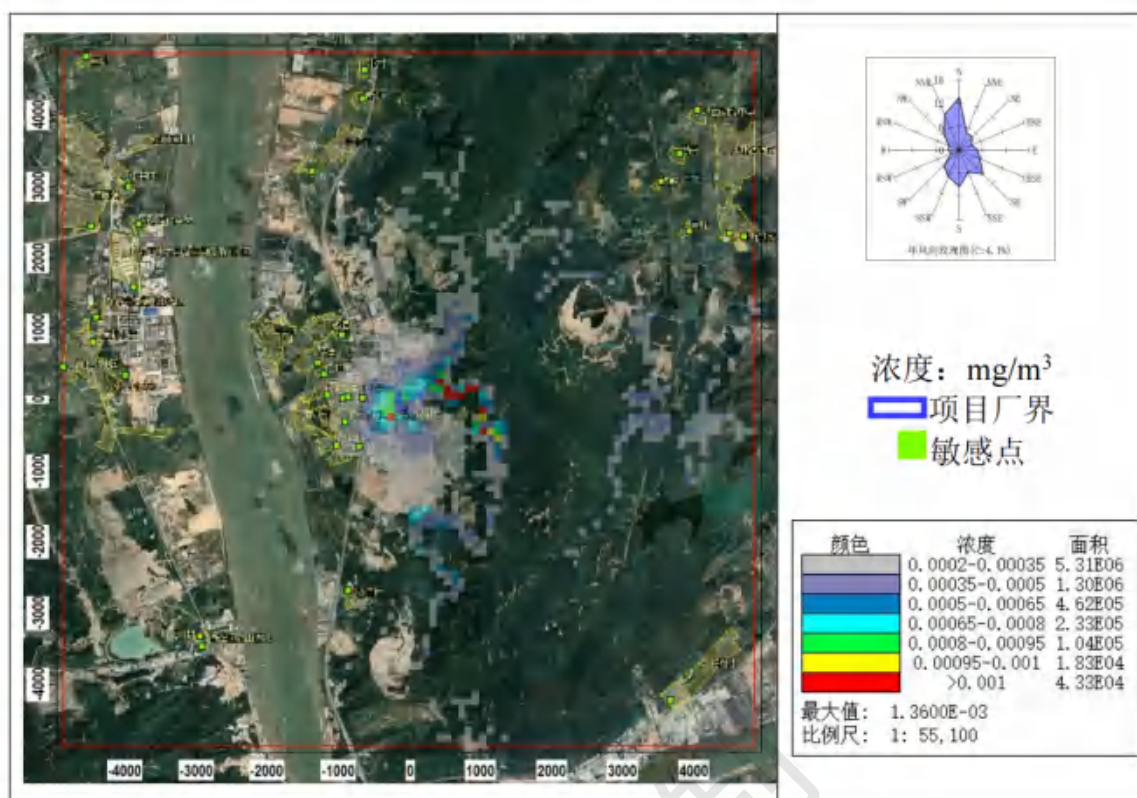
图 8.2-7 \text{SO}_2 日平均浓度分布图 (本项目贡献值)
