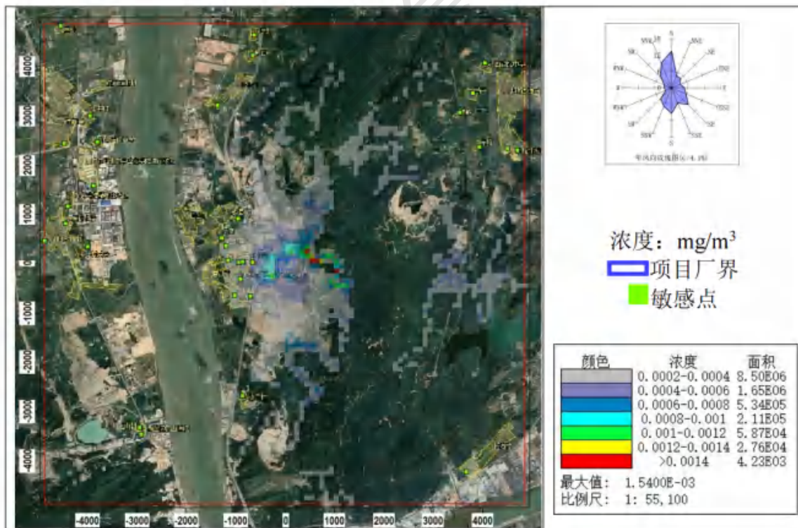
图 8.2-24 \text{PM}_{2.5} 日平均浓度分布图
