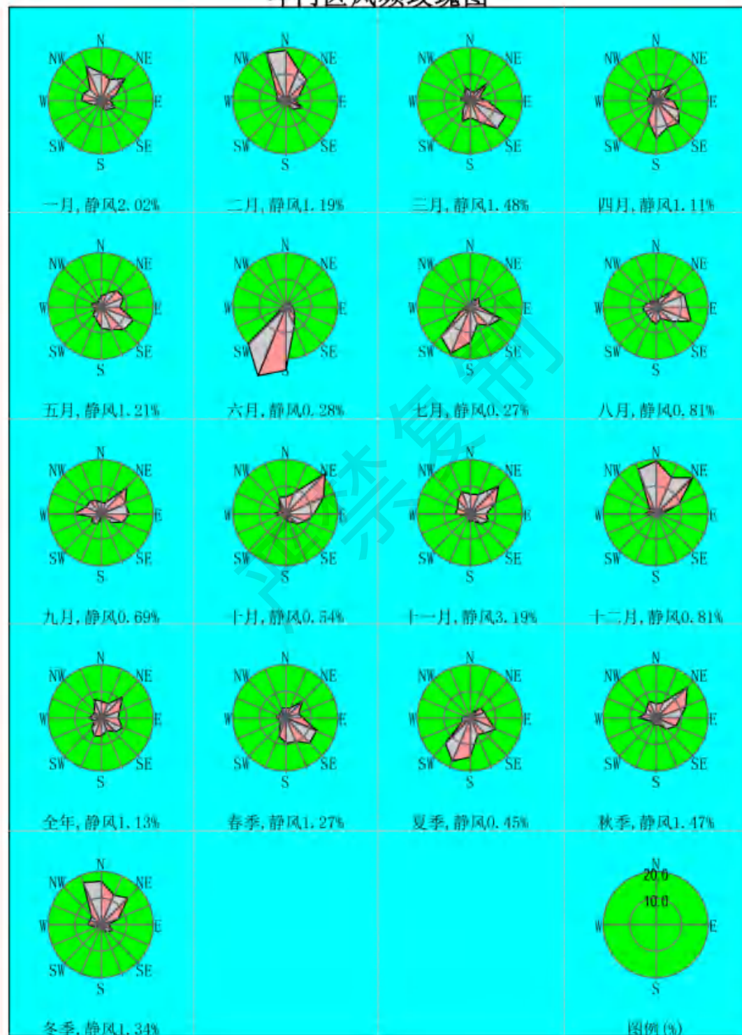
斗门区风频玫瑰图
