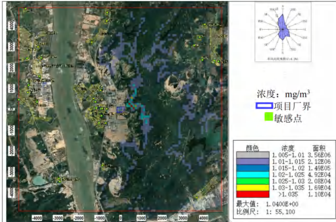
图 8.2-29 NMHC 小时平均浓度分布图 (叠加在建、拟建源及背景后)
