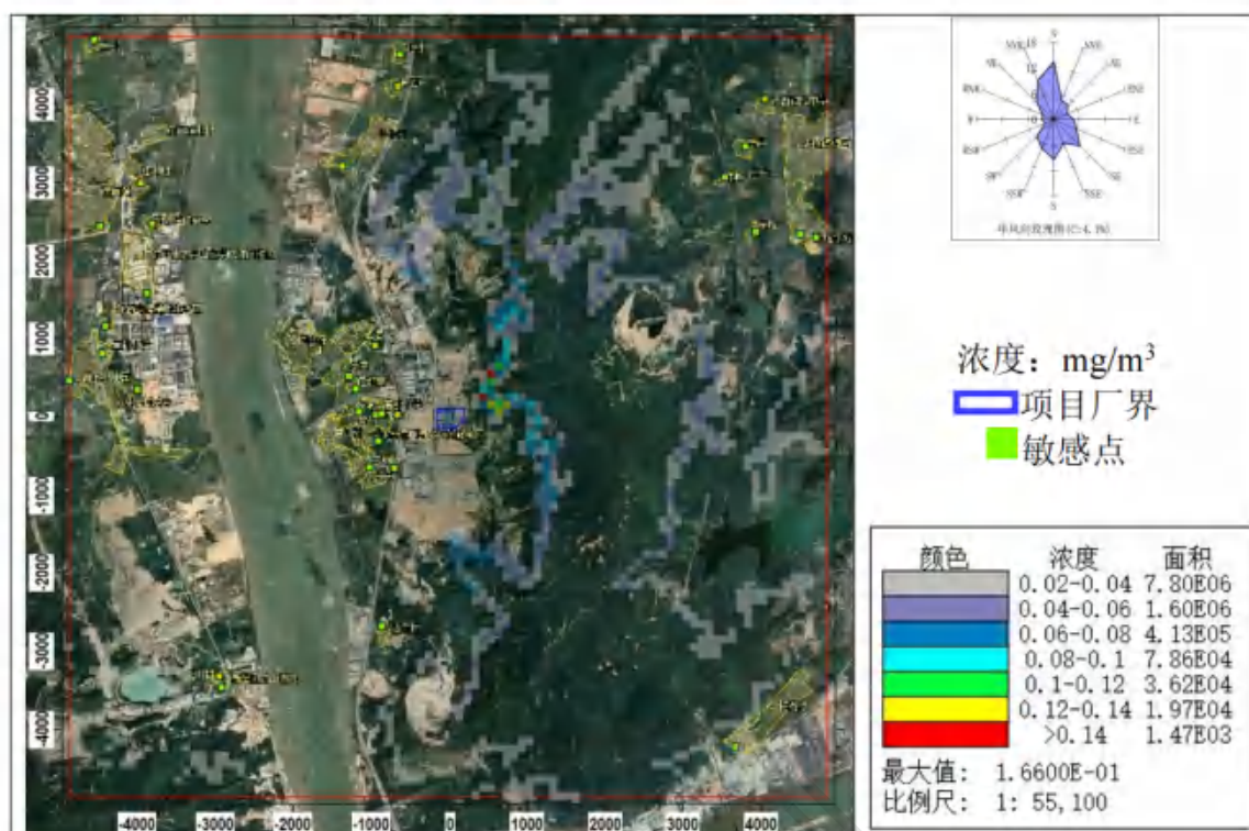
图 8.2-11 \text{NO}_2 小时平均浓度分布图
