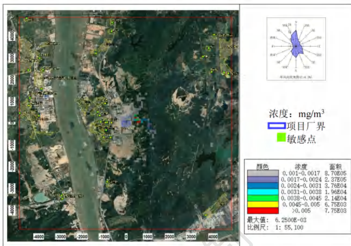
图 8.2-53 CO 日平均浓度分布图
