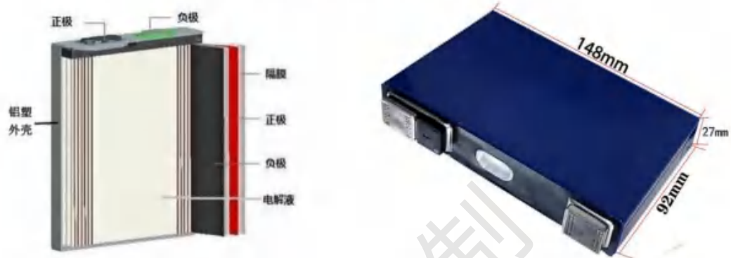
方形锂电池单体结构图与实体图
