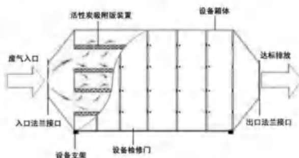
图 10.2-5 活性炭吸附器结构示意图
