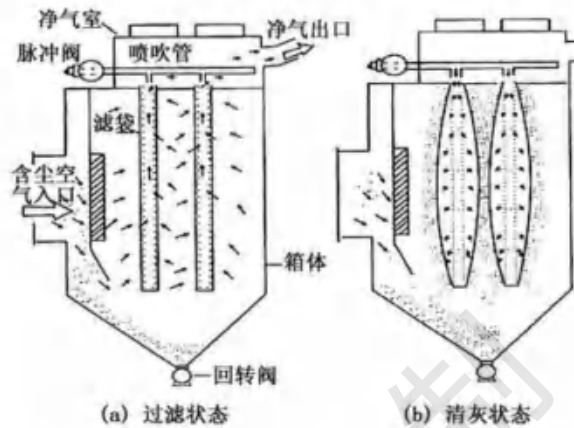
图 10.2-2 布袋除尘原理示意图
