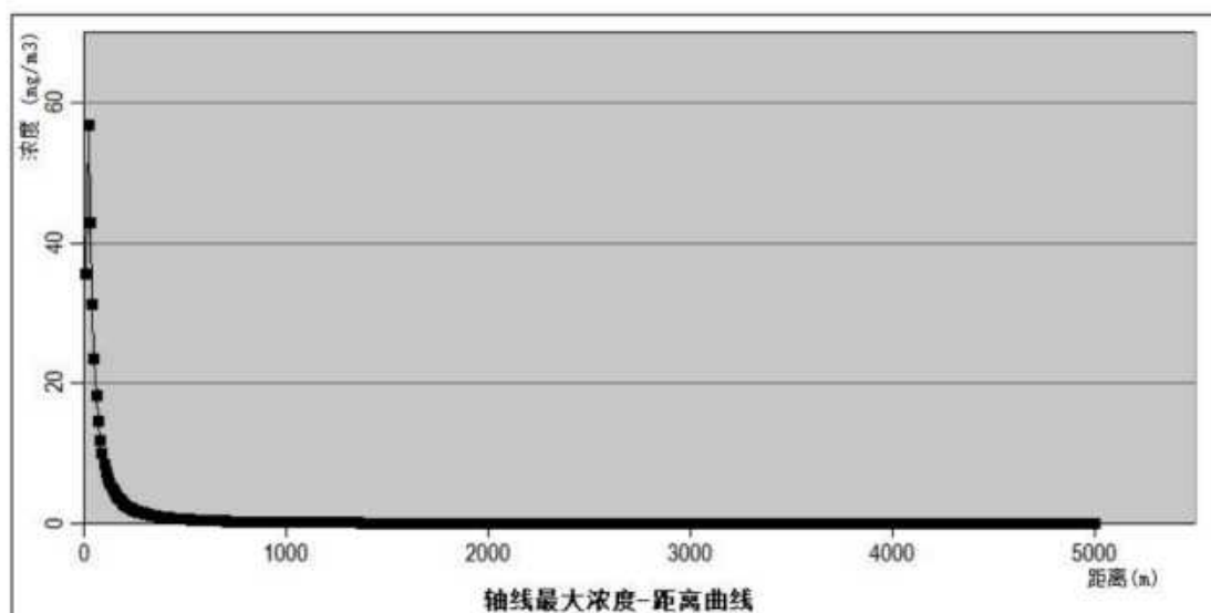
图 9.6-3 盐酸泄露产生的 HCl 在下风向不同距离处的最大浓度（最常见气象条件）
