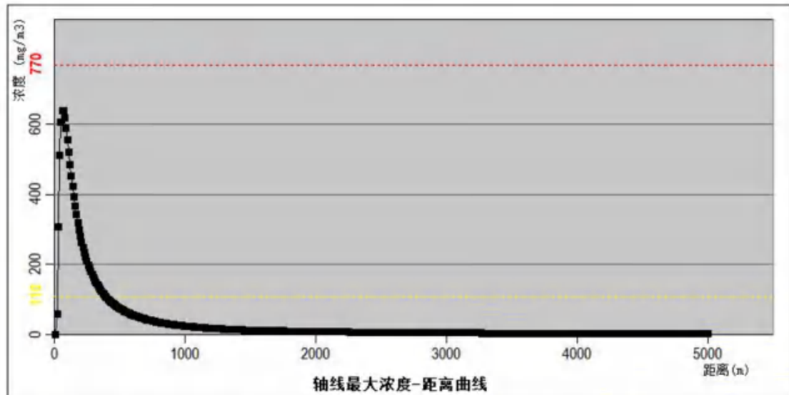
图 9.6-7 脱氨车间管径泄露产生的氨气在下风向不同距离处的最大浓度（最不利气象条件）
