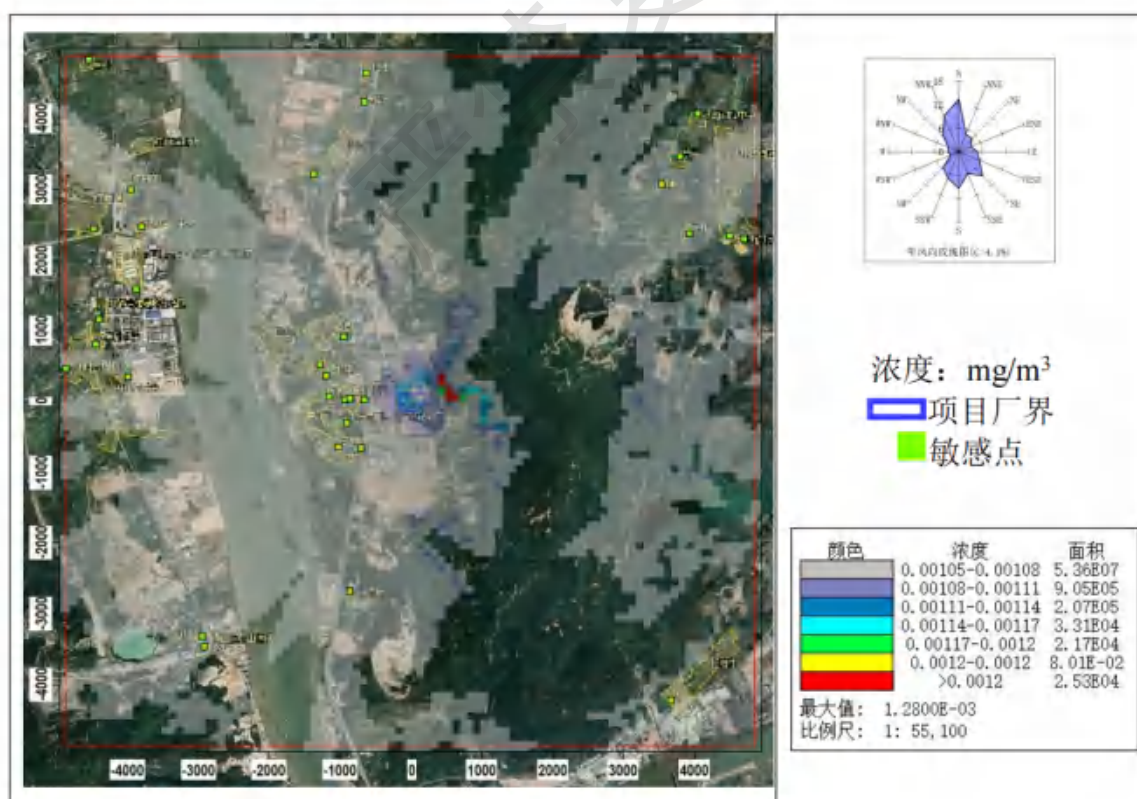
图 8.2-48 氟化物日平均浓度分布图（叠加在建、拟建源及背景后）
