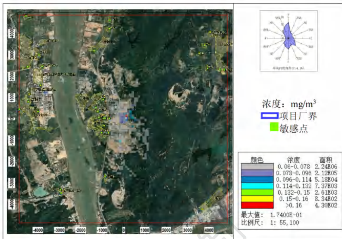
图 8.2-43 氨气小时平均浓度分布图（叠加在建、拟建源及背景后）
