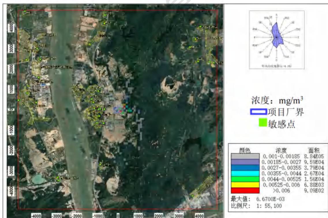
图 8.2-36 HCl 小时平均浓度分布图
