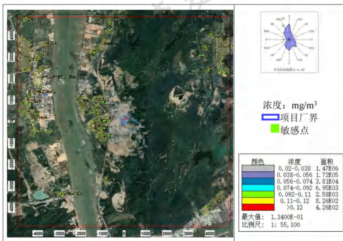
图 8.2-65 氨小时平均浓度分布图（非正常排放状况）
