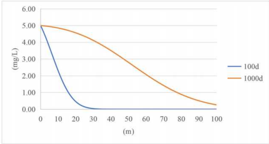
图 8.3-4 污染物连续渗漏情况预测统计图（镍）
