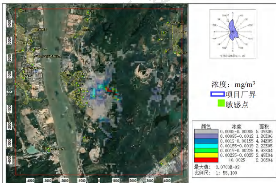
图 8.2-20 \text{PM}_{10} 日平均浓度分布图
