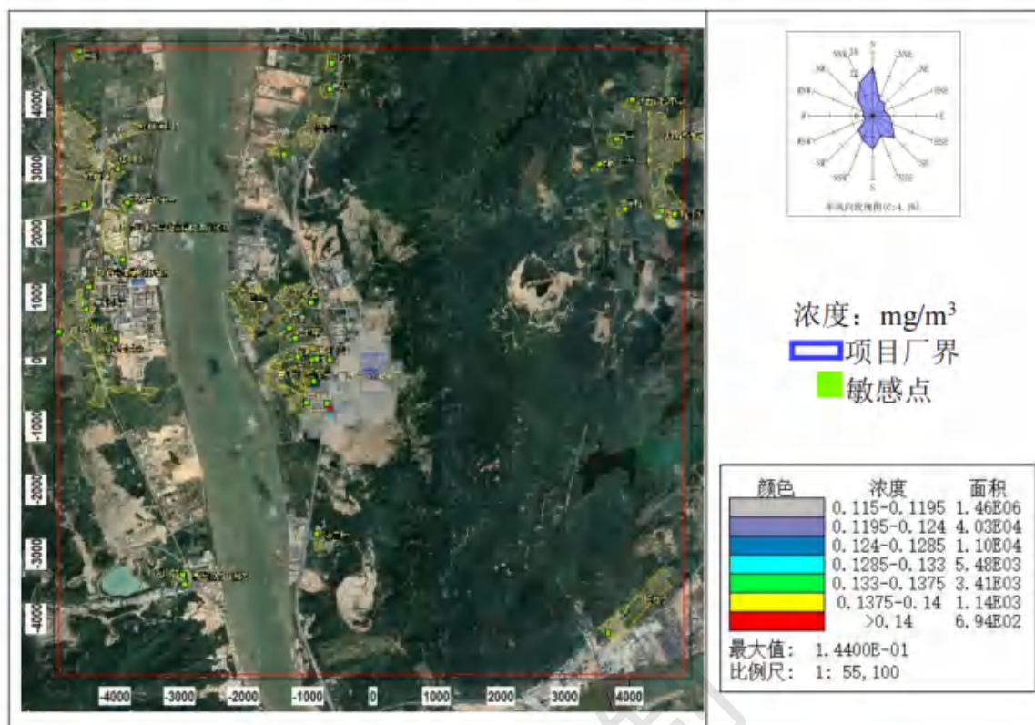
图 8.2-19 TSP 年平均浓度分布图（叠加在建、拟建源及背景后）
