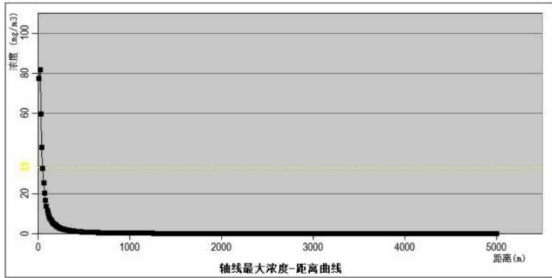
图 9.6-1 盐酸泄露产生的 HCl 在下风向不同距离处的最大浓度（最不利气象条件）
