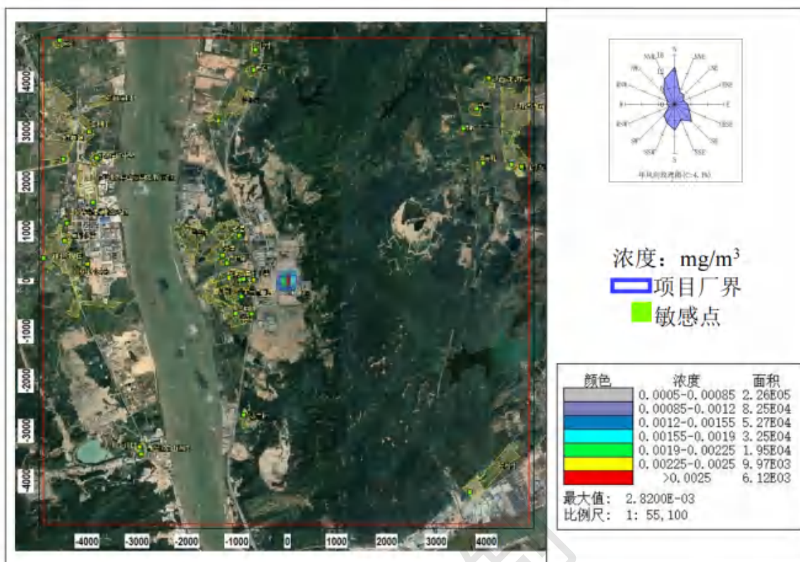
图 8.2-17 TSP 年平均浓度分布图
