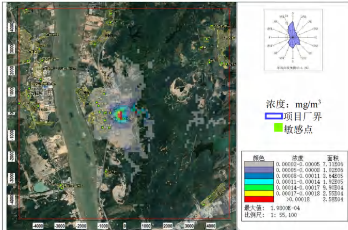
图 8.2-25 \text{PM}_{2.5} 年平均浓度分布图
