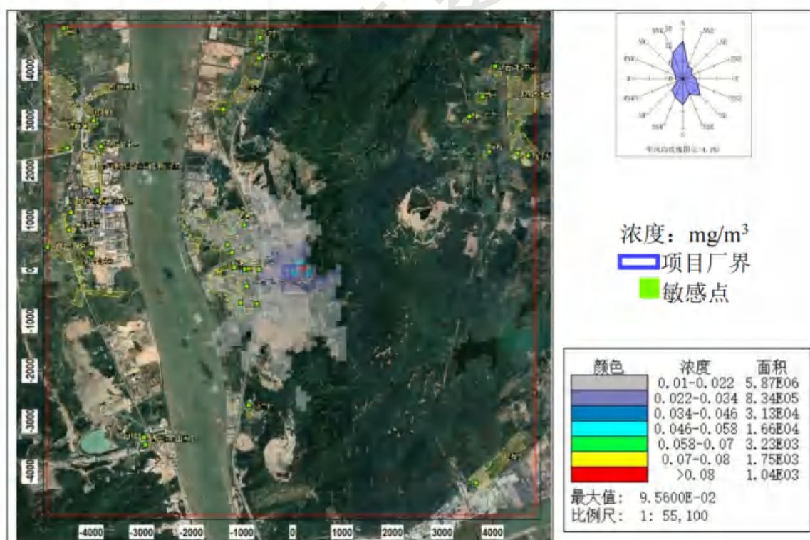
图 8.2-57 TSP 小时平均浓度分布图（非正常排放状况）
