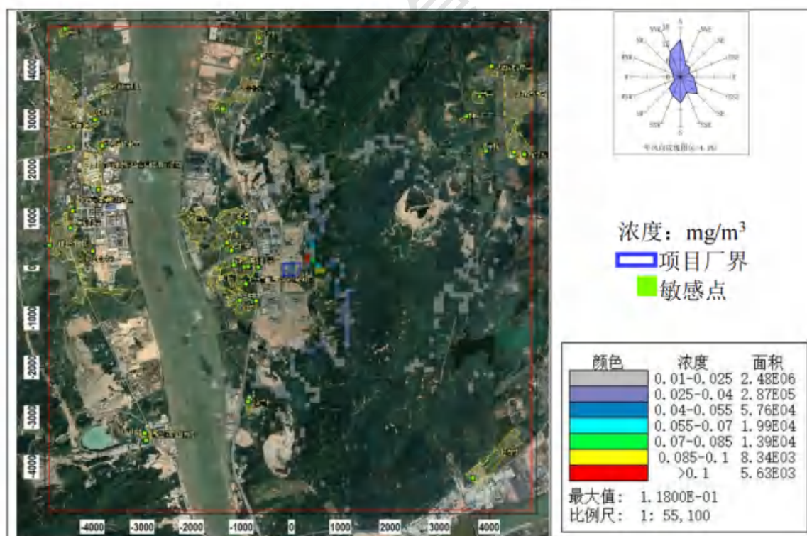
图 8.2-61 TVOC 小时平均浓度分布图（非正常排放状况）
