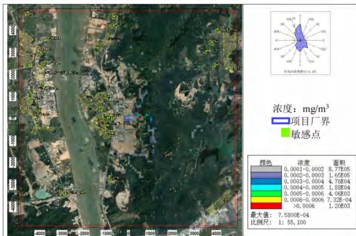
图 8.2-49 硫化氢小时平均浓度分布图
