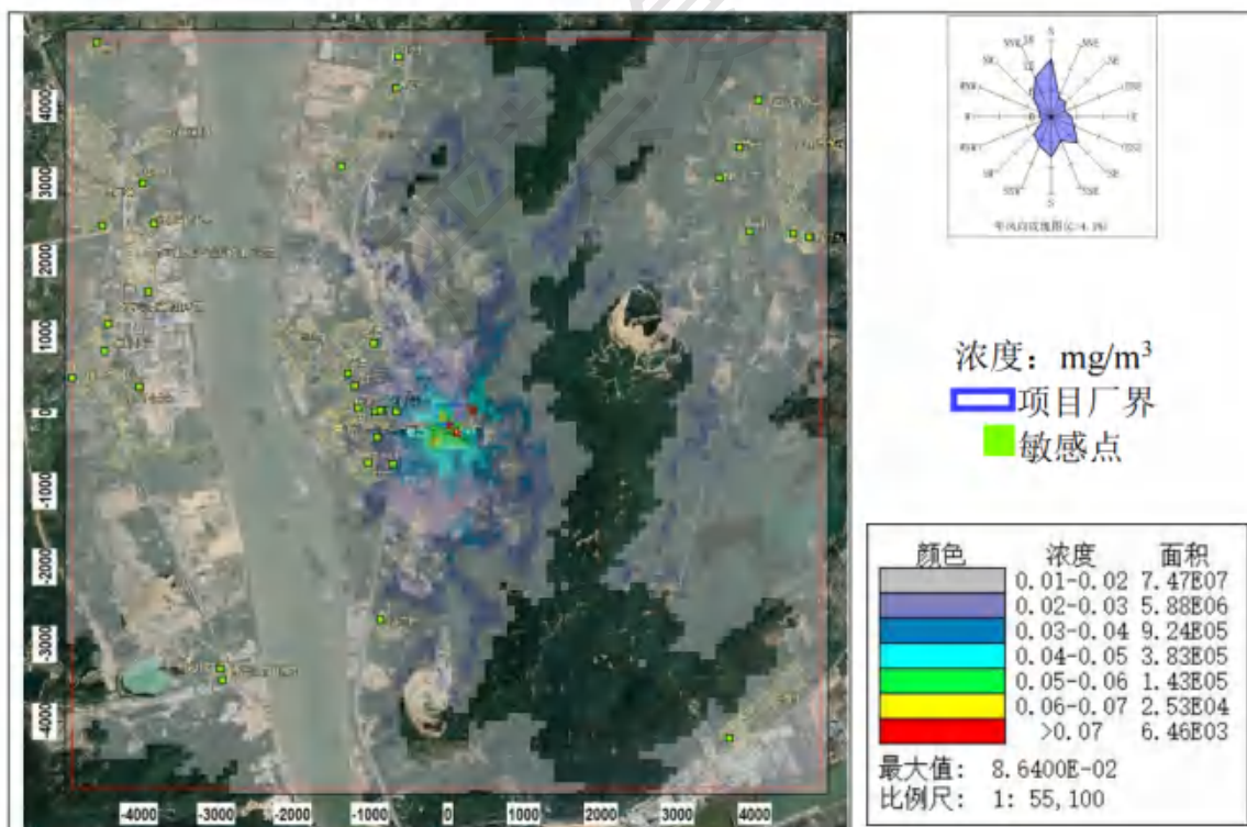
图 8.2-34 硫酸雾小时平均浓度分布图（叠加在建、拟建源及背景后）
