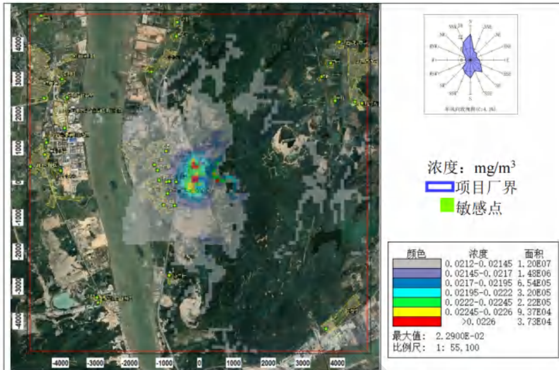
图 8.2-15 \text{NO}_2 年平均浓度分布图 (叠加在建、拟建源及背景后)
