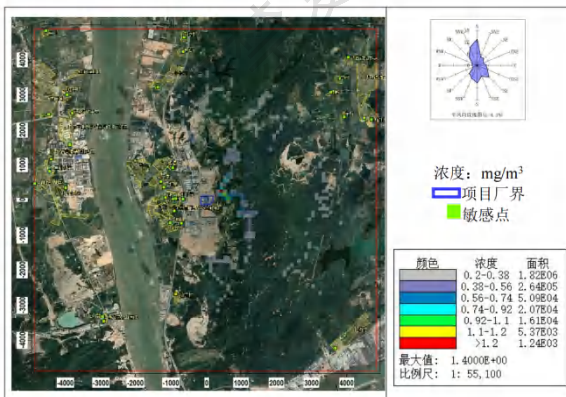
图 8.2-67 氟化物小时平均浓度分布图（非正常排放状况）
