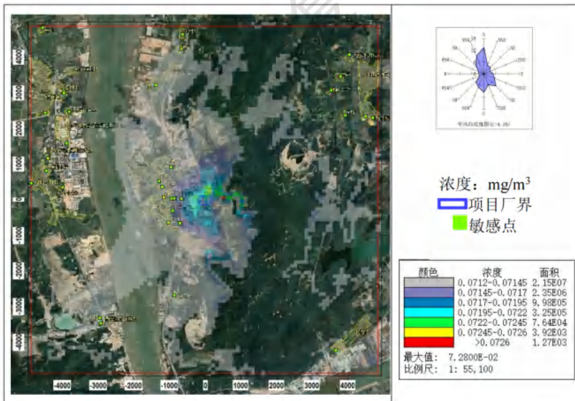
图 8.2-22 \text{PM}_{10} 日平均浓度分布图 (叠加在建、拟建源及背景后)
