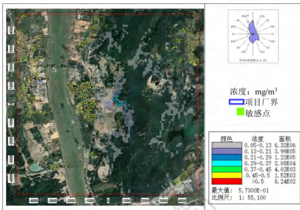
图 8.2-62 硫酸雾小时平均浓度分布图（非正常排放状况）
