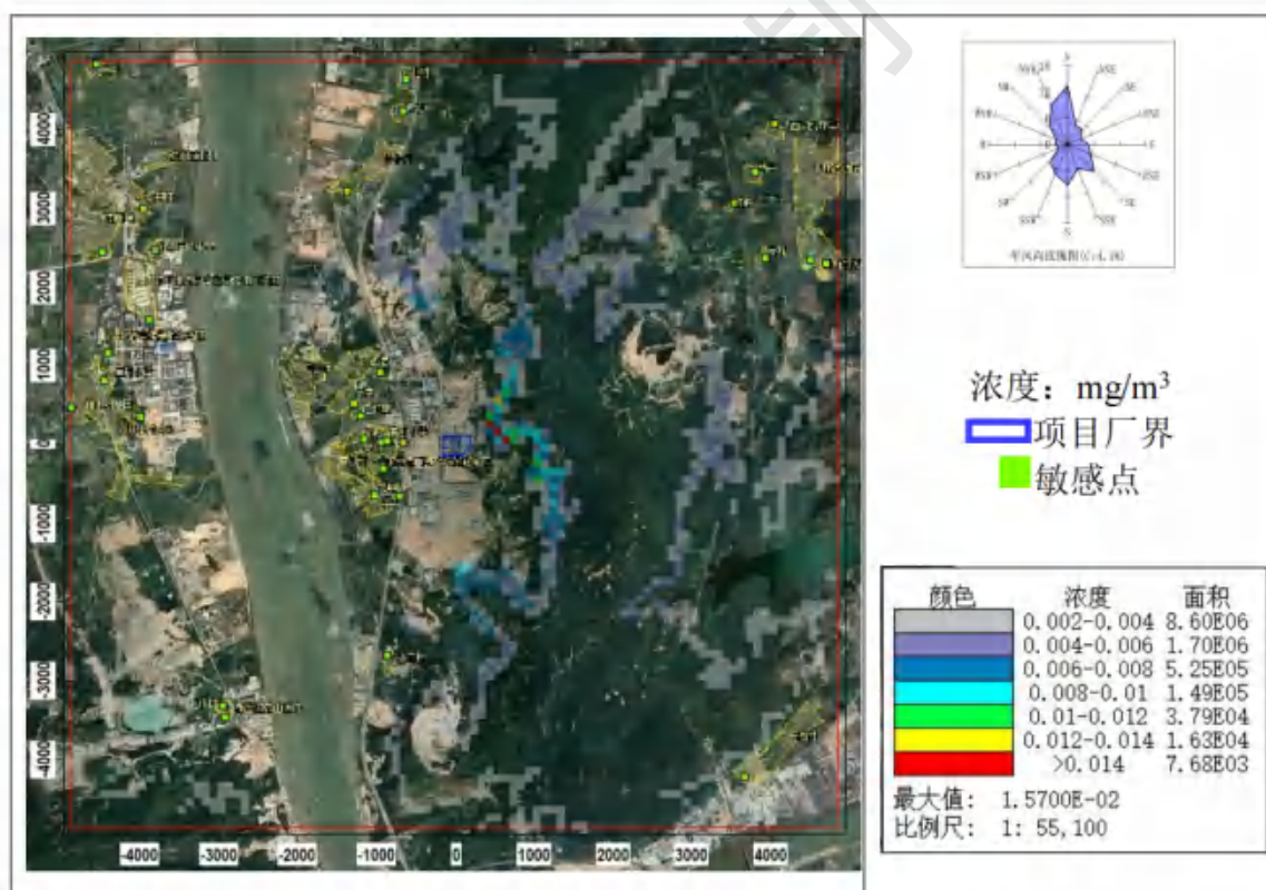
图 8.2-55 \text{SO}_2 小时平均浓度分布图（非正常排放状况）
