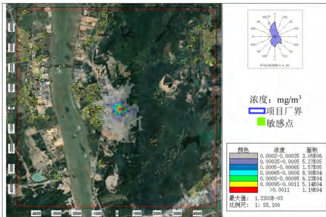
图 8.2-41 锰及其化合物日平均浓度分布图（叠加在建、拟建源及背景后）
