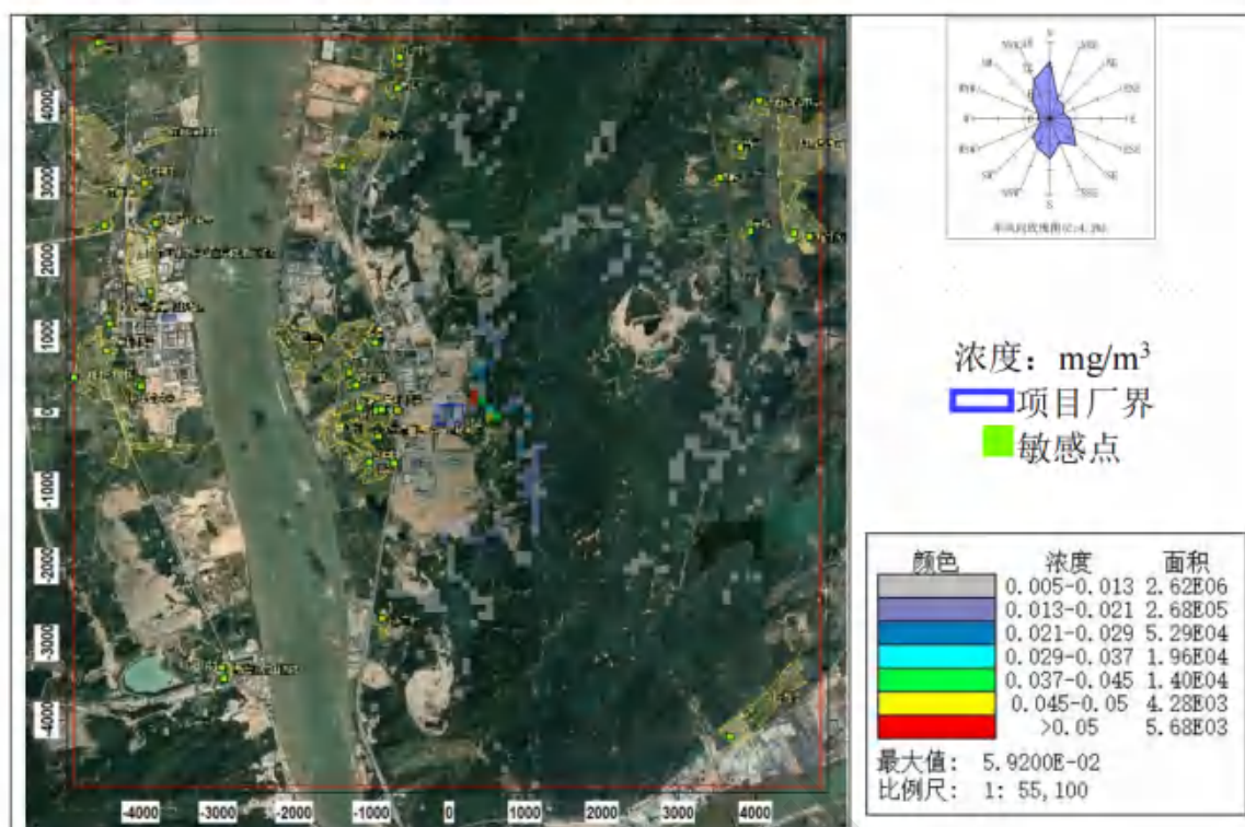
图 8.2-68 硫化氢小时平均浓度分布图（非正常排放状况）
