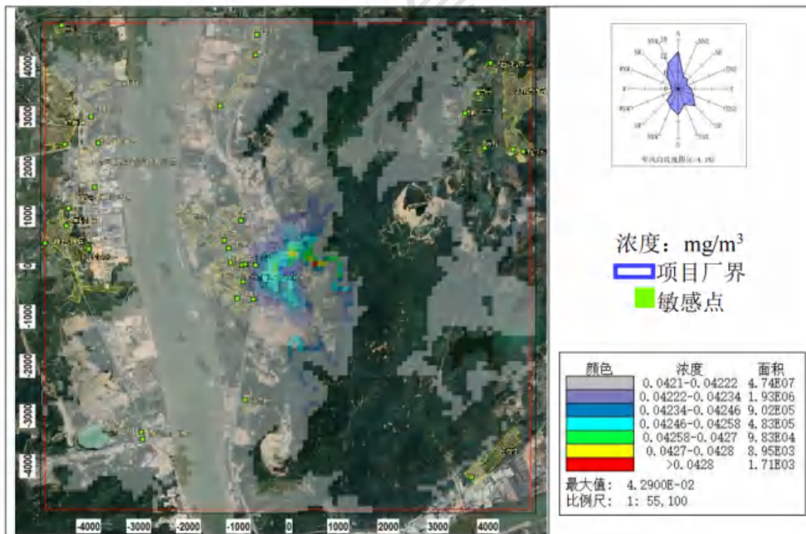
图 8.2-26 \text{PM}_{2.5} 日平均浓度分布图（叠加在建、拟建源及背景后）
