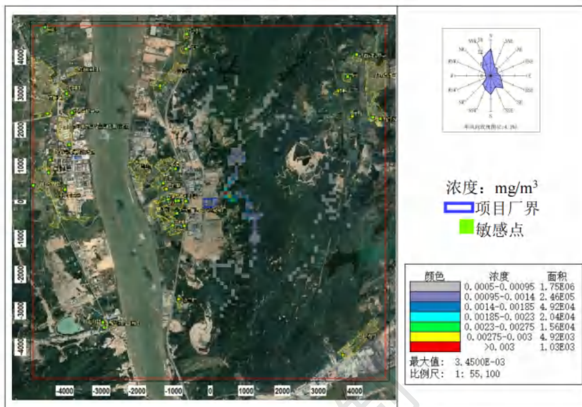
图 8.2-66 二噁英小时平均浓度分布图（非正常排放状况）
