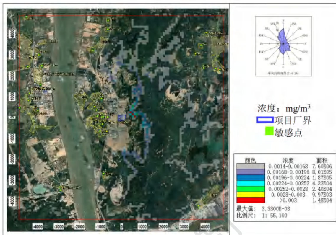
图 8.2-47 氟化物小时平均浓度分布图（叠加在建、拟建源及背景后）
