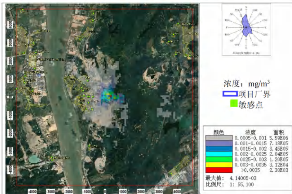
图 8.2-33 硫酸雾日平均浓度分布图
