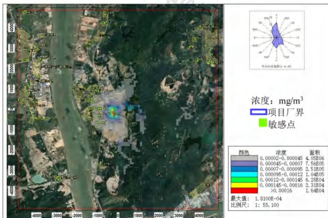
图 8.2-8 \text{SO}_2 年平均浓度分布图 (本项目贡献值)
