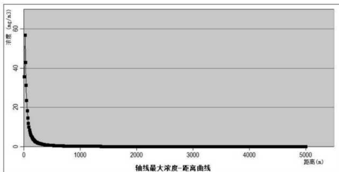
图 9.6-5 氨水泄露产生的氨气在下风向不同距离处的最大浓度（最不利气象条件）
