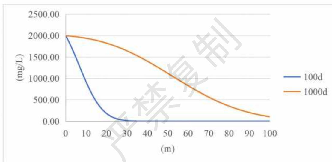
图 8.3-3 污染物连续渗漏情况预测统计图（氟化物）
