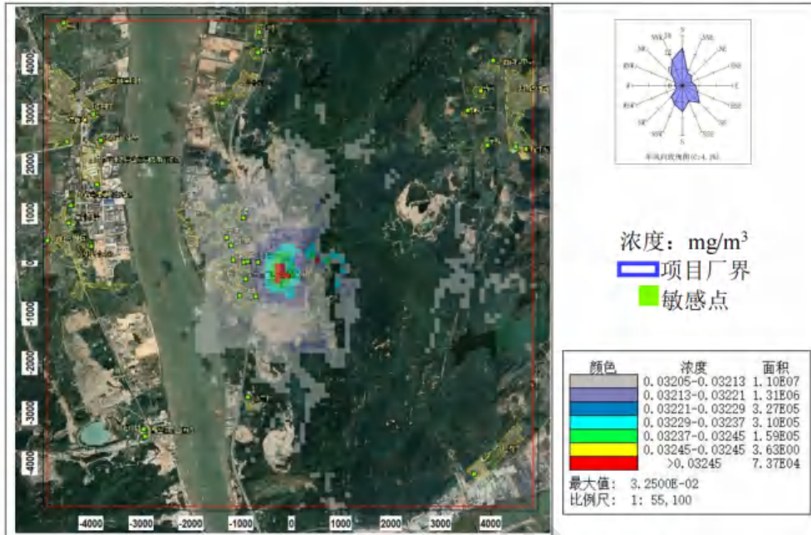
图 8.2-23 \text{PM}_{10} 年平均浓度分布图（叠加在建、拟建源及背景后）
