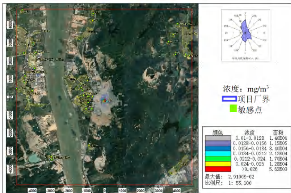
图 8.2-35 硫酸雾日平均浓度分布图（叠加在建、拟建源及背景后）
