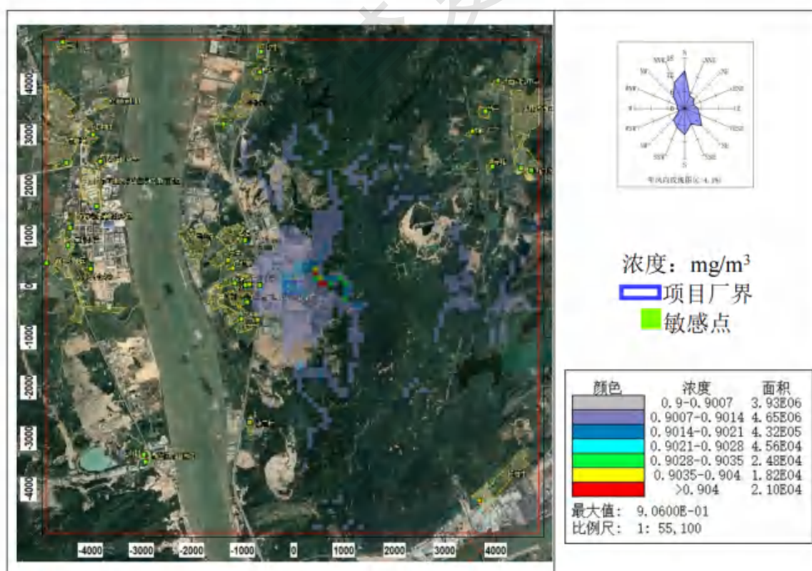
图 8.2-54 CO 日平均浓度分布图 (叠加在建、拟建源及背景后)
