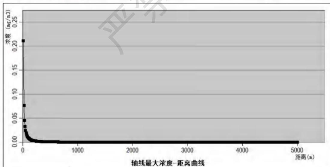
图 9.6-9 二氧化硫泄漏事故排放在下风向不同距离处的最大浓度（最不利气象条件）
