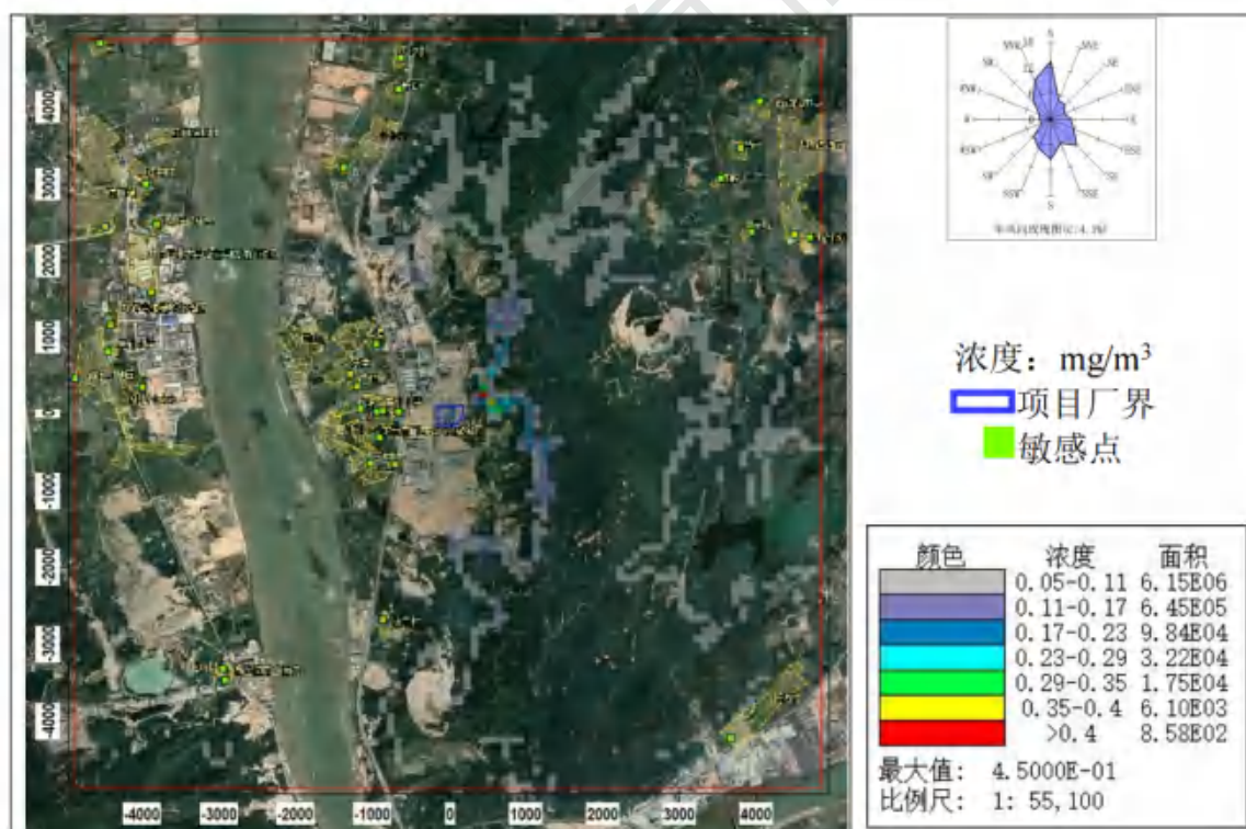
图 8.2-69 镍及其化合物小时平均浓度分布图（非正常排放状况）
