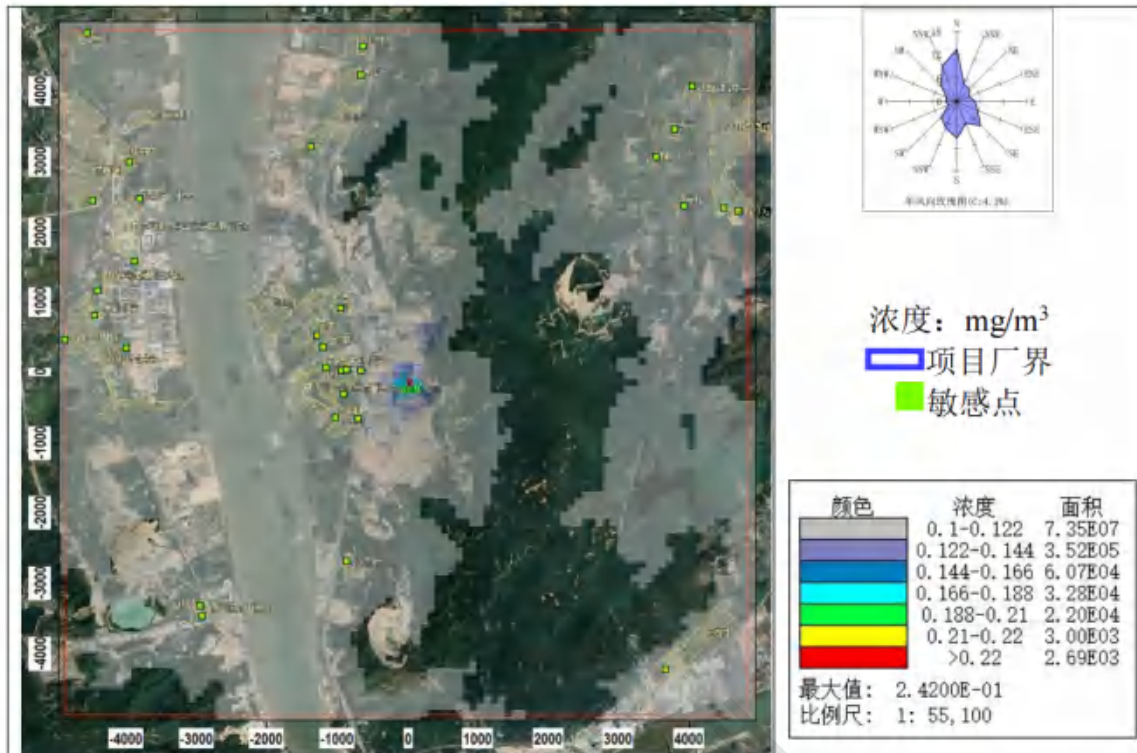
图 8.2-31 TVOC 8 小时平均浓度分布图（叠加在建、拟建源及背景后）
