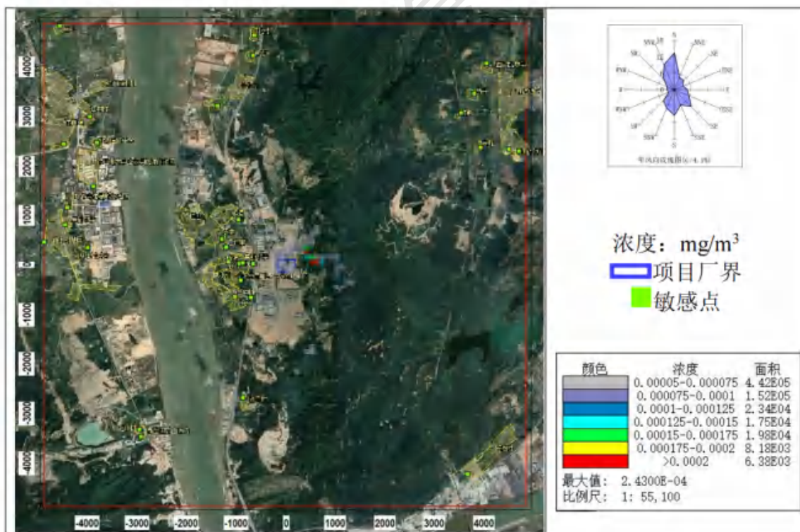
图 8.2-46 氟化物日平均浓度分布图
