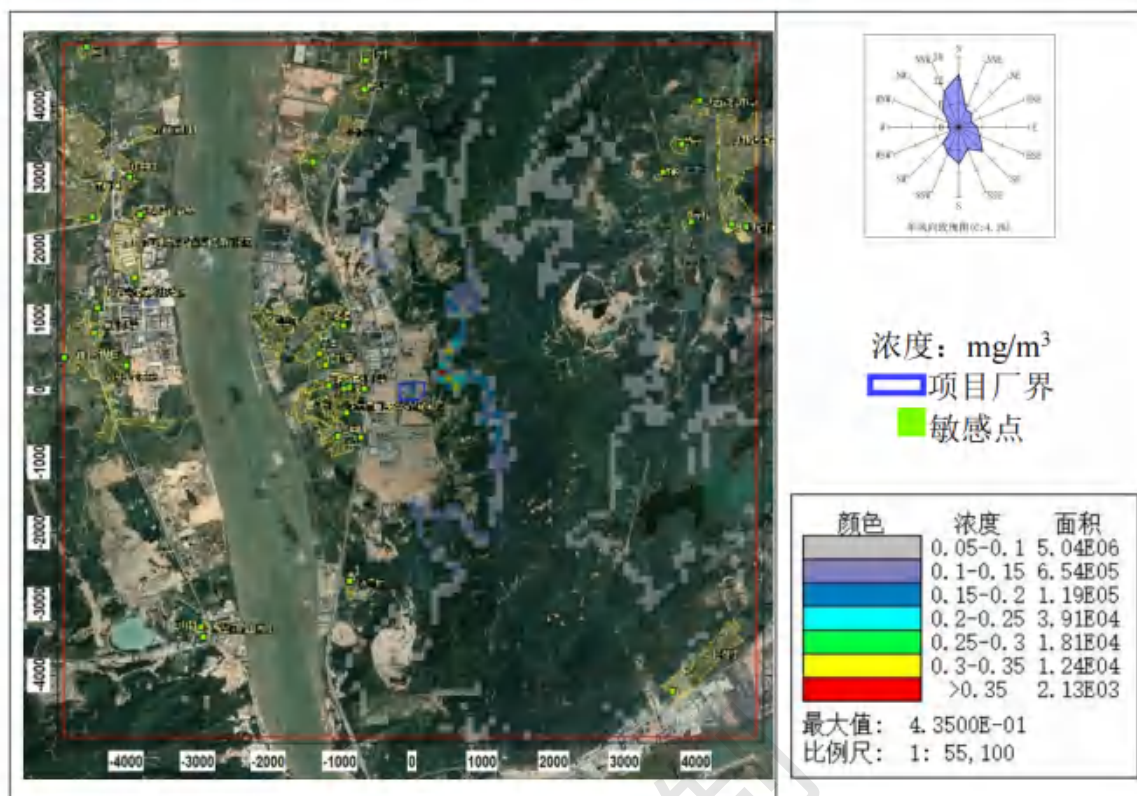
图 8.2-56 \text{NO}_2 小时平均浓度分布图（非正常排放状况）
