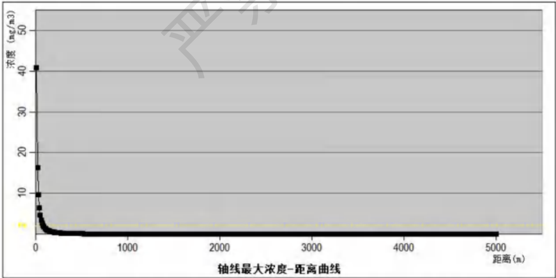
图 9.6-10 二氧化硫泄漏事故排放在下风向不同距离处的最大浓度（最常见气象条件）
