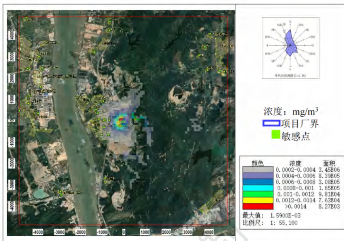
图 8.2-13 \text{NO}_2 年平均浓度分布图
