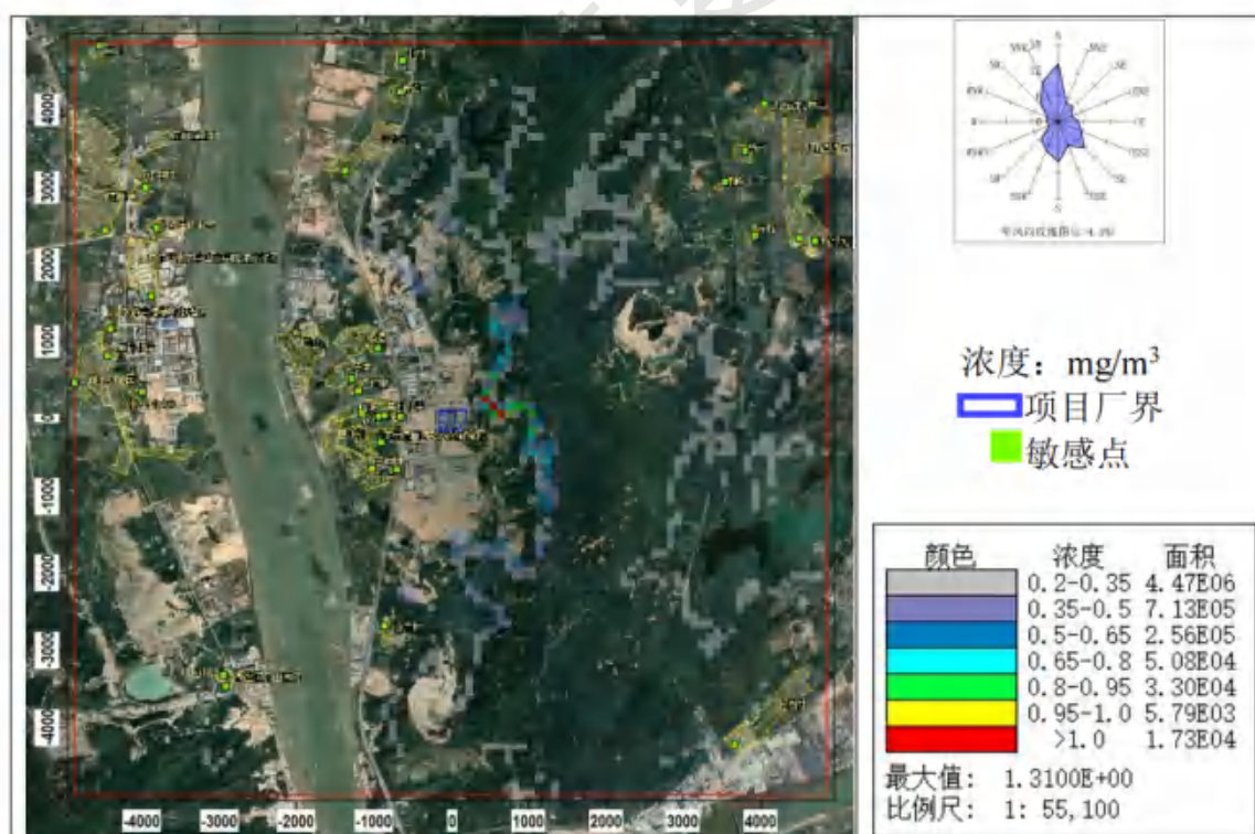
图 8.2-59 \text{PM}_{2.5} 小时平均浓度分布图 (非正常排放状况)
