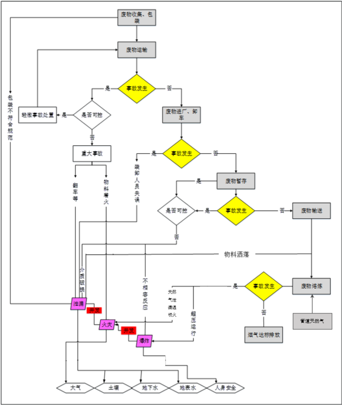
图 6.8.5.1-1 危险废物利用全过程事故树
