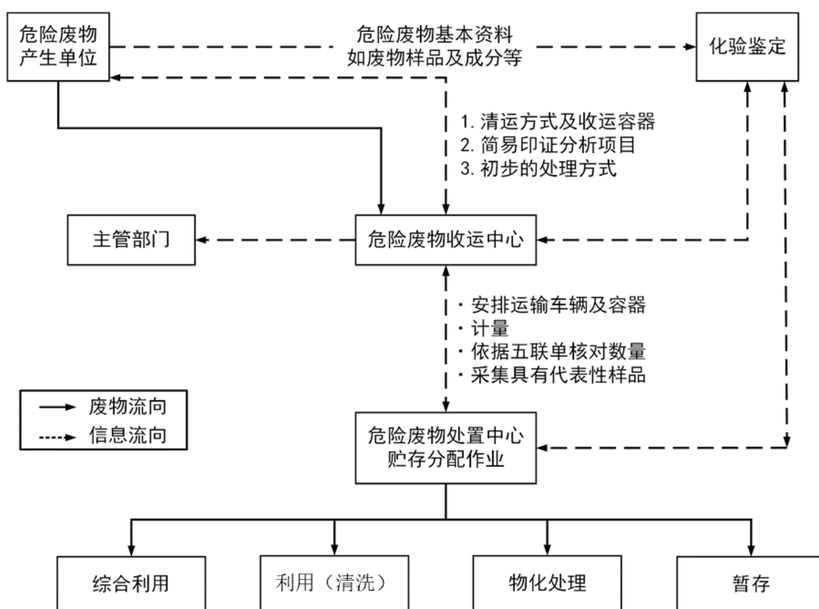
图 3.2.1-1 现有项目总体工艺流程图
