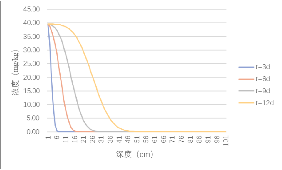
图 6.6.7-1 土壤垂直入渗贡献值图
