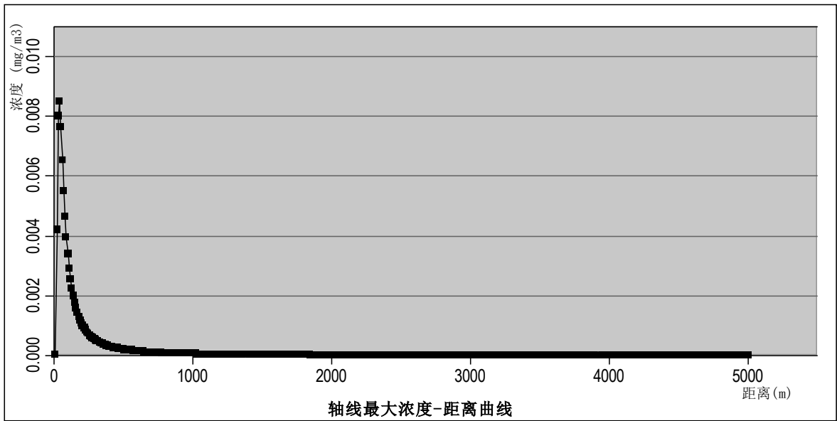
图 6.8.6.2-1 天然气泄漏火灾事故产生 CO 预测轴线最大浓度结果图
