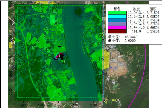
二氧化硫保证率日均值
