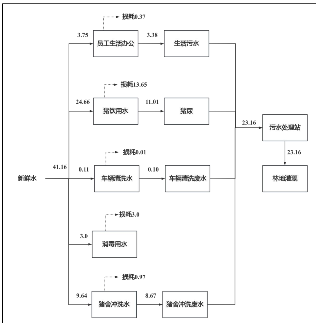
图 3.3-1 建设项目水平衡图
