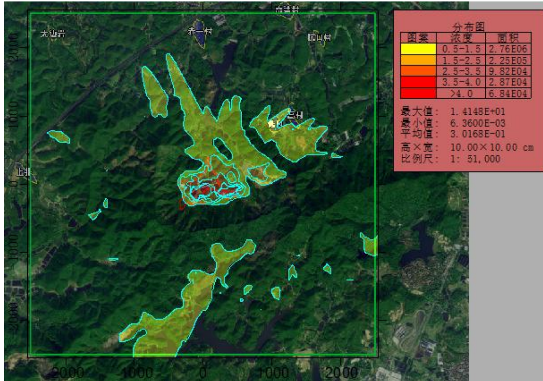
图 5.2-10 NO x 日平均贡献浓度分布图
