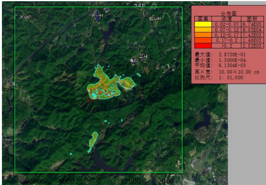
图 5.2-12 \text{PM}_{10} 日平均贡献浓度分布图
