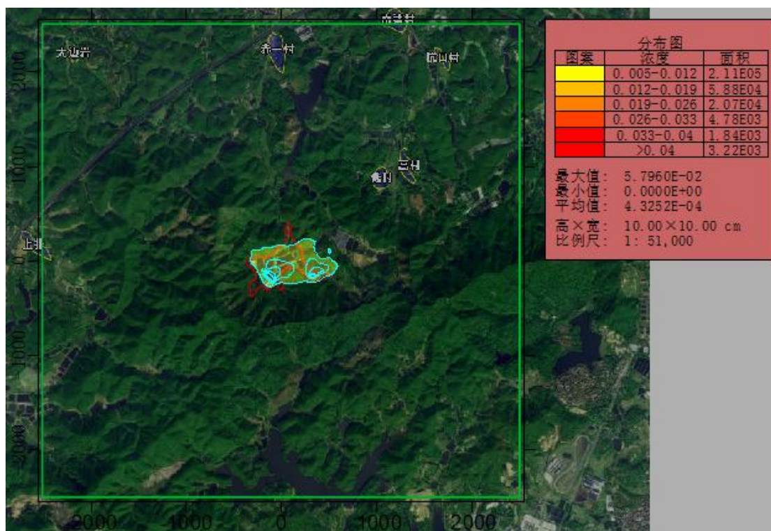
图 5.2-9 SO 2 年平均贡献浓度分布图
