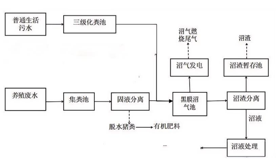
图 3.2-5 沼气工艺流程图
