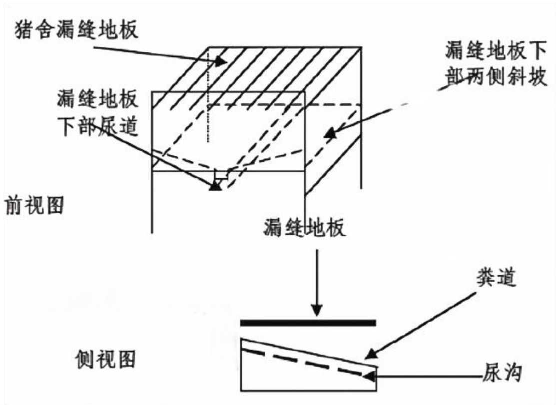
图 3.2-4 项目干清粪工艺结构图
