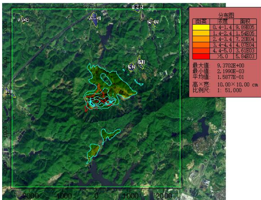
图 5.2-18 叠加环境影响后 \text{NO}_x 的 98%保证率日均质量浓度分布图
