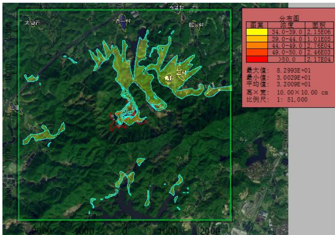
图 5.2-23 叠加环境影响后 \text{NH}_3 的最大小时平均质量浓度分布图
