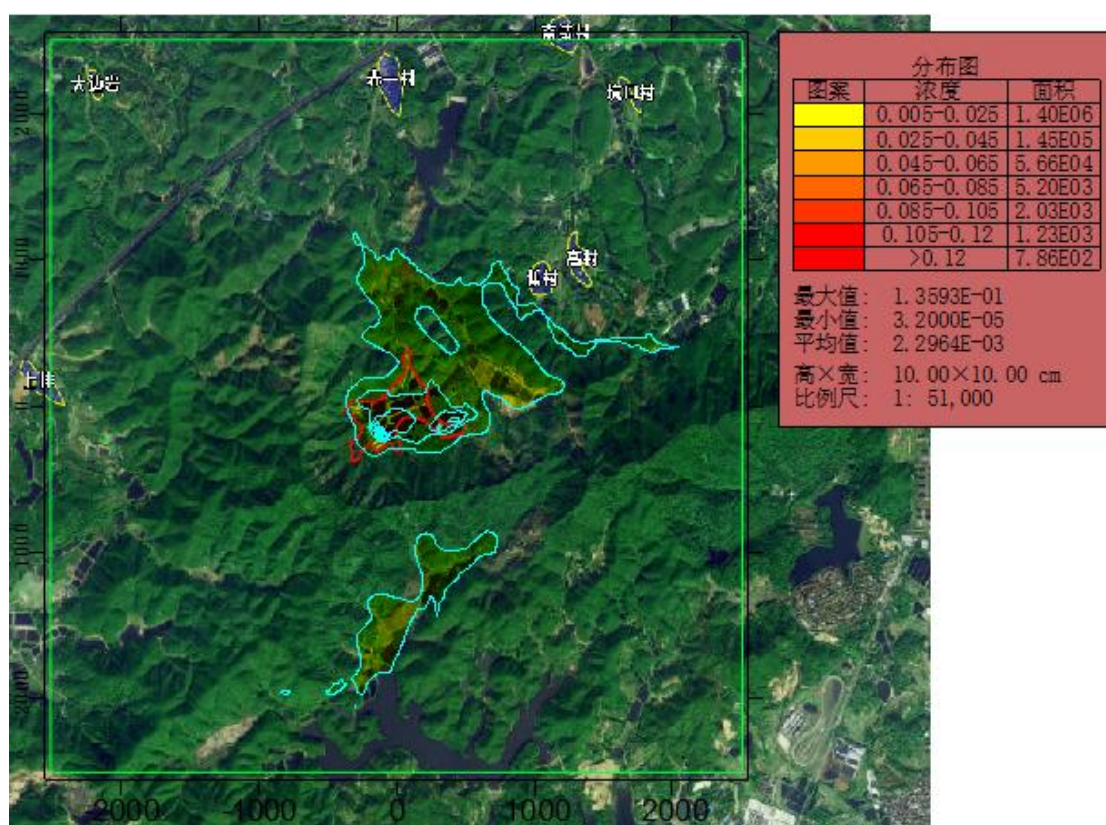
图 5.2-16 叠加环境影响后 SO 2 的 98%保证率日均质量浓度分布图
