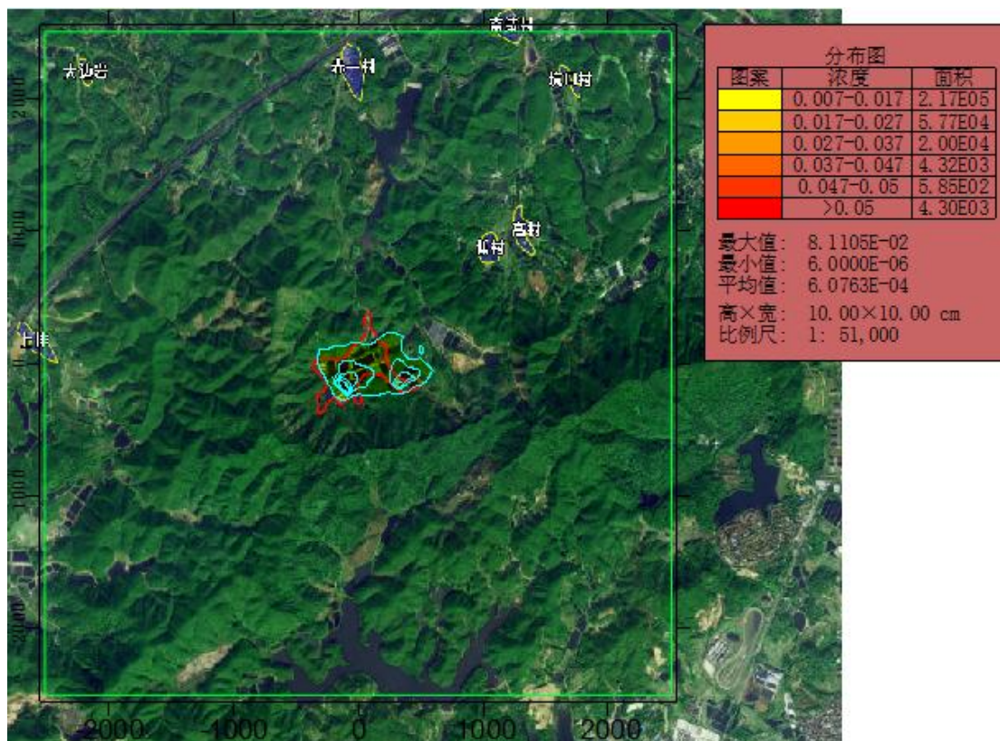
图 5.2-21 叠加环境影响后 PM_{10} 的年平均质量浓度分布图
