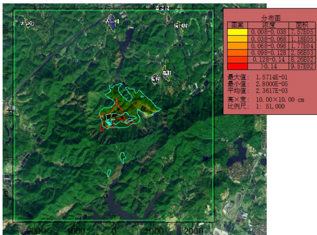
图 5.2-20 叠加环境影响后 \text{PM}_{10} 的 95%保证率日均质量浓度分布图
