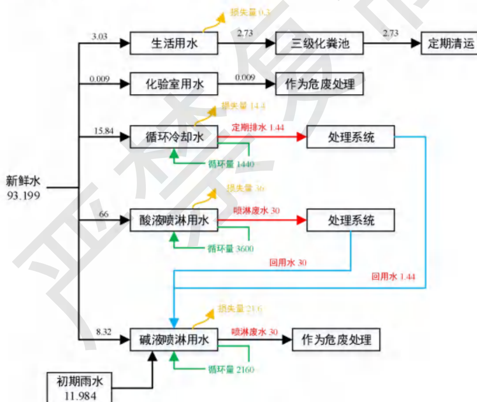
图 3.1-2 全厂水平衡图
