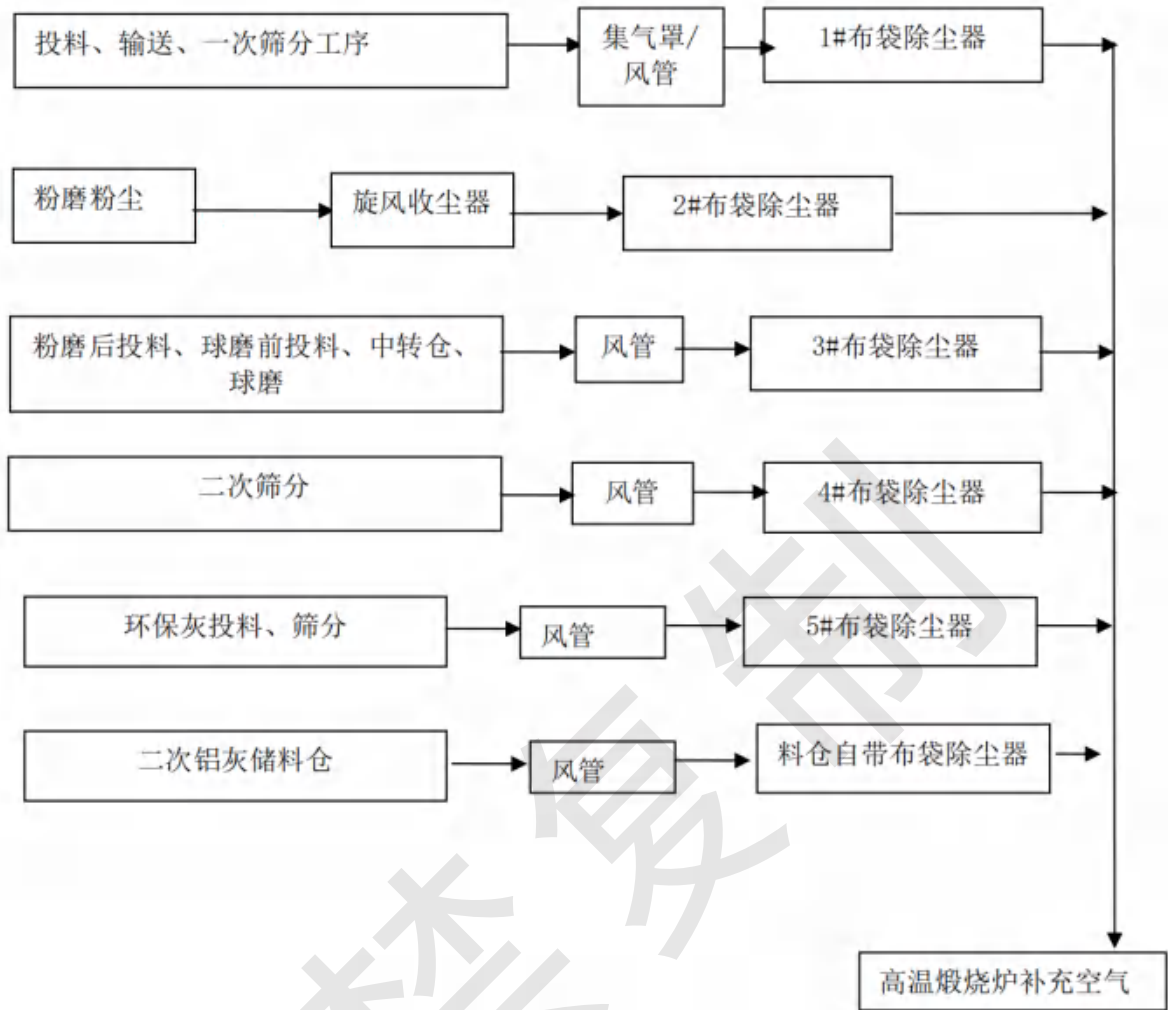
图 8.2-3 球磨生产线粉尘收集示意图
