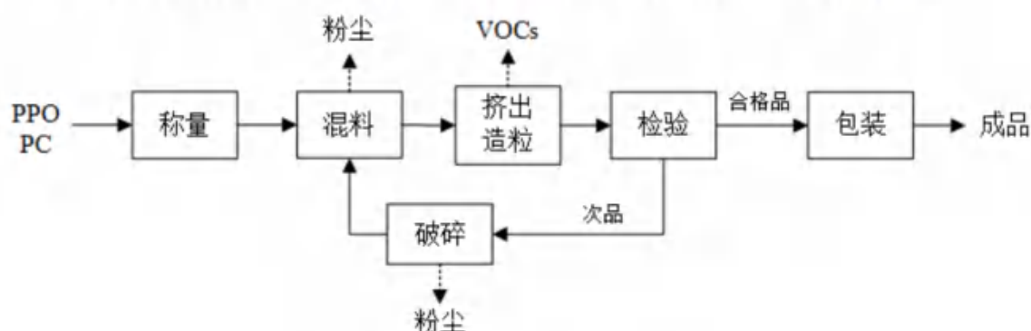
图 1.1-7 改性塑料生产工艺流程图
