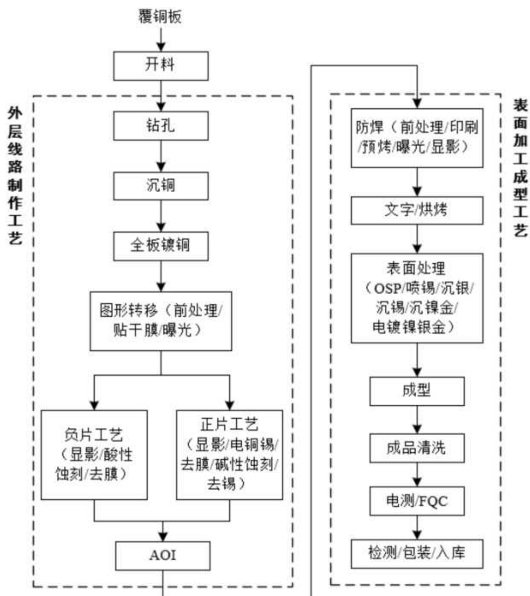
图 1.7-1 IC载板生产工艺流程图
