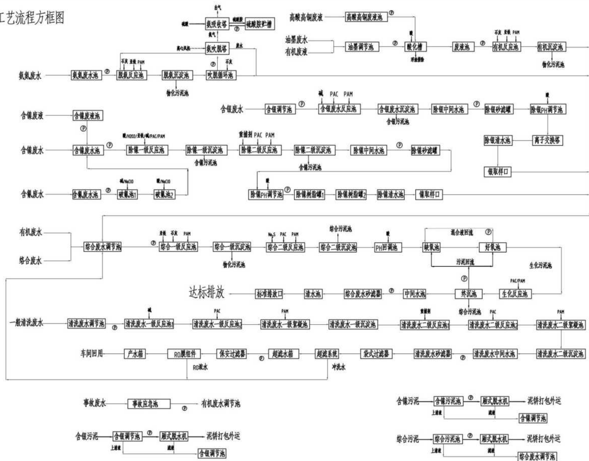
图 1.11-1 本项目生产废水处理系统工艺流程图
