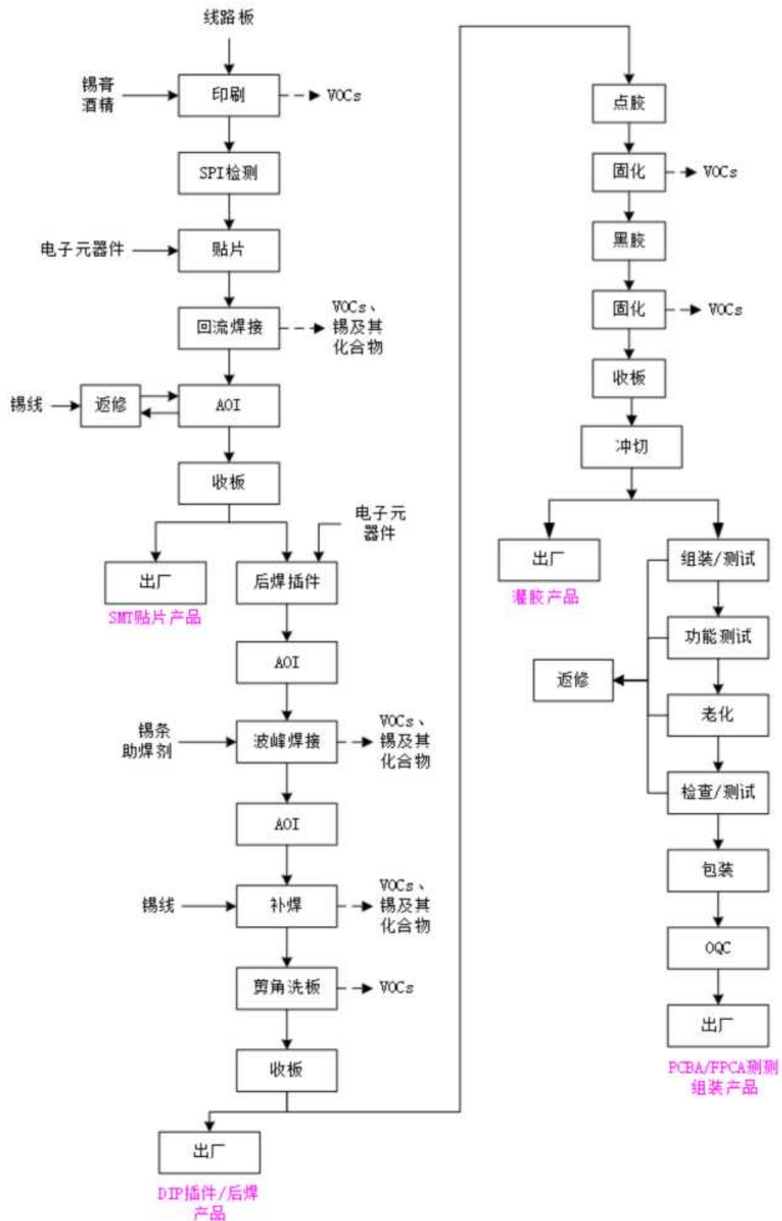
图 1.7-6 SMT 工艺流程及产污节点图
