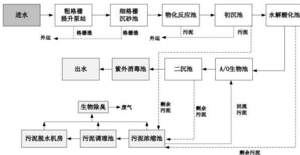
图 1.11-2 一期工程水处理工艺流程简图
