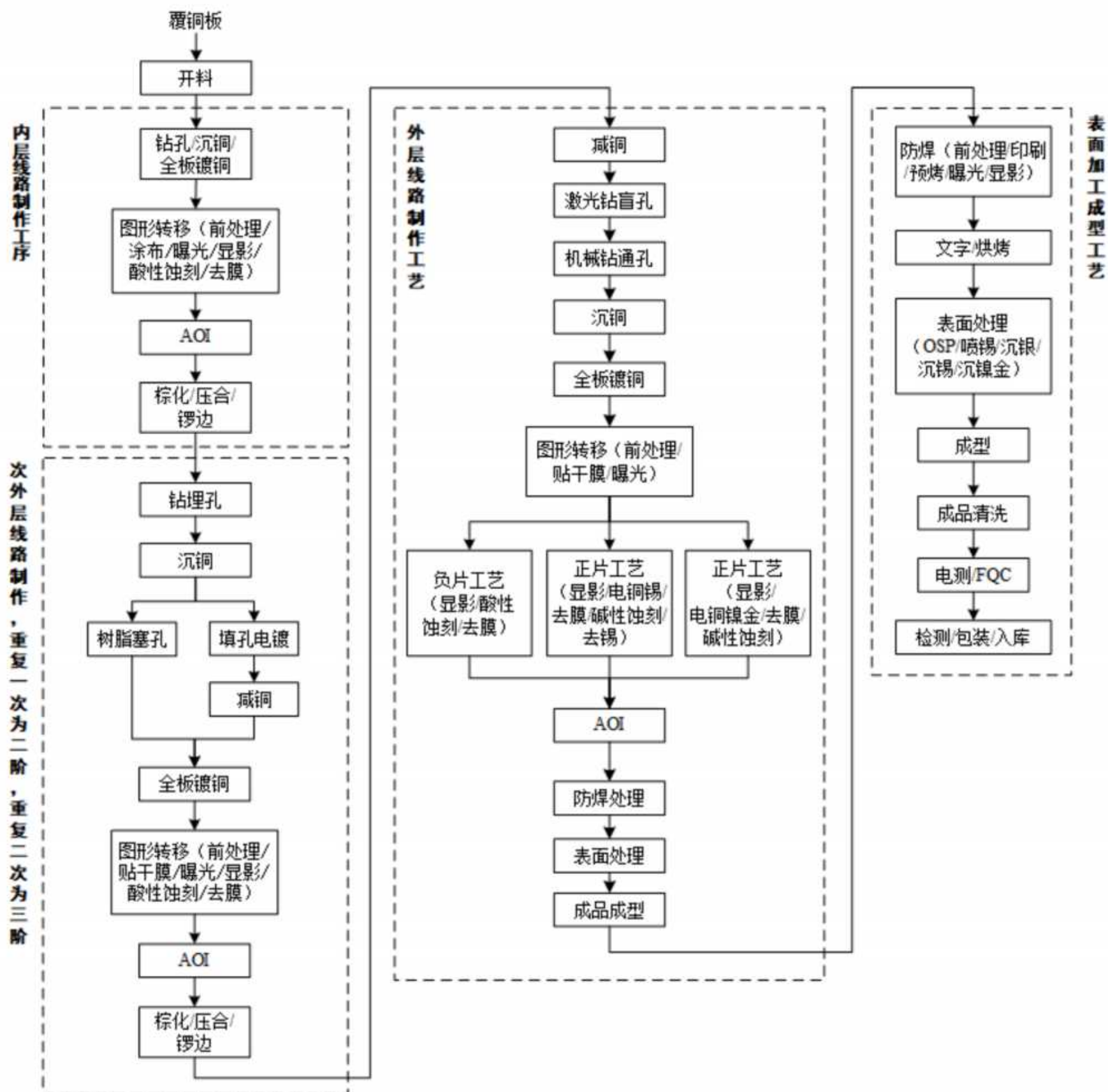
图 1.7-3 HDI板生产工艺流程图
