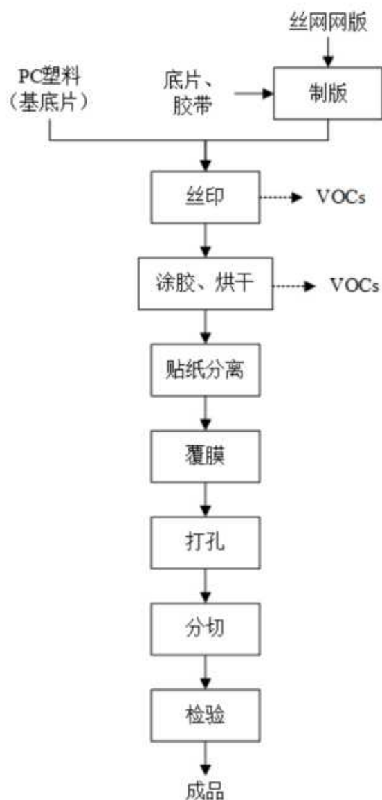
图 1.1-8 LED面膜生产工艺流程图
