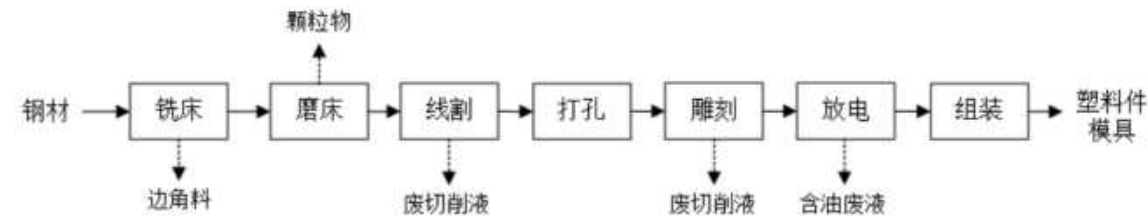
图 1.1-5 模具加工工艺流程图
