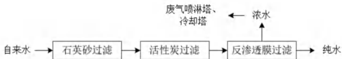
图 1.5-1 本项目纯水系统工艺流程图
