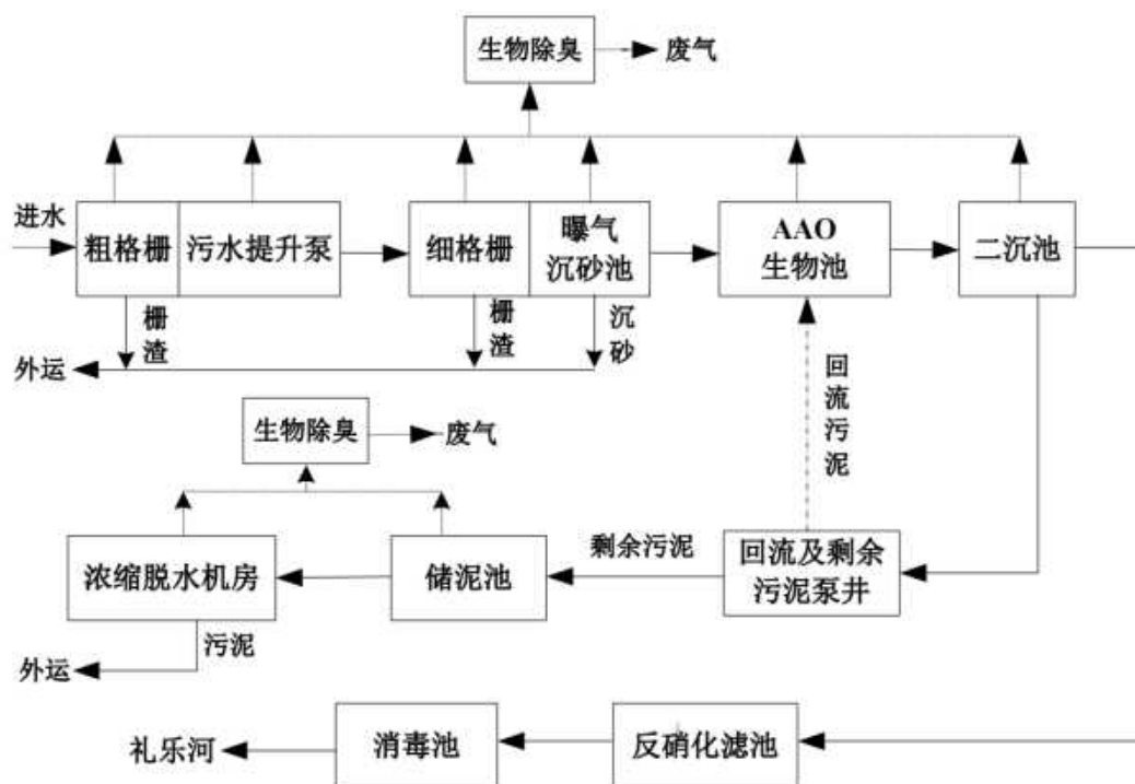
图 1.11-3 二期工程水处理工艺流程简图
