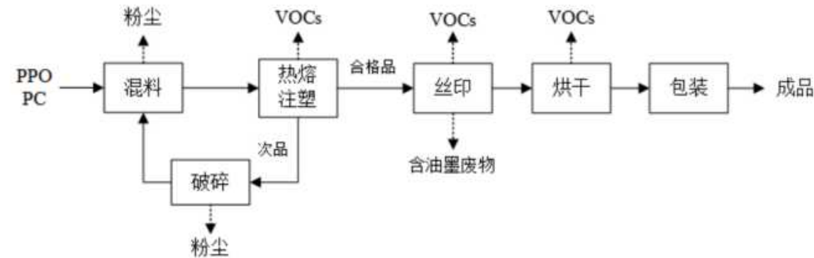
图 1.1-6 塑胶盖子生产工艺流程图
