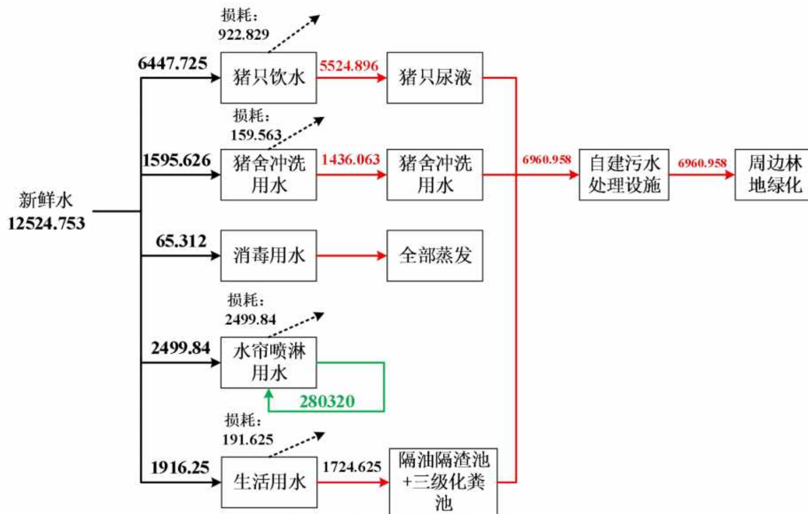
图3.4-1 项目水平衡图 单位: \text{m}^3/\text{a}
