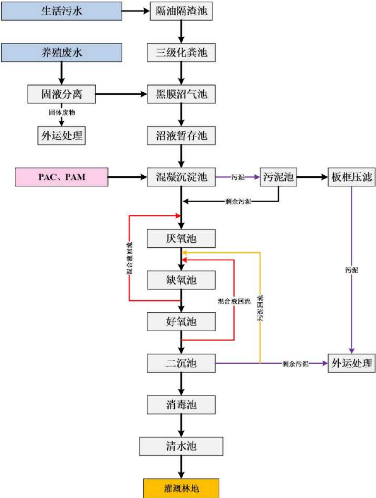
图 7.1-1 自建污水治理设施工艺流程图
