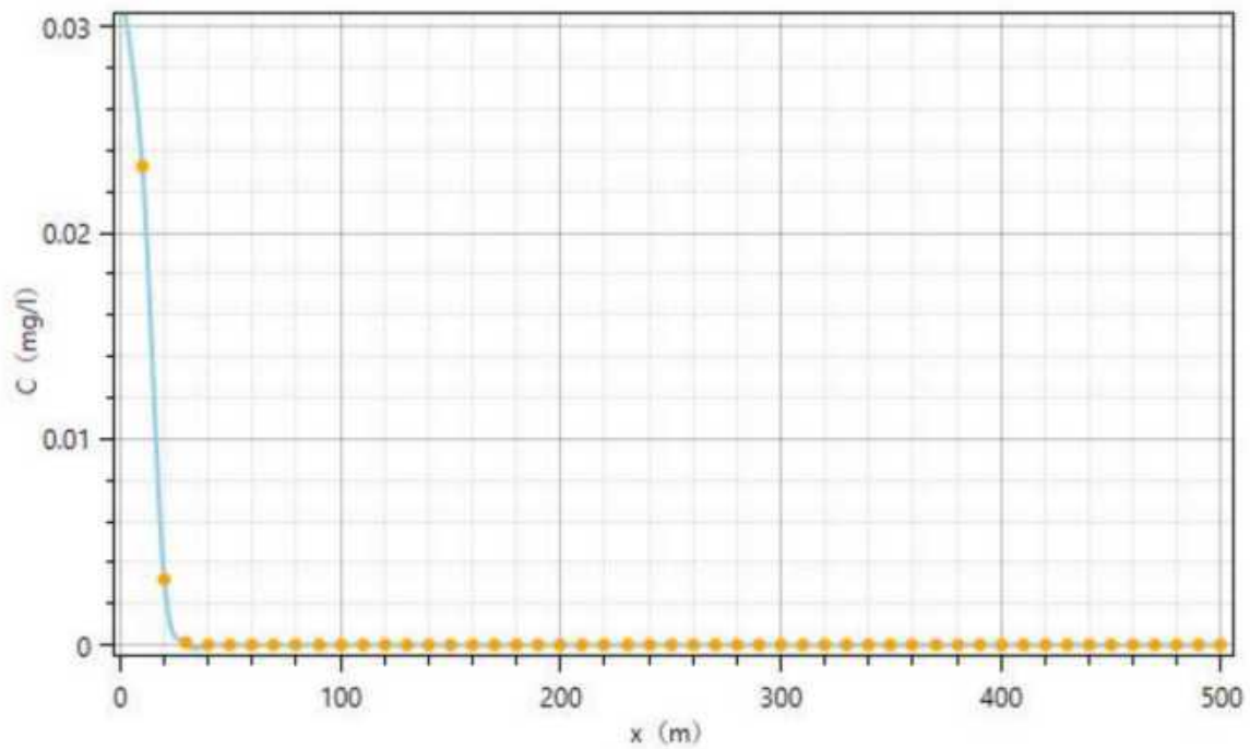
图 5.6-4 污水池渗漏 100d 后，下游不同距离的氨氮浓度分布
