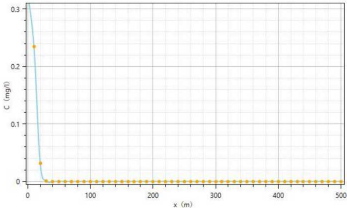
图 5.6-2 污水池渗漏 100d 后，下游不同距离的 COD 浓度分布
