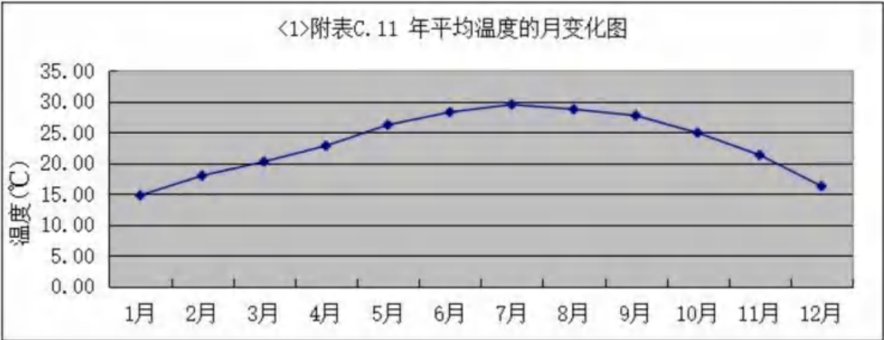
图 5.3-4 鹤山市 2023 年平均气温的月变化图
