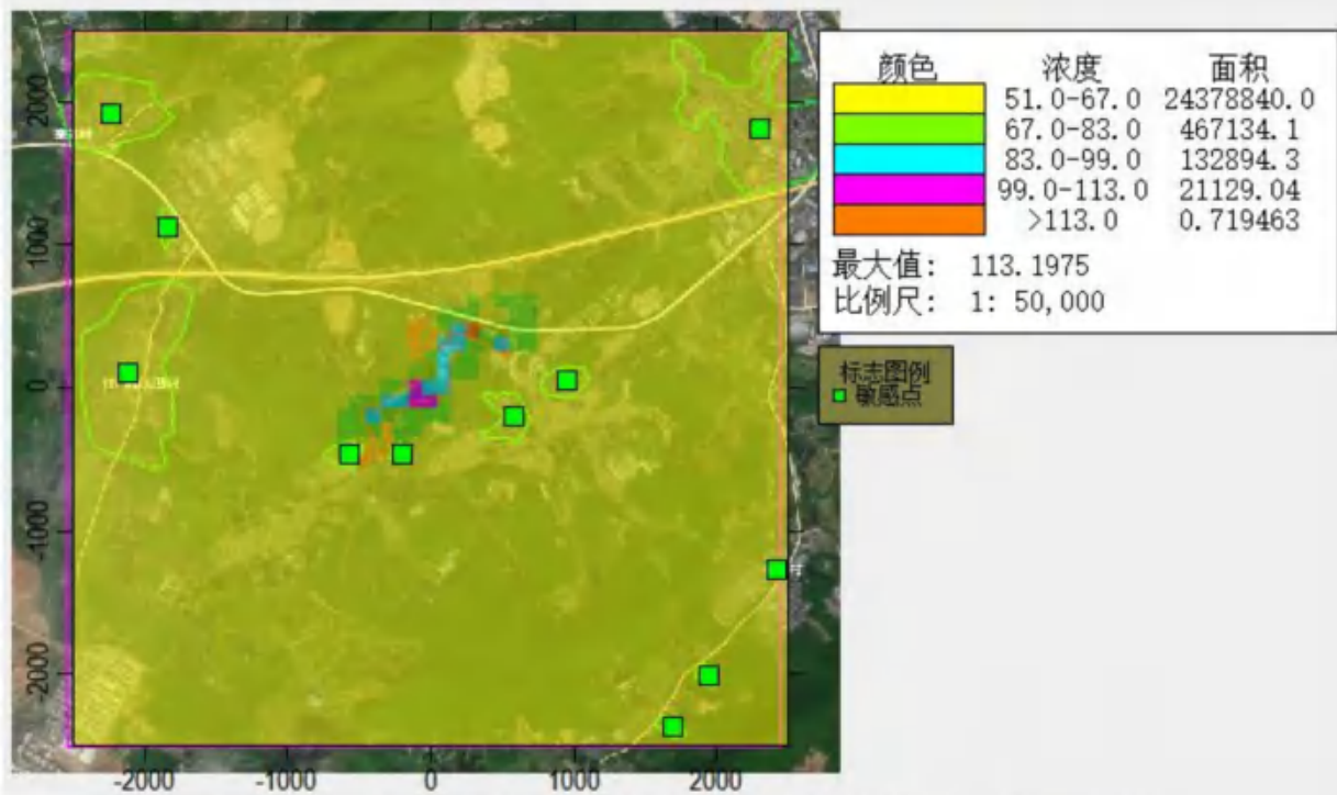
图 5.3-17 氨正常工况下小时平均浓度叠加值等值线图（单位： \mu\text{g}/\text{m}^3 ）
