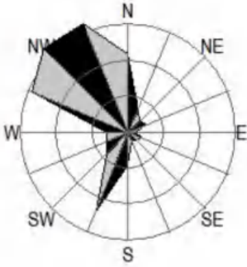
图 5.2-2 鹤山市气象站风向玫瑰图（统计年限：2004-2023 年）
