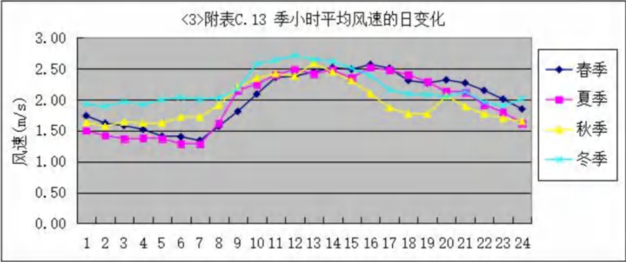
图 5.3-6 鹤山市 2023 年季小时平均风速的日变化图
