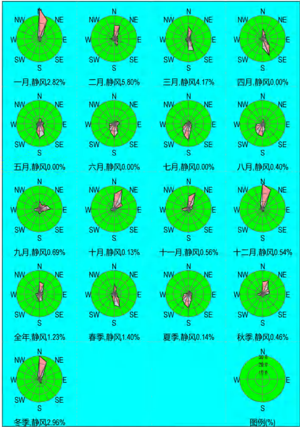
图 5.3-7 鹤山市 2023 年风频玫瑰图
