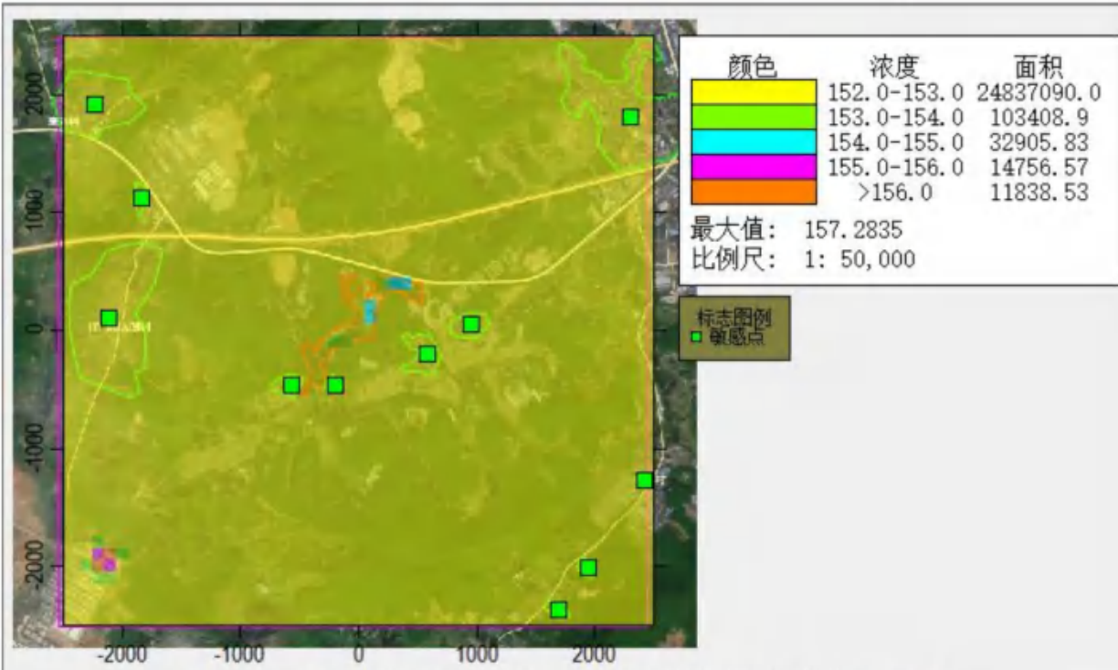
图 5.3-16 TSP 正常工况下年平均浓度叠加值等值线图 (单位: \mu\text{g}/\text{m}^3 )
