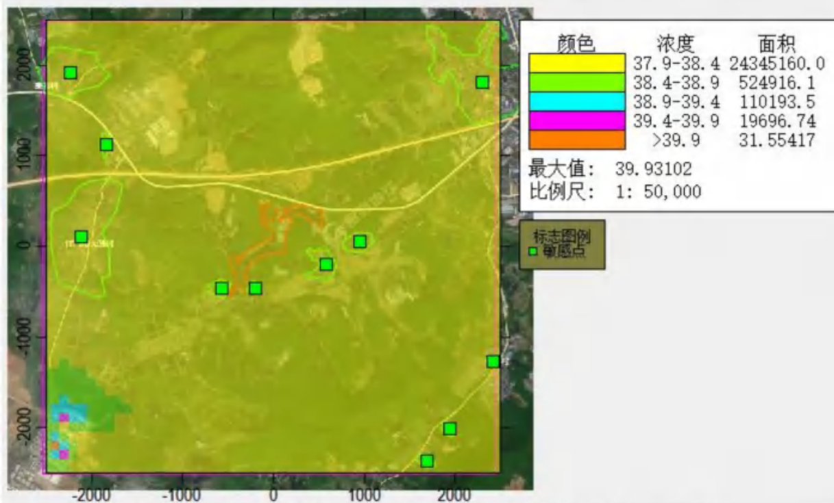
图 5.3-14 PM 10 正常工况下年平均浓度叠加值等值线图 (单位: \mu\text{g}/\text{m}^3 )
