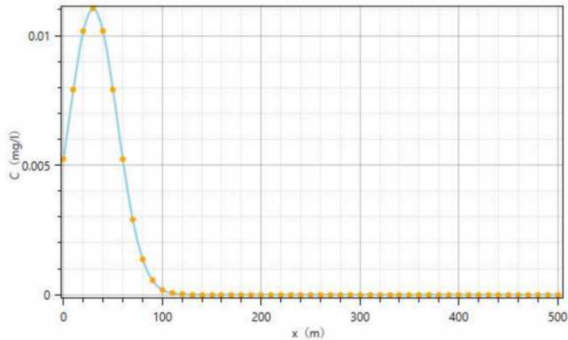
图 5.6-5 污水池渗漏 1000d 后，下游不同距离的氨氮浓度分布
