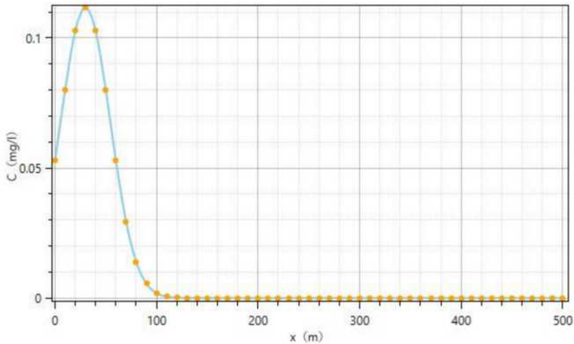
图 5.6-3 污水池渗漏 1000d 后，下游不同距离的 COD 浓度分布
