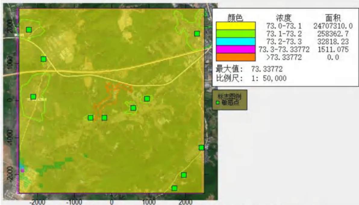
图 5.3-11 NO 2 正常工况下 98%保证率日均浓度等值线图 (单位: \mu\text{g}/\text{m}^3 )
