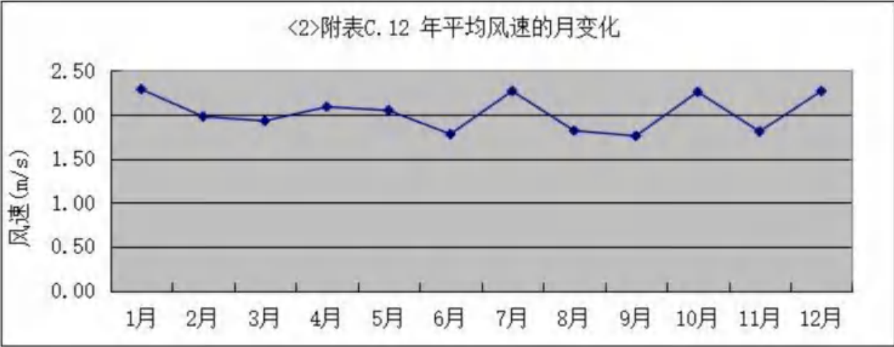
图 5.3-5 鹤山市 2023 年平均风速的月变化图
