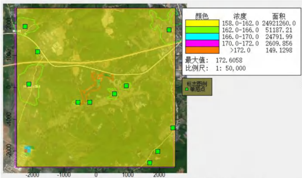
图 5.3-15 TSP 正常工况下 95%保证率日均浓度等值线图 (单位: \mu\text{g}/\text{m}^3 )
