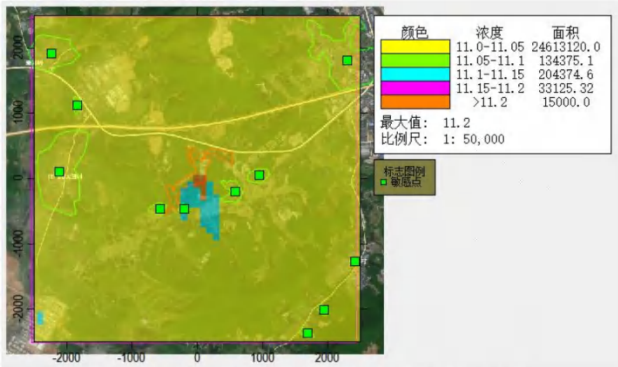
图 5.3-9 SO 2 正常工况下 98% 保证率日均浓度等值线图 (单位: \mu\text{g}/\text{m}^3 )
