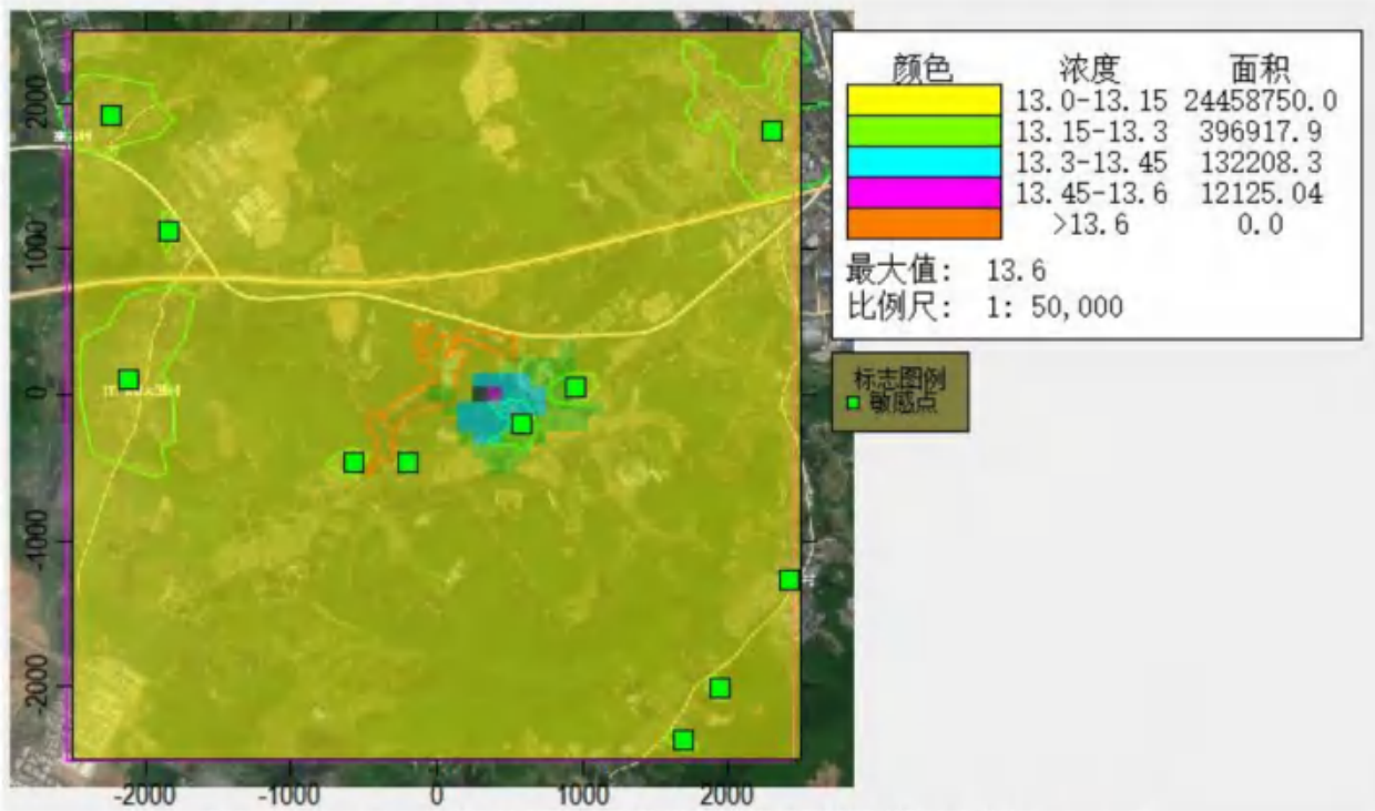
图 5.3-10 SO 2 正常工况下年平均浓度叠加值等值线图 (单位: \mu\text{g}/\text{m}^3 )
