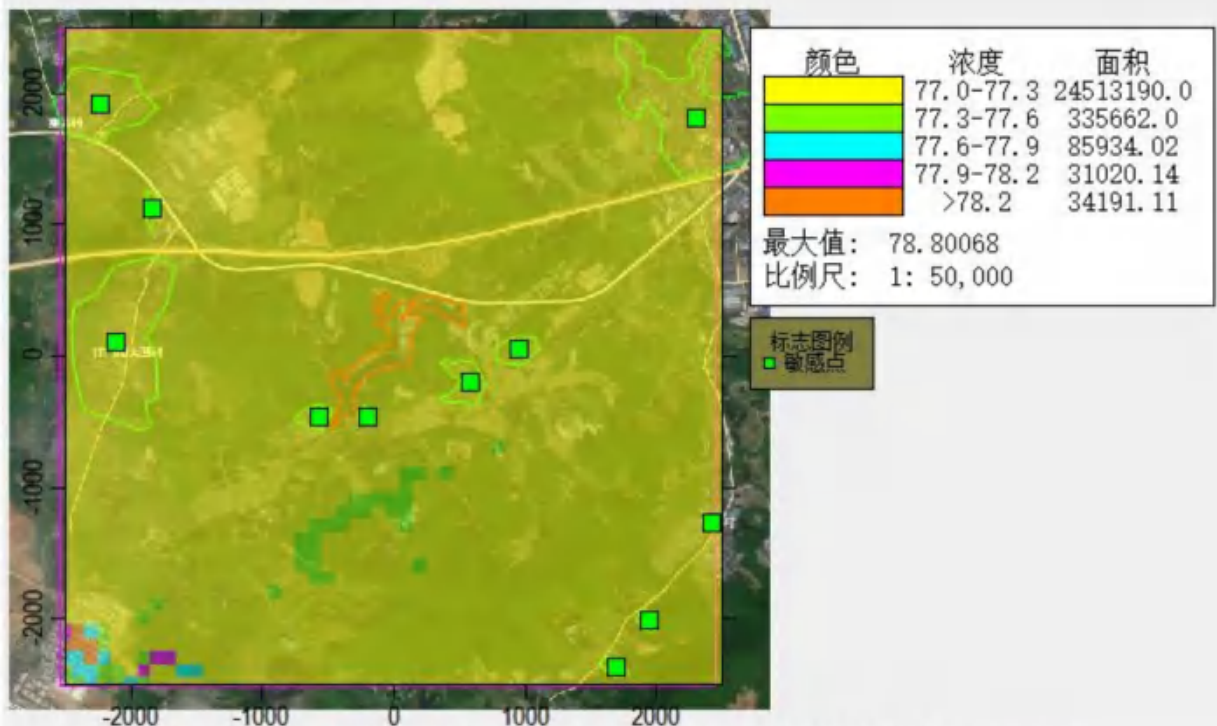
图 5.3-13 PM 10 正常工况下 95%保证率日均浓度等值线图 (单位: \mu\text{g}/\text{m}^3 )
