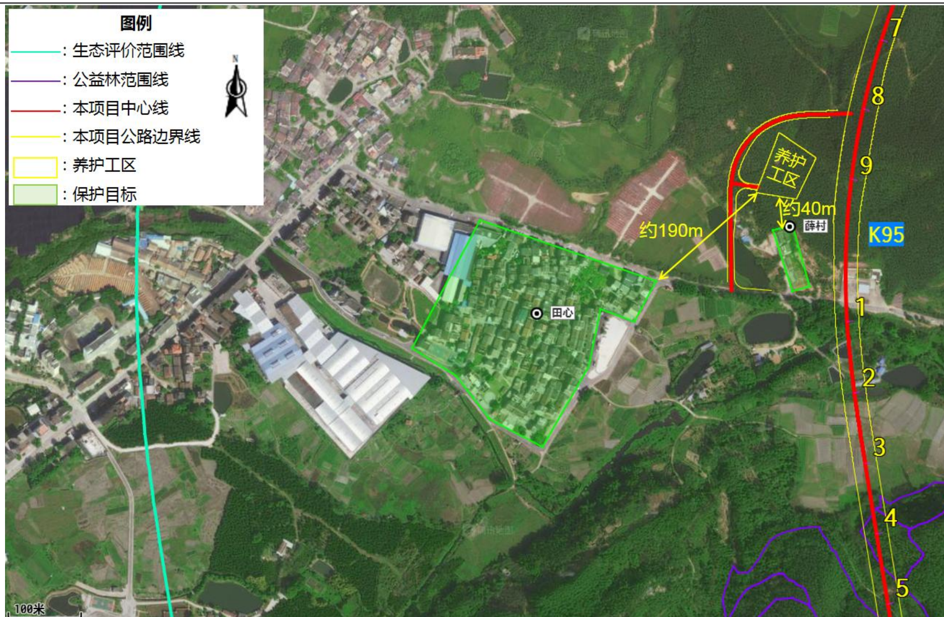
图 1.7-5 大临工程和附属设施分布图 (k)
