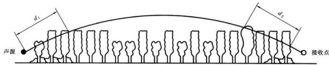
图 4.4-3 通过树和灌木时噪声衰减示意图
