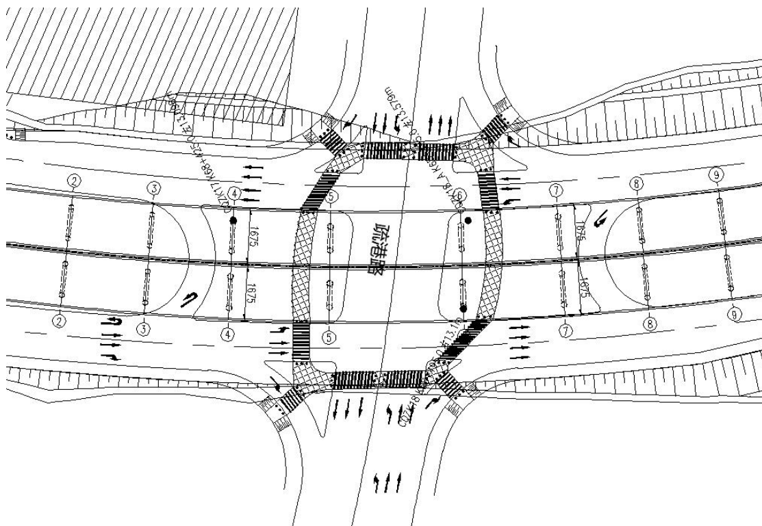
图 2.2-9 疏港大道跨线桥平面
