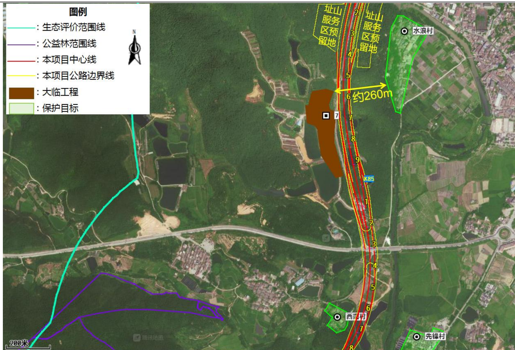
图 1.7-5 大临工程和附属设施分布图 (h)
