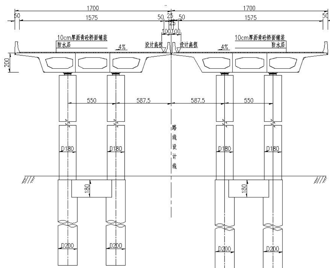
图 2.2-8 疏港大道现浇箱梁断面
