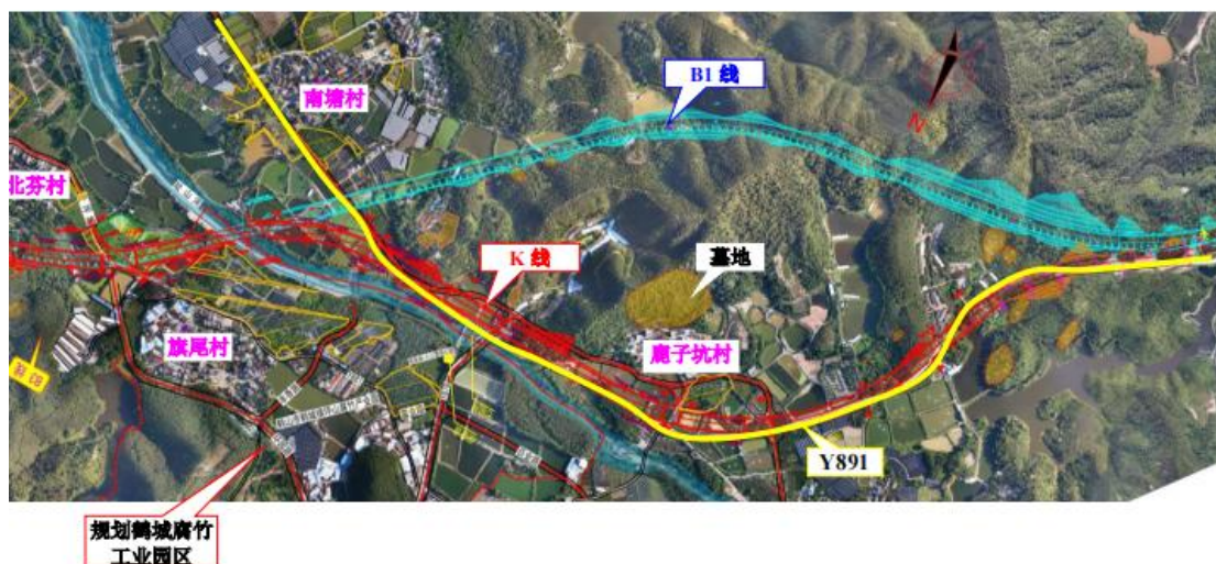
图 2.1-14 K 线与 B1 线卫星平面图
