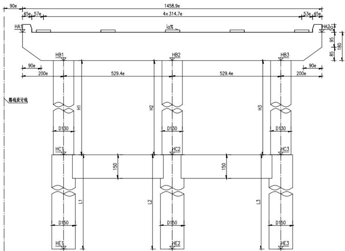
图 2.2-15 城西大桥桥墩一般构造图
