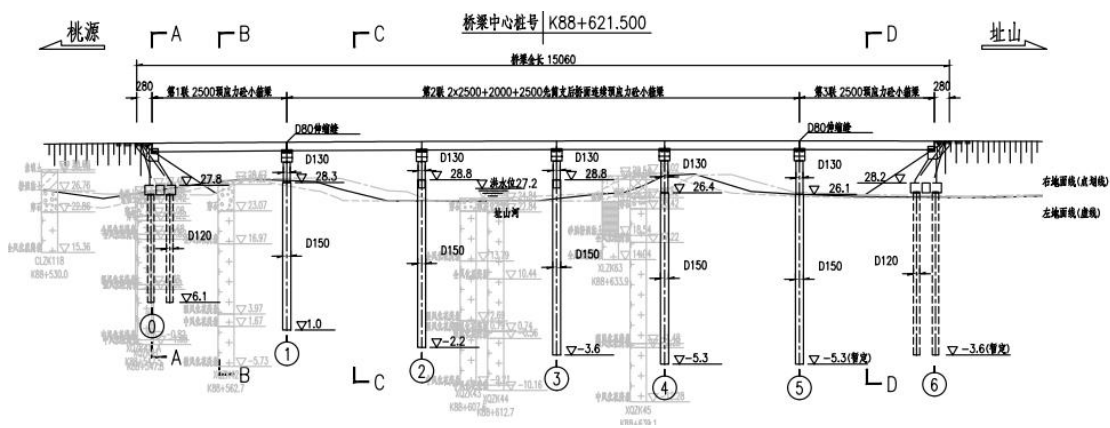
图 2.2-19 址山河大桥桥型立面图
