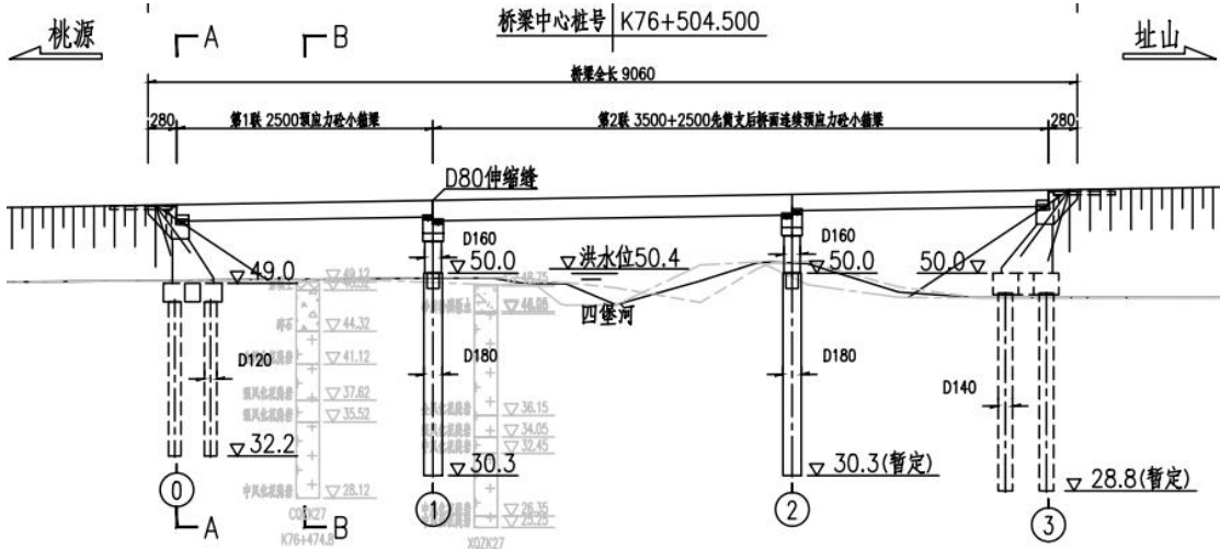
图 2.2-13 横岗 3#桥桥型立面
