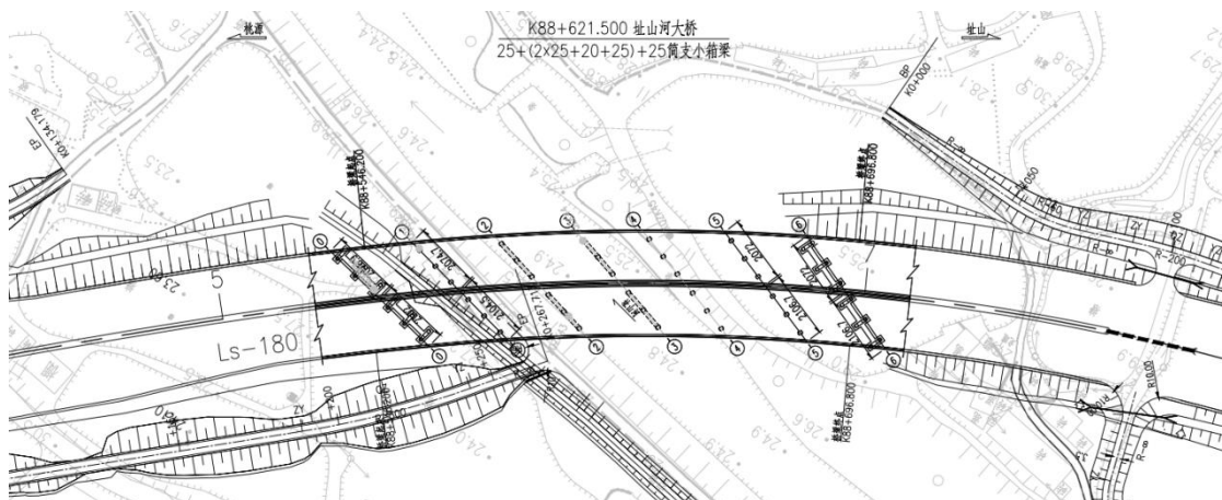
图 2.2-18 址山河大桥桥位平面图
