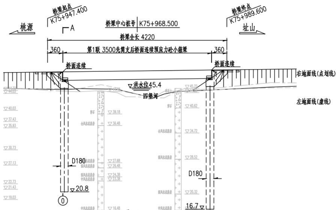
图 2.2-11 横岗 1#桥桥型立面
