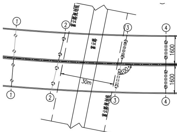
图 2.2-22 富云路跨越平面布置图
