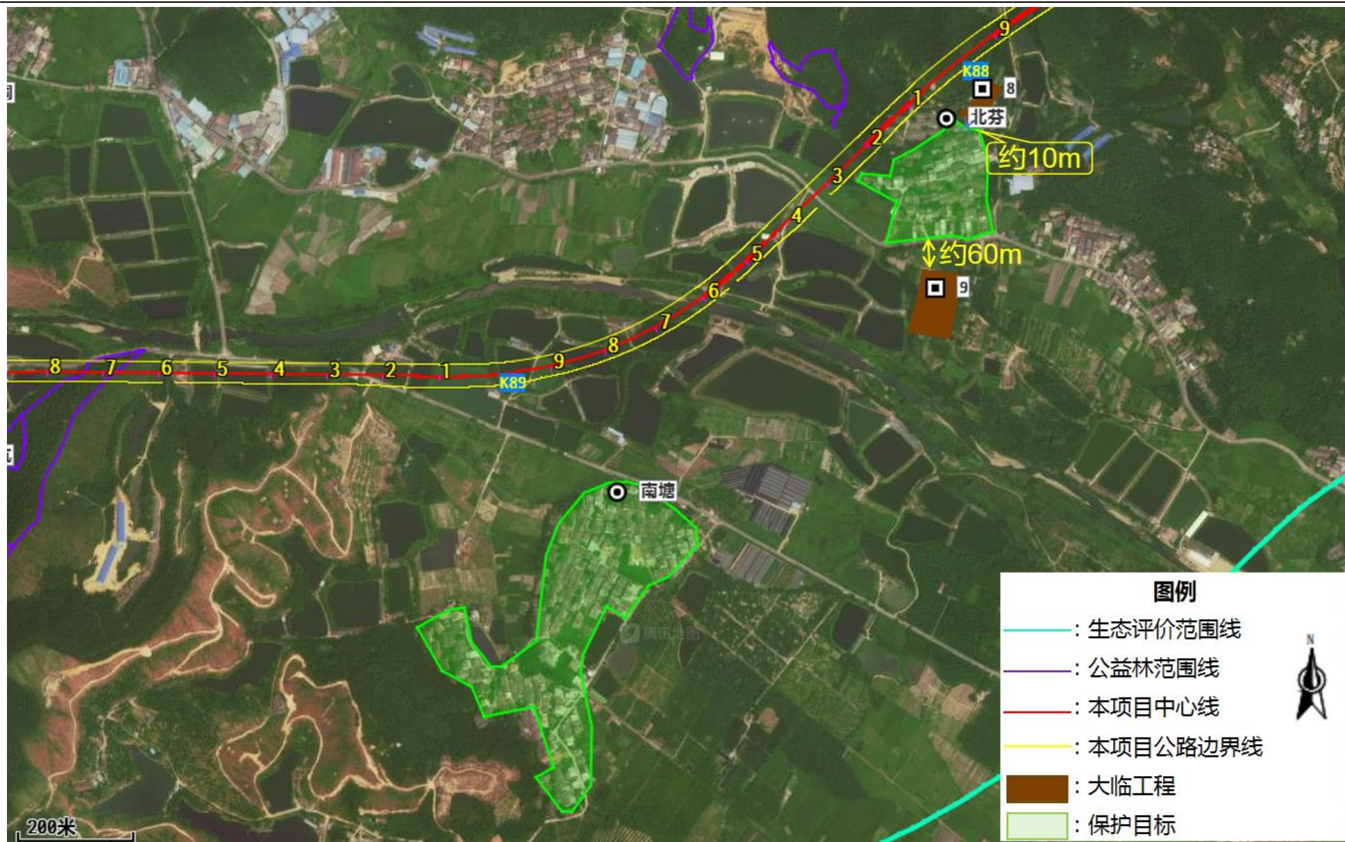
图 1.7-5 大临工程和附属设施分布图 (i)
