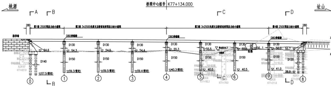
图 2.2-14 横水新村桥桥型立面
