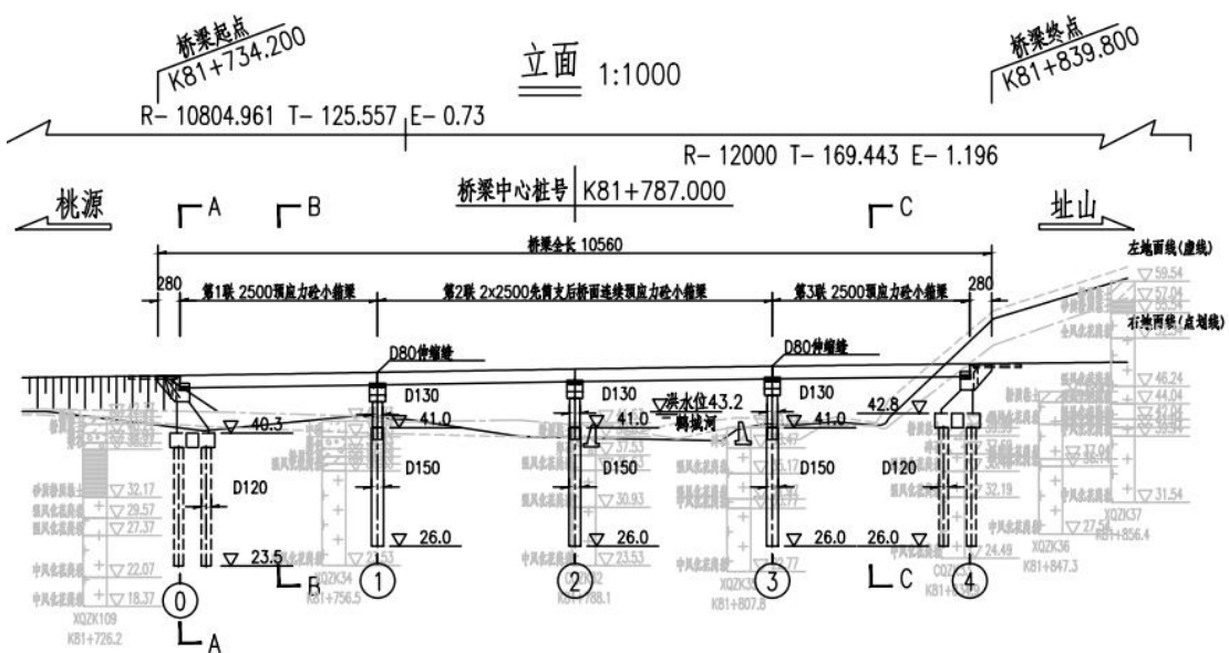
图 2.2-16 城西大桥桥型布置图
