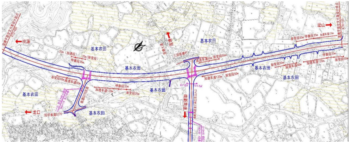
图 2.2-28 莲塘互通立交平面图
