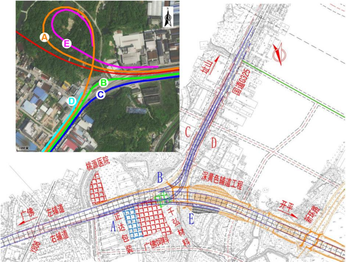
图 2.2-26 桃源西互通立交平面图
