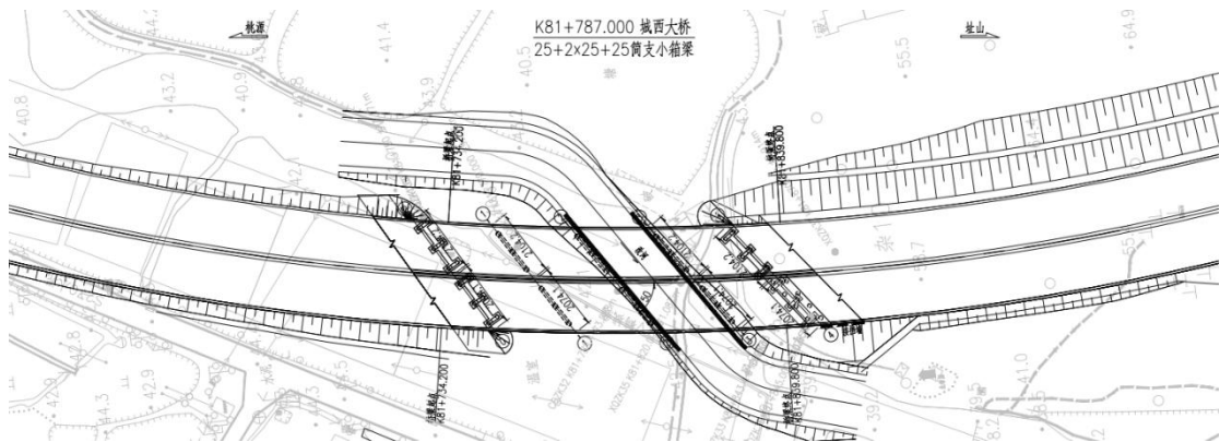
图 2.2-17 城西大桥桥位平面图
