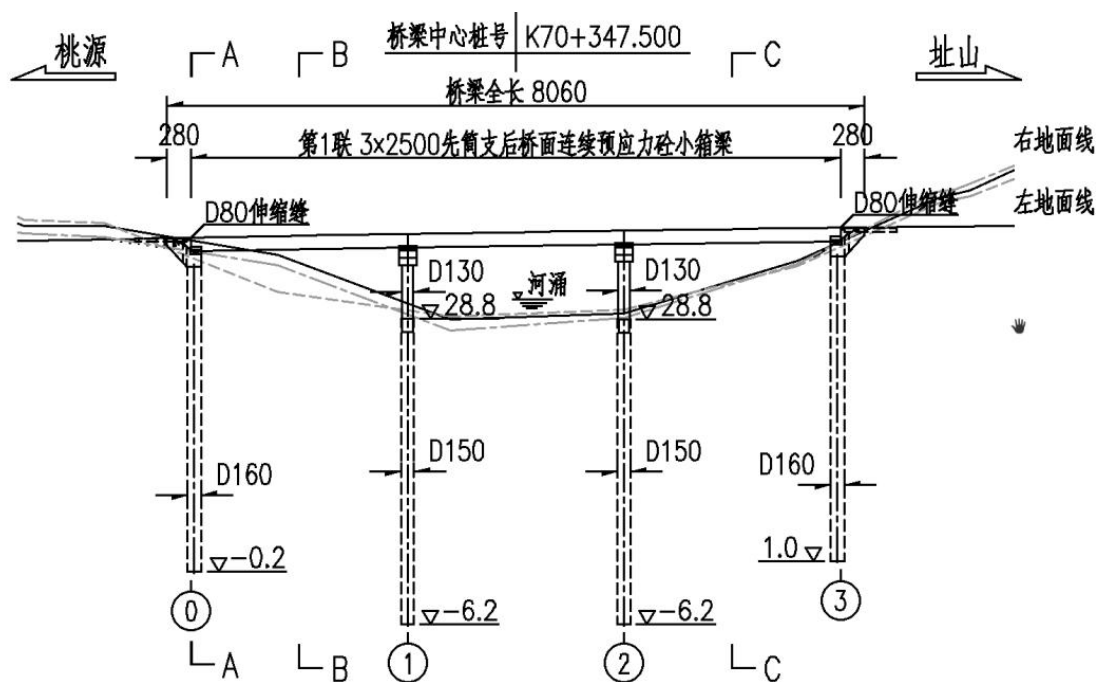
图 2.2-10 那白中桥桥型立面
