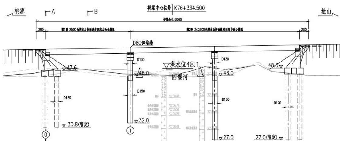
图 2.2-12 横岗 2#桥桥型立面
