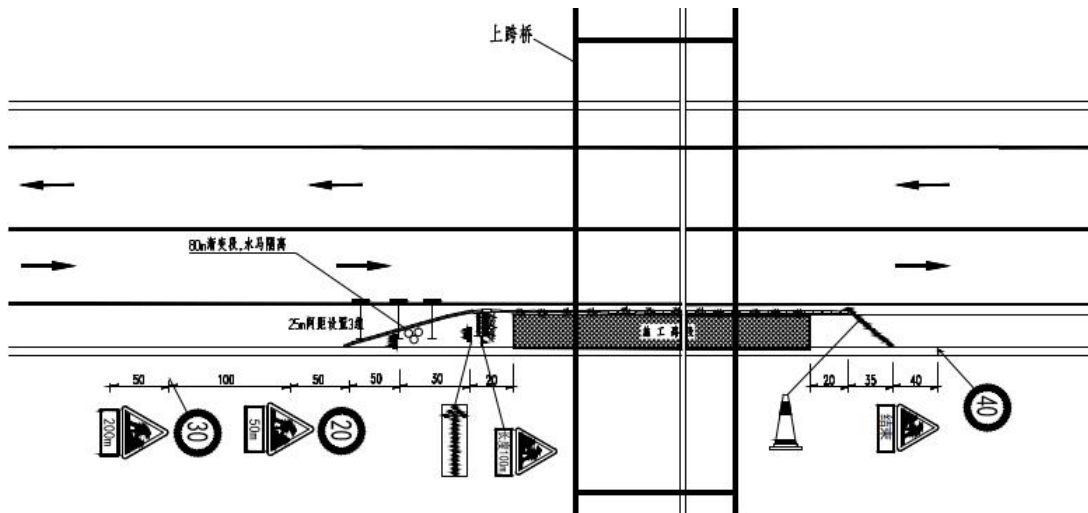
图 2.4-1 临时设施布置图
