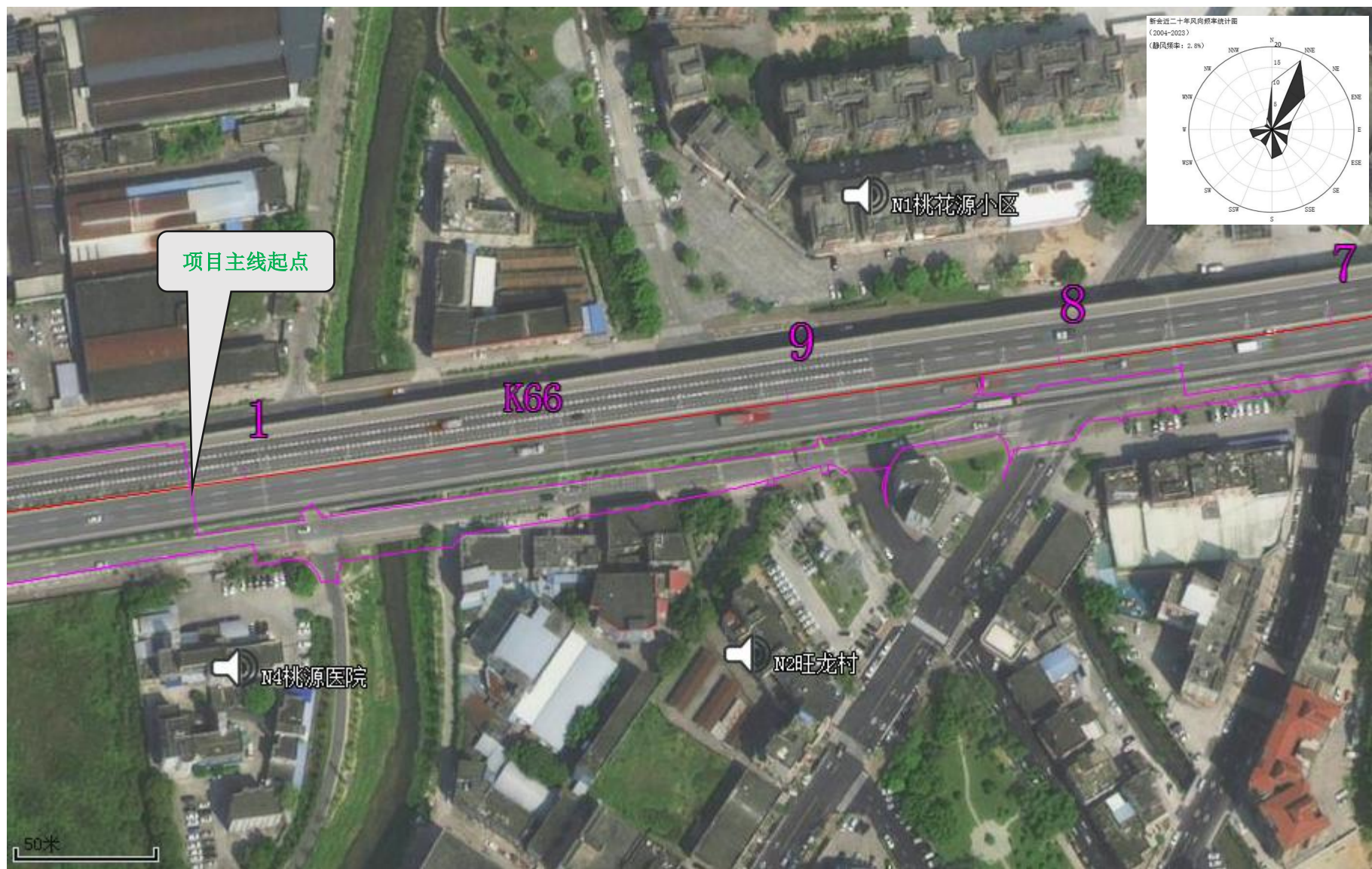
图 3.2-1 (1) 本项目的噪声监测点位布置图
