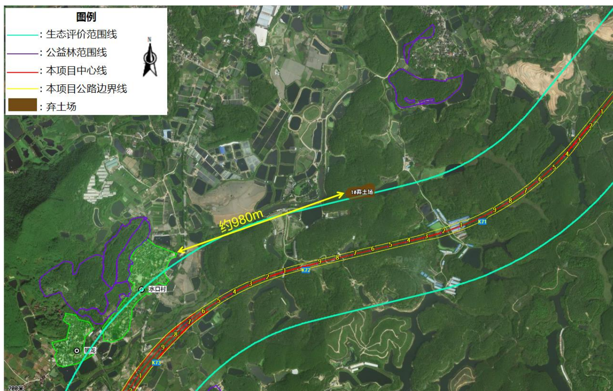
图 2.2-30 施工期弃土场分布图（1）
