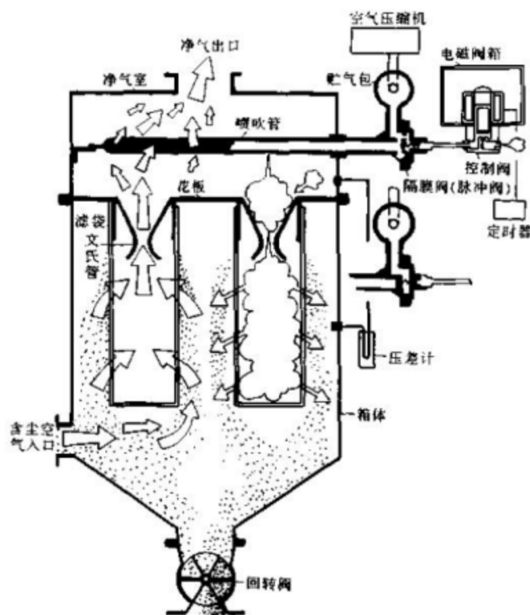
图 6.6-2 袋式除尘器工作原理图
