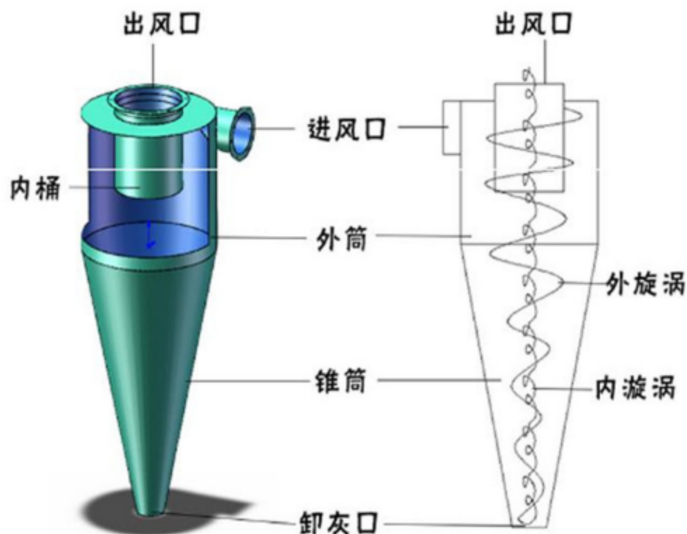
图 6.6-1 旋风除尘器工作原理图
