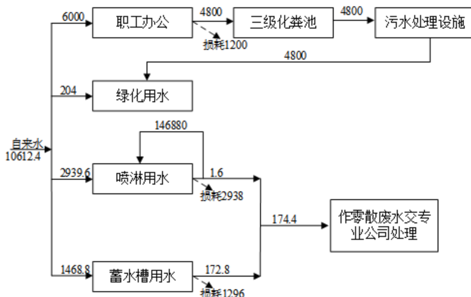
图 2.6-1 项目水平衡图 (单位: t/a)
