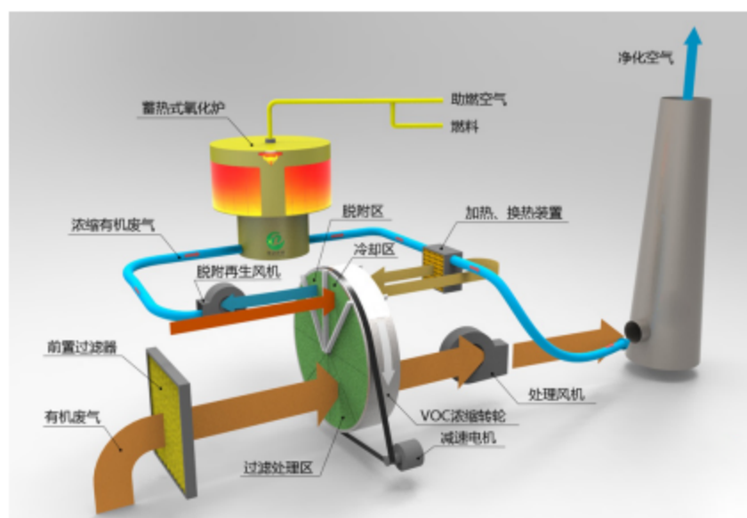
图 6.6-3 废气处理工艺示意图
