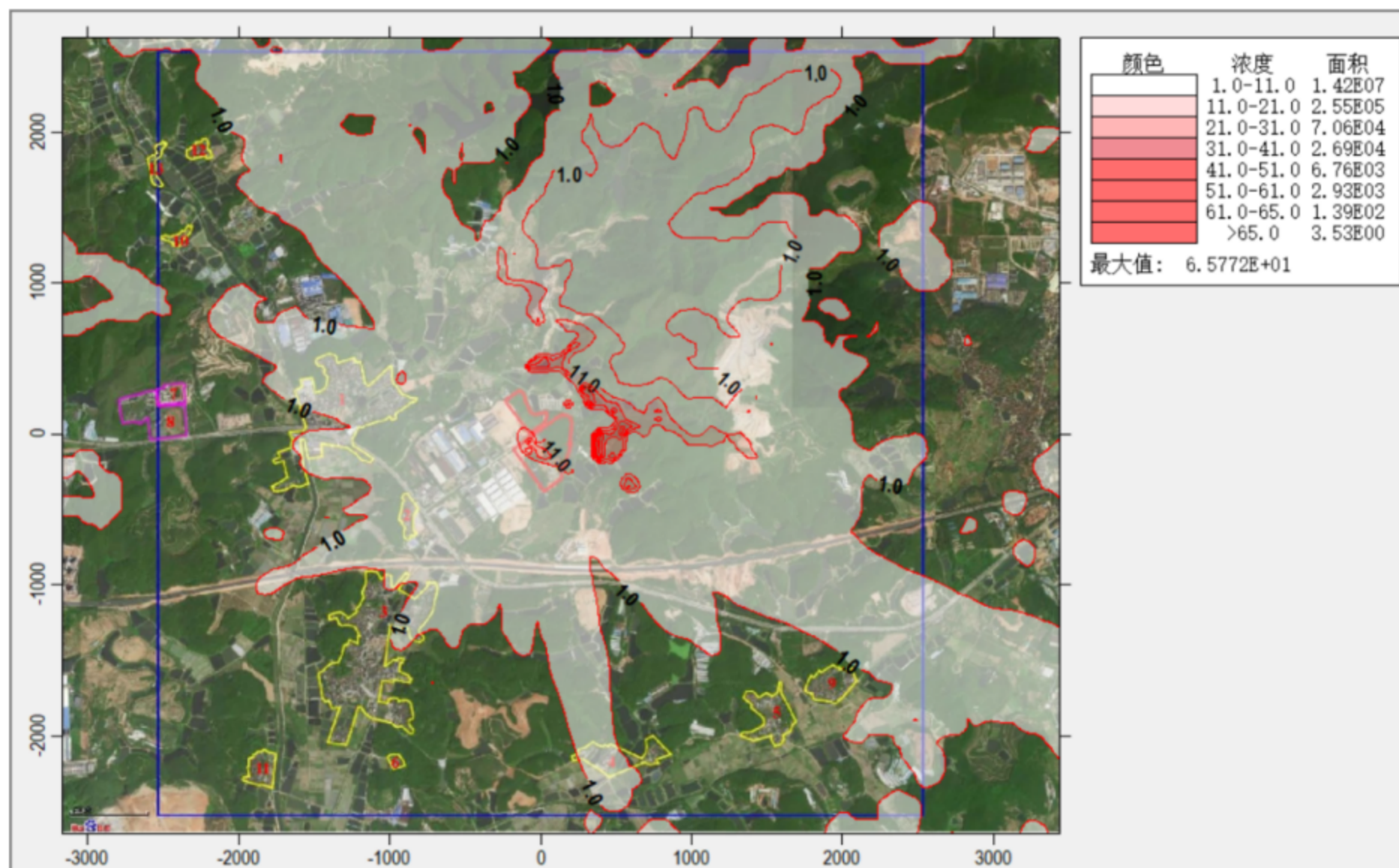
图 5.2-10 (a) 正常排放 PM_{10} 贡献值预测结果情况 (1h 均值) 图 单位: \mu g/m^3
