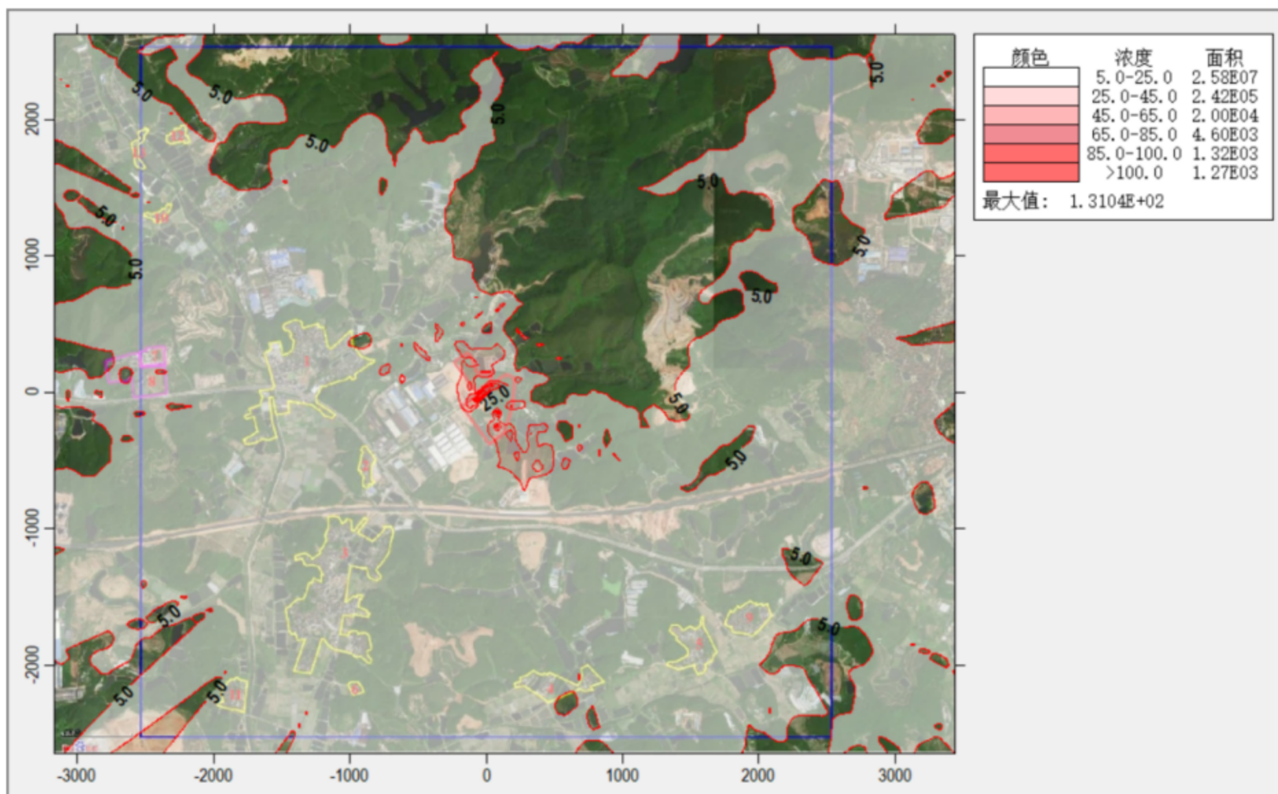
图 5.2-17 正常排放二甲苯叠加值预测结果情况 (1h 均值) 图 单位: \mu\text{g}/\text{m}^3
