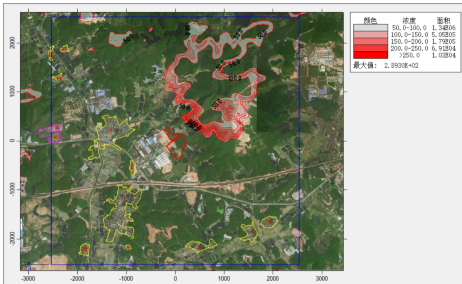
图 5.2-19 非正常排放，非甲烷总烃贡献值预测结果情况 (1h 均值) 图 单位: \mu\text{g}/\text{m}^3
