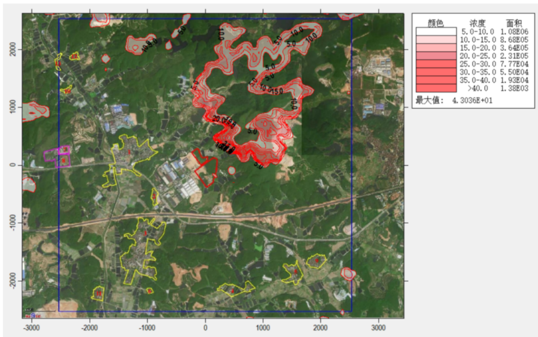
图 5.2-20 非正常排放，二甲苯贡献值预测结果情况 (1h 均值) 图 单位: \mu\text{g}/\text{m}^3
