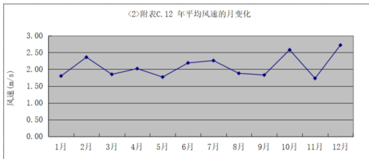
图 5.2-5 鹤山气象站 2022 年平均风速的月变化图
