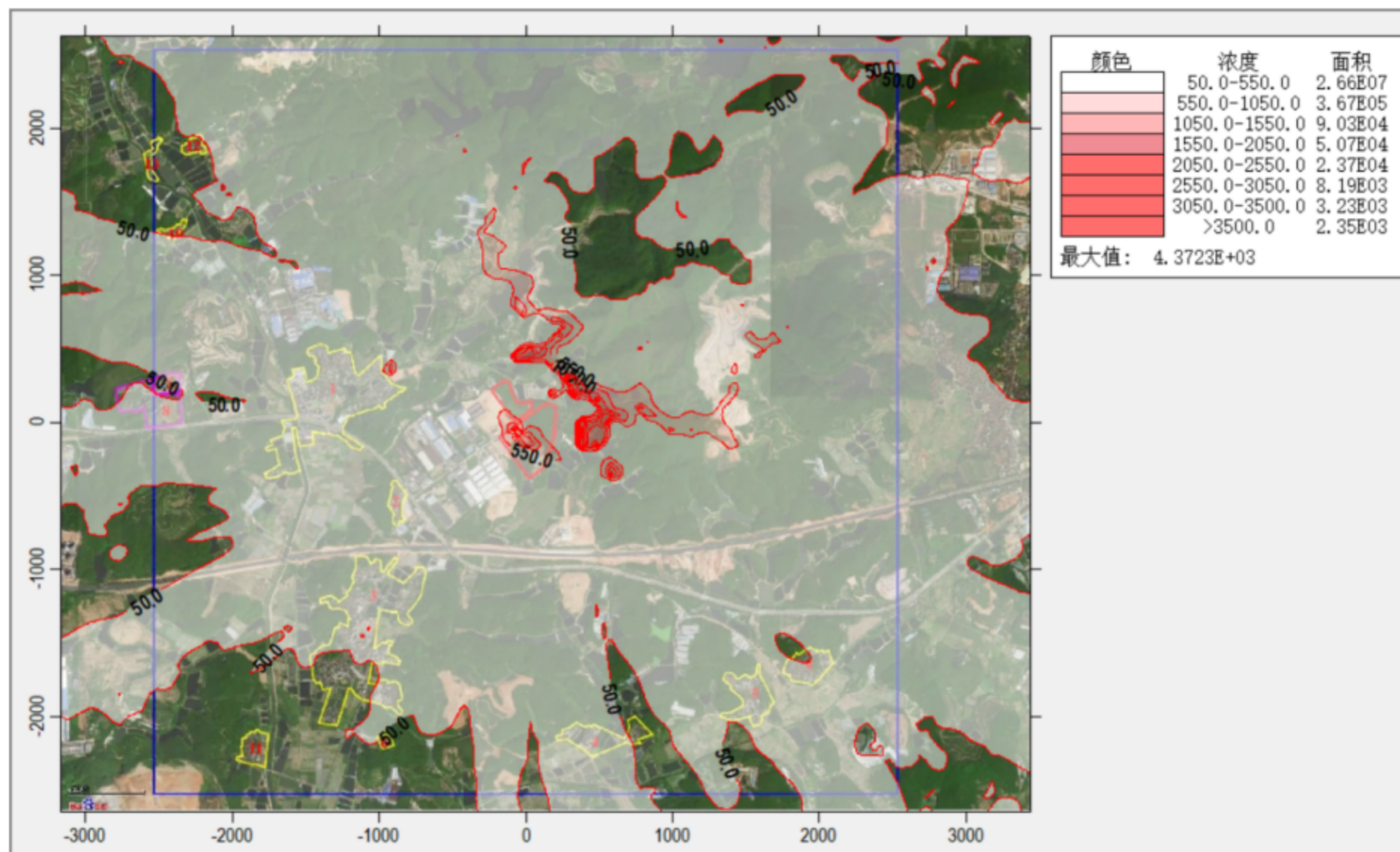
图 5.2-18 非正常排放，PM 10 贡献值预测结果情况（1h 均值）图 单位：μg/m 3
