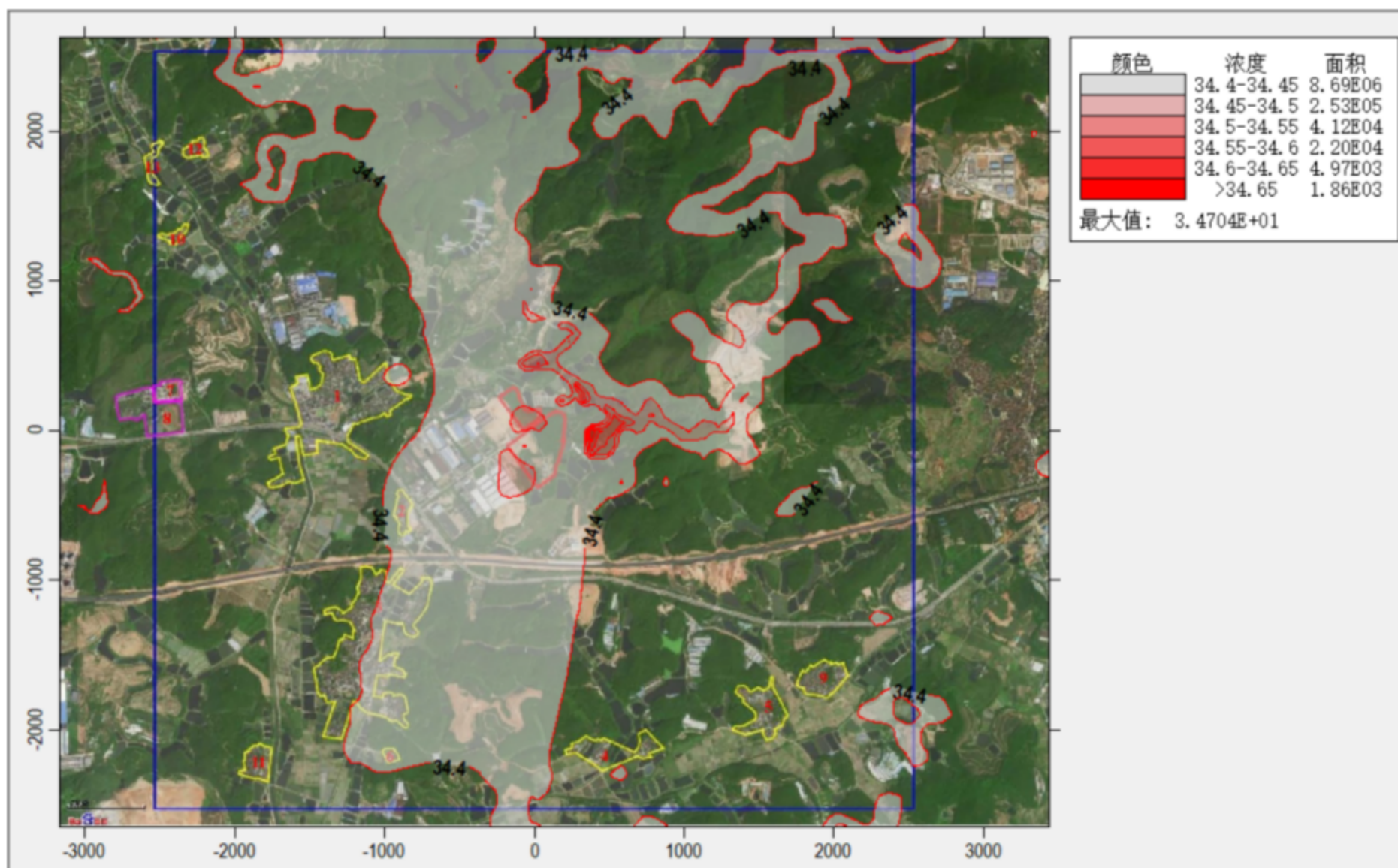
图 5.2-14 (b) 正常排放 PM_{10} 叠加值预测结果情况 (年均值) 图 单位: \mu g/m^3
