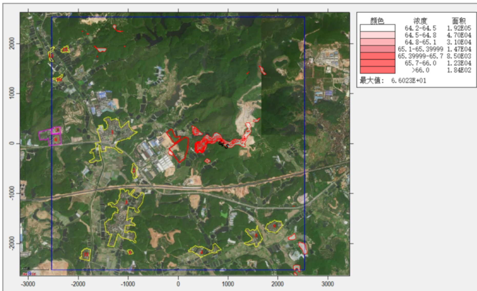
图 5.2-14 (a) 正常排放 PM_{10} 叠加值预测结果情况 (24h 均值) 图 单位: \mu g/m^3
