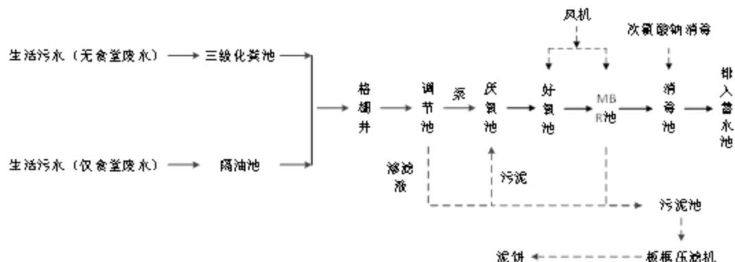
图 6.5-1 废水处理工艺流程图
