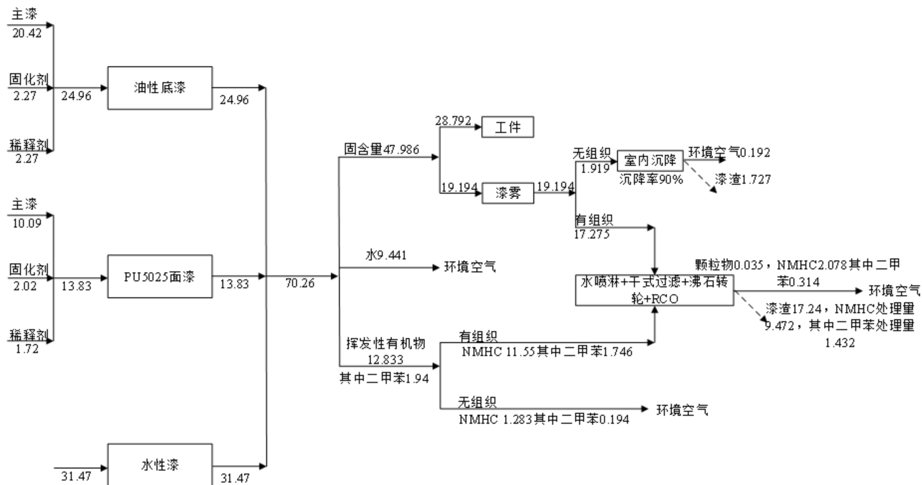
图 2.6-2 全厂漆料平衡图 (单位: t/a)
