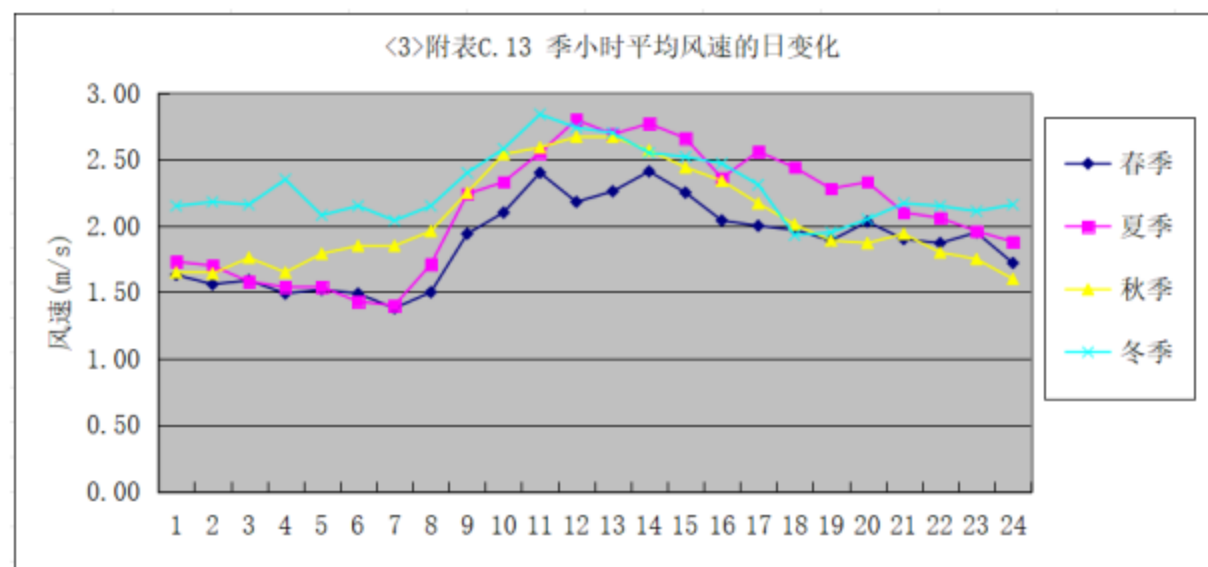
图 5.2-6 鹤山气象站 2022 年各季小时平均风速的日变化图
