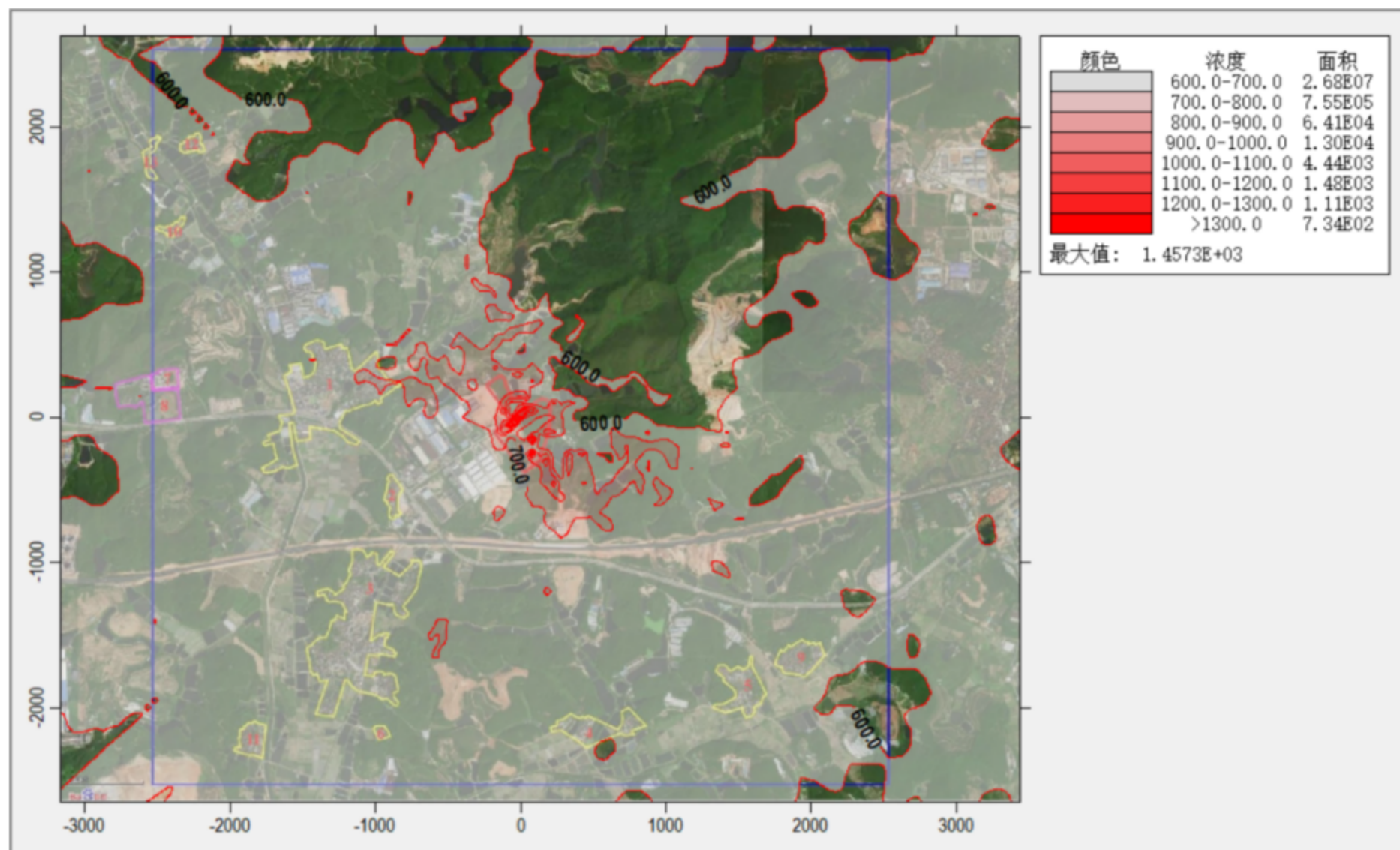
图 5.2-16 正常排放非甲烷总烃叠加预测结果情况 (1h 均值) 图 单位: \mu\text{g}/\text{m}^3
