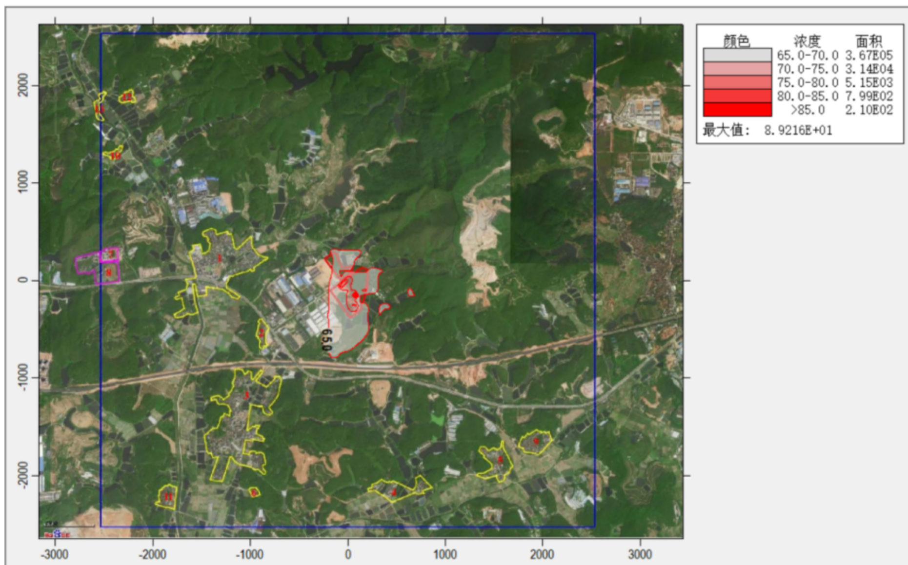
图 5.2-15 (b) 正常排放 TSP 叠加值预测结果情况 (年均值) 图 单位: \mu\text{g}/\text{m}^3
