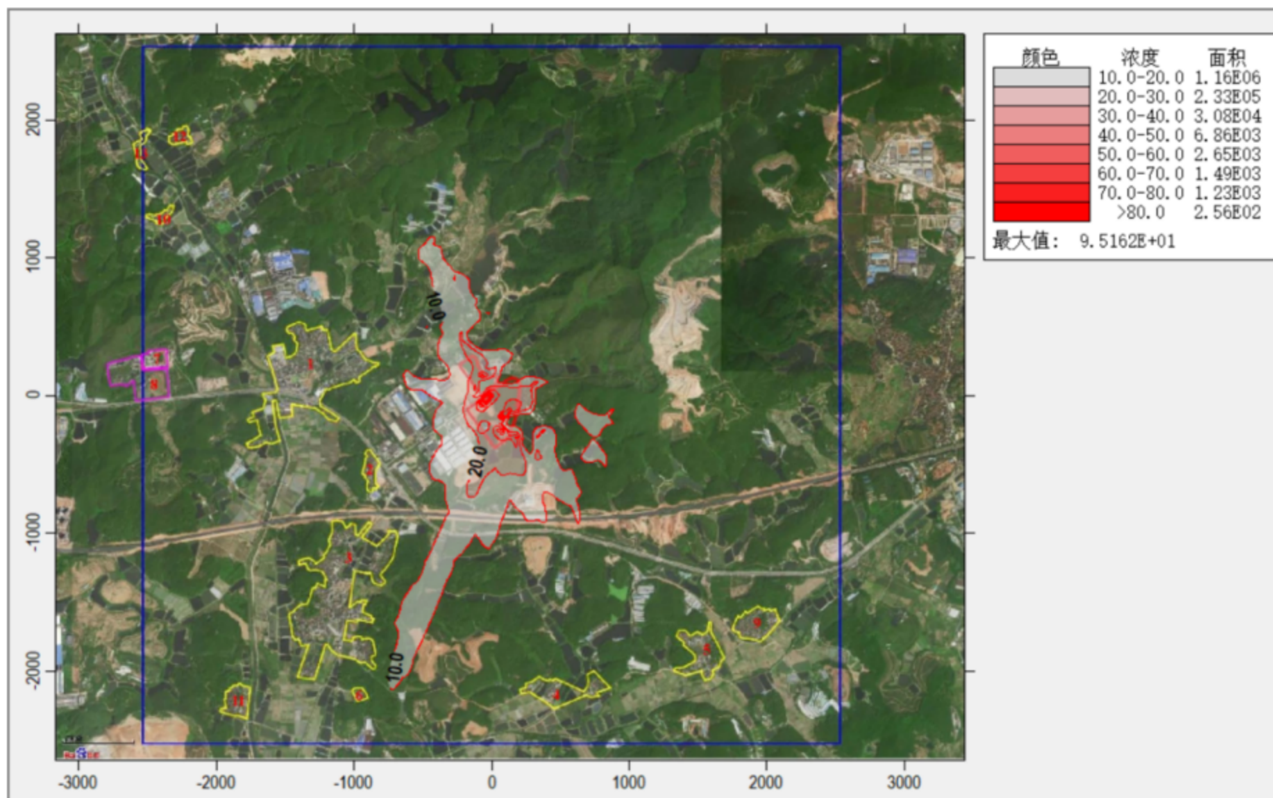
图 5.2-11 (b) 正常排放 TSP 贡献值预测结果情况 (24h 均值) 图 单位: \mu\text{g}/\text{m}^3
