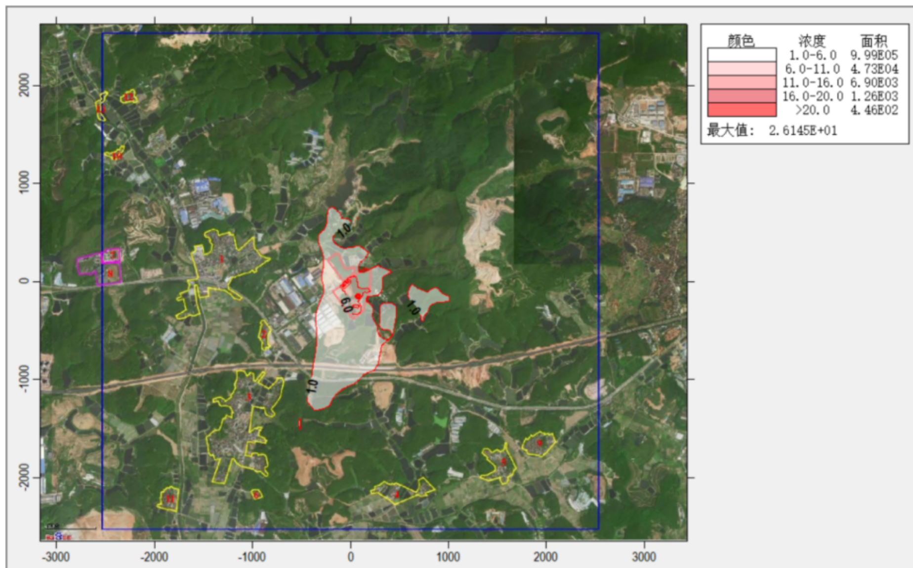
图 5.2-11 (c) 正常排放 TSP 贡献值预测结果情况 (年均值) 图 单位: \mu\text{g}/\text{m}^3
