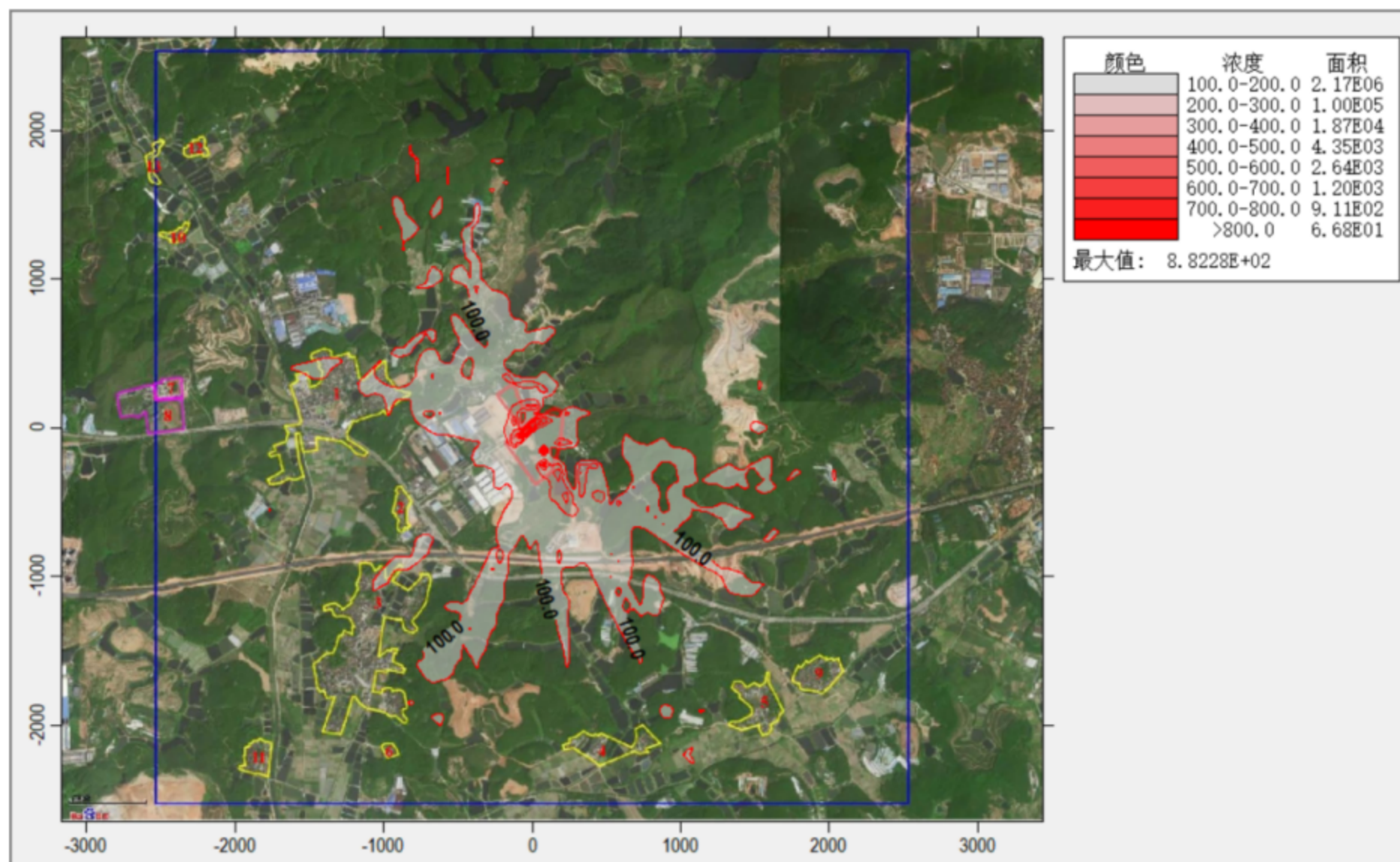
图 5.2-12 正常排放非甲烷总烃贡献值预测结果情况 (1h 均值) 图 单位: \mu\text{g}/\text{m}^3
