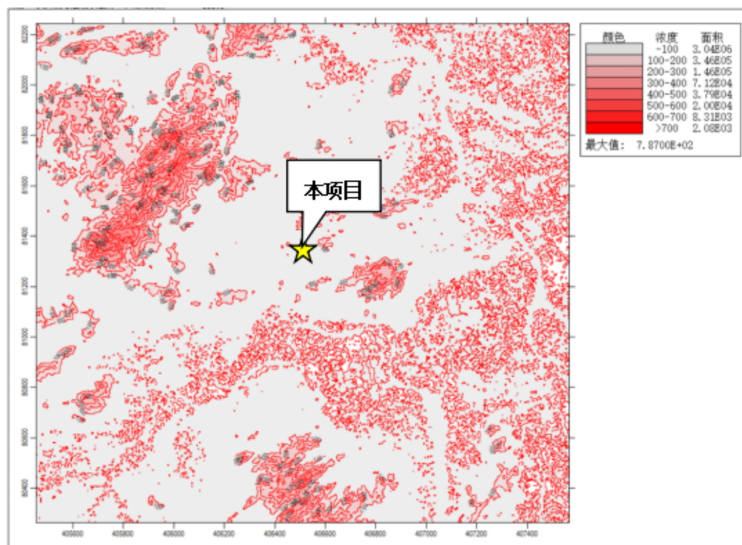
图 5.2-9 项目所在区域地形等高线示意图
