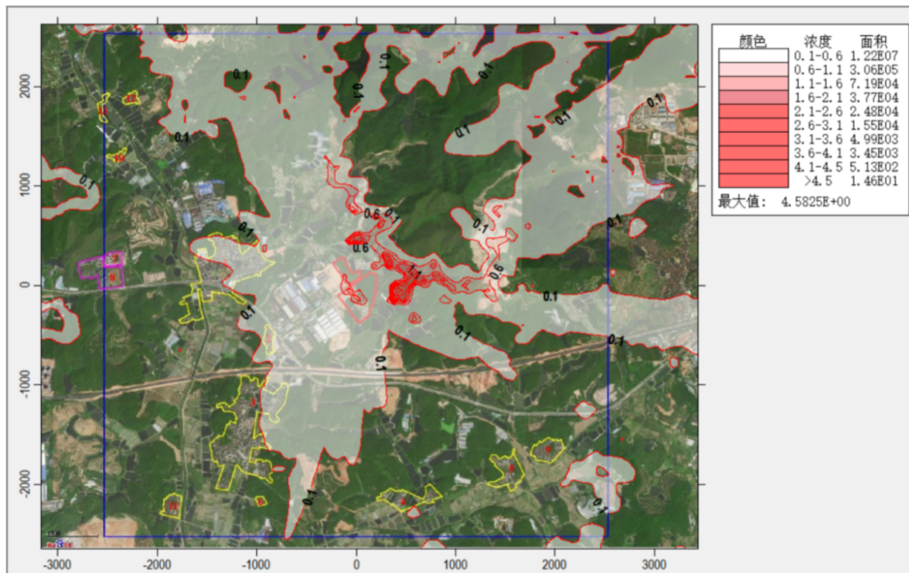
图 5.2-10 (b) 正常排放 PM_{10} 贡献值预测结果情况 (24h 均值) 图 单位: \mu g/m^3
