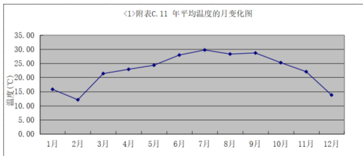
图 5.2-4 鹤山气象站 2022 年平均温度的月变化图
