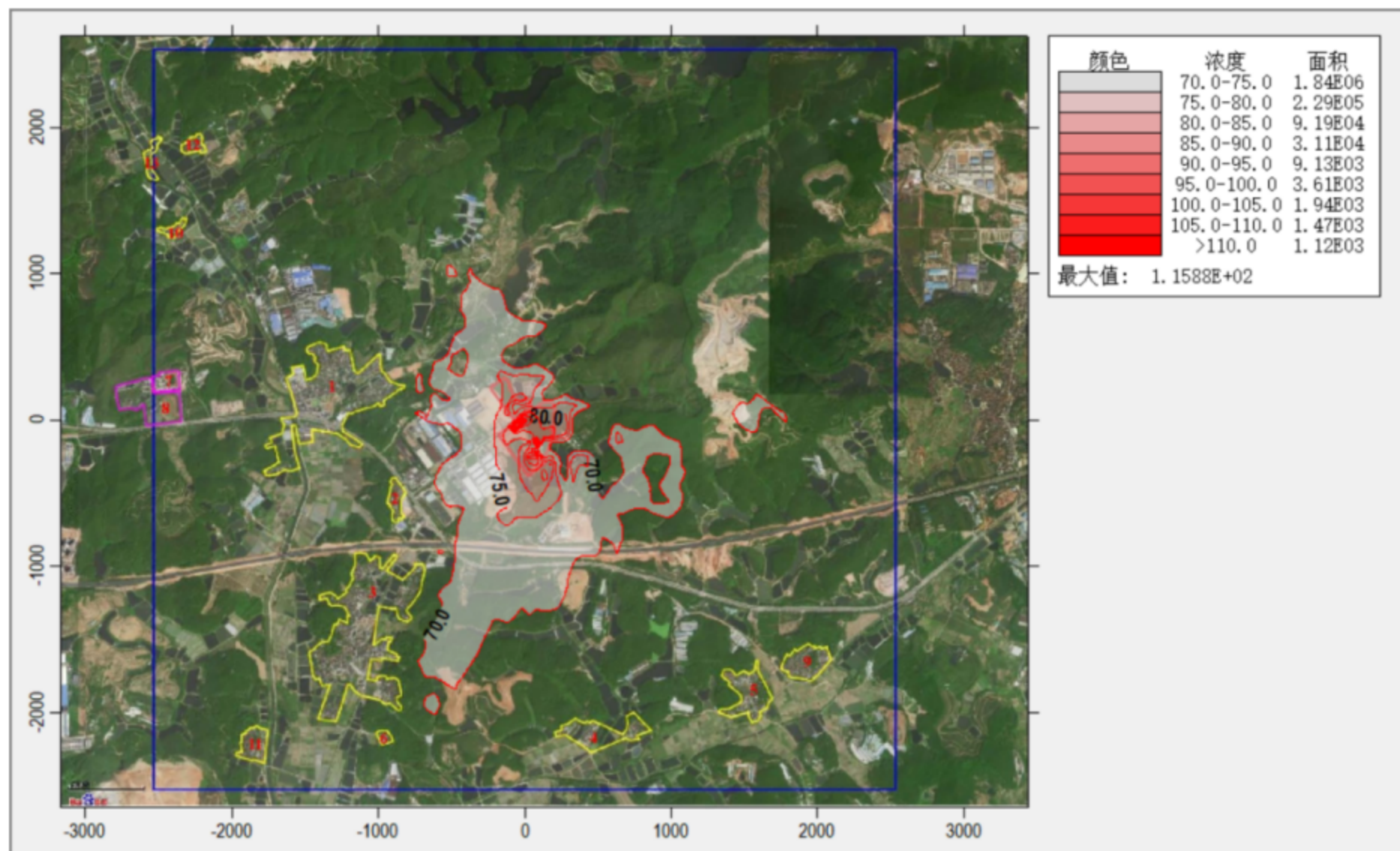
图 5.2-15 (a) 正常排放 TSP 叠加值预测结果情况 (24h 均值) 图 单位: \mu\text{g}/\text{m}^3
