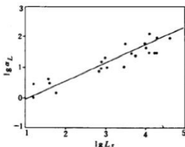
图 5.3-2 孔隙介质数值模型的 \lg \alpha_L - \lg L_s 图
