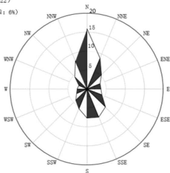
图 5.2-3 鹤山气象站近 20 年风向玫瑰图（统计年限：2003~2022 年）
