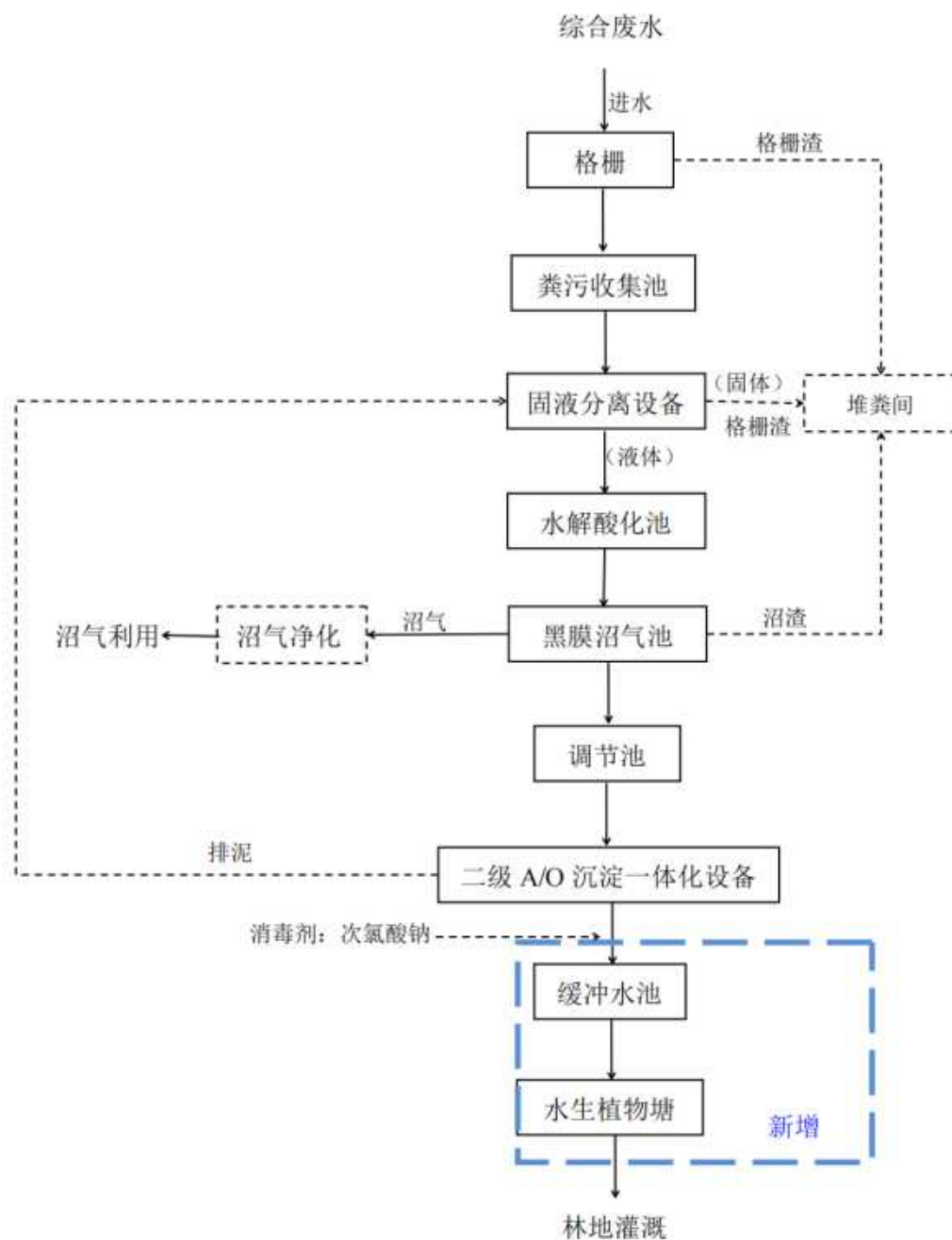
图 7.2-1. 改扩建后项目废水处理流程图
