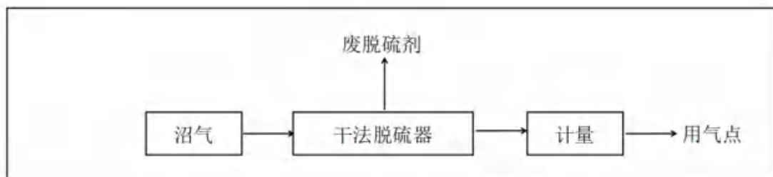
图 4.2-4. 项目沼气净化示意图
