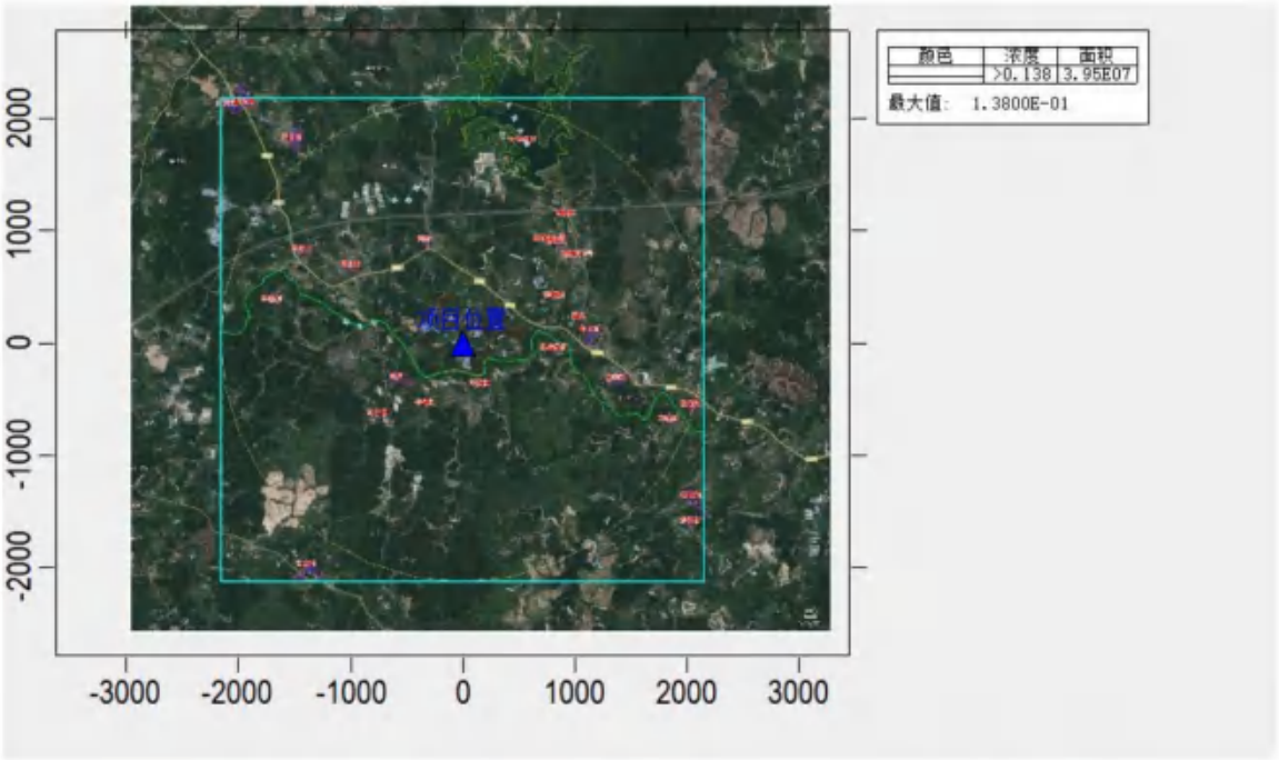
图 6.2-34. PM_{10} 叠加后 95%保证率日平均浓度分布图 (单位 mg/m^3 )
