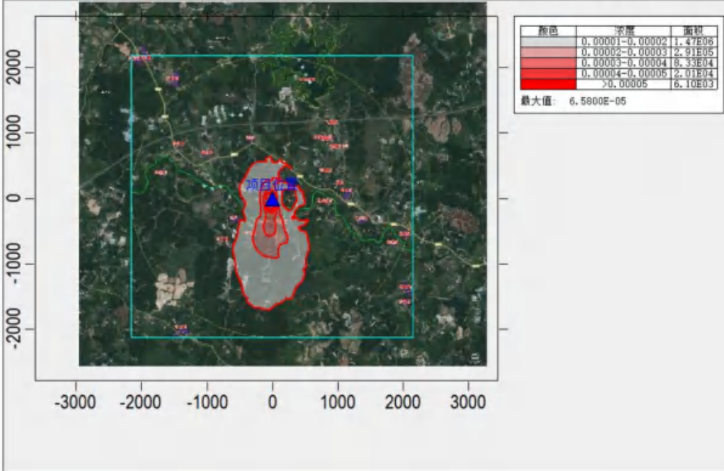
图 6.2-24. SO 2 贡献值年平均浓度分布图 (单位 mg/m 3 )
