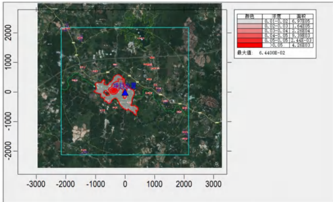
图 6.2-36. 氨贡献值 1 小时平均浓度分布图 (单位 mg/m³)
