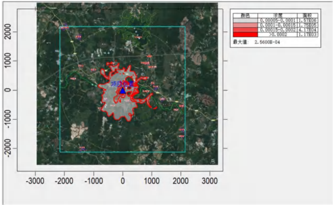
图 6.2-32. PM 10 贡献值日平均浓度分布图 (单位 mg/m 3 )
