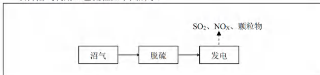
图 4.2-3. 项目沼气利用发电工艺图
