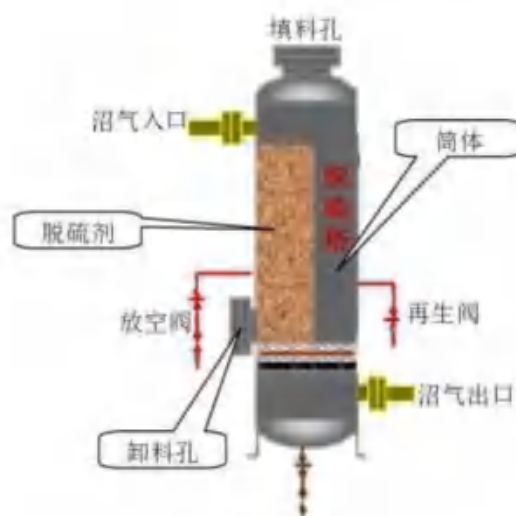
图 7.2-6. 脱硫塔结构图
