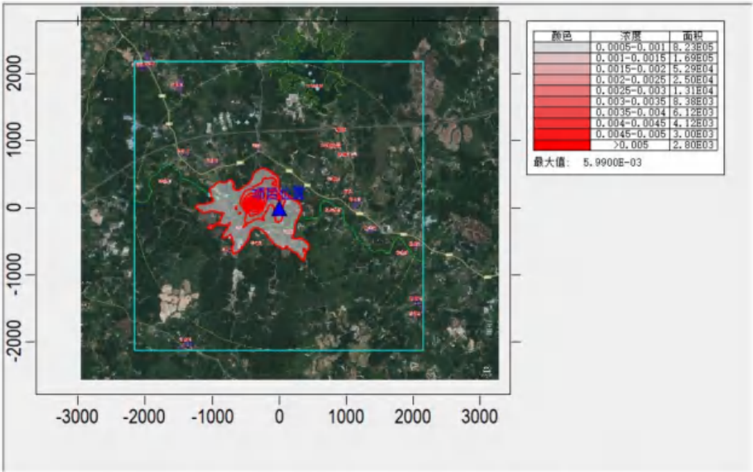
图 6.2-38. 硫化氢贡献值 1 小时平均浓度分布图（单位 \text{mg}/\text{m}^3 ）
