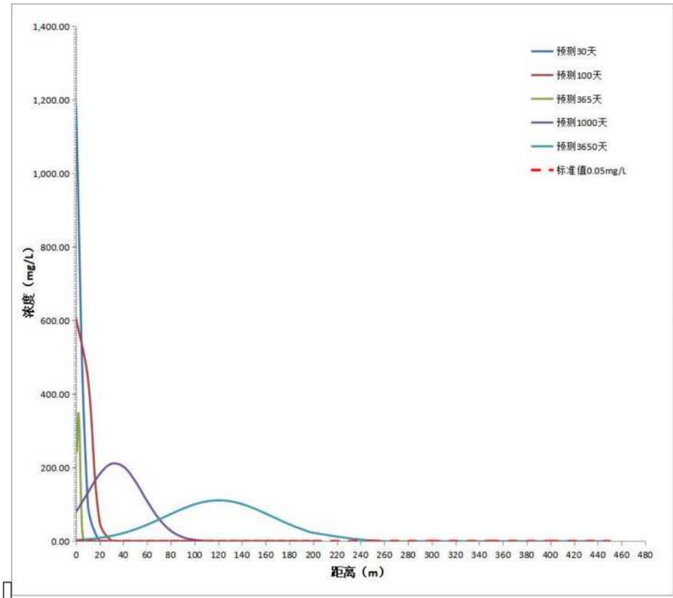
①下游 CODMn 瞬时注入随距离变化分布图
