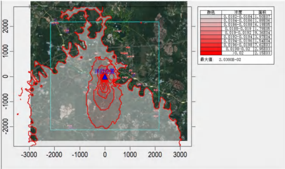
图 6.2-31. NO 2 叠加后年平均浓度分布图 (单位 mg/m 3 )
