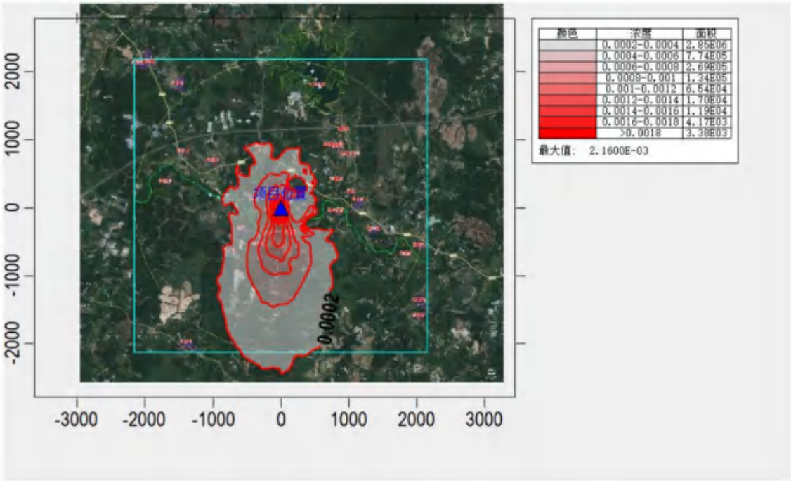
图 6.2-29. NO 2 贡献值年平均浓度分布图 (单位 mg/m 3 )
