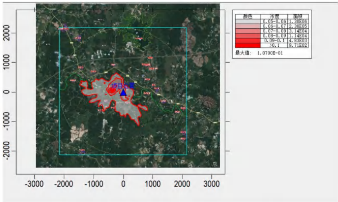
图 6.2-37. 氨叠加后 1 小时平均浓度分布图 (单位 mg/m³)
