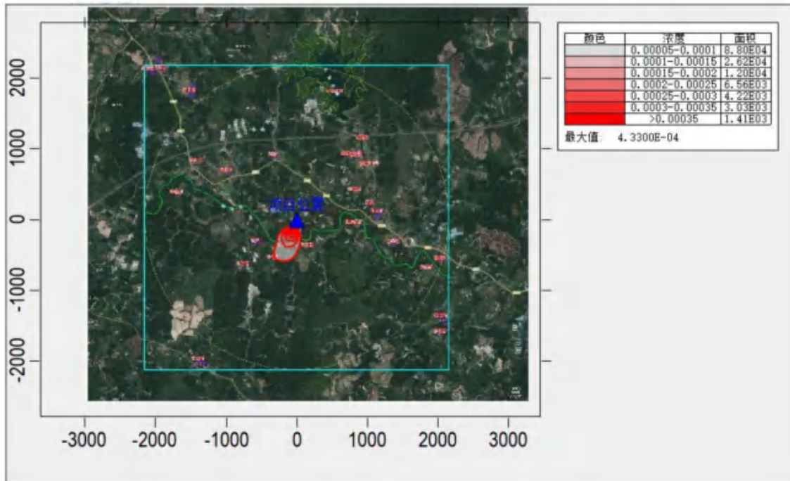
图 6.2-22. SO 2 贡献值 1 小时平均浓度分布图 (单位 mg/m 3 )
