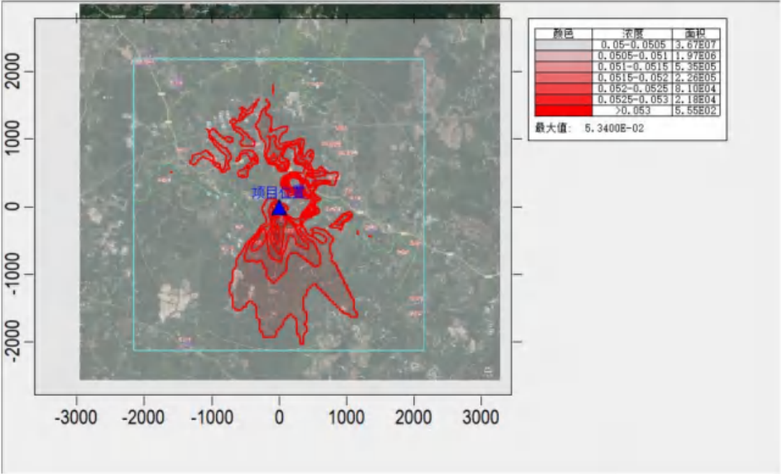
图 6.2-30. NO 2 叠加后 98%保证率日平均浓度分布图 (单位 mg/m 3 )
