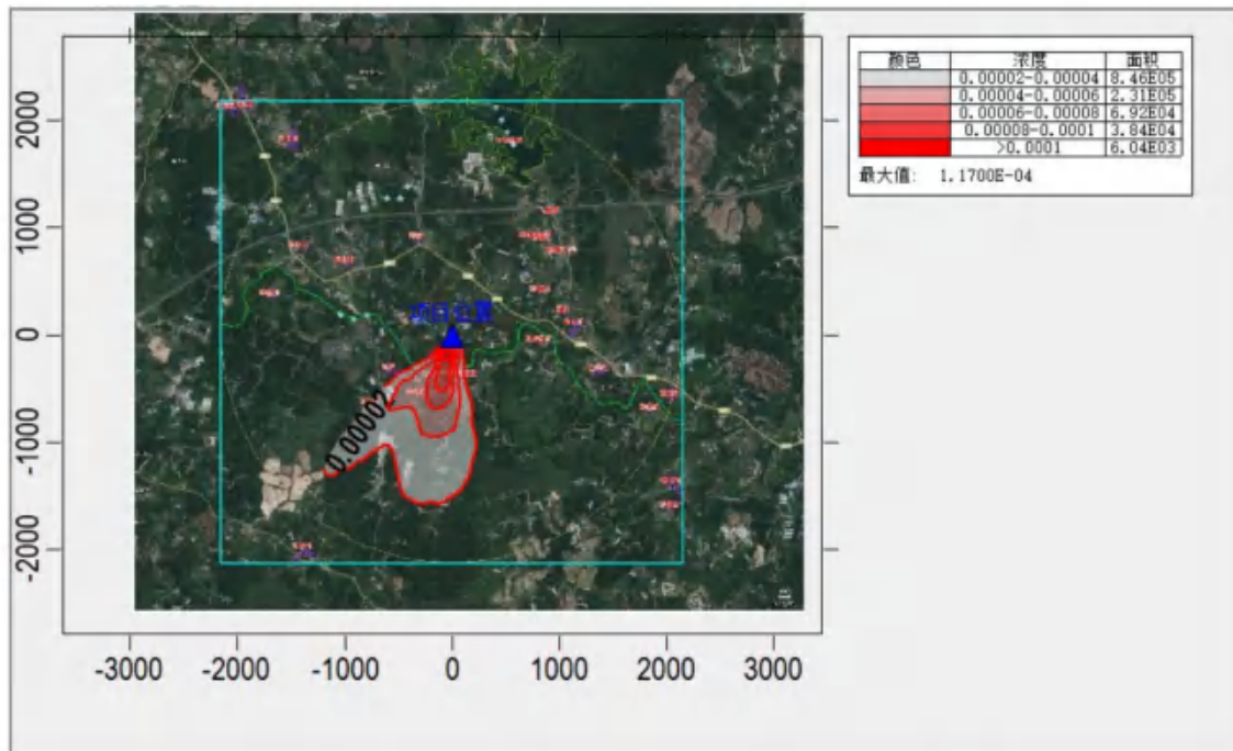
图 6.2-23. SO 2 贡献值日平均浓度分布图 (单位 mg/m 3 )
