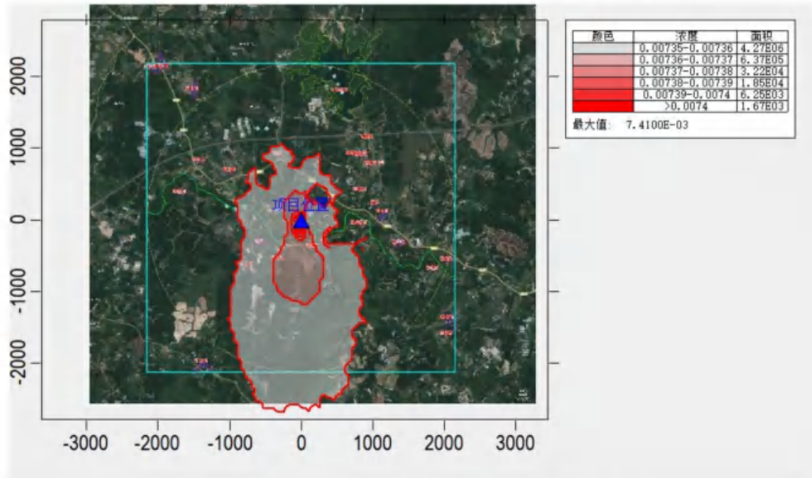
图 6.2-26. SO 2 叠加后年平均浓度分布图 (单位 mg/m 3 )
