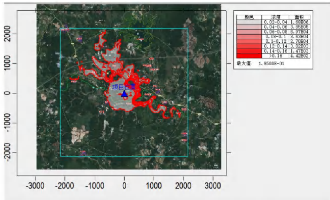
图 6.2-27. NO 2 贡献值 1 小时平均浓度分布图 (单位 mg/m 3 )
