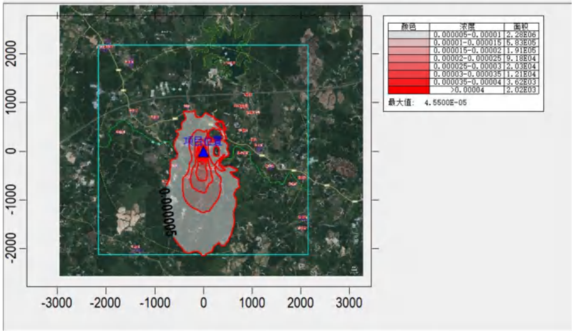
图 6.2-33. PM 10 贡献值年平均浓度分布图 (单位 mg/m 3 )
