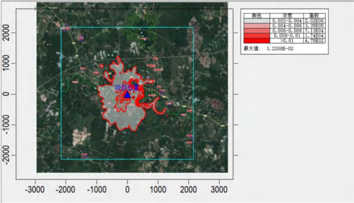
图 6.2-28. NO 2 贡献值日平均浓度分布图 (单位 mg/m 3 )
