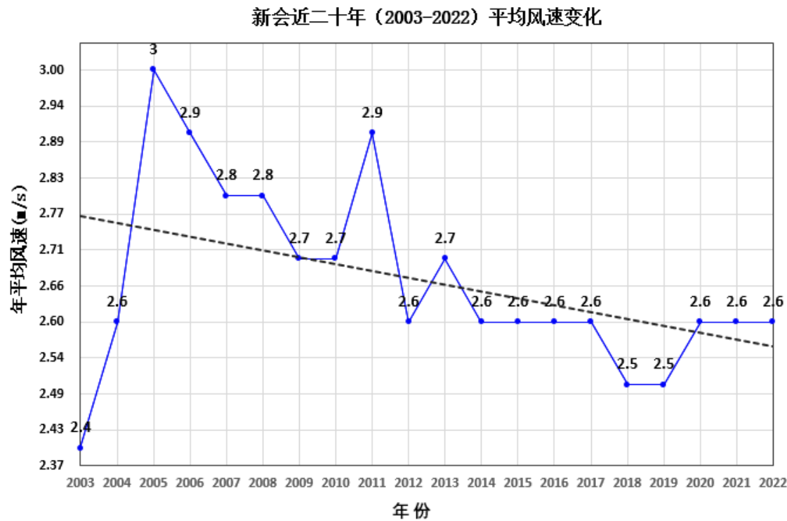
图5.4-7 新会气象站年平均风速(单位：m/s)
