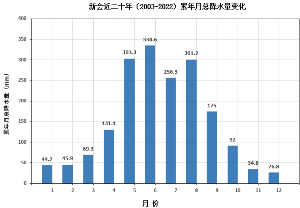
图5.4-3 新会气象站 2003~2022 年平均降雨量月变化
