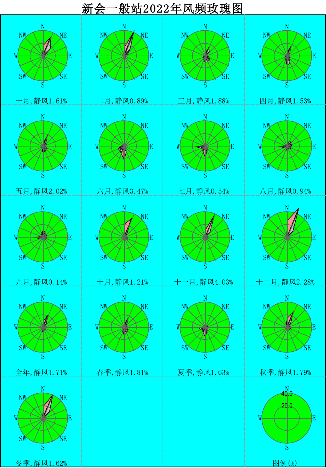
图5.4-11 2022 年新会风向玫瑰图
