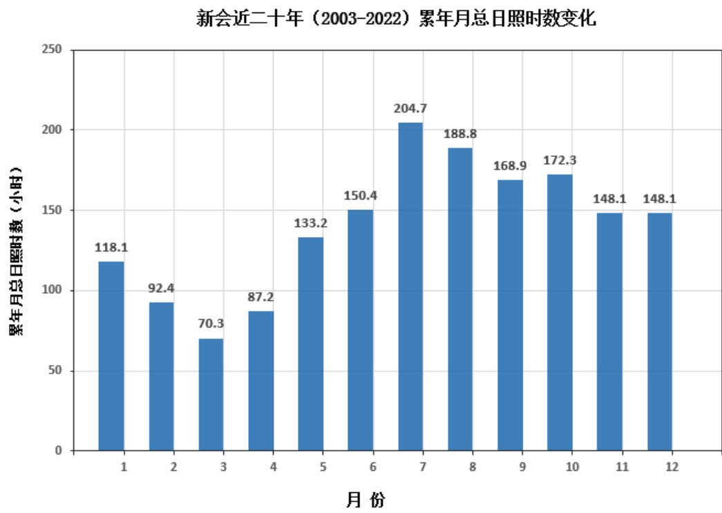
图5.4-4 新会气象站 2003~2022 年月日照时数变化
