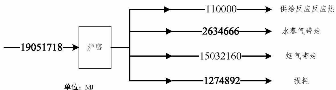
图2.3-13 项目热平衡图
