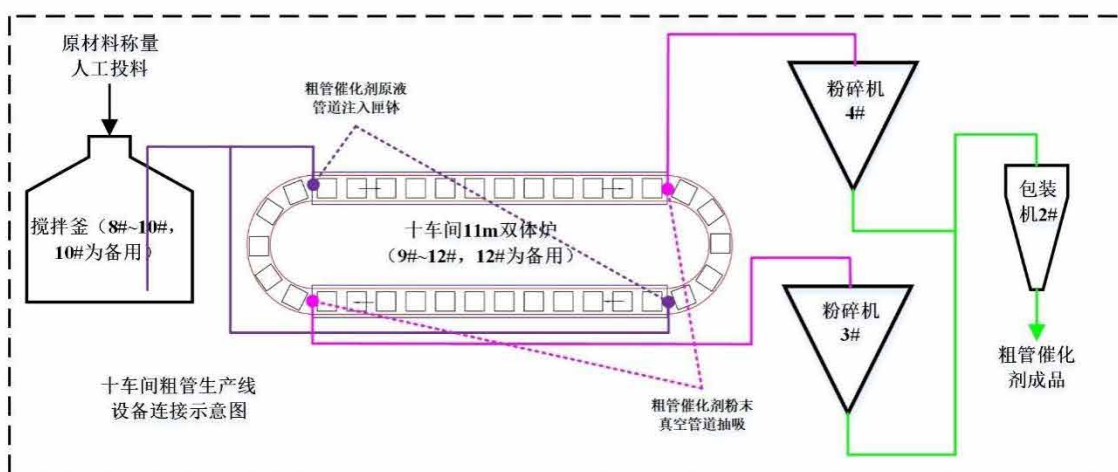
图2.3-4 十车间粗管生产线设备连接示意图
