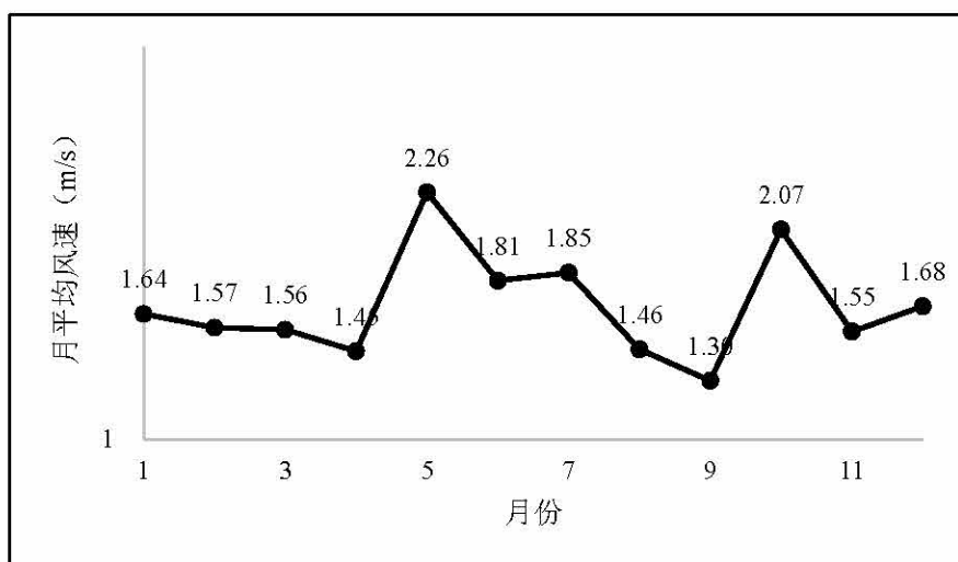
图5.2-12 2022 年月平均风速变化曲线
