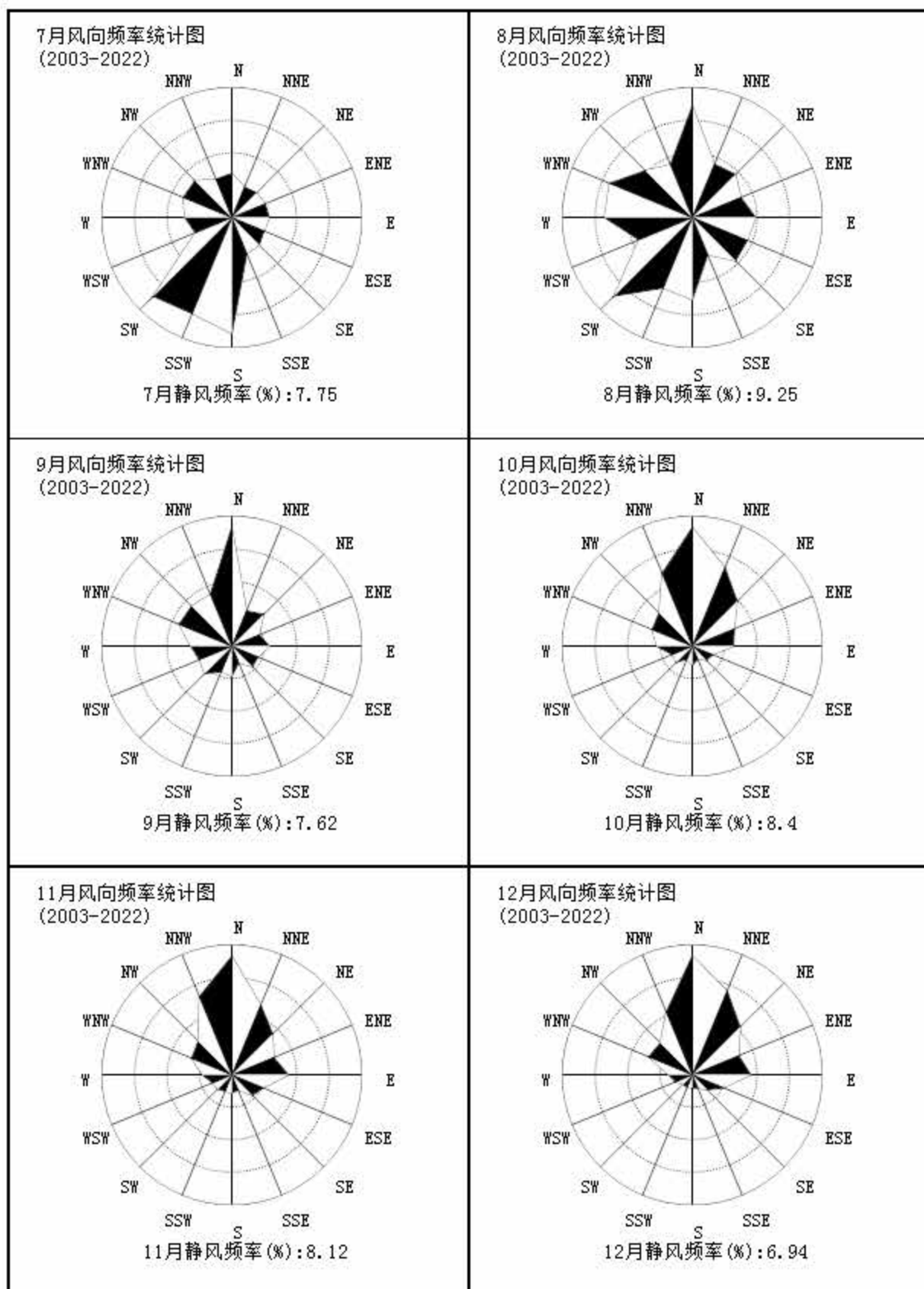
图5.2-2 各月风向频率统计图
