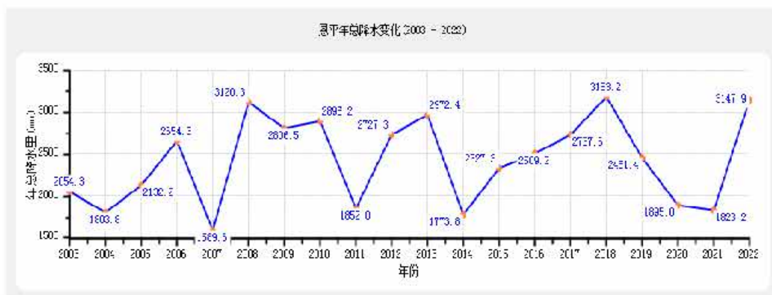
图5.2-6 恩平年总降水量(单位：毫米)
