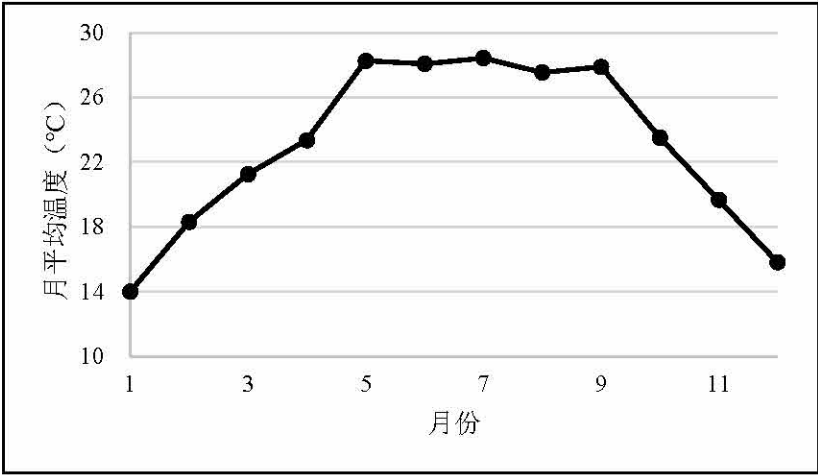
图5.2-11 2022 年月平均气温变化曲线
