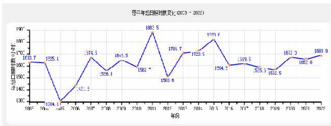
图5.2-8 恩平年日照时长(单位: 小时)
