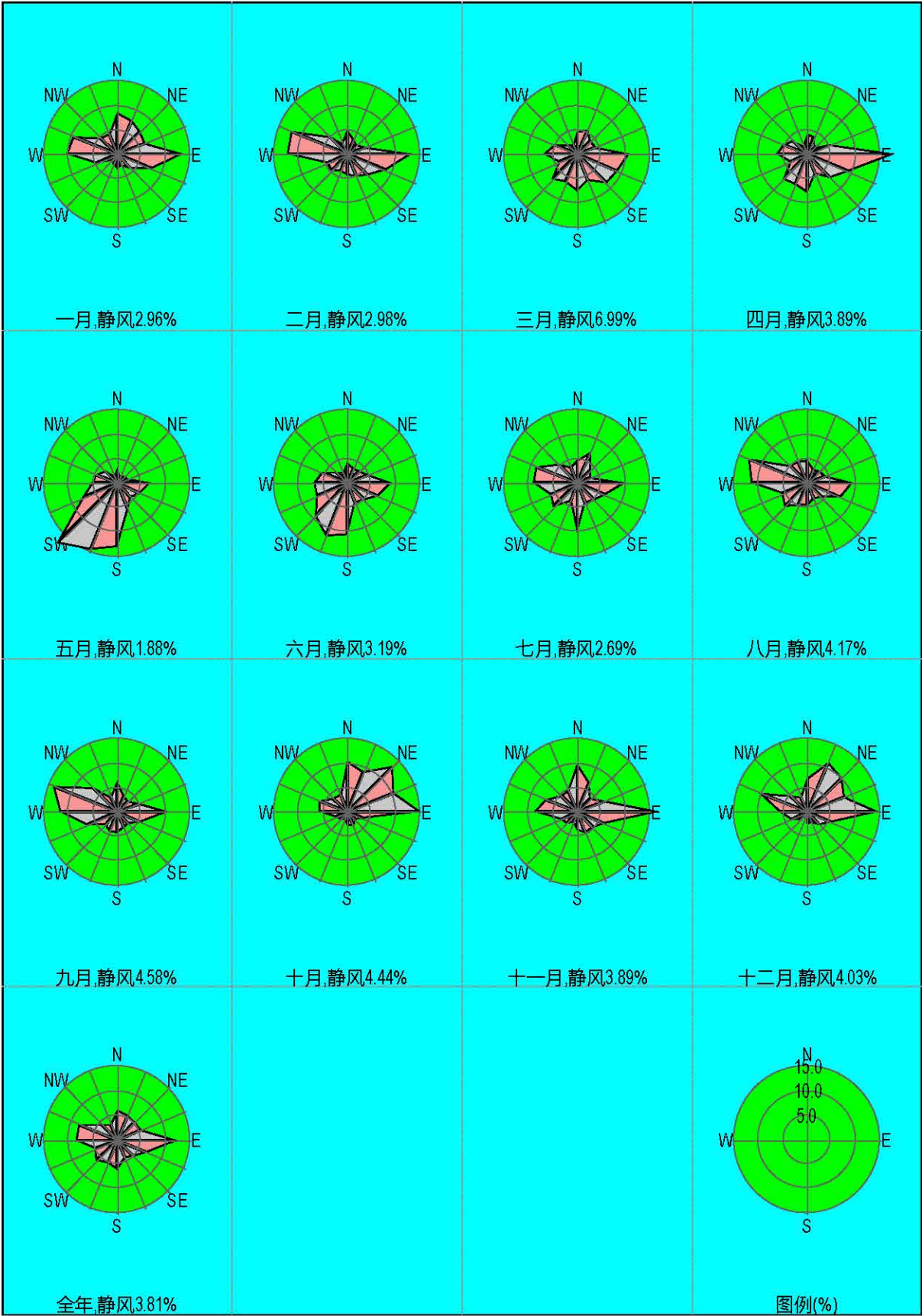
图5.2-13 恩平 2022 年风频玫瑰图
