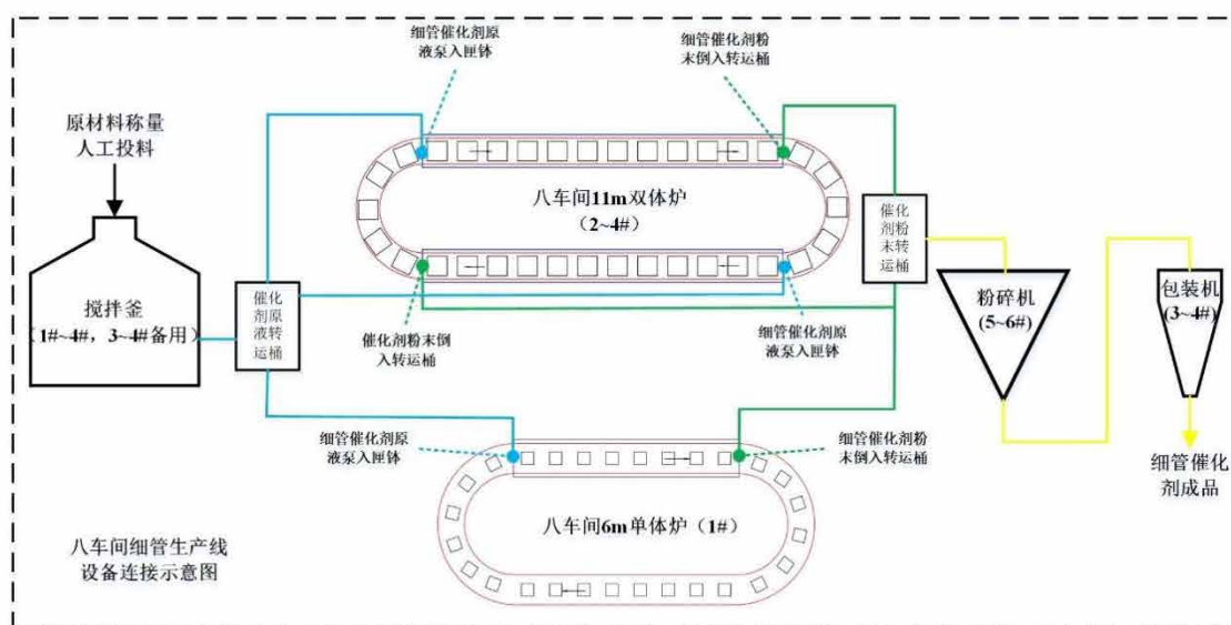
图2.3-5 八车间细管生产线设备连接示意图
