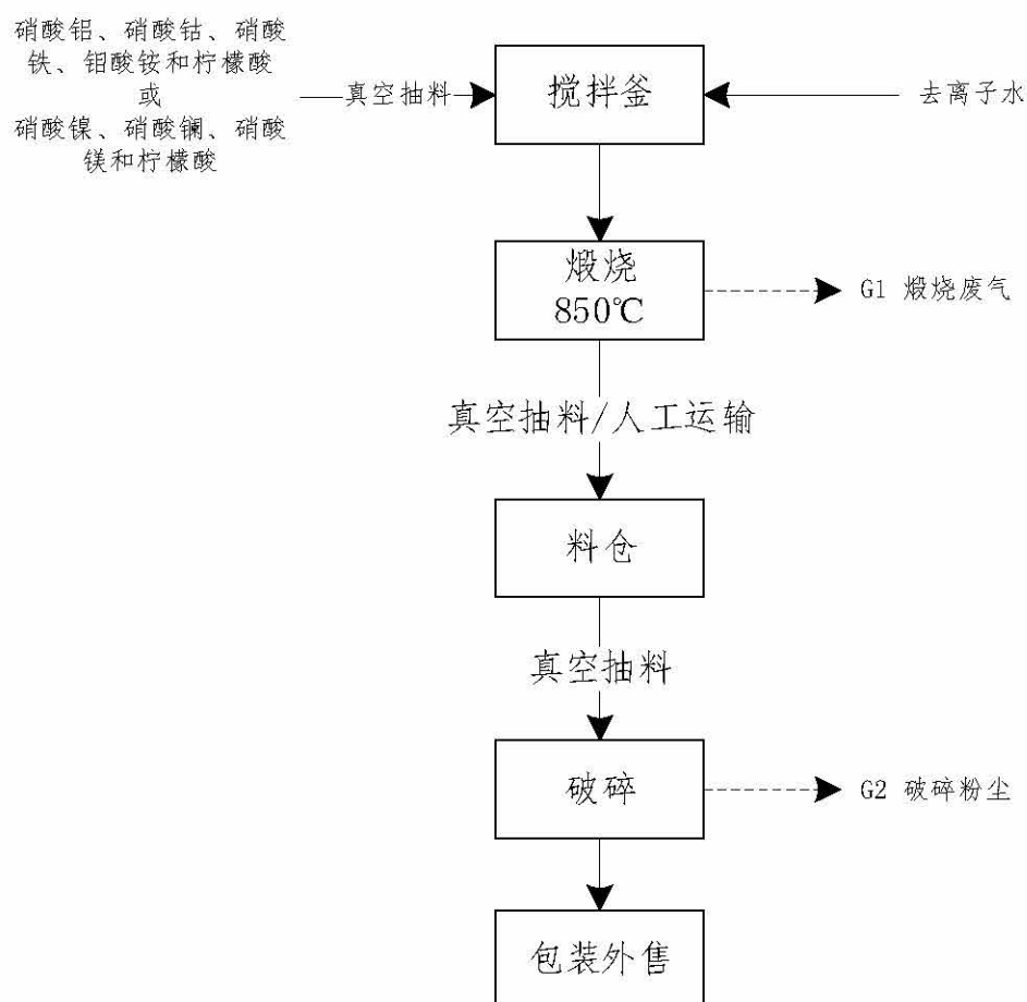
图2.3-11 项目工艺流程图
