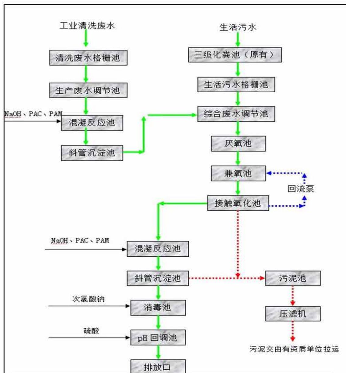
图6.2-1 废水处理工艺流程
