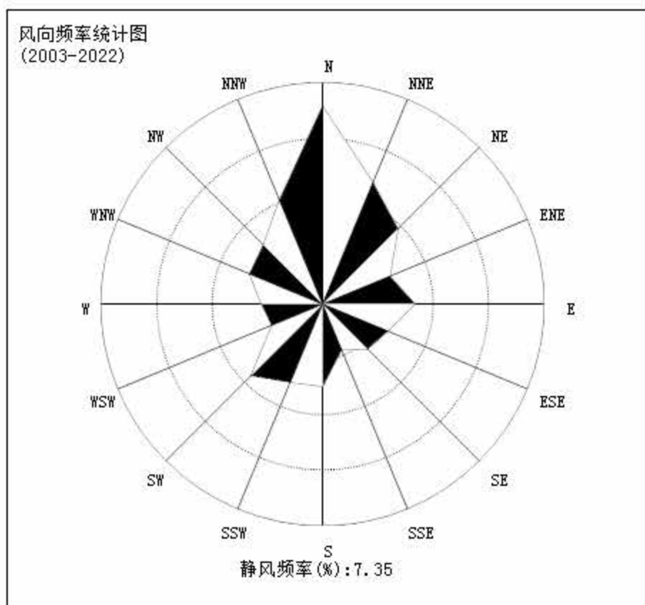
图5.2-1 恩平多年风向玫瑰图
