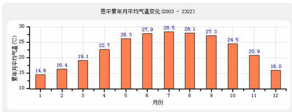
图5.2-3 恩平月平均气温变化示意图 (单位: °C)
