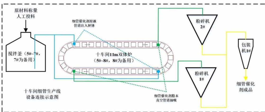
图2.3-3 十车间细管生产线设备连接示意图
