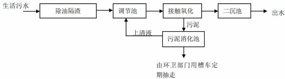
图5.3-1 废水处理系统处理流程一览
