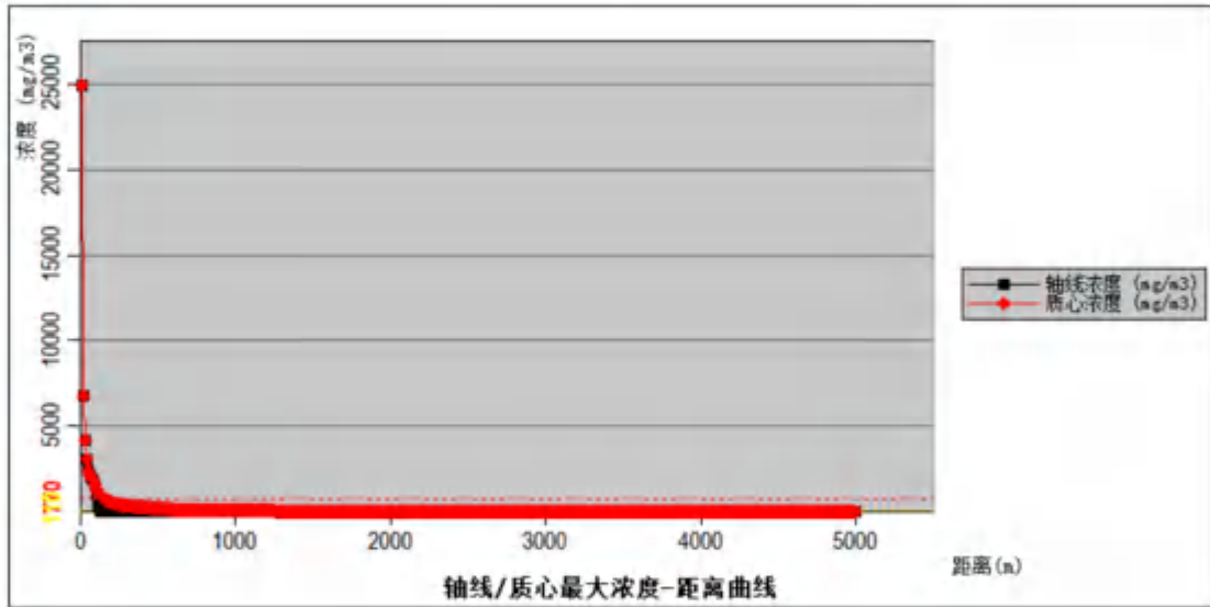
图 2.6-6 最不利气象条件下，液氨泄漏 \text{NH}_3 的最大落地浓度曲线图
