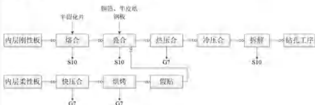
图2-11 压合工序
