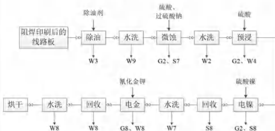
图 2-20 电镍金工艺流程
