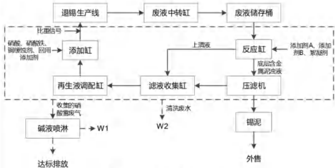
图 2-4 锡资源回收工艺流程图
