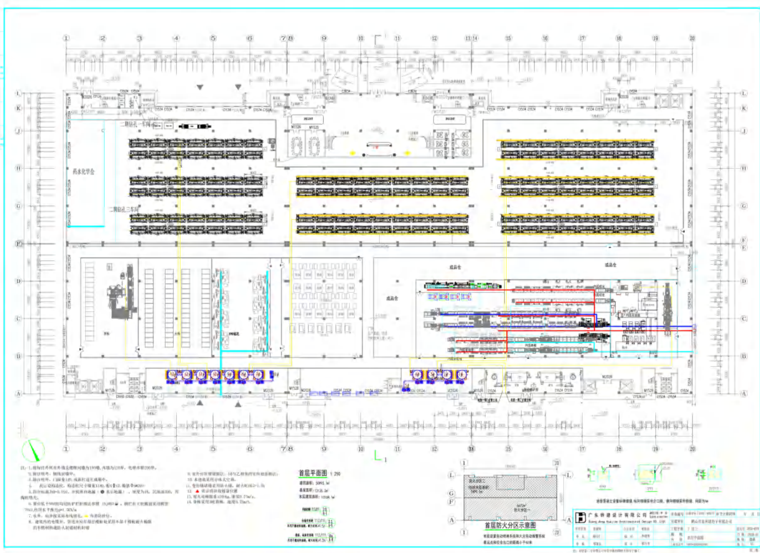
附图 43 号厂房各楼层设备布局图
