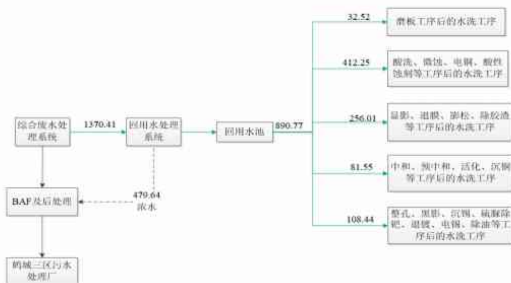
扩建项目中水回用系统水平衡图
