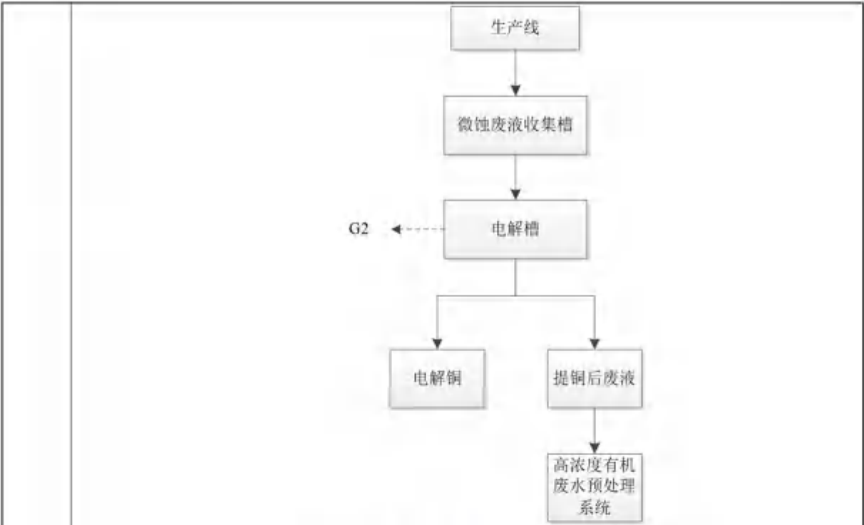
图 2-3 微蚀废液提铜系统工艺流程示意图
