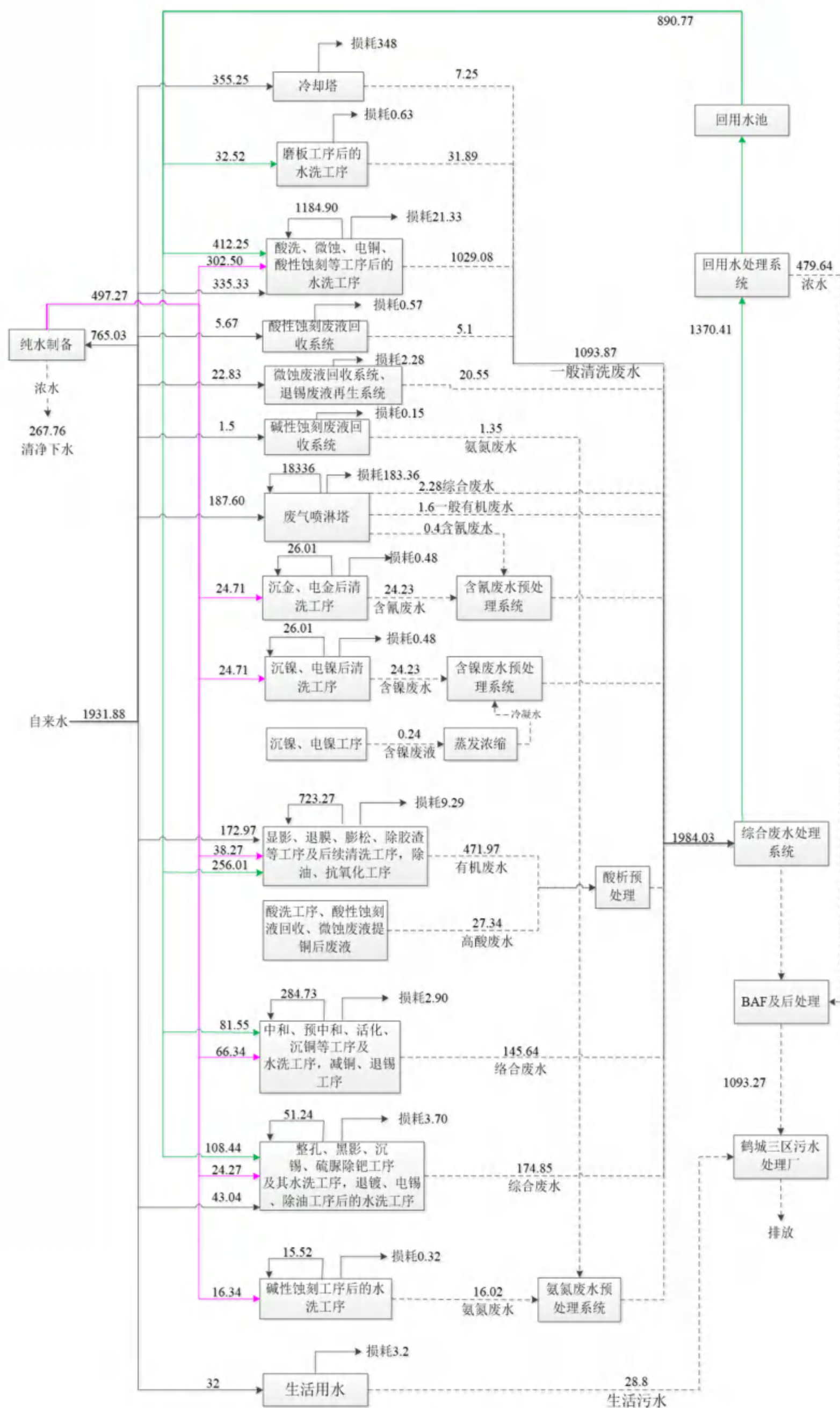
图2-27 扩建项目水平衡图 (单位: t/d)
