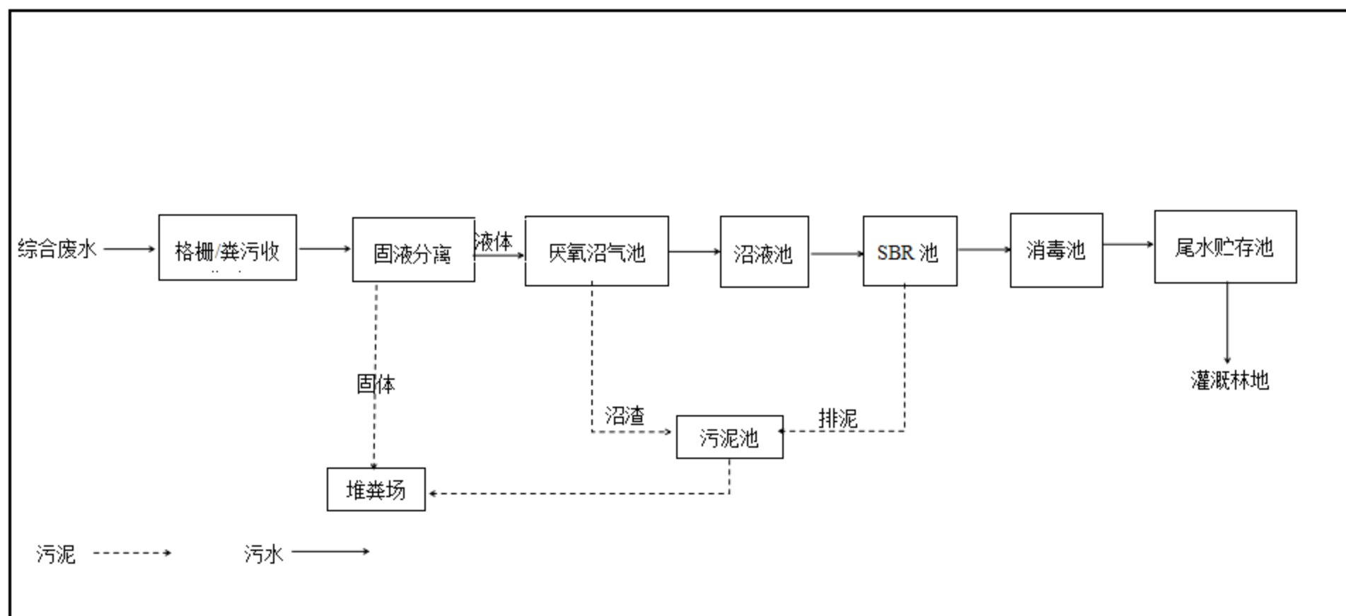
图 3.2-1. 现有项目废水处理流程图
