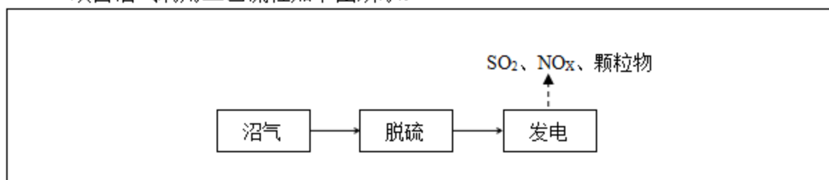
图 4.2-5 项目沼气利用发电工艺图
