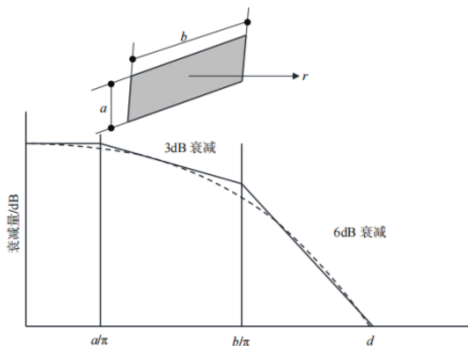
图 6.2-41.长方形面声源中心轴线上的衰减特性
