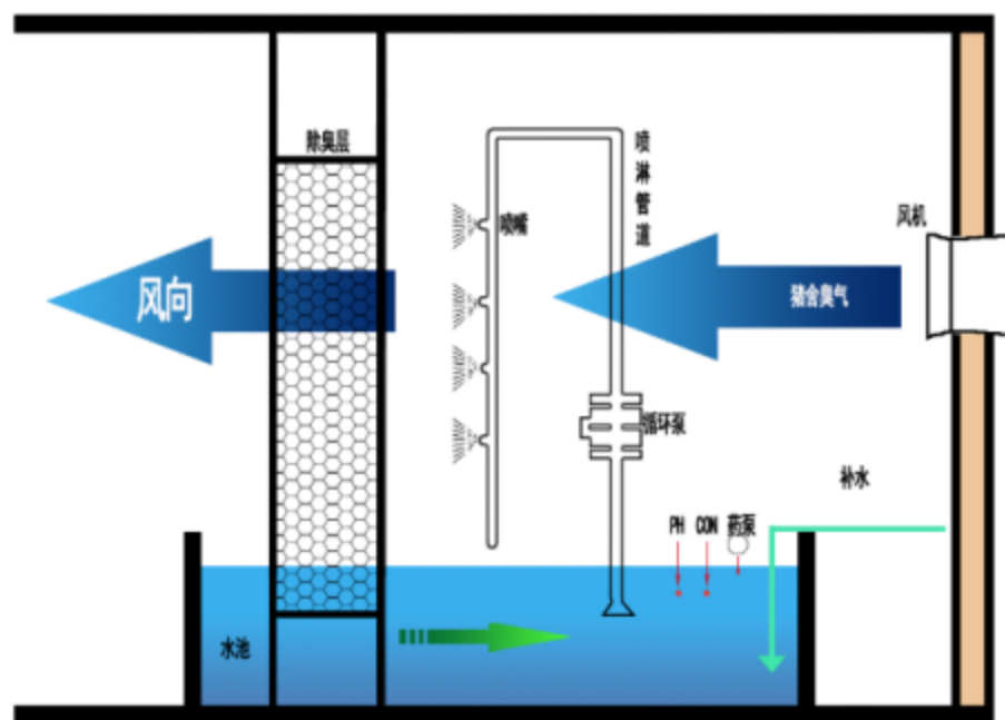
图 7.2-5 猪舍使用生物除臭剂喷淋除臭示意图
