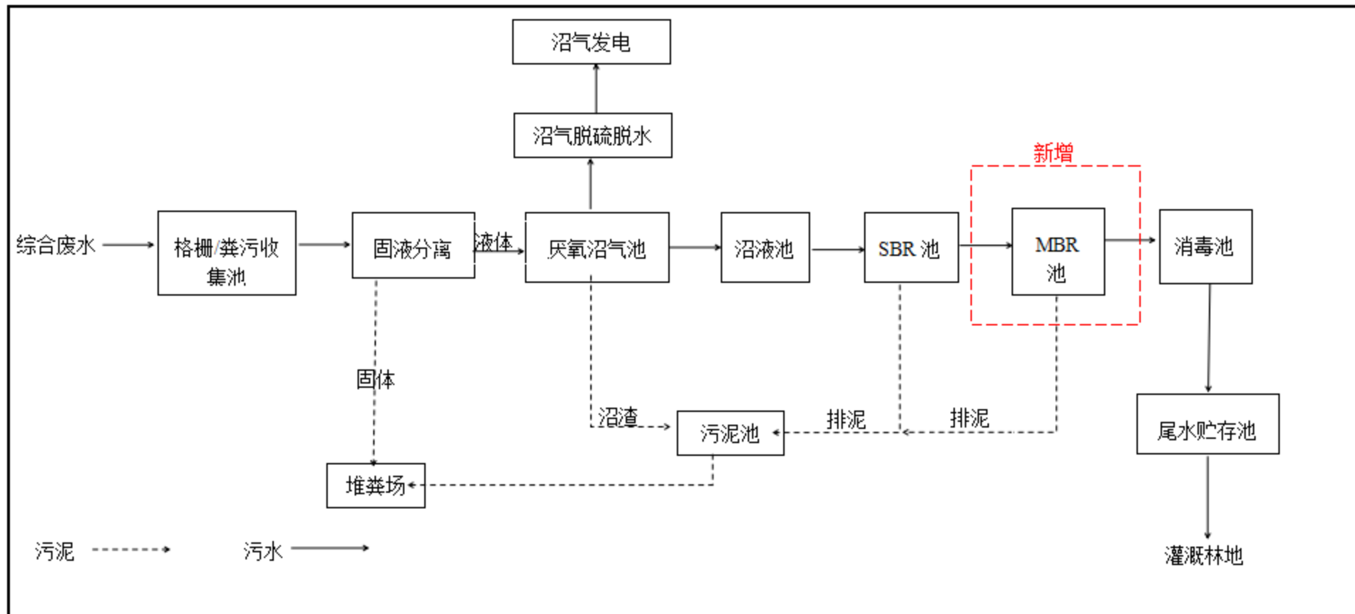
图 7.2-1.改扩建项目废水处理流程图
