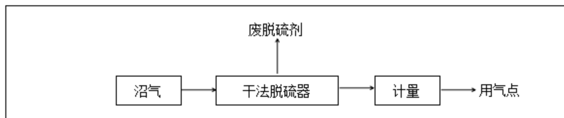
图 4.2-6 项目沼气净化示意图
