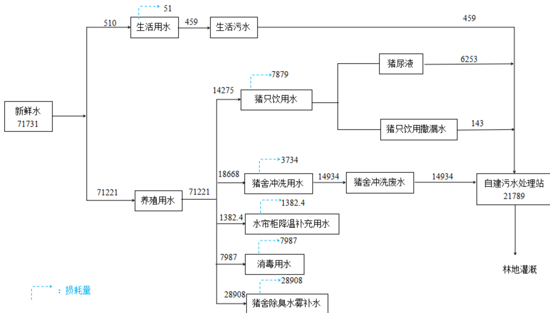
图 4.1-8.改扩建后项目水平衡图 (单位: t/a)
