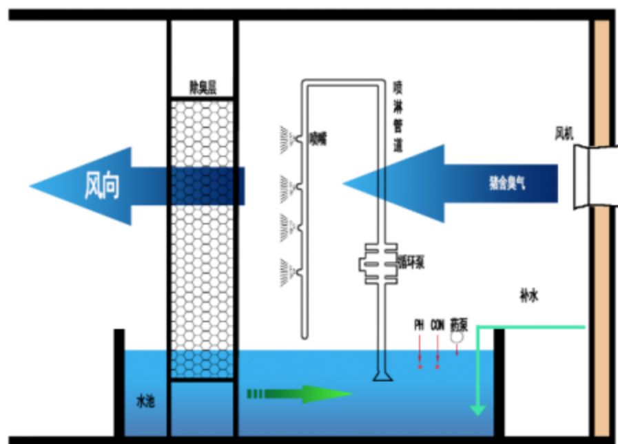
图 4.3-1.猪舍使用生物除臭剂喷淋除臭示意图
