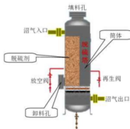
图 7.2-6. 脱硫塔结构图
