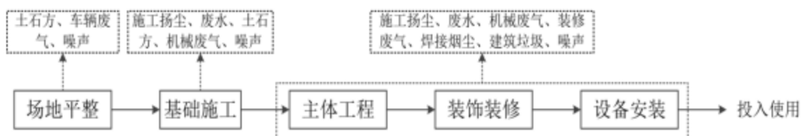
图 4.2-1. 项目施工期工艺流程及产污环节示意图
