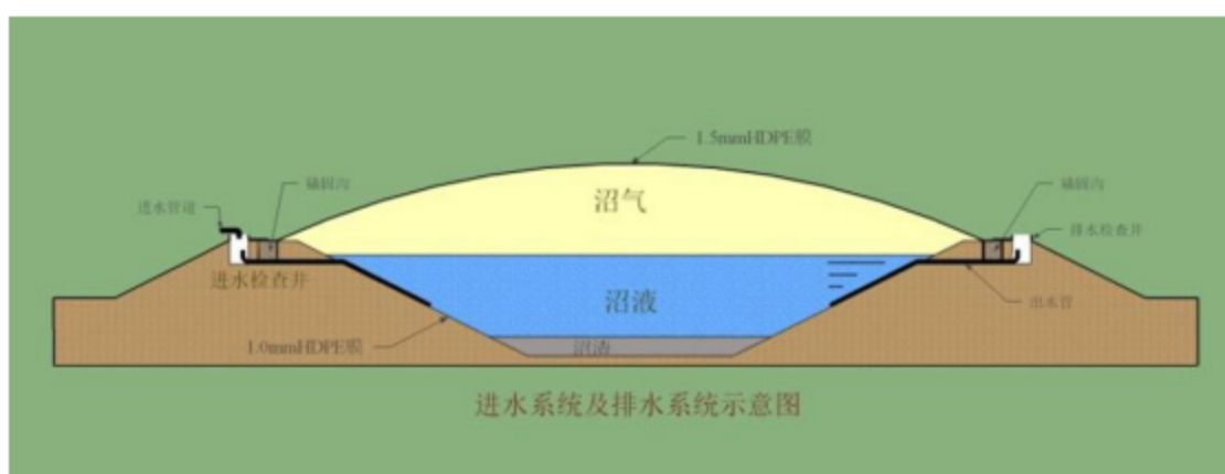
图 7.2-4.项目沼气池进水、排水系统示意图
