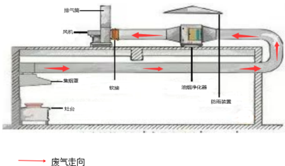
图 7.2-7.油烟净化处理工艺
