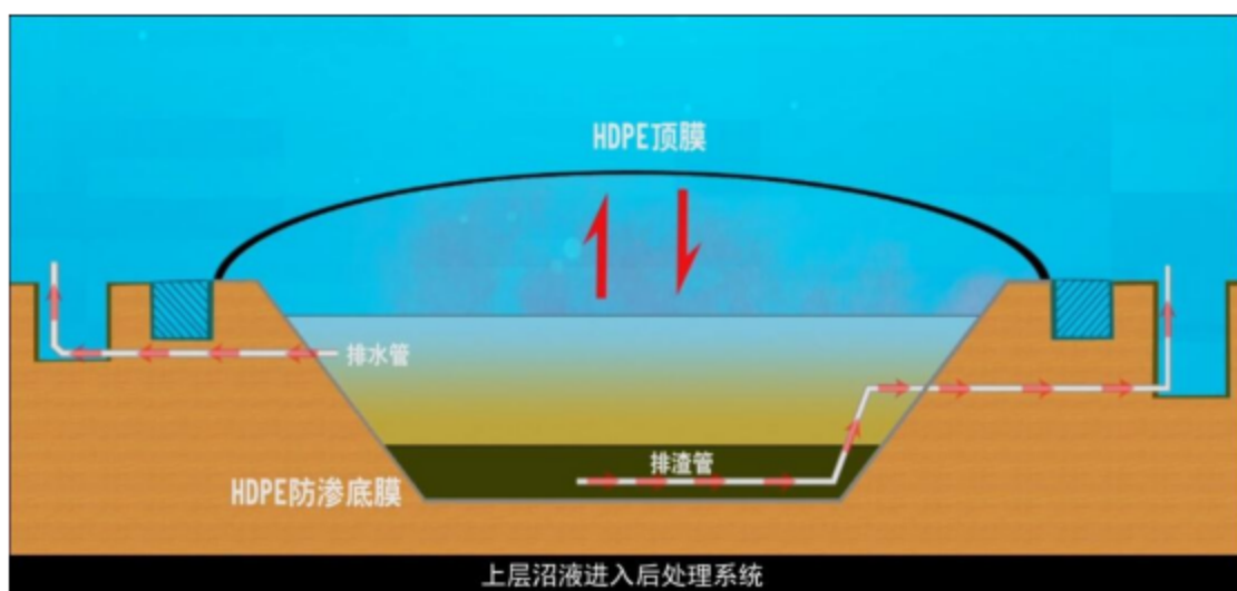
图 7.2-3.项目沼气池剖面示意图
