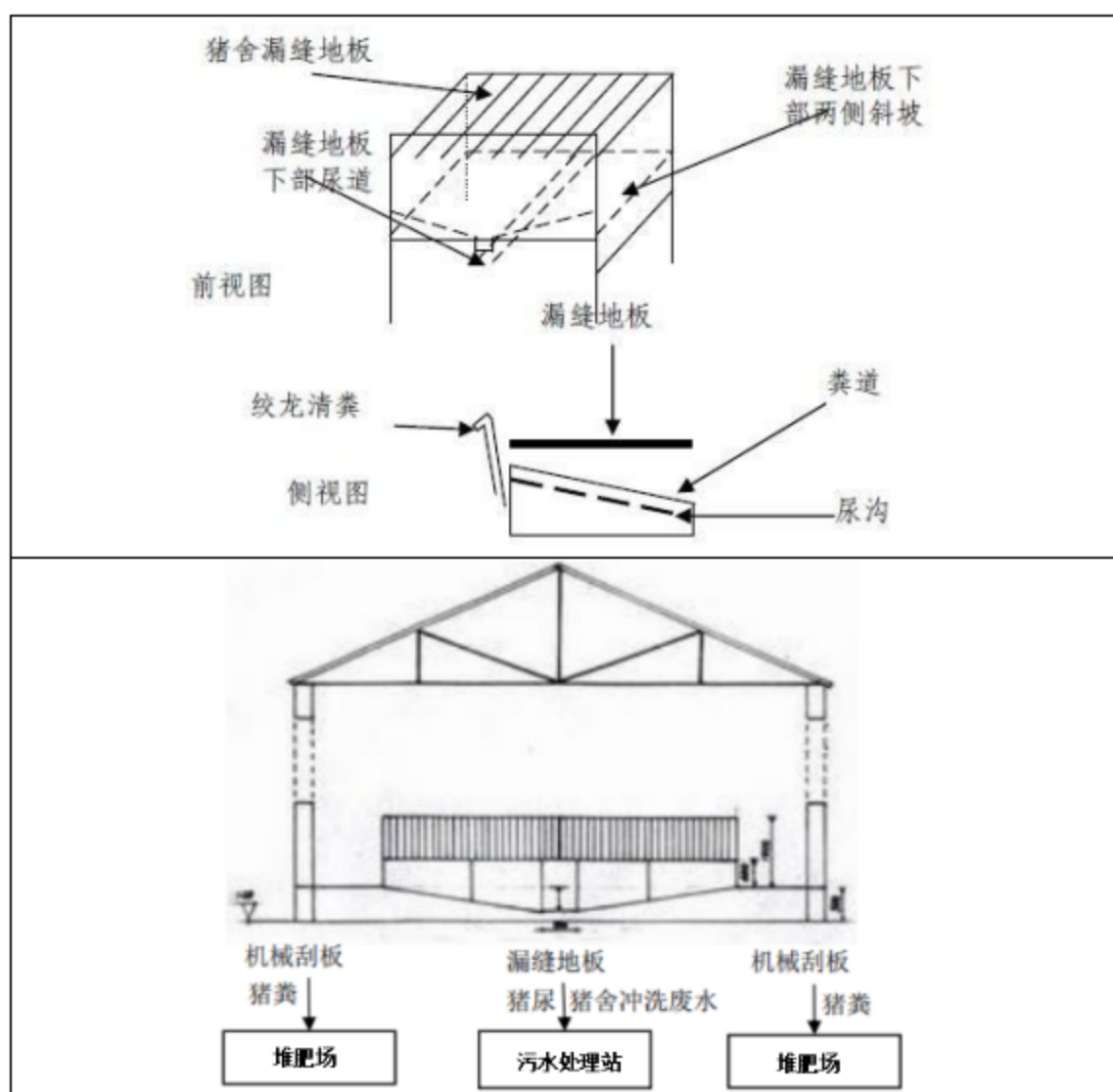
图 4.2-4.项目清粪工艺示意图
