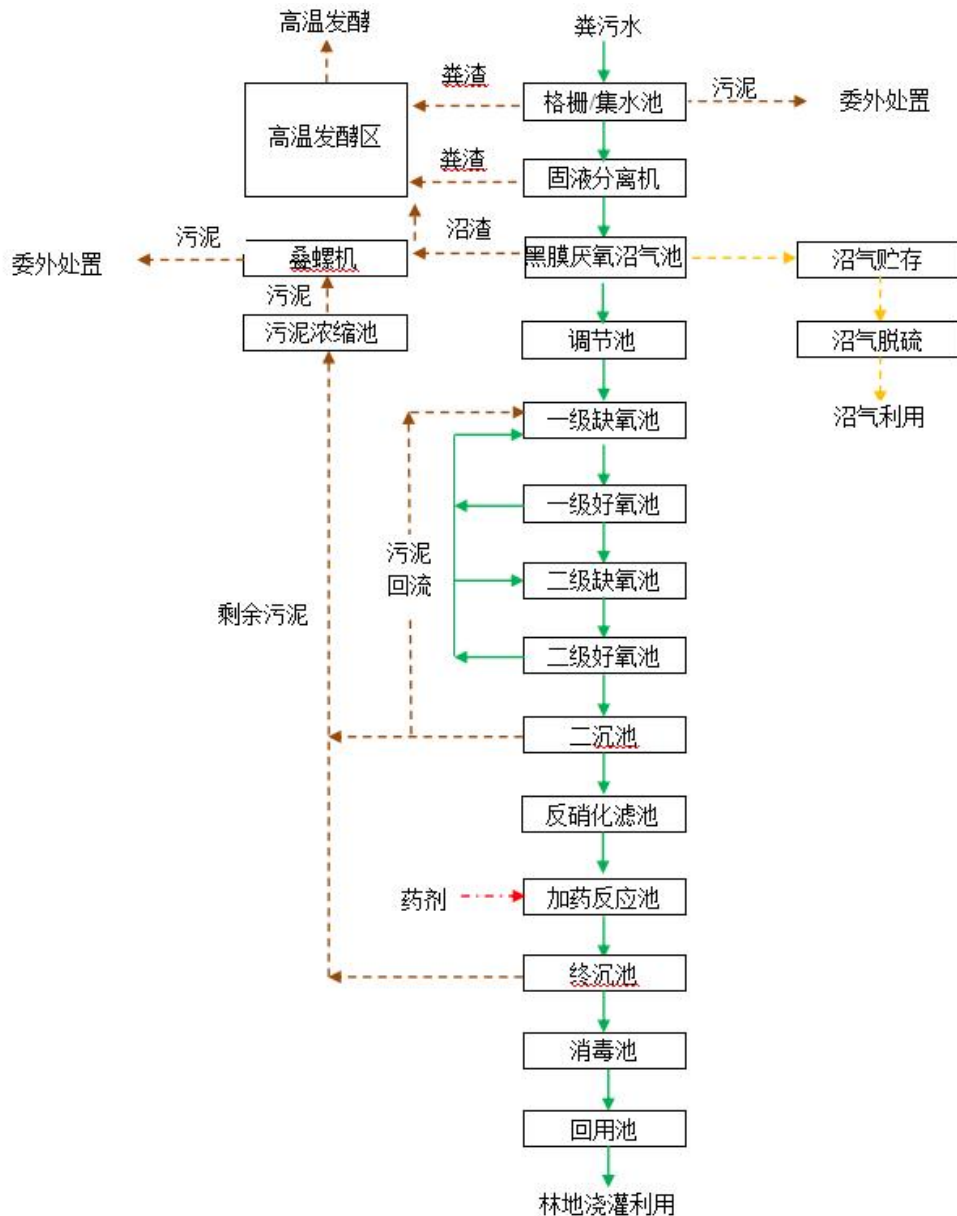
图 5.2-3 废水处理站处理工艺流程图
