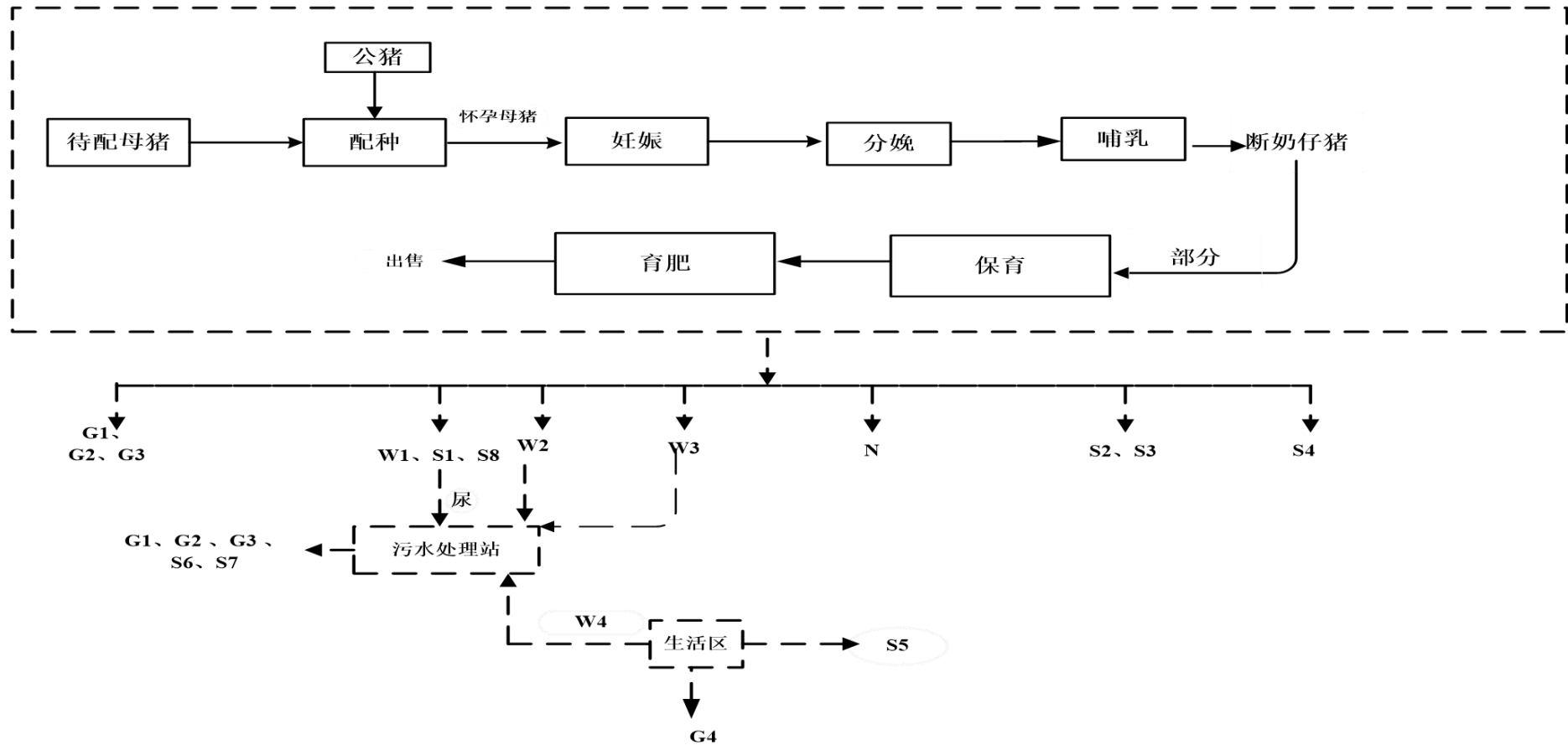
图 2.1-4 生猪养殖工艺流程和产污环节图
