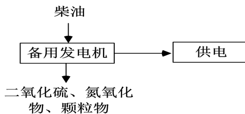
图 2.2-12 备用发电机供电工艺流程图
