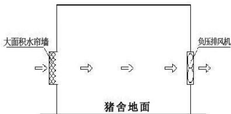
图 2.1-3 通风和降温示意图
