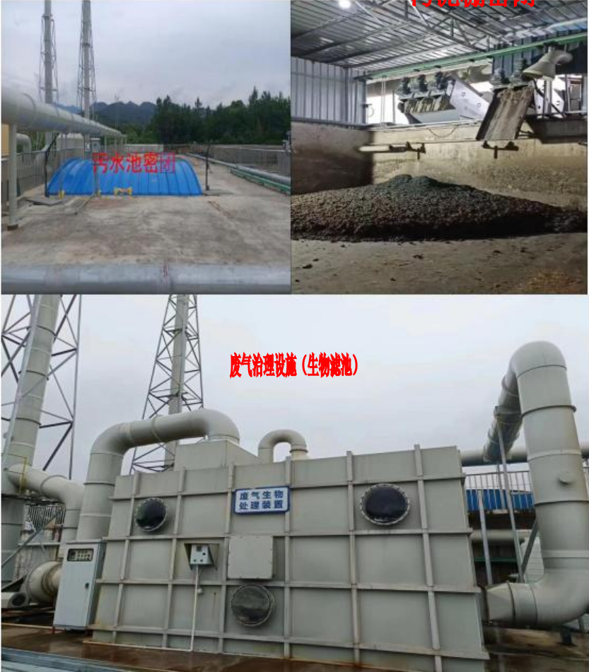
类比项目衢州华统现代化东方生猪养殖建设项目（先行）污水处理站恶臭收集治理设施照片
