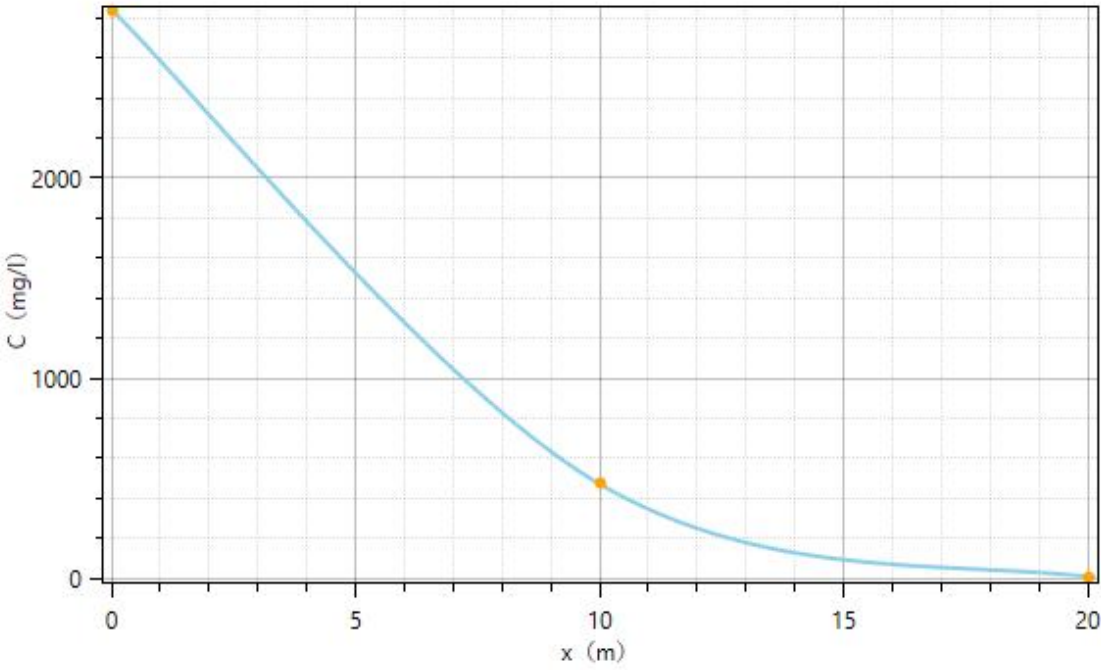
图 4.2-25 非正常工况下 30d 时下游轴向耗氧量浓度变化曲线
