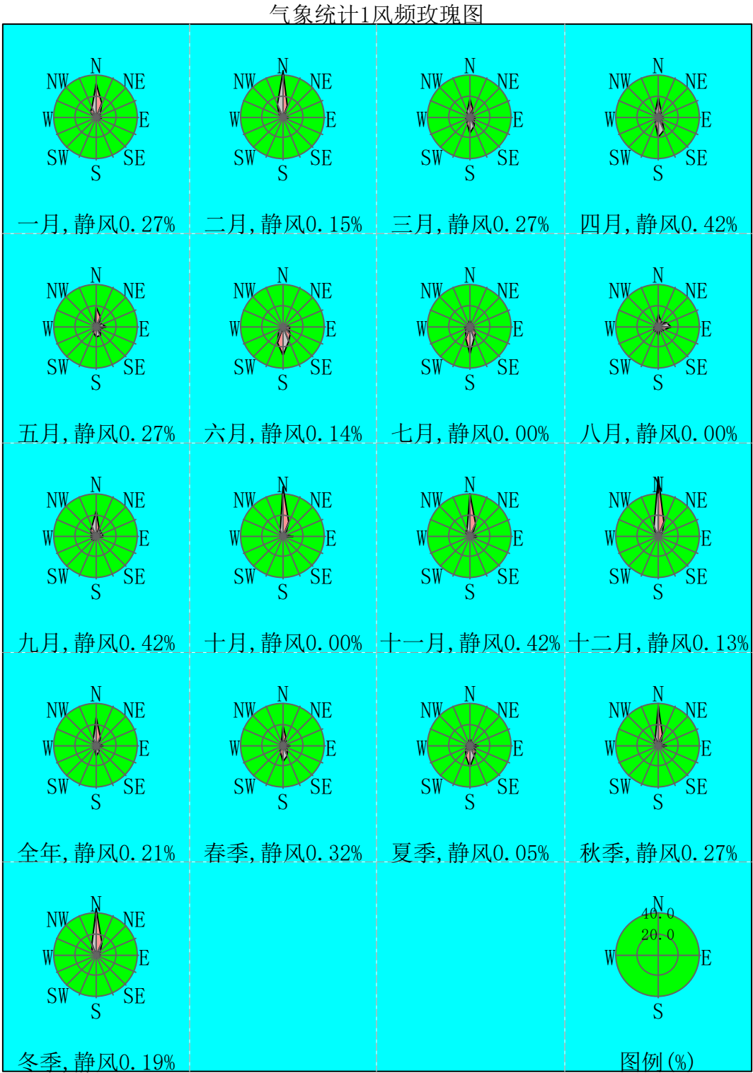
图 4.2-5 风频玫瑰图
