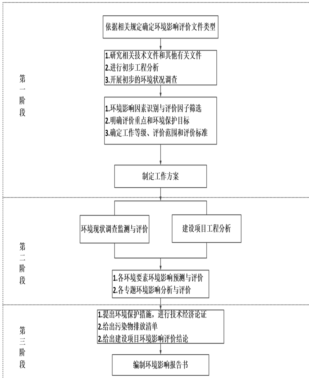
图 1.1-2 环评工作程序流程图
