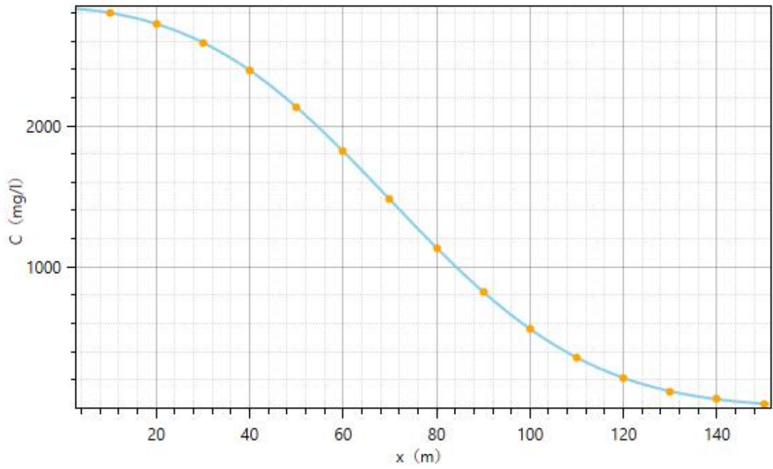
图 4.2-27 非正常工况下 1000d 时下游轴向耗氧量浓度变化曲线
