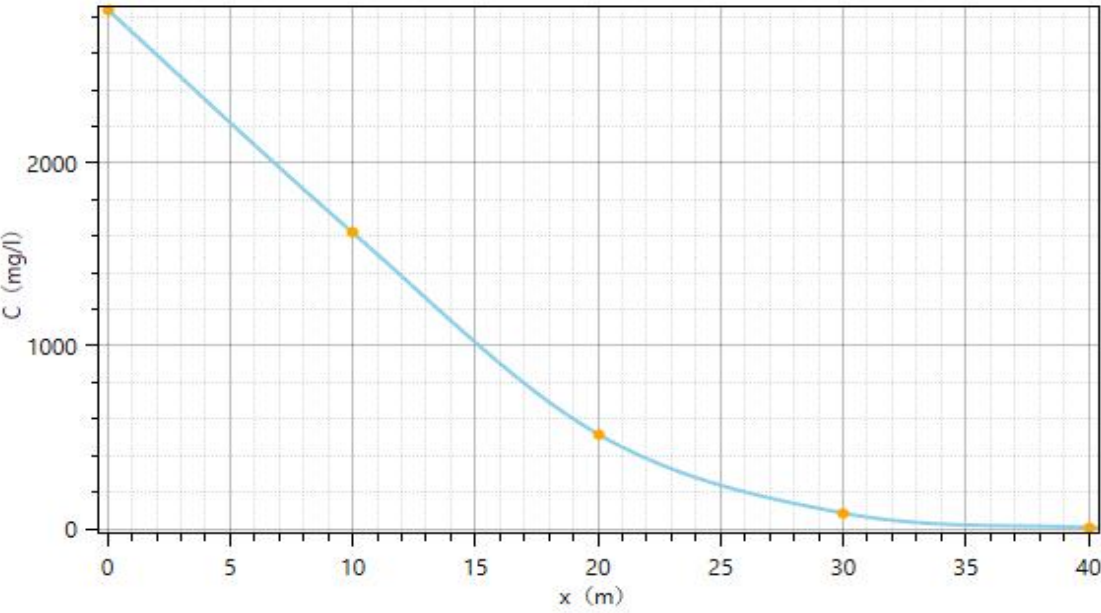
图 4.2-26 非正常工况下 100d 时下游轴向耗氧量浓度变化曲线
