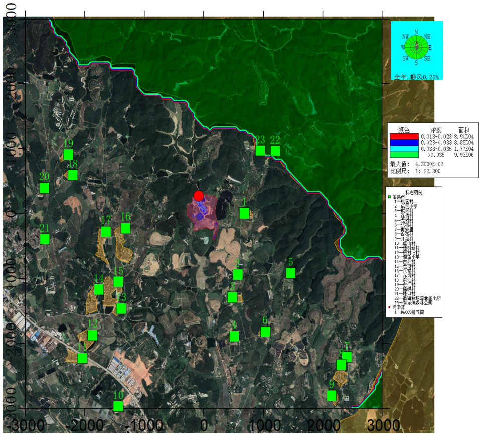
图 4.2-17B 正常排放条件下一类区 PM 10 日平均浓度预测值分布图
