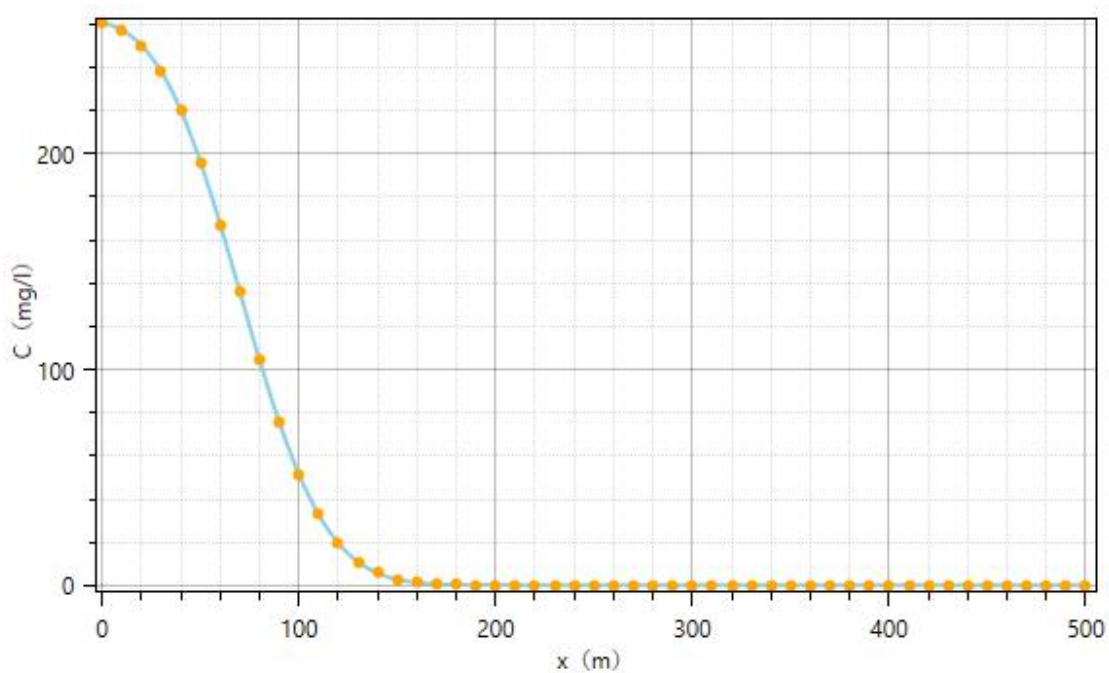
图 4.2-30 项目非正常工况下 1000d 时下游轴向氨氮浓度变化曲线
