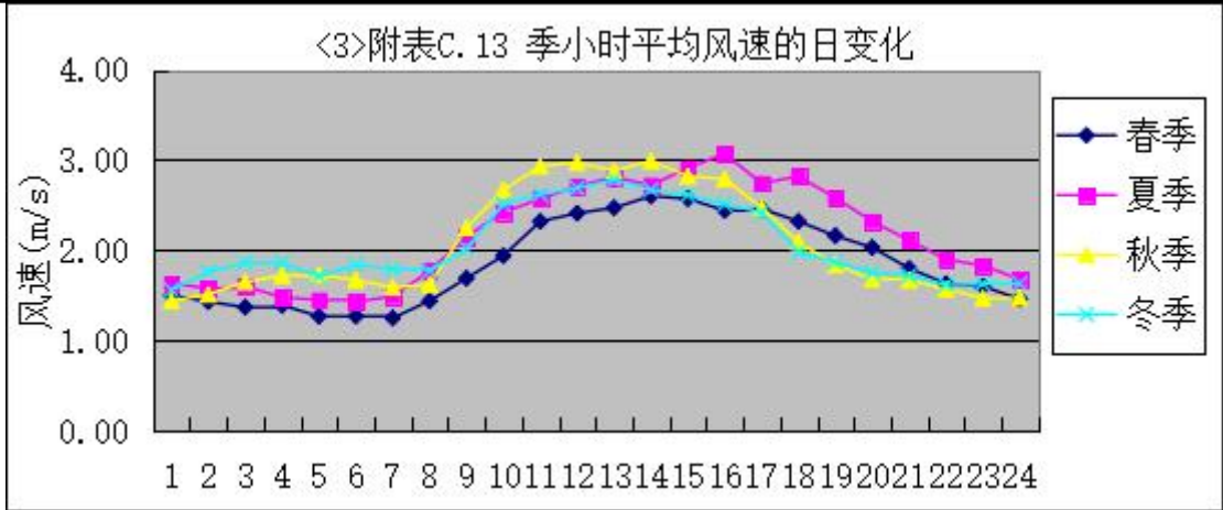
图 4.2-4 季小时平均风速的日变化图
