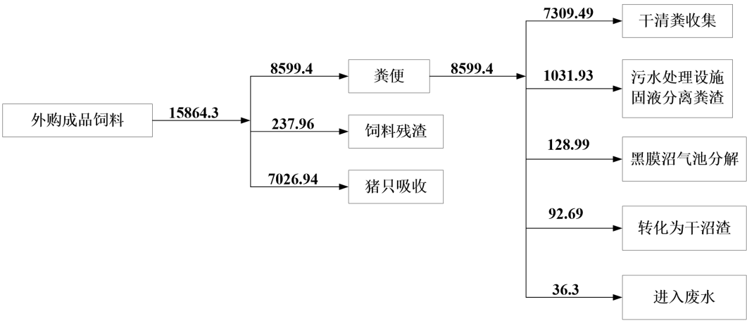
图 2.2-6 项目总物料平衡图（单位：t/a）
