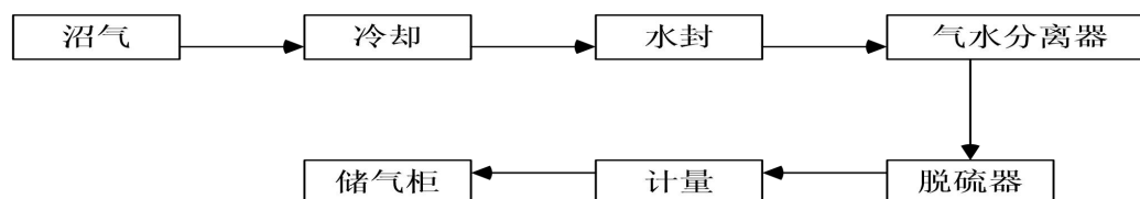
图 2.3-8 沼气净化工艺流程
