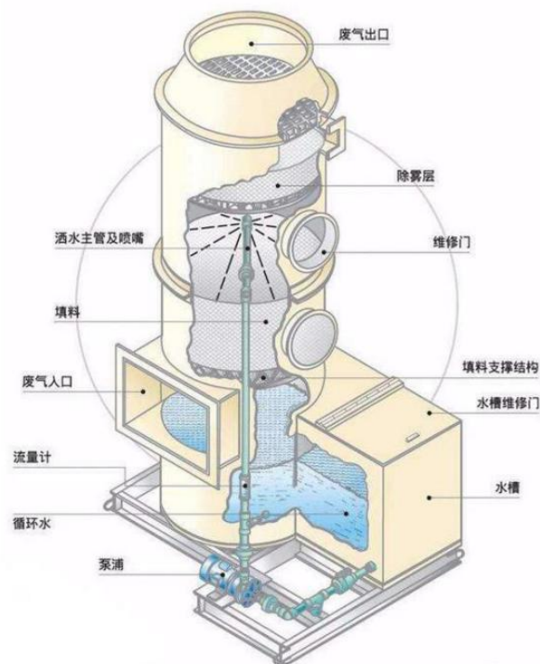
图 5.2-1 生物滴滤塔示意图
