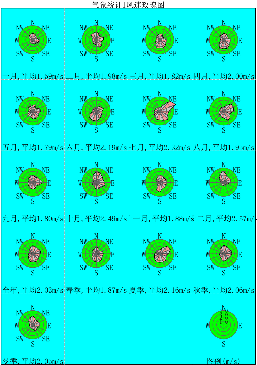
图 4.2-6 风速玫瑰图
