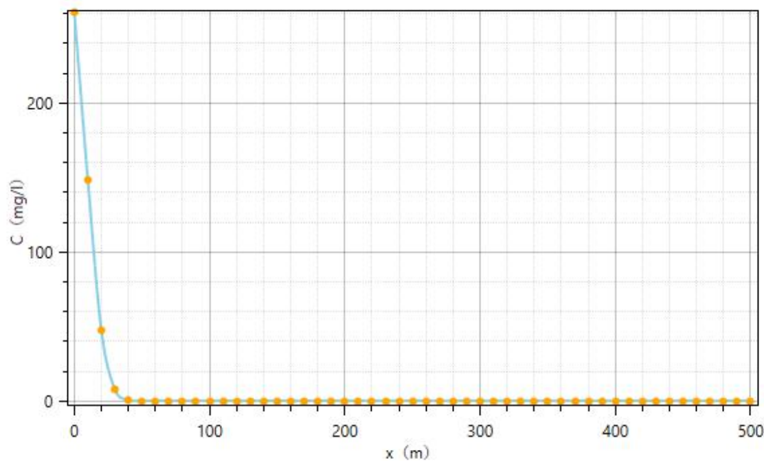
图 4.2-29 项目非正常工况下 100d 时下游轴向氨氮浓度变化曲线
