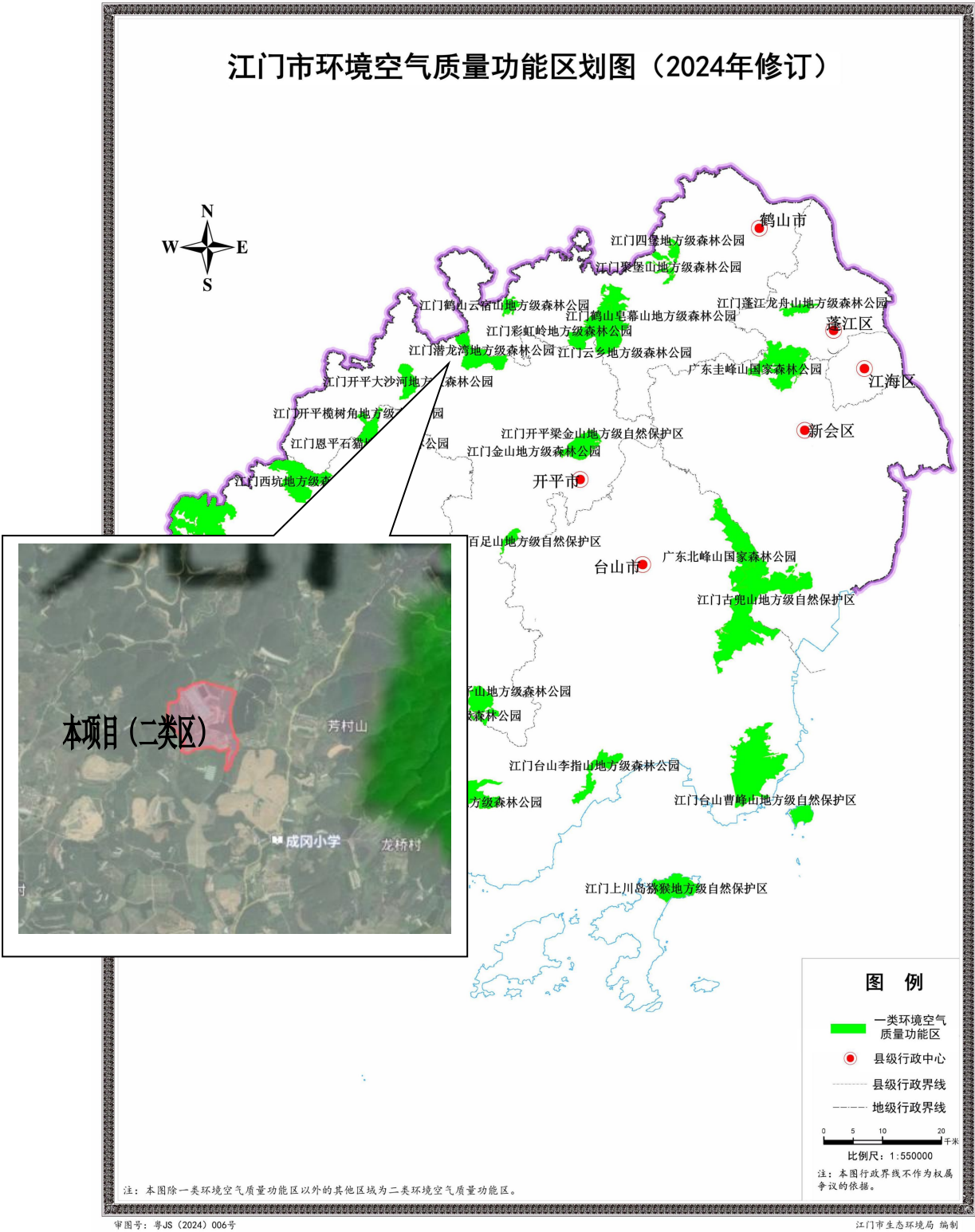
图 1.3-3 江门市大气环境功能区划图
