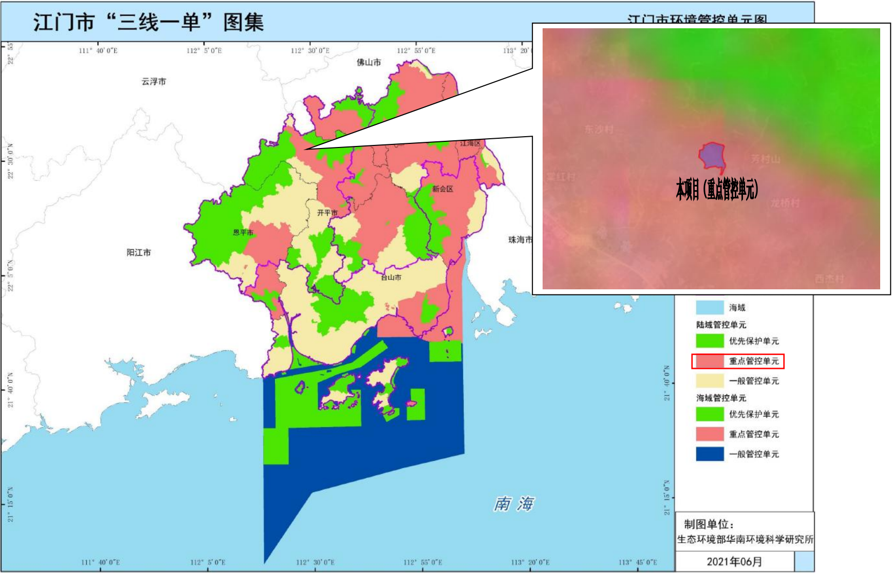
图 1.1-7 江门市环境管控单元图
