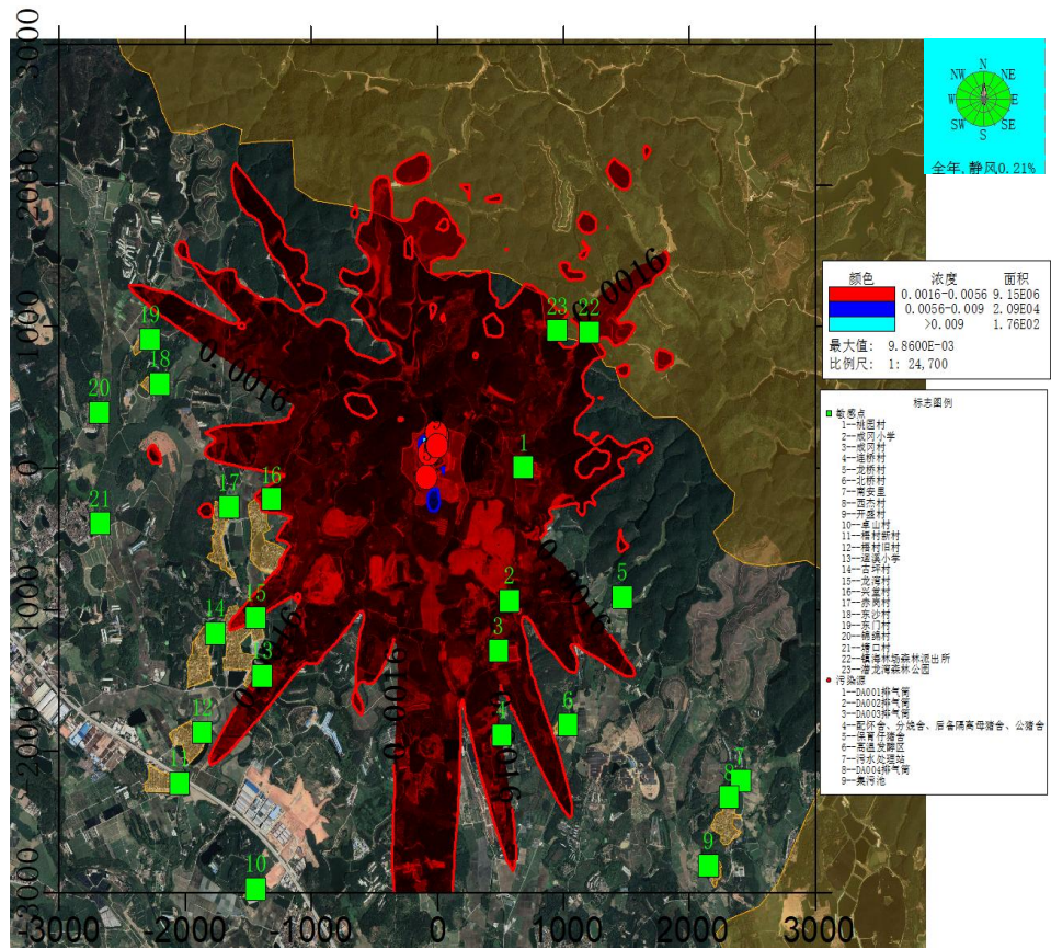
图 4.2-19 正常排放条件下各敏感点 H_2S 的 1 小时浓度预测值分布图
