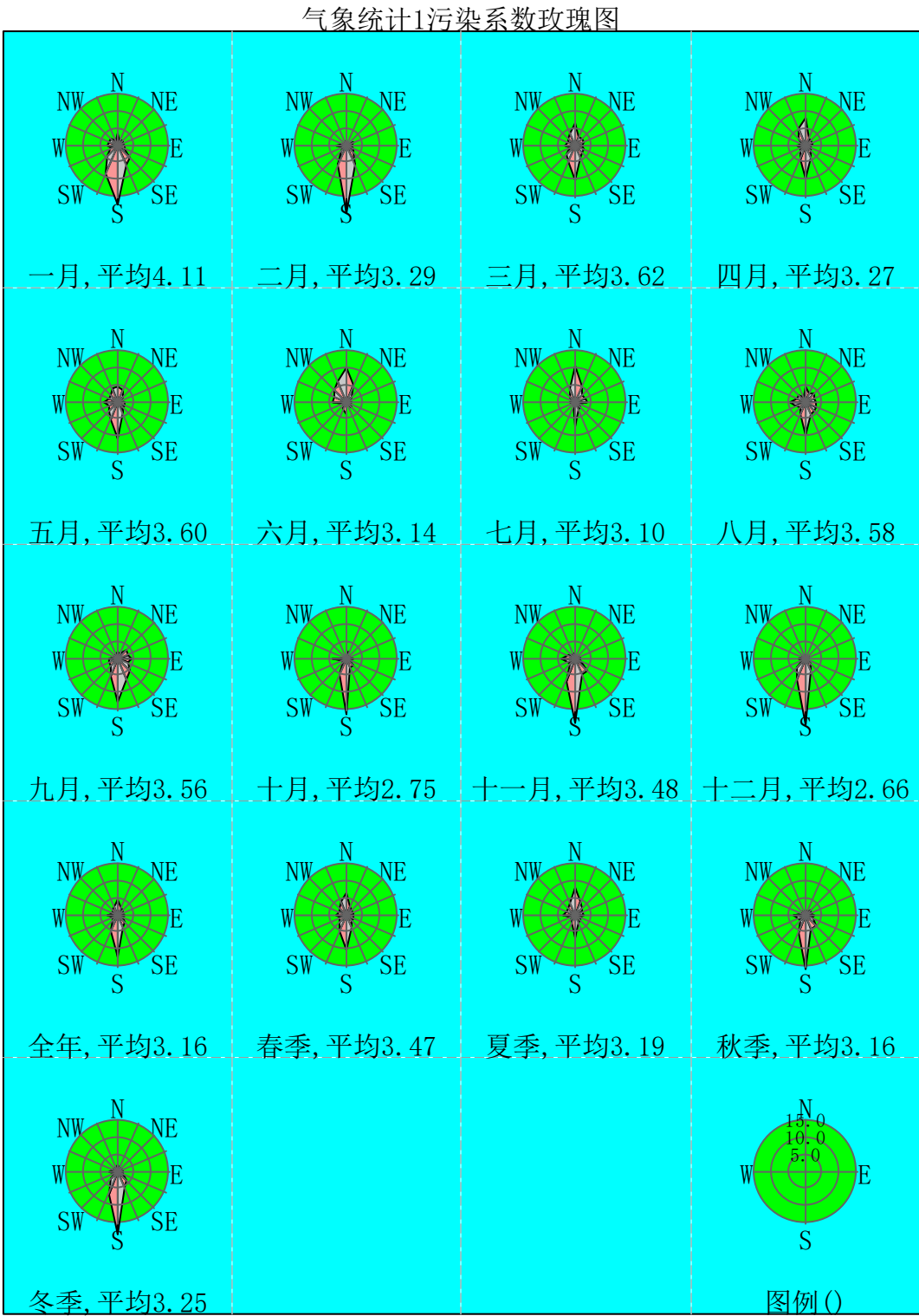
图 4.2-7 污染系数玫瑰图
