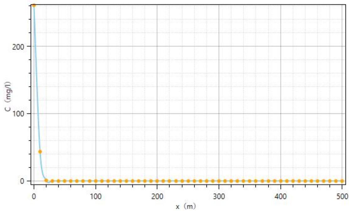
图 4.2-28 项目非正常工况下 30d 时下游轴向氨氮浓度变化曲线
