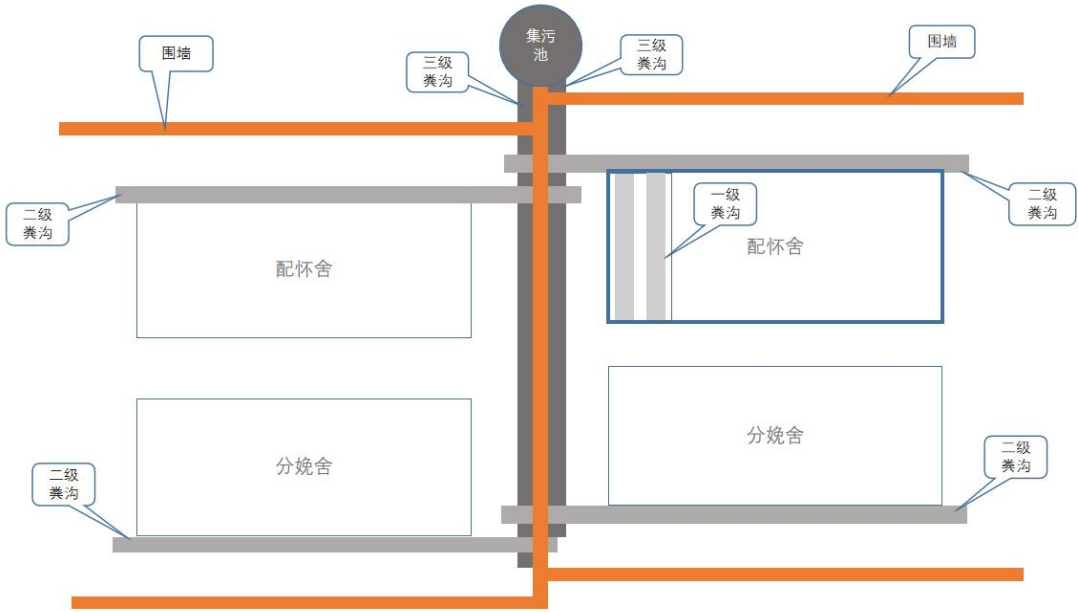
图 2.3-4 项目粪污沟与集污池关系图
