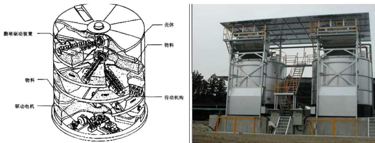
图 2.3-6 高温发酵罐设备示意图和同类养殖场设备照片
