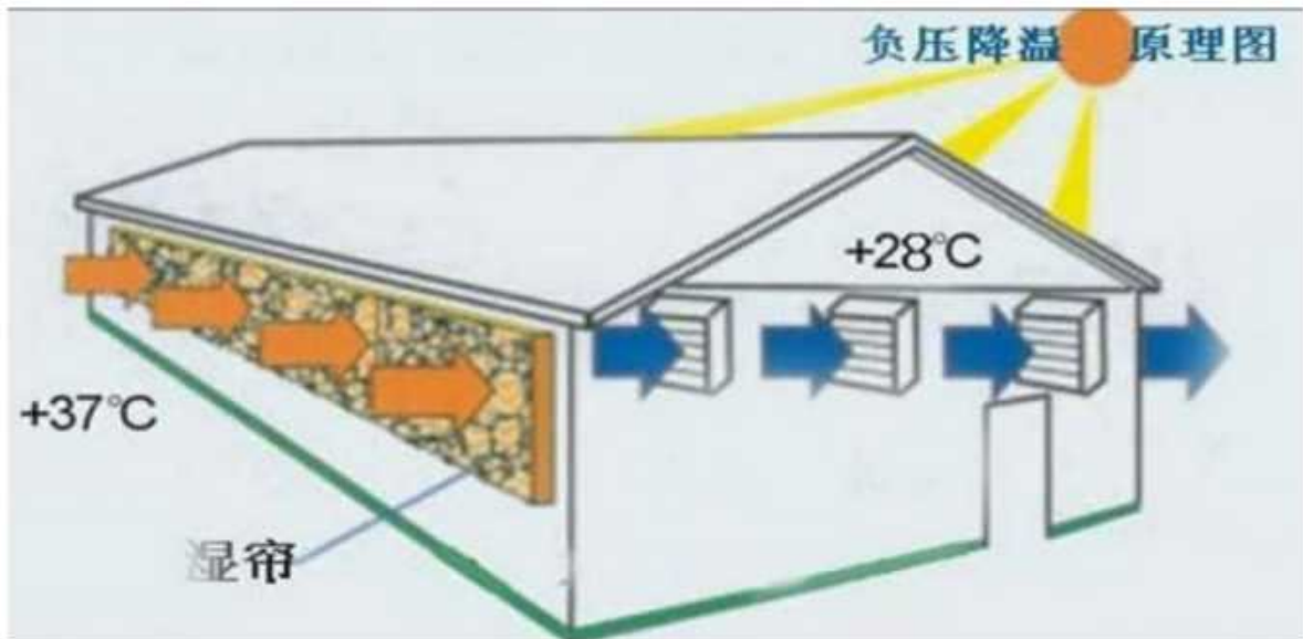
图 3.1-3 猪舍水帘降温系统示意图
