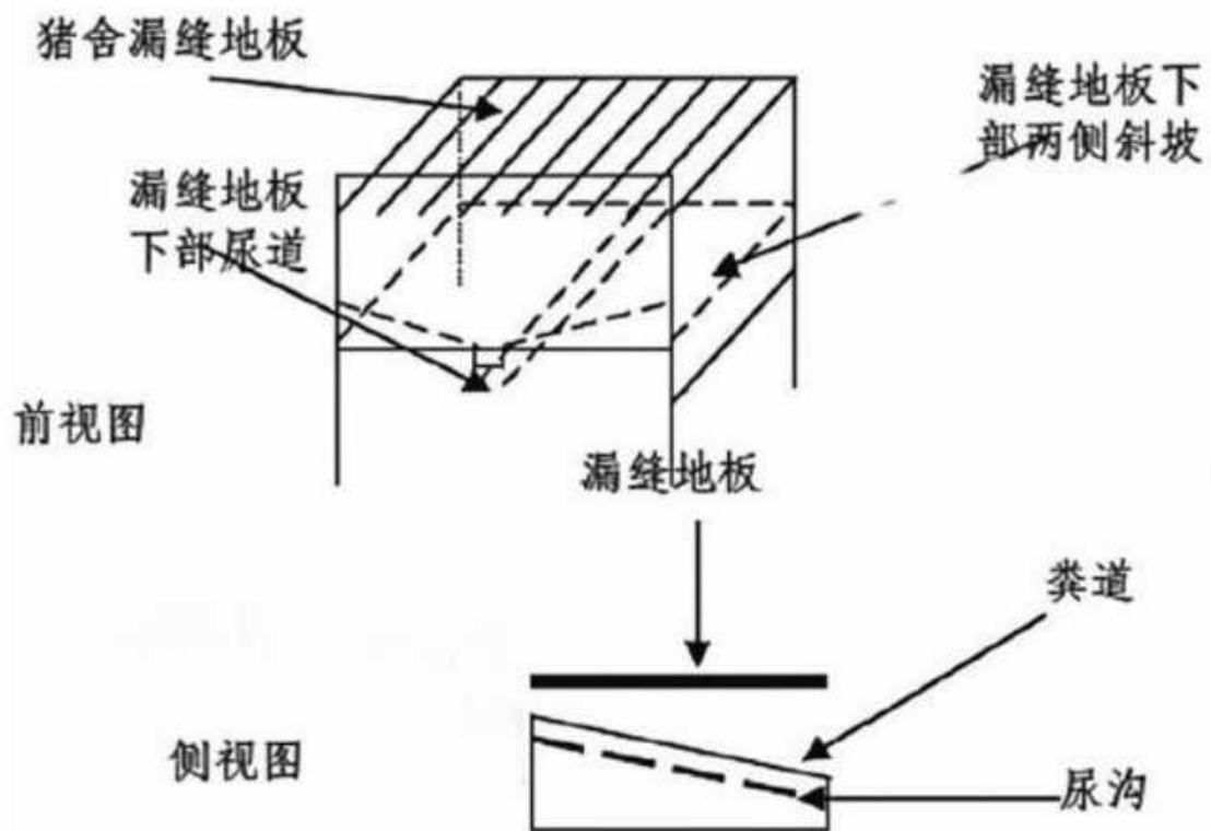
图 3.1-3 猪舍地板结构示意图
