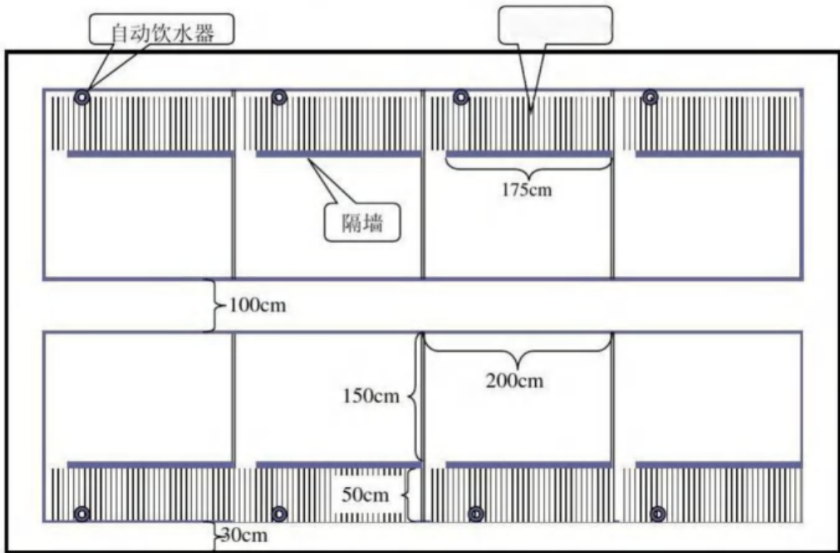
图 3.1-6 猪舍（保育舍、公猪舍）结构示意图
