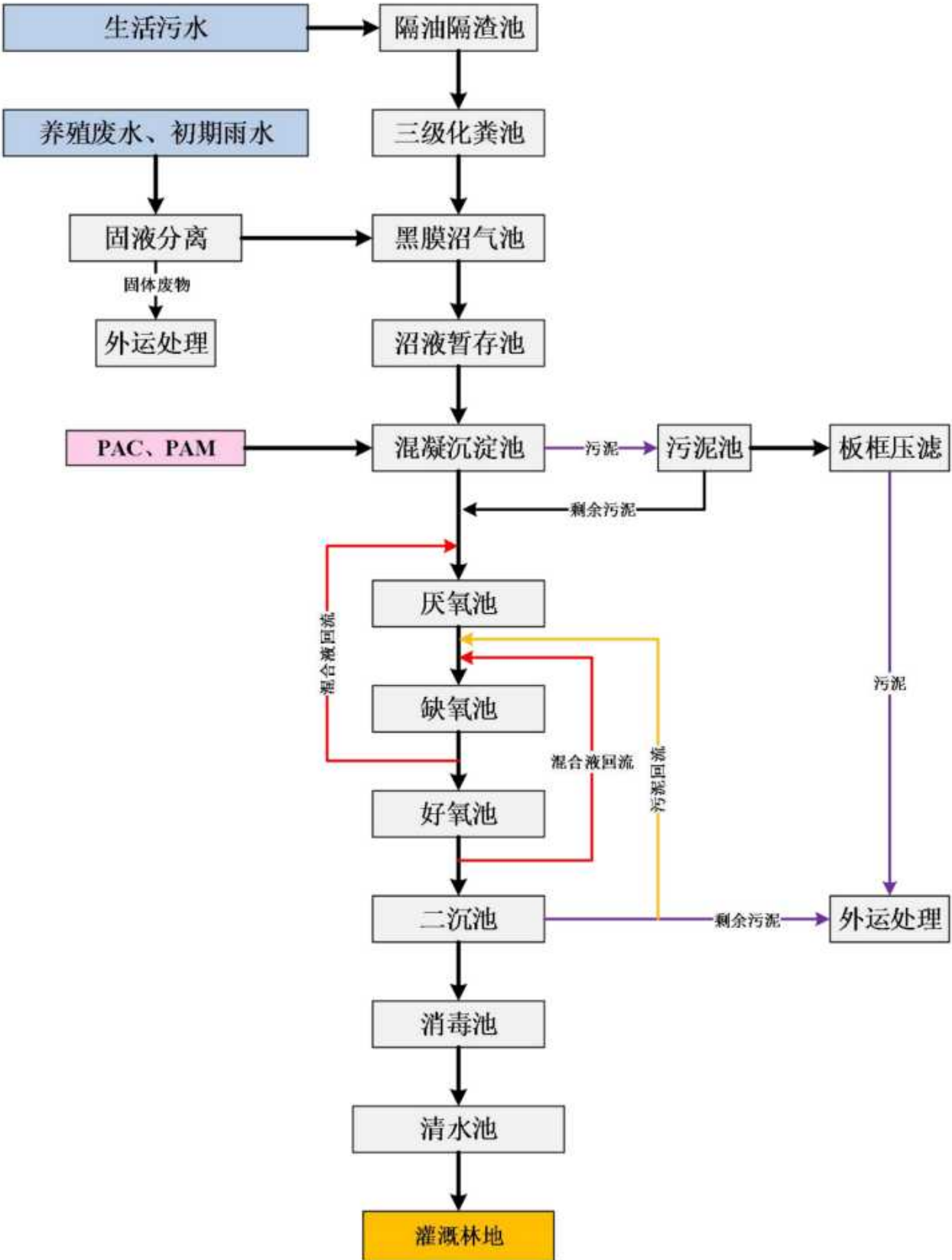
图 8.1-1 自建污水治理设施工艺流程图
