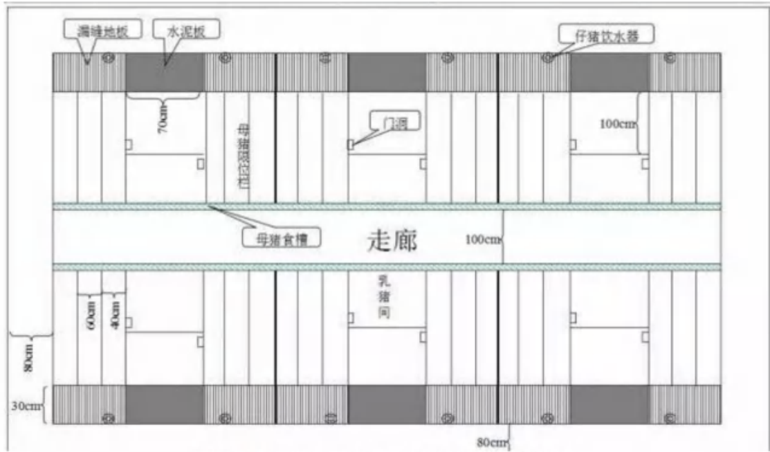
图 3.1-5 猪舍（产房、空怀舍）结构示意图
