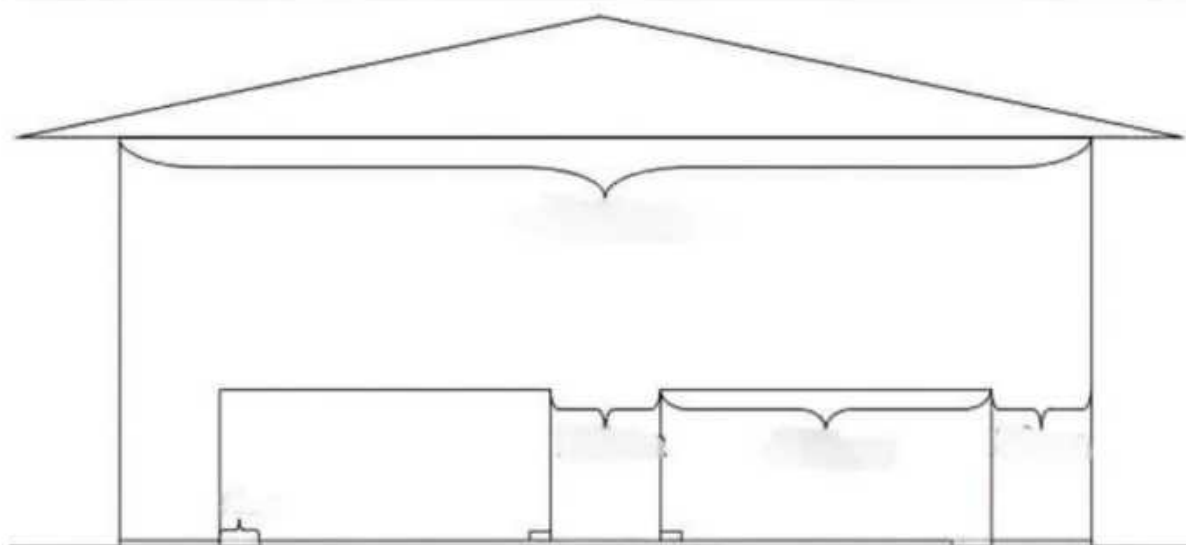
图 3.1-4 猪舍（空怀舍、保育舍、产房、公猪舍）立式结构示意图
